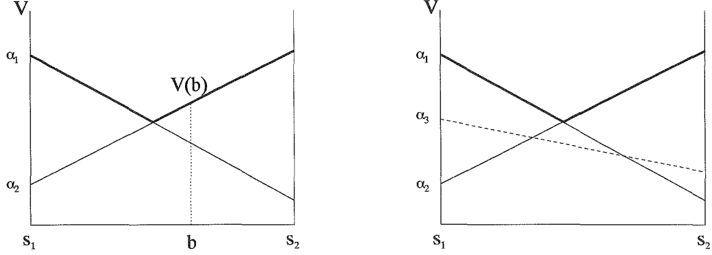
FIG. 1.2 – La fonction de valeur d'un POMDP à deux états s_1 et s_2 . L'action associée au vecteur \alpha_2 correspond à l'action optimale en b . Le vecteur \alpha_3 est entièrement dominé et peut être supprimé sans affecter la représentation de la fonction de valeur optimale.
