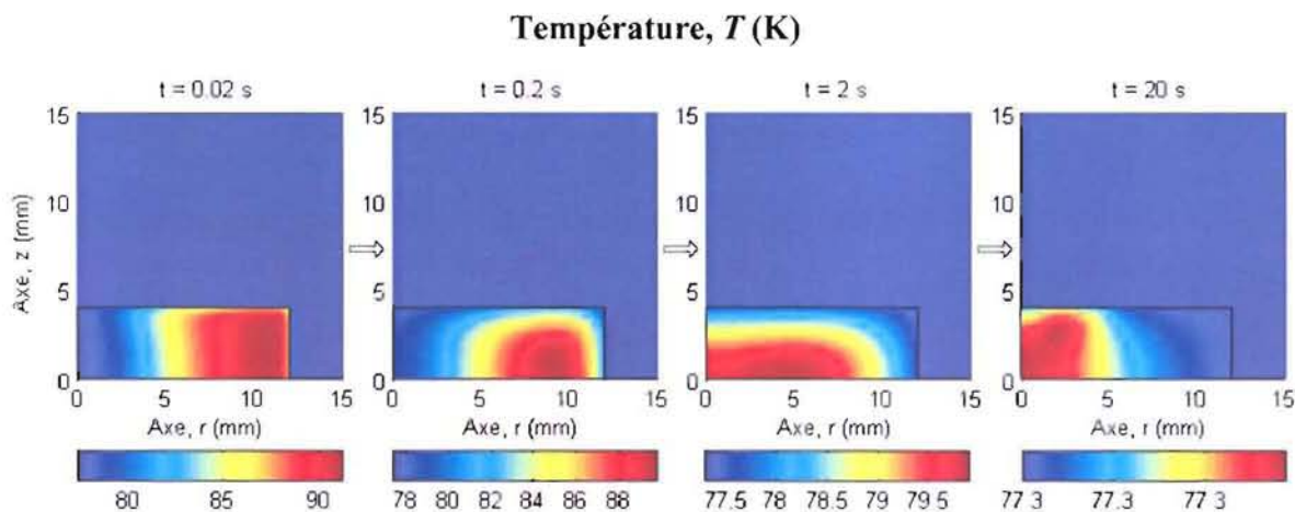
Figure 4.8 : Evolution de la température dans la pastille « 8-0-24 » avec la loi de comportement E-J-T pour \tau = 0.001 s et B_m = 5 T .
