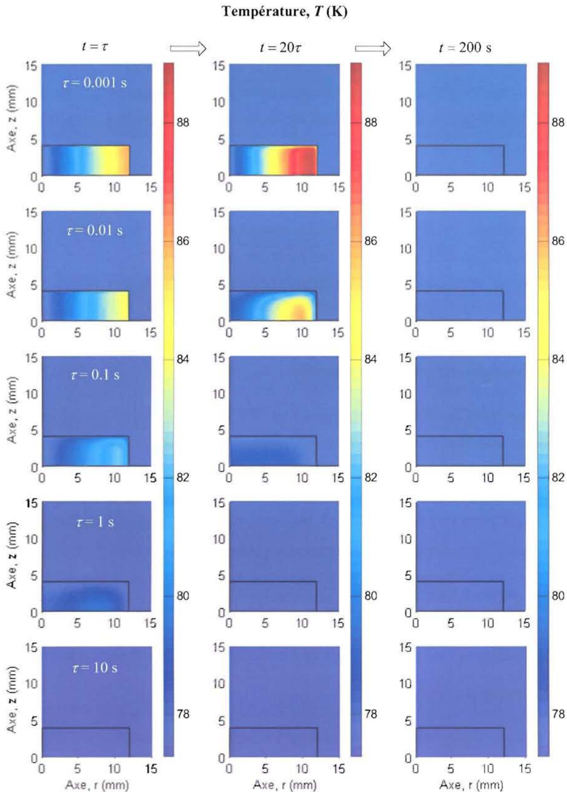
Figure 4.13 : Profils de température dans la pastille « 8-0-24 » à différents instants pour B_m = 5 \text{ T} et des valeurs de \tau comprises entre 0.001 et 10 s avec la loi de comportement « E - J - B - T ».
