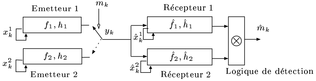
FIG. 3.10 – Modulation chaotique
