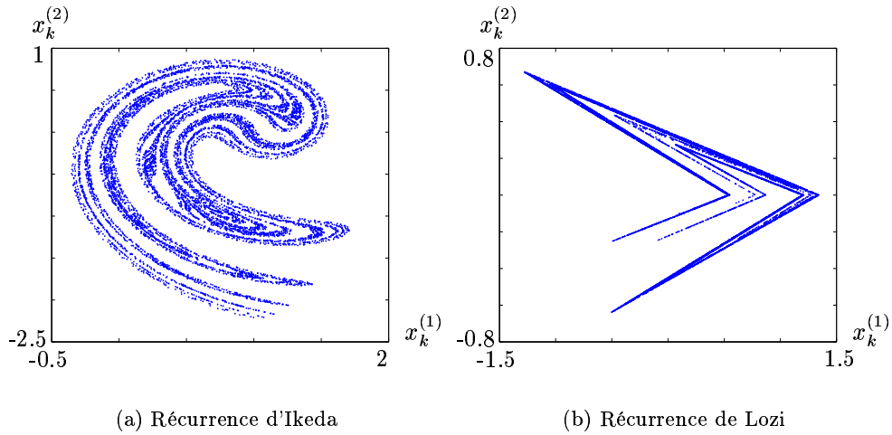
FIG. 1.9 – Attracteurs chaotiques
