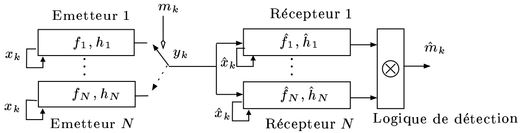
FIG. 2.6 – Modulation chaotique
