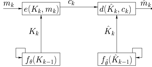
FIG. 2.3 – Chiffrement par flot synchrone
