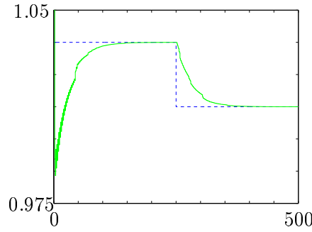
FIG. 4.4 – Trait pointillé : \theta_k , trait plein : \hat{\theta}_k
