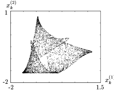
FIG. 1.8 – Exemple d'attracteur chaotique
