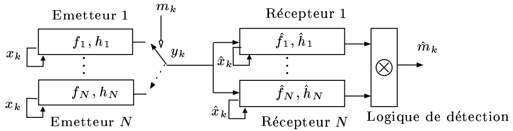
FIG. 3.1 – Modulation chaotique
