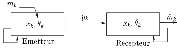
FIG. 4.1 – Modulation paramétrique
