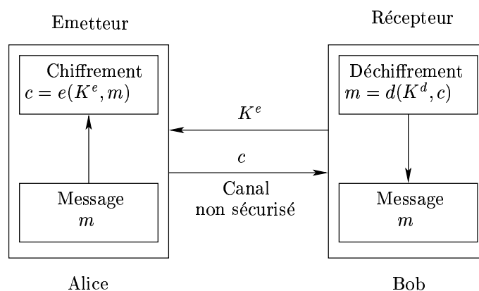
FIG. 2.1 – Chiffrement à clé publique
