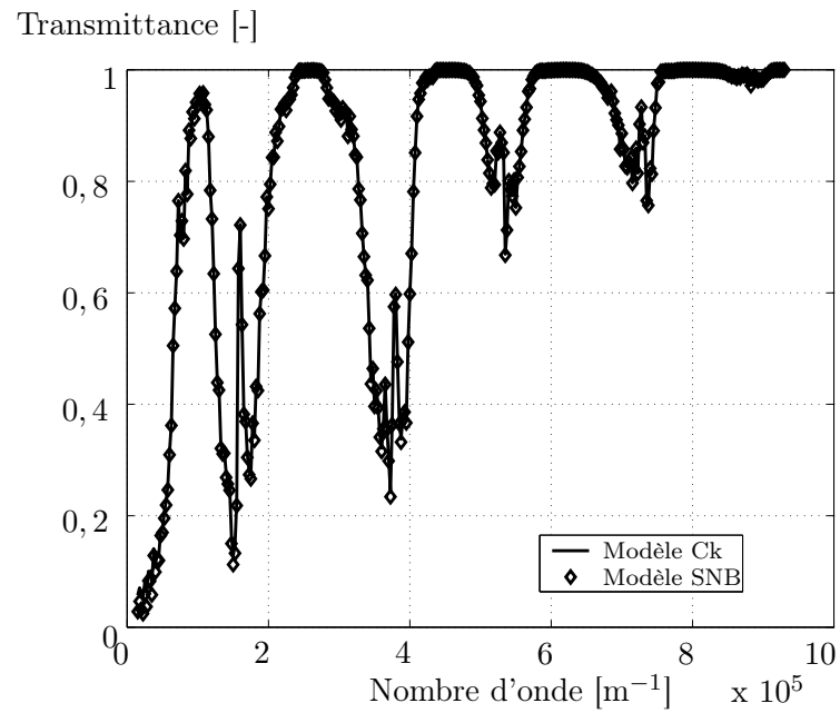
FIG. 4.7 – Transmittances d'un mélange gazeux \text{H}_2\text{O} et \text{N}_2
