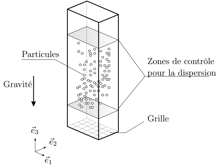
FIG. A.5 – Schéma de principe de la manipulation - Snyder & Lumley [Snyder et Lumley, 1971]
