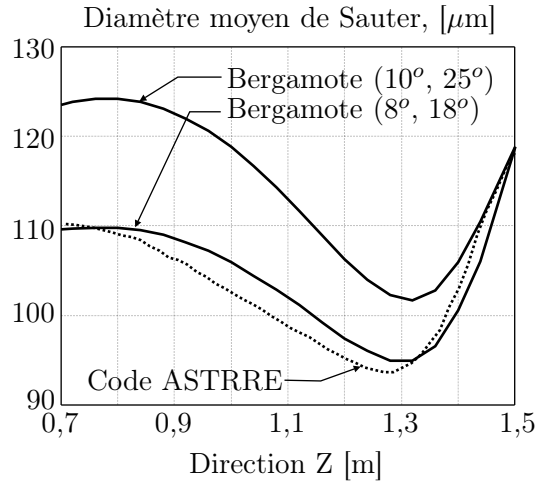
FIG. 7.21 – Évolution du D_{32} selon la direction Z
