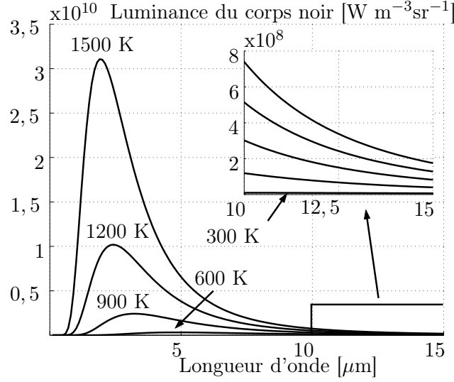
FIG. C.3 – Évolution de la luminance du corps noir en fonction de la longueur d'onde et de la température du corps
