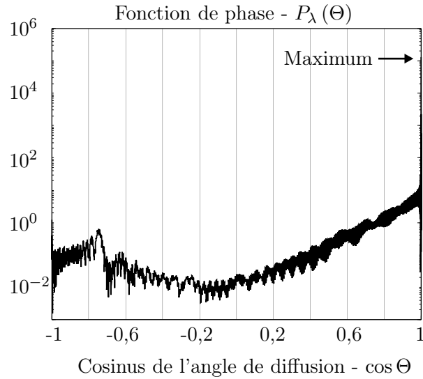
FIG. 6.2 – Représentation de la fonction de phase pour la TP 400 067 à 1,5 bars pour la longueur d'onde de 1,1 \mu m
