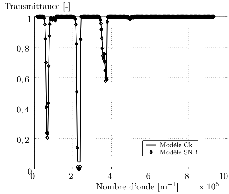
FIG. 4.6 – Transmittances d'un mélange gazeux \text{CO}_2 et \text{N}_2
