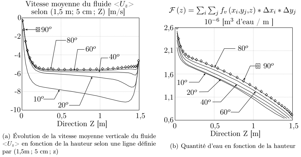
FIG. 8.20 – Comparaison sur la dynamique de la rampe
