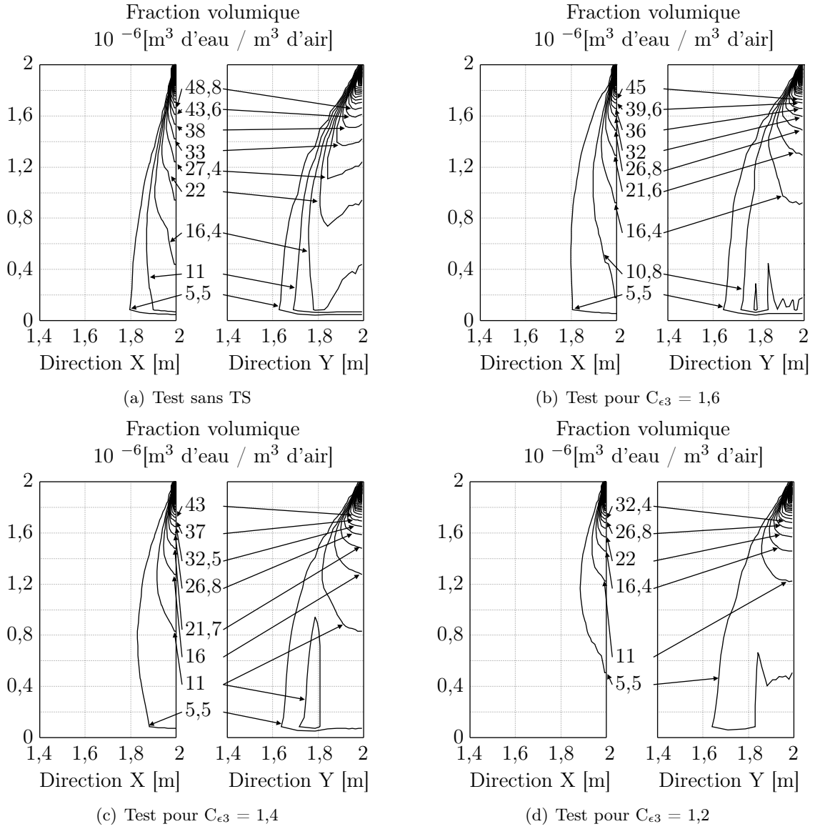
FIG. 7.35 – Comparaison des différentes fractions volumiques
