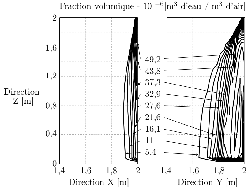
FIG. 7.30 – Fraction volumique en gouttes dans le spray sans dispersion turbulente
