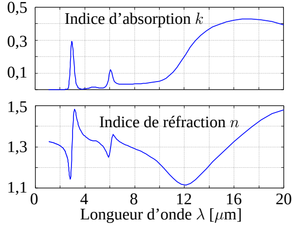
FIG. 4.1 – Indice d'absorption et de réfraction de l'eau d'après Hale et al. [Hale et Query, 1973]
