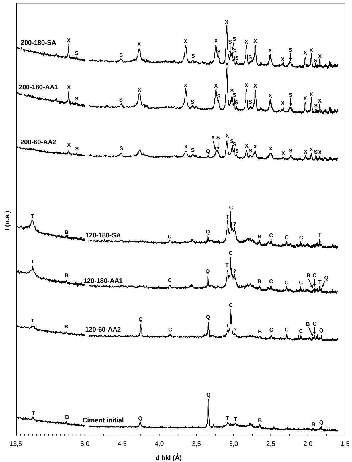
Figure 2. Diffractogrammes de rayons-X sur les ciments initiaux et vieillis.
