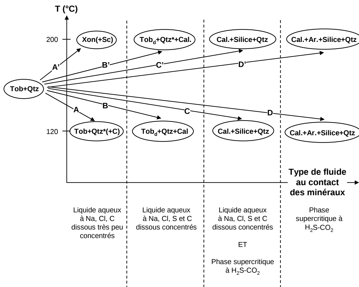
Figure 2. Stabilité des phases minérales d'un ciment de puits pétrolier à farine de silice, en fonction de la température et de la phase fluide coexistante à 500 bar.
