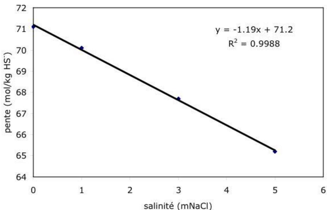
Figure 7. Evolution de la pente de la droite de calibrage Raman du sulfure d'hydrogène dissous en fonction de la salinité.
