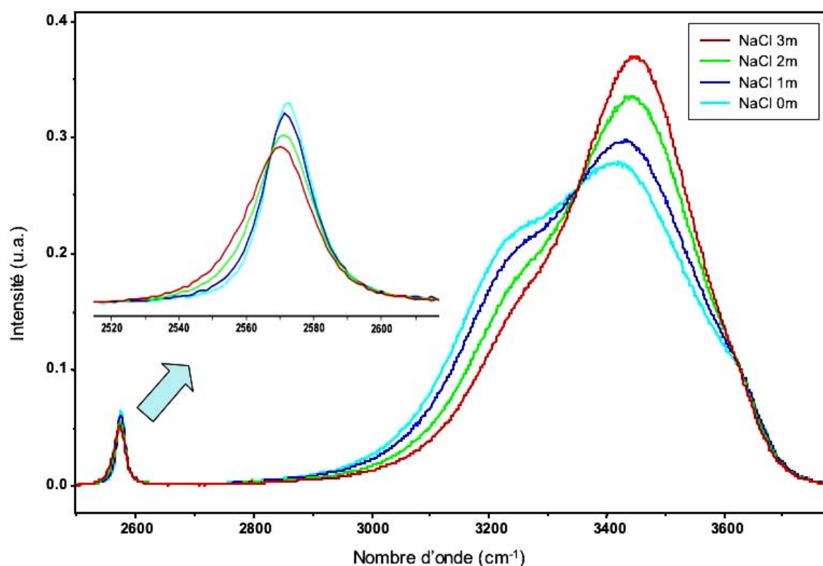
Figure 4. Spectres Raman du sulfure d'hydrogène ( \text{mHS}^- = 0,55 ) et de l'eau pour différentes chlorinités.
