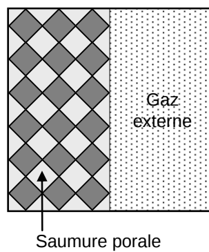
Figure 1. Géométrie des trois systèmes à 25°C, avant expérimentation.
