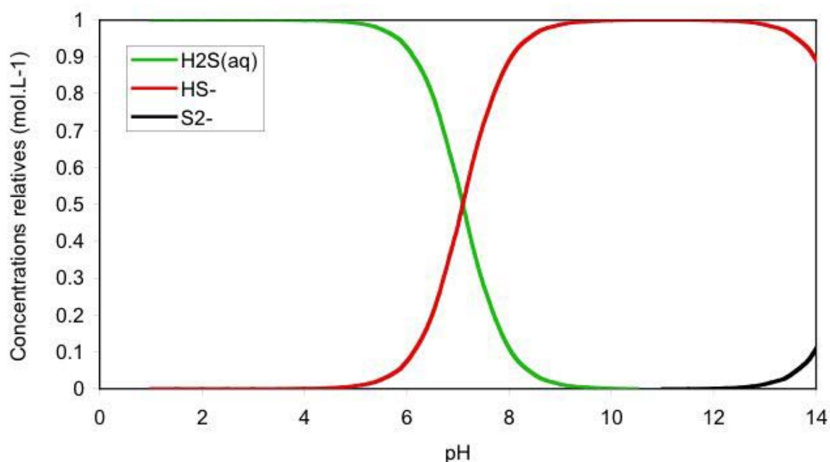
Figure 1. Diagramme de stabilité des espèces dissoutes du soufre dans l'eau à 25°C.
