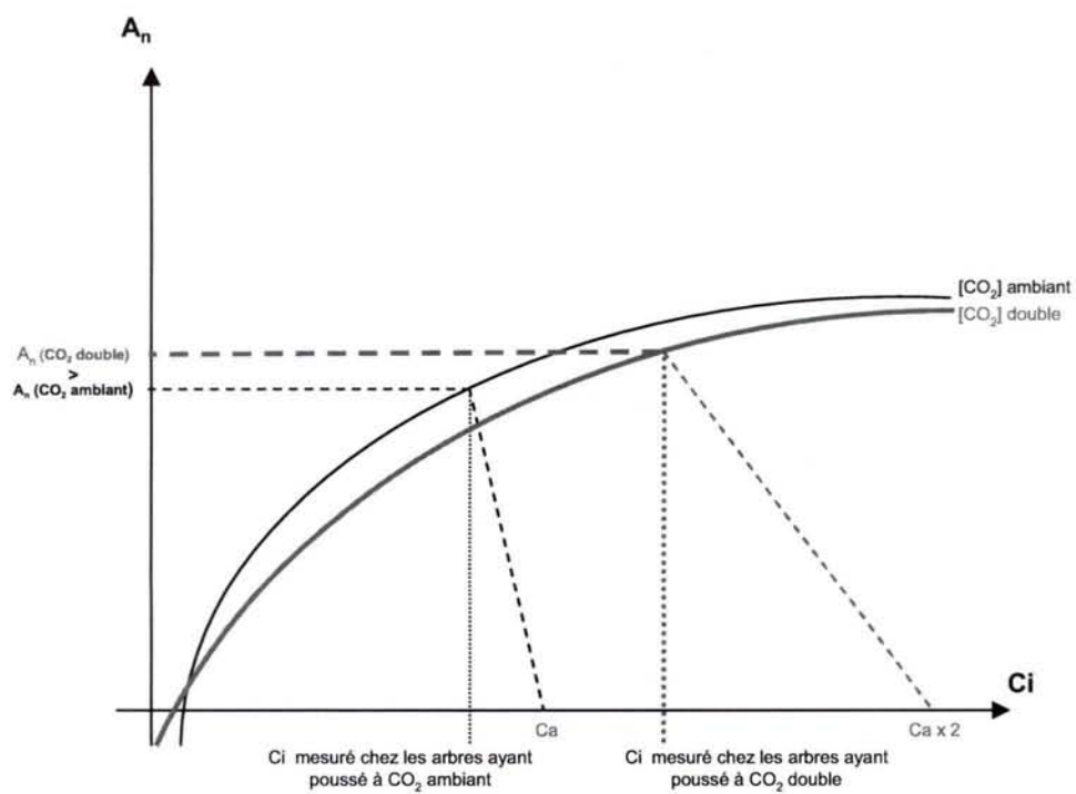
Figure 33 : Modèle de réponse de la relation A/C_i pour des concentrations en \text{CO}_2 de mesure ambiante ( \text{Ca} ) et doublée ( \text{Ca} \times 2 ) (d'après le modèle de Farquhar et al. , 1980; Webber et al. , 1994 ; Besford et al. , 1998).
