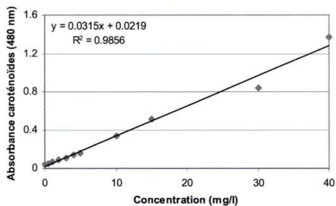
Figure 15: Courbes étalons de dosage de la chlorophylle a (A), la chlorophylle b (B) et des caroténoïdes (C) au DMSO.
