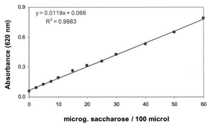
Figure 14: Courbe étalon de dosage du Saccharose à l'anthrone.
