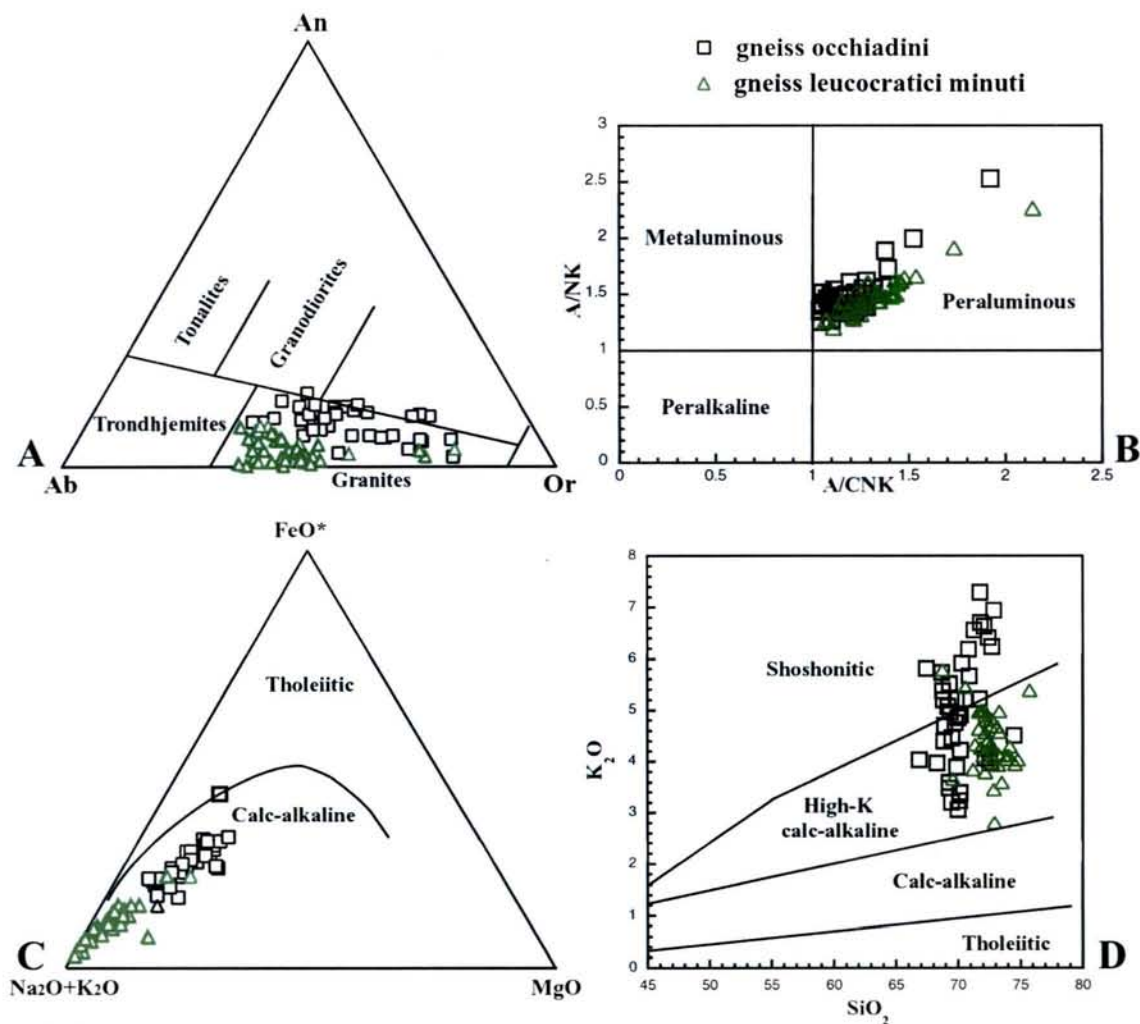
Fig. 3.1 Diagrammi mostrandoti il carattere granitico, peralluminoso e calc-alcino alto in K 2 O degli gneiss occhiadini (Diagrams showing granitic, peraluminous and K-rich calc-alkaline affinity of augen gneisses)
