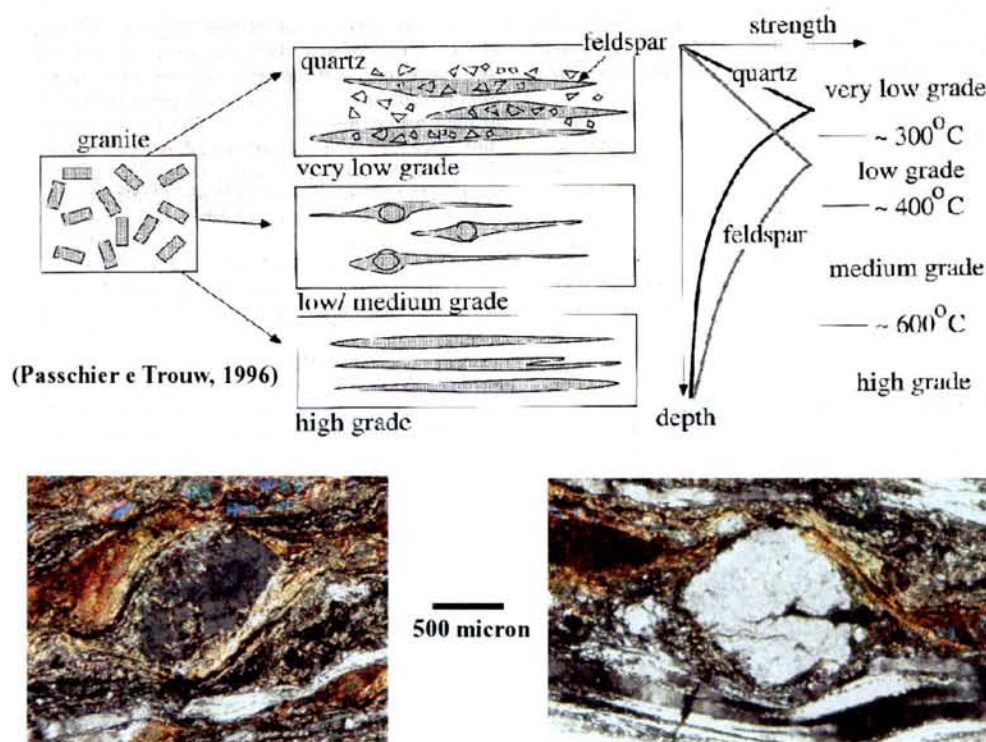
Fig.2.3 - Formazione delle strutture core and mantle (Core and mantle structure formation)
