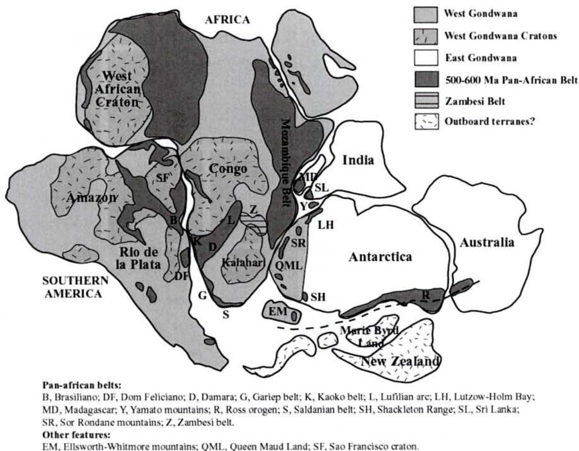
Fig.8.2 - Ricostruzione del supercontinente Gondwana (Grunow et al., 1996, modif.) (Gondwana supercontinent reconstruction)
