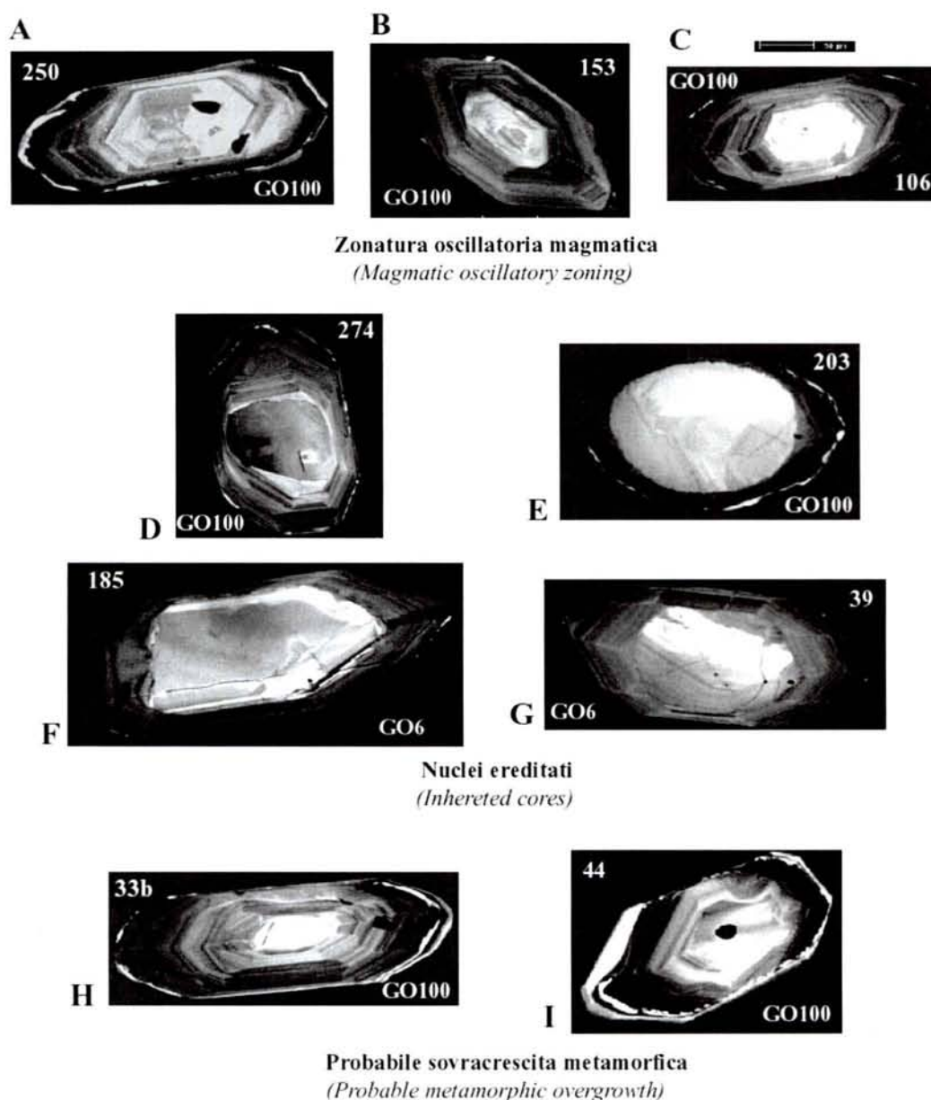
Fig.6.1 - Principali tipologie di zonature osservate nei cristalli di zircone dei cinque campioni datati (Main typologies of zoning observed in zircon crystals of five dated sample)
