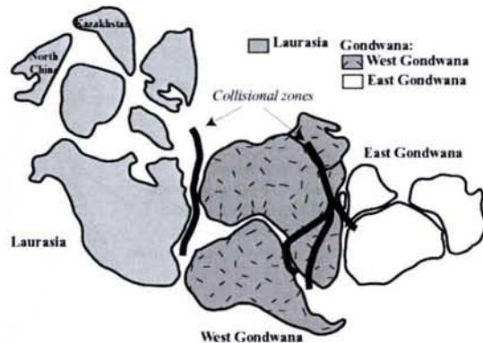
Fig. 8.3D - Riorganizzazione di Rodinia nel supercontinente Pangea (700-500 Ma) (Reorganization of Rodinia to Pangea; Mallard et al., 1997, modif.)
