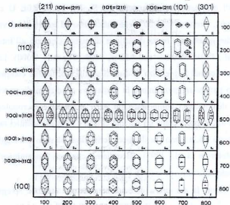
Fig. 4.1 Diagramma classificativo dei cristalli di zircone su base morfologica (Pupin et al., 1972) (Morphological classification of zircon crystals)
