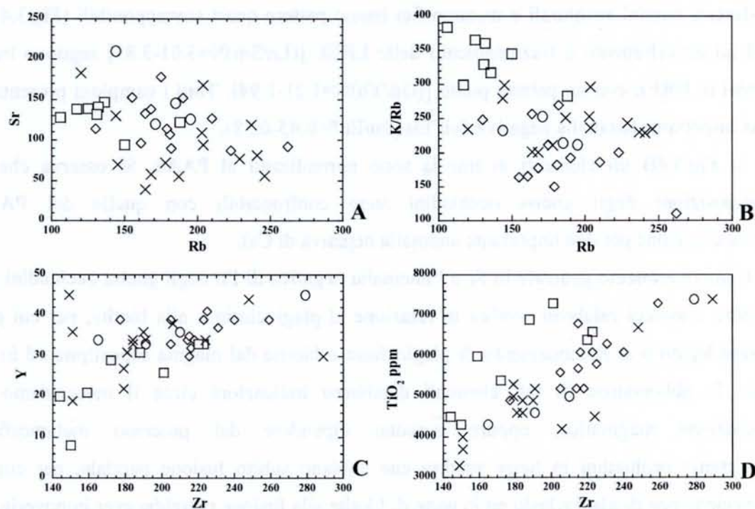
Fig.3.3 - Variazione di alcuni elementi in traccia negli gneiss occhiadini (Rb vs Sr, Rb vs K/Rb, Zr vs Y, Zr vs \text{TiO}_2 ppm) (Trace element variation in augen gneisses)
