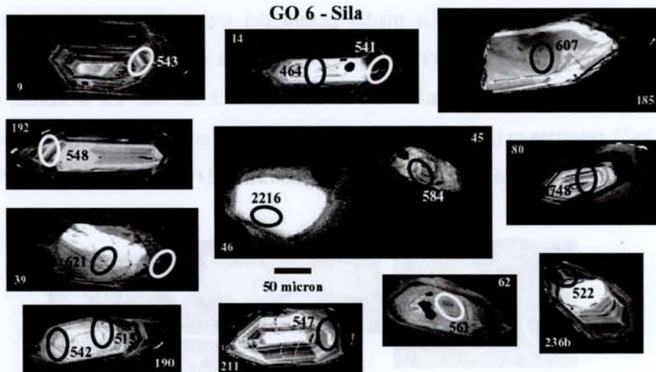
Fig.6.3A - Cristalli di zirconio datati alla microsonda ionica. Le ellissi indicano la posizione dello spot. (Zircon crystals dated by the microprobe. The ellipses represent the spot position).
