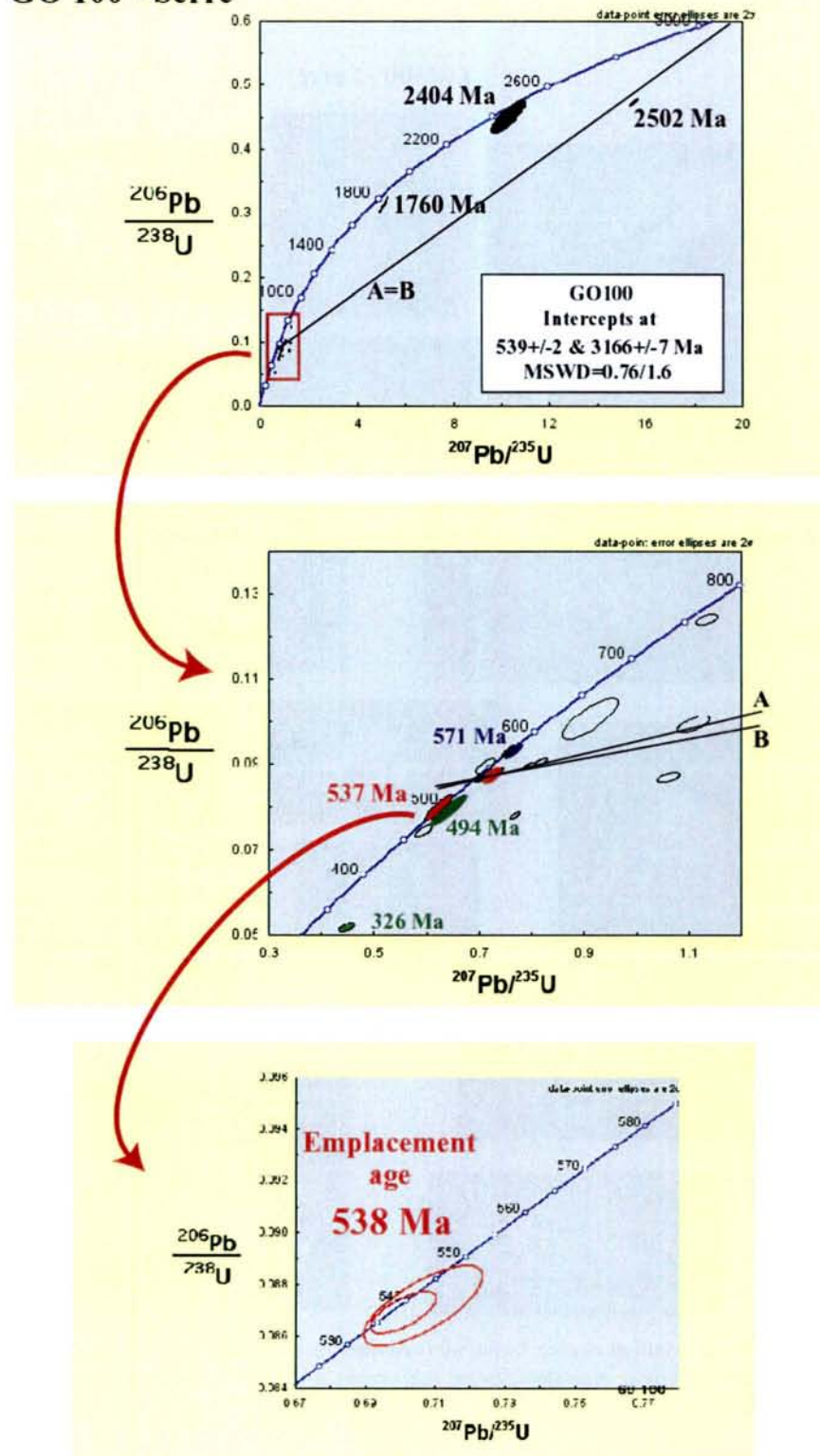
Fig.6.5B - Diagrammi \frac{^{207}\text{Pb}}{^{235}\text{U}} - \frac{^{206}\text{Pb}}{^{238}\text{U}} in cui sono rappresentate le determinazioni effettuate (Le dimensioni delle ellissi sono proporzionali all'errore analitico) (Diagrams \frac{^{207}\text{Pb}}{^{235}\text{U}} - \frac{^{206}\text{Pb}}{^{238}\text{U}} representing the performed determinations. Ellipse dimensions are proportional to the analytical error)
