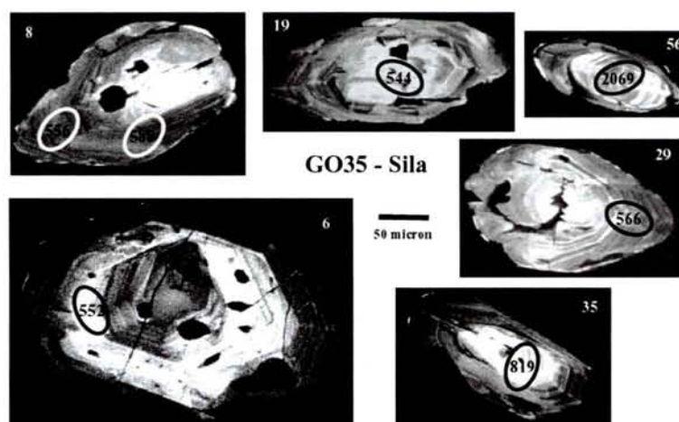
Fig.6.4A - Cristalli di zirconio datati alla microsonda ionica. Le ellissi indicano la posizione dello spot. (Zircon crystals dated by the microprobe. The ellipses represent the spot position).
