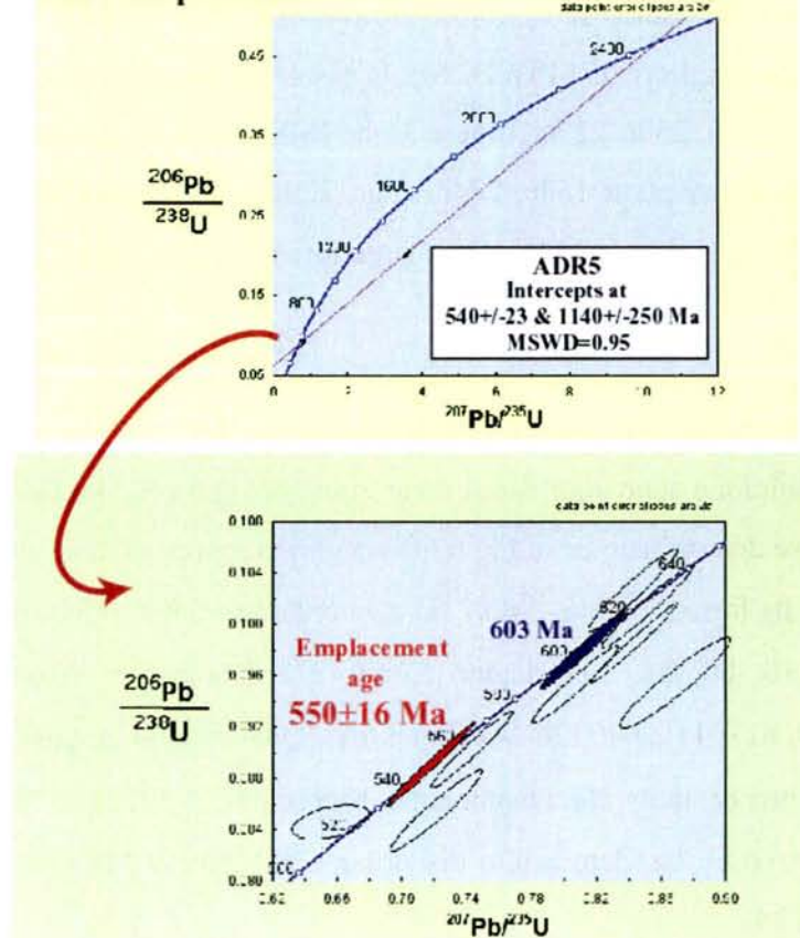
Fig.6.6B - Diagrammi ^{207}\text{Pb}/^{235}\text{U} - ^{206}\text{Pb}/^{238}\text{U} in cui sono rappresentate le determinazioni effettuate (Le dimensioni delle ellissi sono proporzionali all'errore analitico) (Diagrams ^{207}\text{Pb}/^{235}\text{U} - ^{206}\text{Pb}/^{238}\text{U} representing the performed determinations. Ellipse dimensions are proportional to the analytical error)
