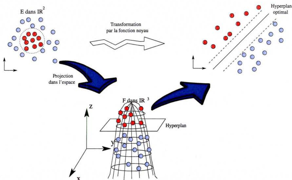
FIG. 5.8 – Représentation du pré-traitement sur un jeu d'échantillons non séparable linéairement. Les échantillons ne sont pas linéairement séparables. Le pré traitement consiste à projeter les données dans un nouvel espace de représentation grâce à la fonction (le noyau) qui pré-traite les données. Dans ce nouvel espace de représentation, la feature space , les données projetées sont linéairement séparables.
