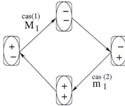
FIG. 10.6 – Graphe de transition partiel pour un système à deux variables. M_1 représente le passage par un pic de maximum pour la variable x_1 . m_1 représente le passage par un minimum pour la variable x_1 .
