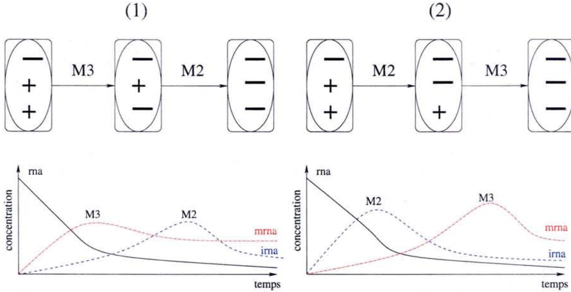
FIG. 10.8 – Comportement qualitatif du modèle de régulation au site A3. Pour une initialisation correspondant à une concentration d'ARN immatures ( rna ) seul, il existe deux comportements qualitatifs possibles. (1) correspond à un pic de production (M3) de ARN mature ( mrna ) suivi d'un pic (M2) d'ARN intermédiaires ( irna ). (2) correspond à un pic de production (M2) d'ARN intermédiaires ( irna ) suivi d'un pic (M3) de ARN matures ( mrna ).
