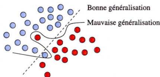
FIG. 5.4 – Illustration d'un effet de sur-apprentissage. La fonction f en trait continu ne fait aucune erreur d'apprentissage mais ne généralise pas bien par rapport à la fonction f en trait pointillé qui fait deux erreurs mais qui permet de mieux généraliser.
