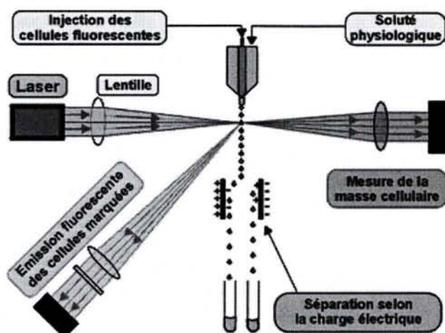
Figure C12 : description d'un appareillage de cytométrie de flux.
