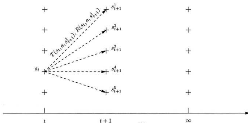
FIG. 2.5 – Comment fonctionne le principe de Bellman.
