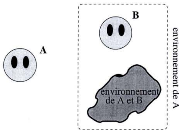
FIG. 2.7 – Ici, l'agent A perçoit B comme faisant partie de l'environnement. Donc si le comportement de B évolue, il en est de même de la fonction de transition \mathcal{T} (vue par A).
