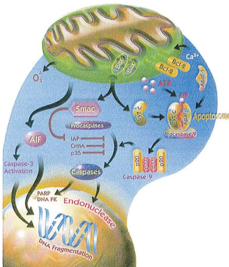
Figure 17 Représentation schématique des principaux mécanismes moléculaires du processus apoptotique, impliquant Bax, Bcl-2, les caspases initiateurs et effectrices et l'AIF (« apoptosis inducing factor »)
