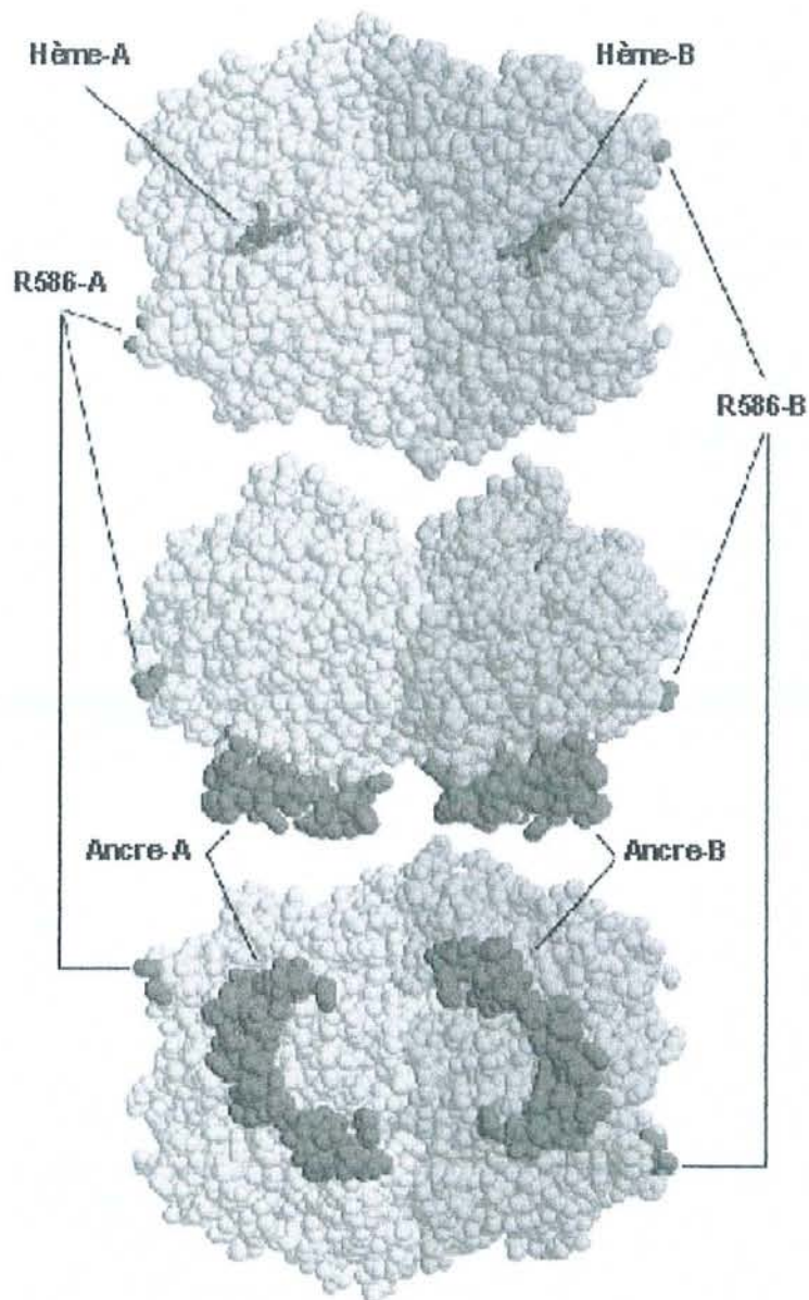
Figure 4 Structure cristallographique d'un dimère de COX-1 ovine, solubilisé par du détergent. Trois parties sont localisées : 1) le groupement hème prosthétique ; 2) le dernier résidu aa identifié, Arg586 (R586); 3) le domaine de liaison à la membrane (d'après Guo et Kulmacz, 2000).
