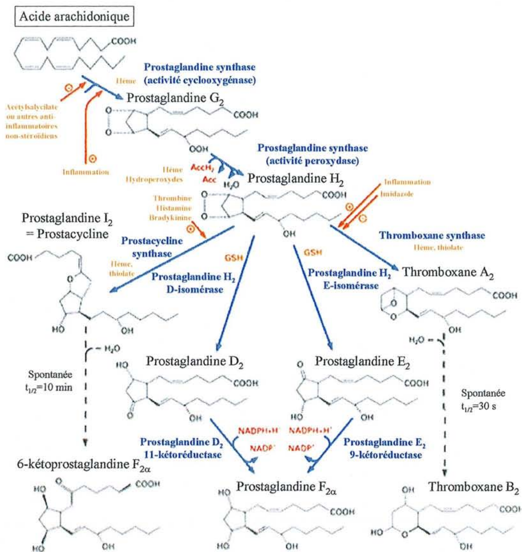
Figure 12 Biosynthèse des eicosanoïdes à partir de l'AA
