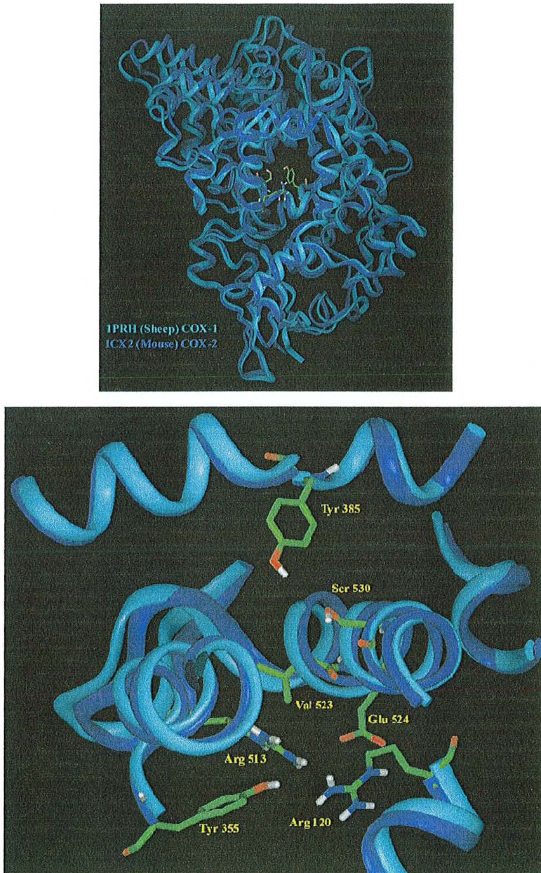
Figure 5 Alignement des structures en ruban de COX-1 ovine (bleu) et de COX-2 murine (violet) et agrandissement du site actif pour localiser les aa importants
