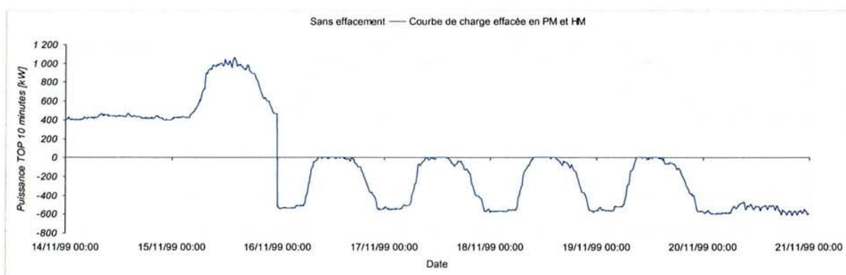
Figure 5-50 – Tarif A Mod TLU, optimisation par effacement selon la conduite 2
