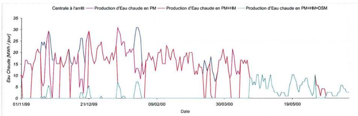
Figure 5-26 – Conduite de la centrale en A Mod, appoint de charge d'Eau Chaude demandée en chaufferie
