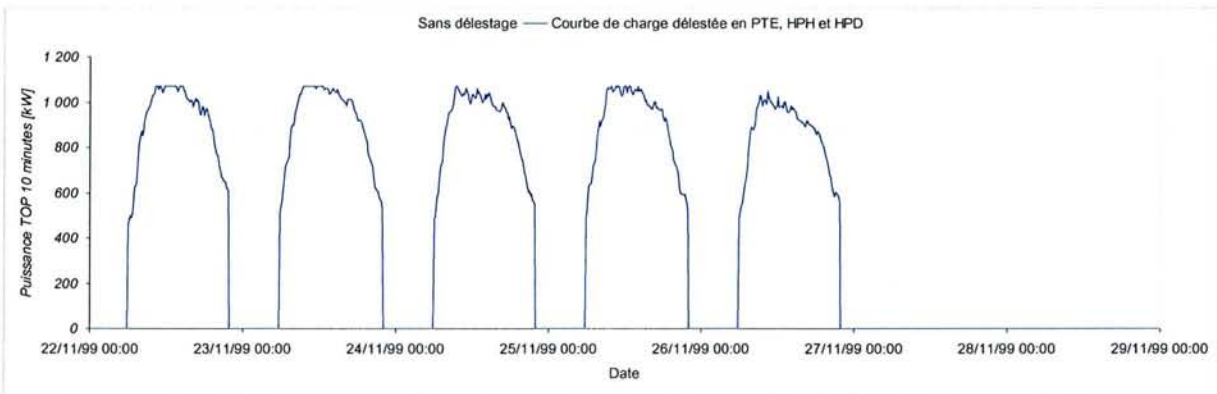
Figure 4-18 – Tarif A8 Base LU, optimisation par délestage dans les tranches PTE, HPH & HPD
