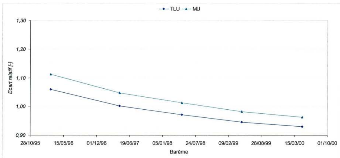
Figure 3-41 – A8 EJP, sensibilité des factures globales par rapport aux fluctuations des barèmes de prix
