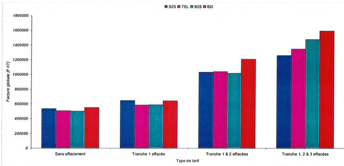
Figure 5-23 – Conduite avec le Tarif A8 EJP, factures globales des tarifs gaz selon les conduites adoptées
