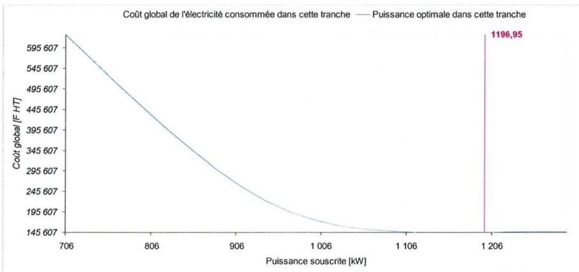
Figure 3-24 – Tarif A8 EJP Version TLU, puissance souscrite optimale dans la tranche JA
