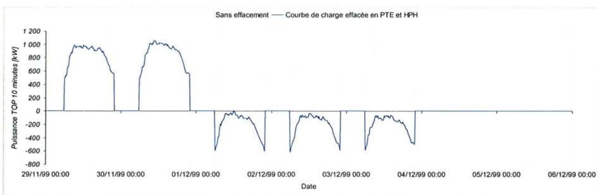
Figure 5-37 – Tarif A8 Base LU, optimisation par effacement selon la conduite 2
