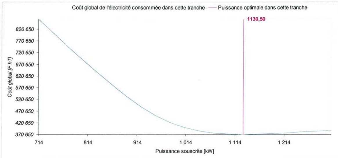
Figure 3-26 – Tarif A Mod. Version TLU, puissance souscrite optimale dans la tranche HM
