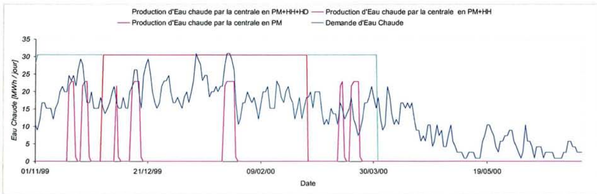
Figure 5-15 – Conduite de la centrale en A8 EJP, distribution des besoins et production d'Eau Chaude
