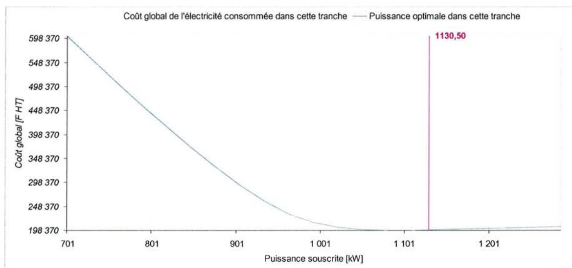
Figure 3-21 – Tarif A8 EJP Version TLU, puissance souscrite optimale dans la tranche HD
