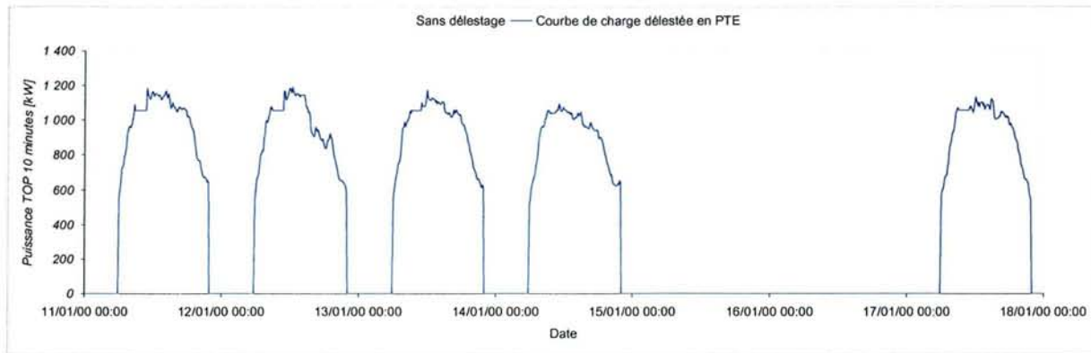
Figure 4-16 – Tarif A8 Base LU, optimisation par délestage dans la tranche PTE
