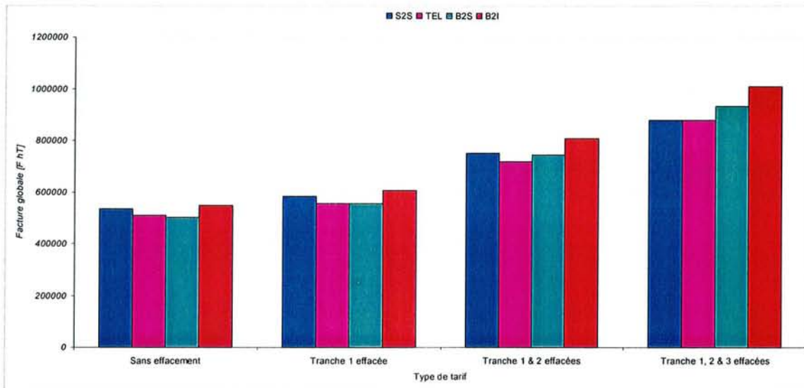
Figure 5-14 – Conduite avec le Tarif A8 Base, factures globales des tarifs gaz selon les conduites adoptées
