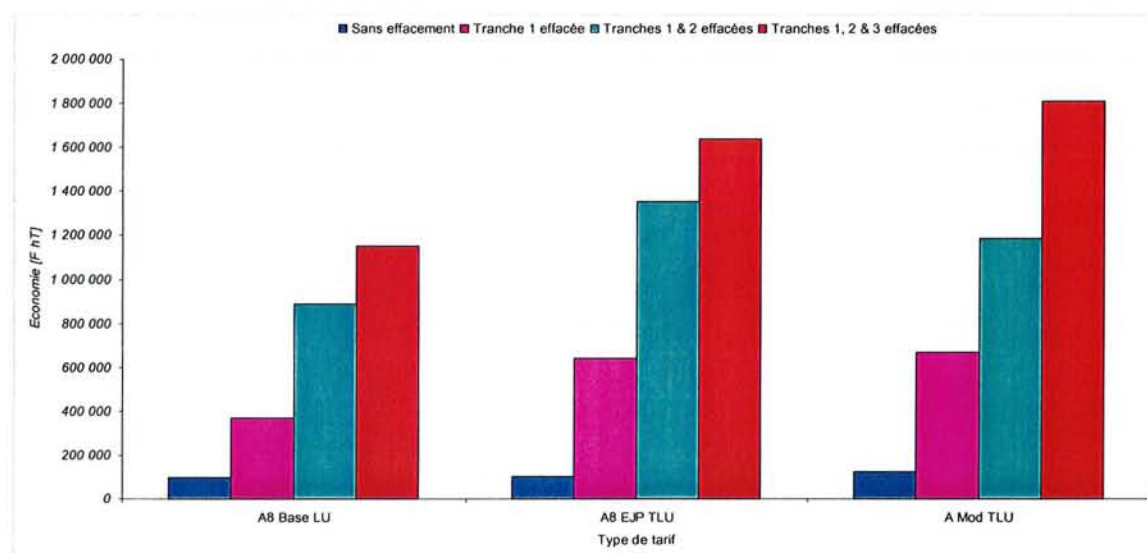
Figure 5-54 – Economie absolue par rapport à la souscription actuelle du consommateur
