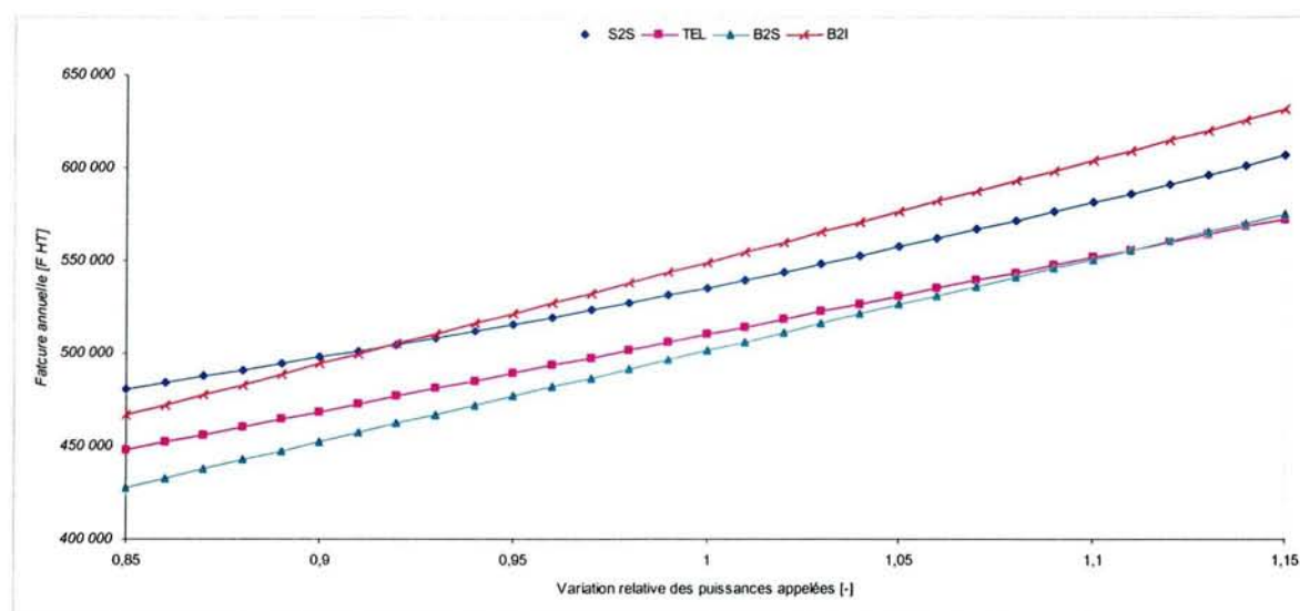
Figure 3-7 – Influence de l'évolution des puissances appelées sur la facture globale
