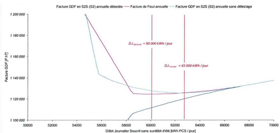
Figure 5-31 – A Mod conduite 3, facture S2S optimale avec et sans délestage du Gaz par le Fioul
