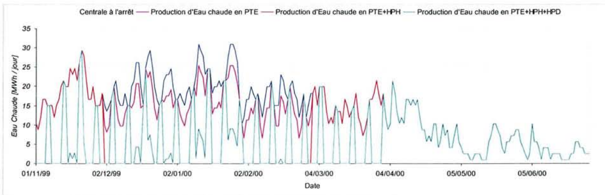
Figure 5-8 – Conduite de la centrale en A8 Base, appoint de charge d'Eau Chaude demandée en chaufferie
