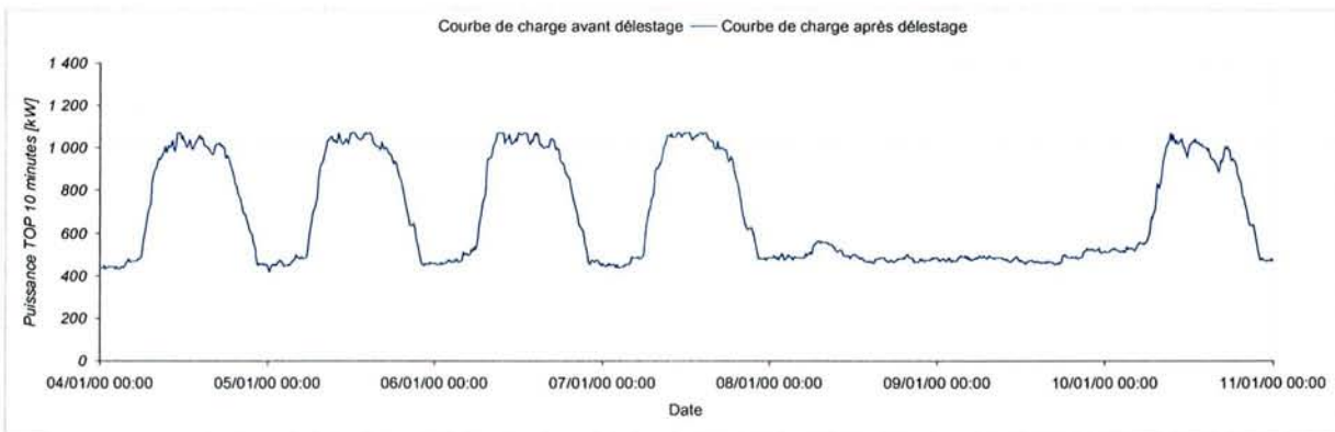
Figure 4-27 – Tarif A Mod TLU, tranche DSM délestée
