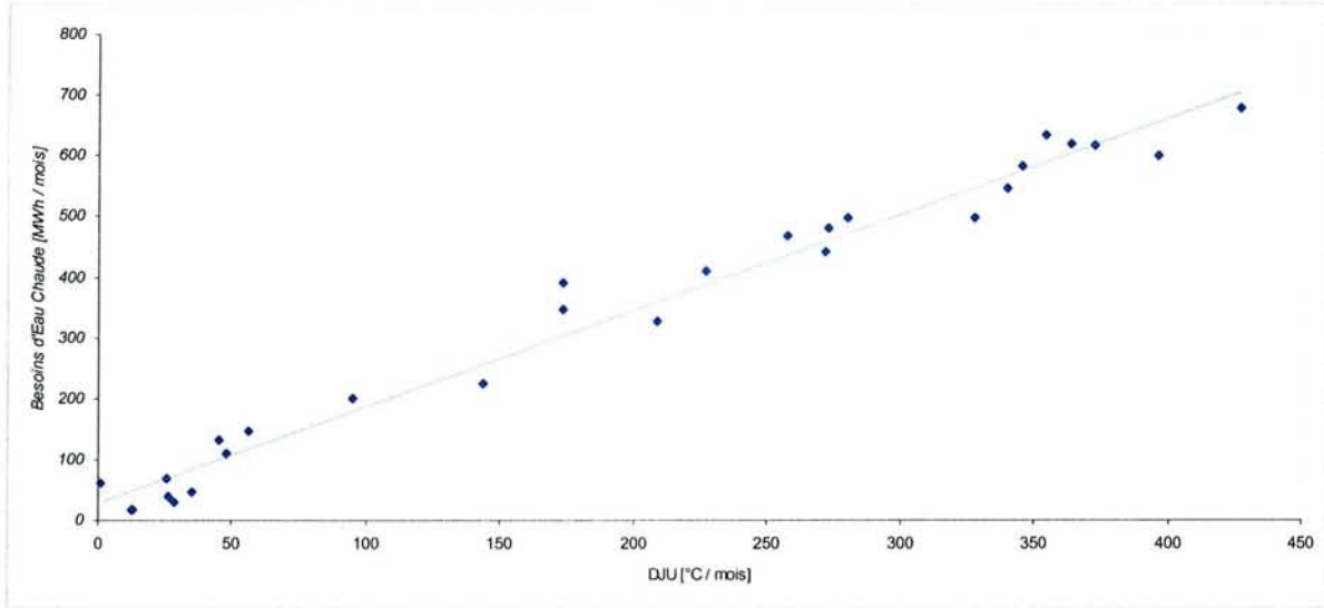
Figure 3-1 – Corrélation entre consommation d'eau chaude et DJU
