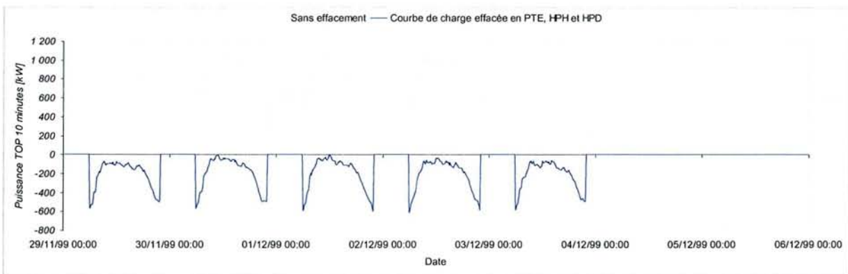
Figure 5-38 – Tarif A8 Base LU, optimisation par effacement selon la conduite 3
