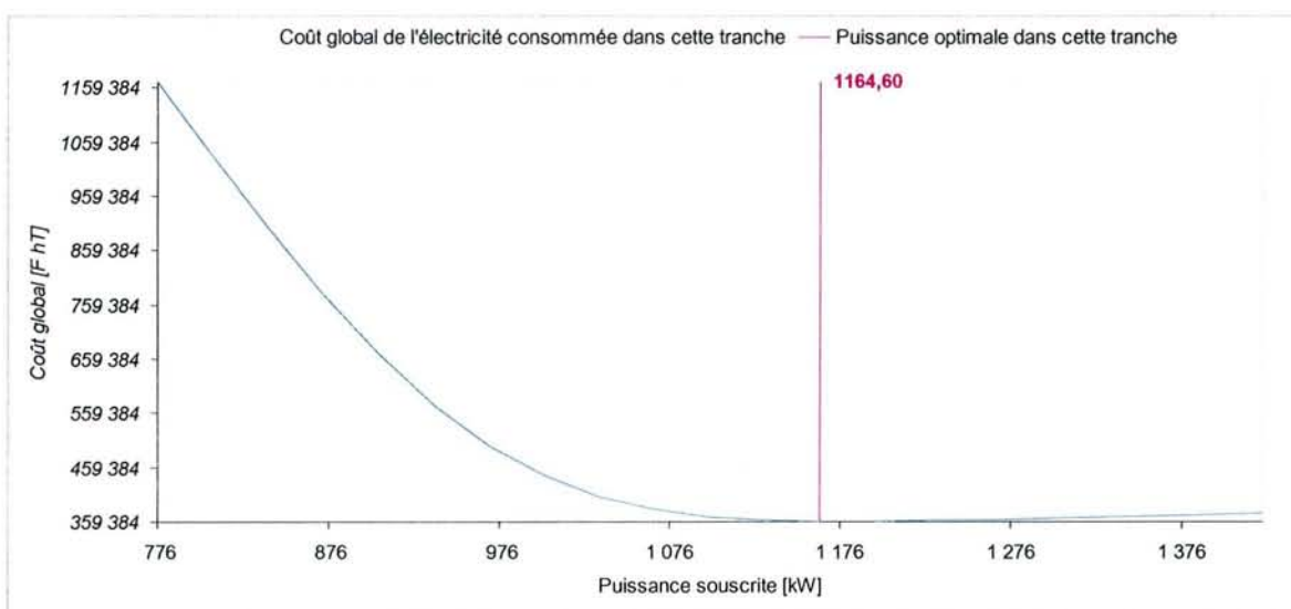
Figure 3-28 – Tarif A Mod. Version TLU, puissance souscrite optimale dans la tranche SCM
