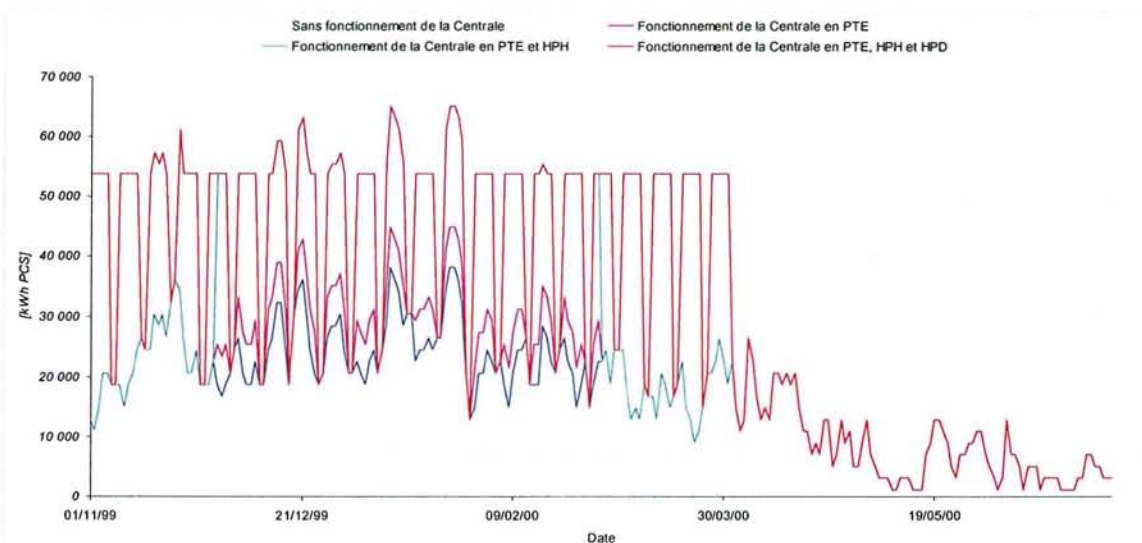
Figure 5-10 – Conduite de la centrale en A8 Base, distribution des appels globaux journaliers de Gaz
