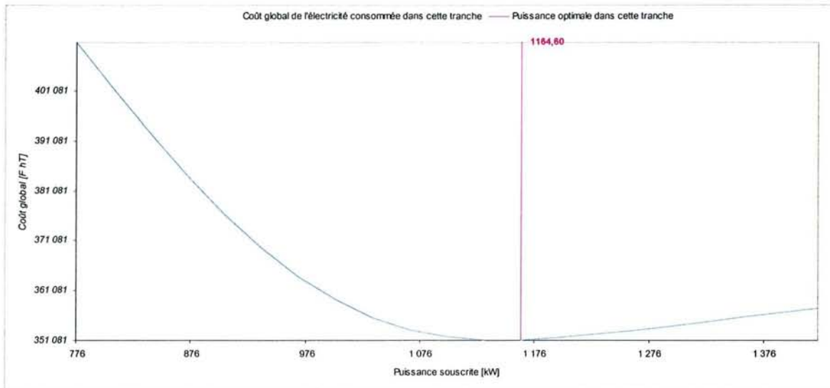
Figure 3-17 – Tarif A5 Base Version LU, puissance souscrite optimale dans la tranche HPE
