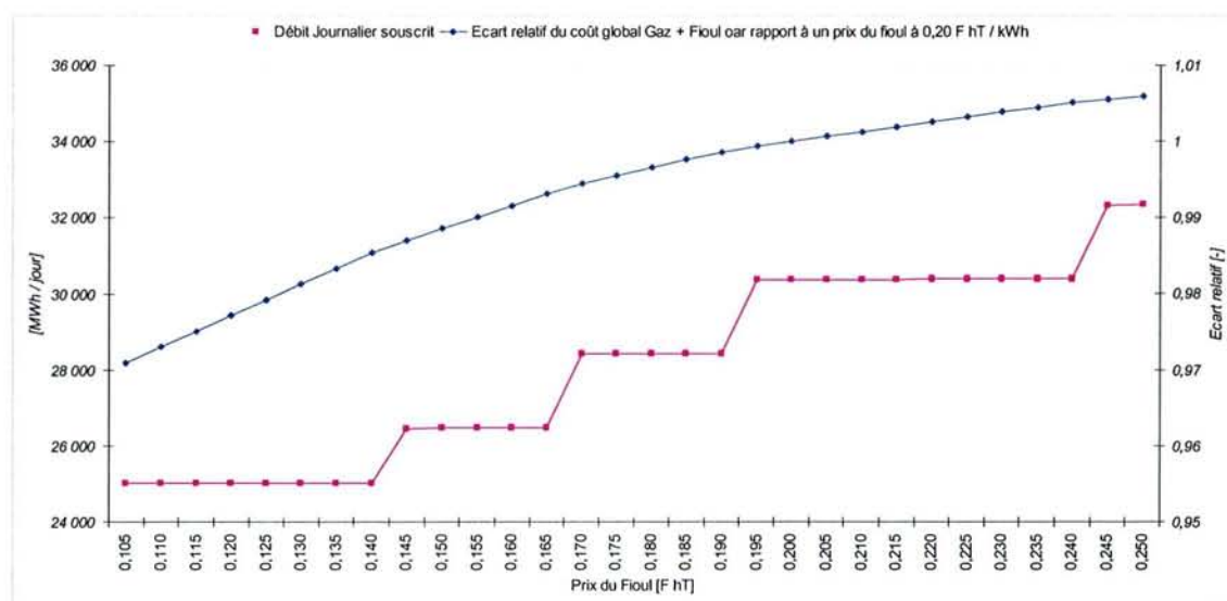
Figure 4-3 – Evolution du débit journalier et de la facture globale optimums en délestage Gaz / Fioul
