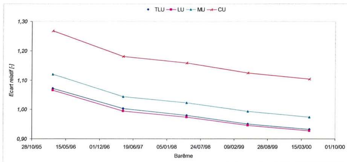
Figure 3-40 – A8 Base, sensibilité des factures globales par rapport aux fluctuations des barèmes de prix
