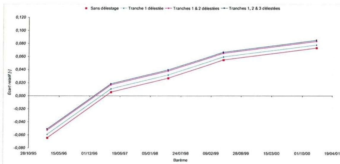
Figure 4-37 – A8 Base LU, sensibilité des factures délestées selon les fluctuations des barèmes de prix
