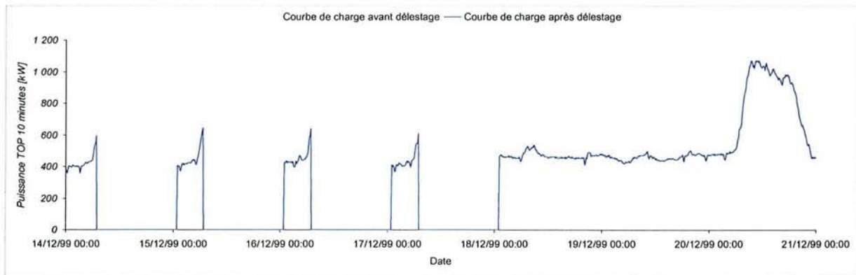
Figure 4-20 – Tarif A8 EJP TLU, tranche HH délestée
