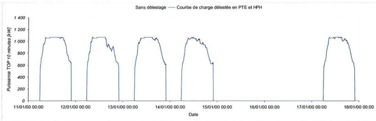
Figure 4-17 – Tarif A8 Base LU, optimisation par délestage dans les tranches PTE & HPH
