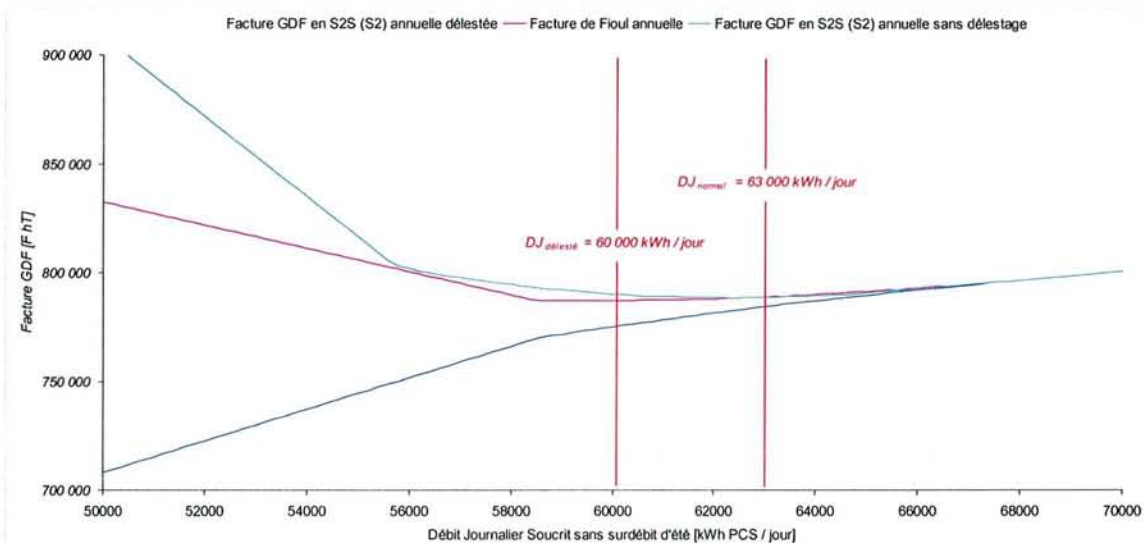
Figure 5-30 – A Mod conduite 2, facture S2S optimale avec et sans délestage du Gaz par le Fioul
