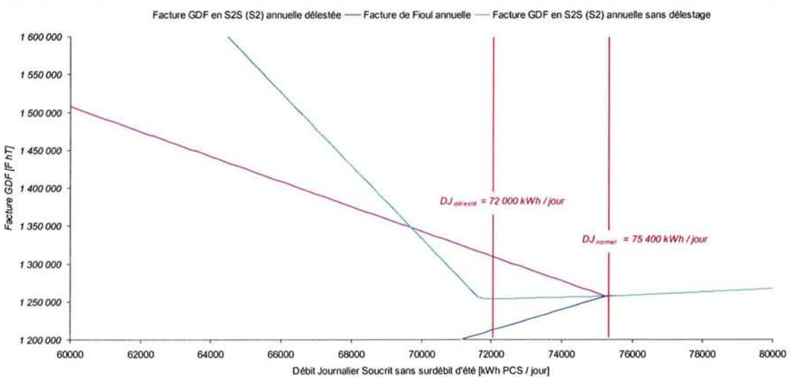
Figure 5-22 – A8 EJP conduite 3, facture S2S optimale avec et sans délestage du Gaz par le Fioul
