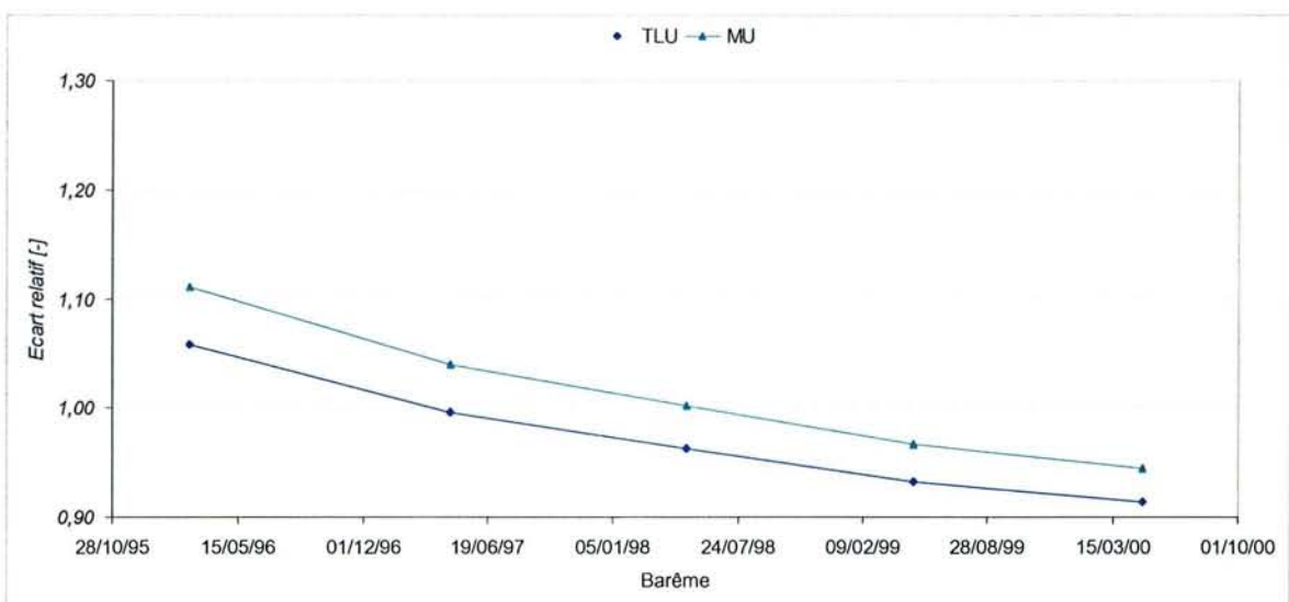
Figure 3-42 – A Mod, sensibilité des factures globales par rapport aux fluctuations des barèmes de prix
