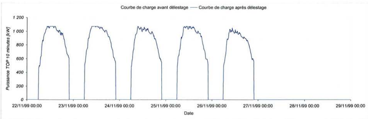
Figure 4-15 – Tarif A8 Base LU, tranche HPD délestée
