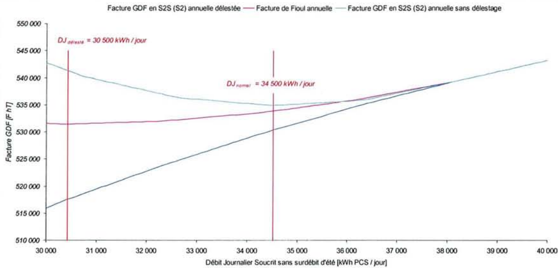
Figure 4-1 – Optimum des factures Gaz / Fioul avec et sans délestage
