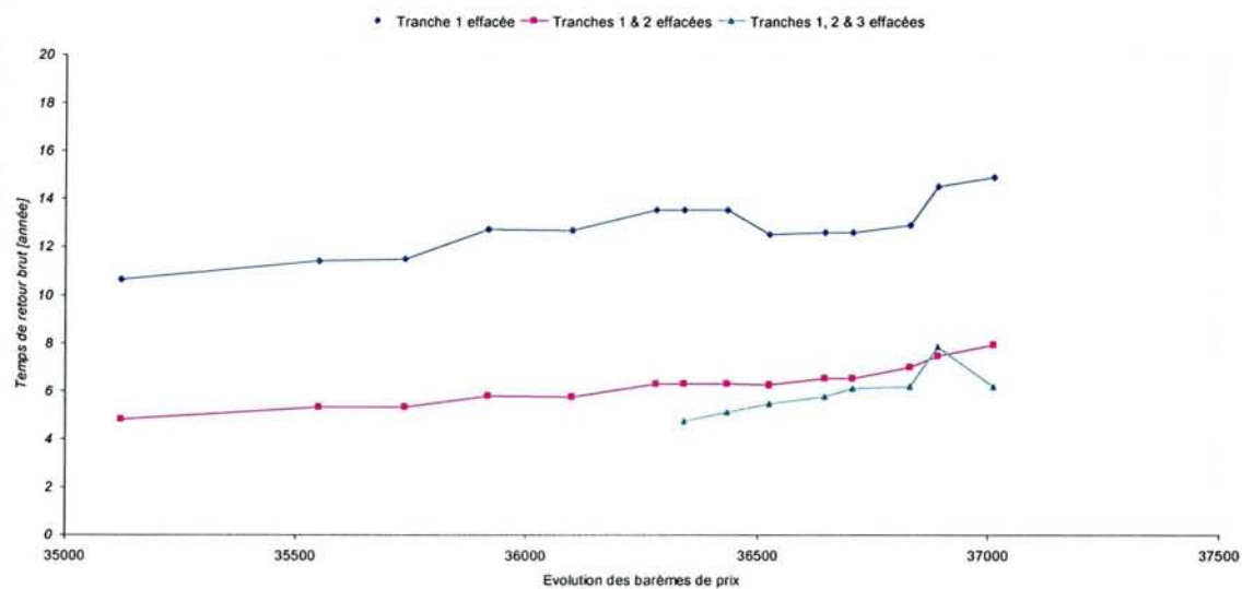
Figure 5-67 – Tarif A8 Base LU, sensibilité du temps de retour brut par rapport aux évolutions tarifaires
