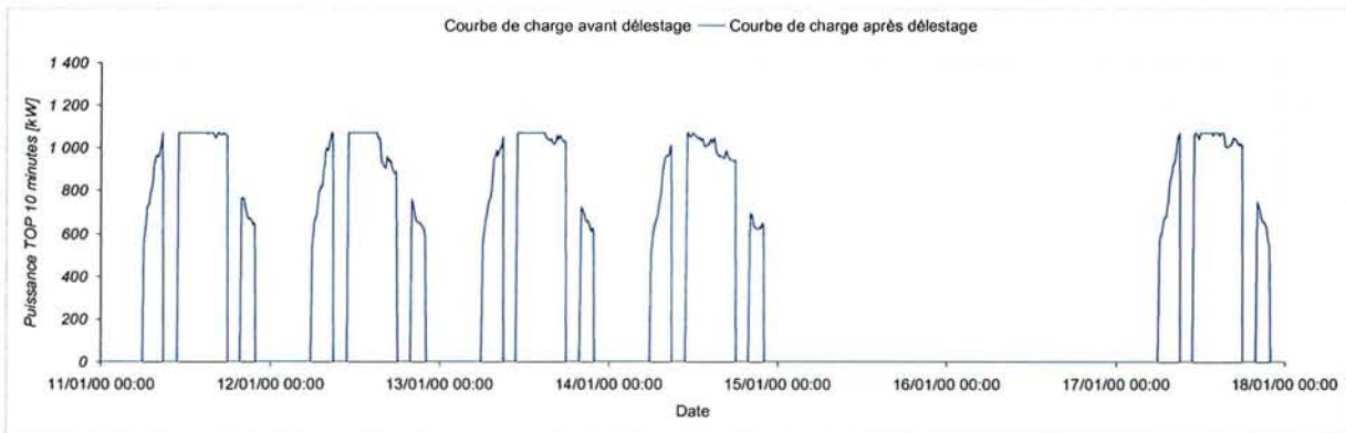
Figure 4-14 – Tarif A8 Base LU, tranche HPH délestée
