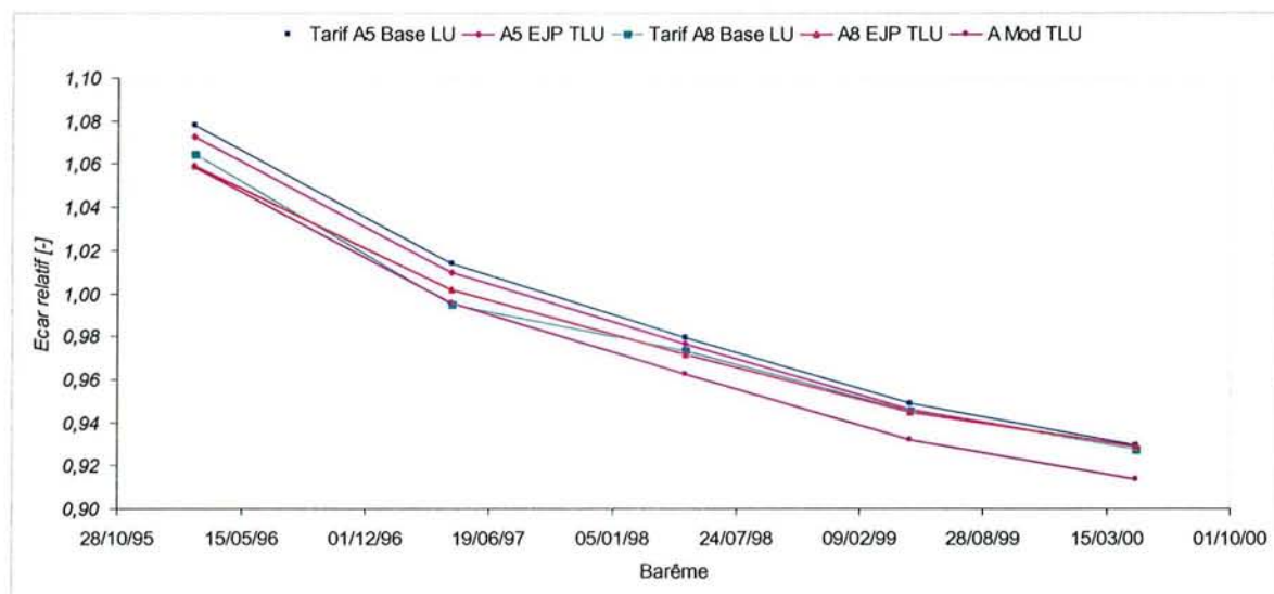
Figure 3-37 – Sensibilité des optimums trouvés par rapport aux fluctuations des barèmes de prix
