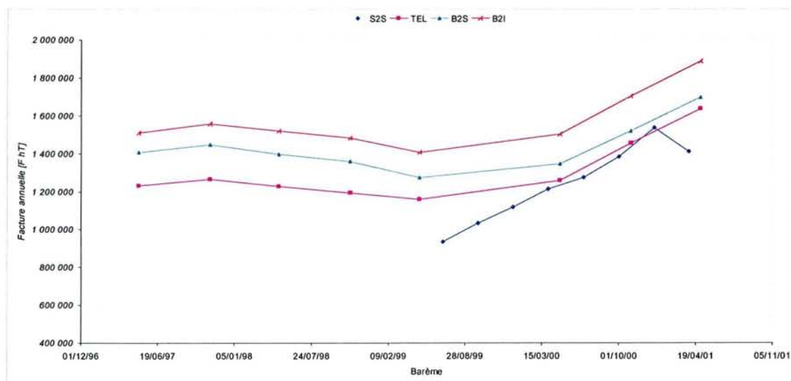
Figure 5-63 – Tarif A Mod centrale en conduite 3, évolution des factures gaz en fonction des barèmes
