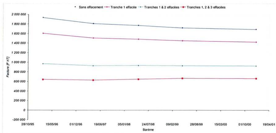
Figure 5-64 – Tarif A8 Base LU effacé, influence de l'évolution des barèmes sur la facture annuelle
