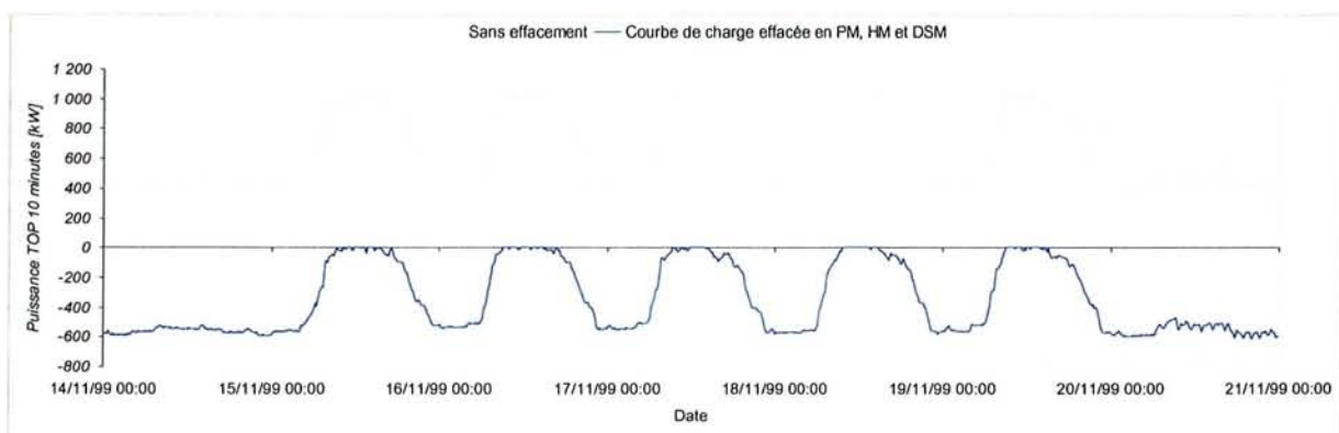
Figure 5-51 – Tarif A Mod TLU, optimisation par effacement selon la conduite 3
