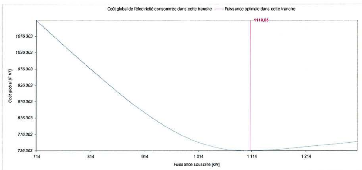
Figure 3-15 – Tarif A5 Base Version LU, puissance souscrite optimale dans la tranche HPH
