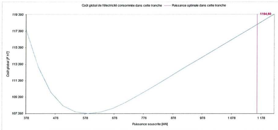
Figure 3-23 – Tarif A8 EJP Version TLU, puissance souscrite optimale dans la tranche HCE
