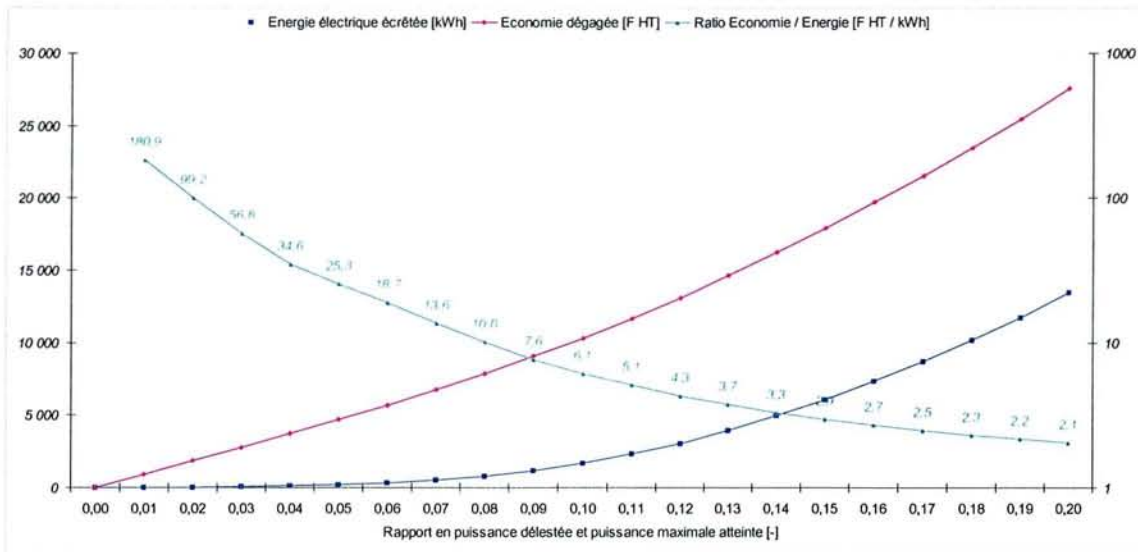
Figure 4-4 – Tarif A8 Base LU, économie réalisée par kWh délestés
