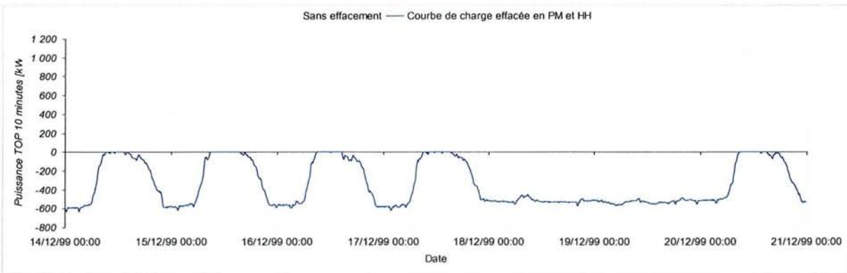
Figure 5-44 – Tarif A8 EJP TLU, optimisation par effacement selon la conduite 2
