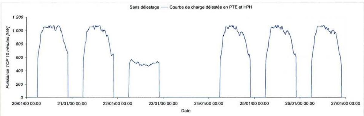
Figure 4-8 – Tarif A5 Base LU, optimisation par délestage dans les tranches PTE & HPH
