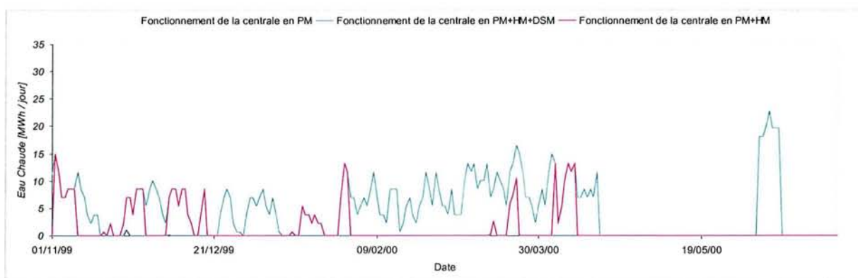
Figure 5-25 – Conduite de la centrale en A Mod, Eau Chaude excédentaire envoyée aux aérorefrigérants
