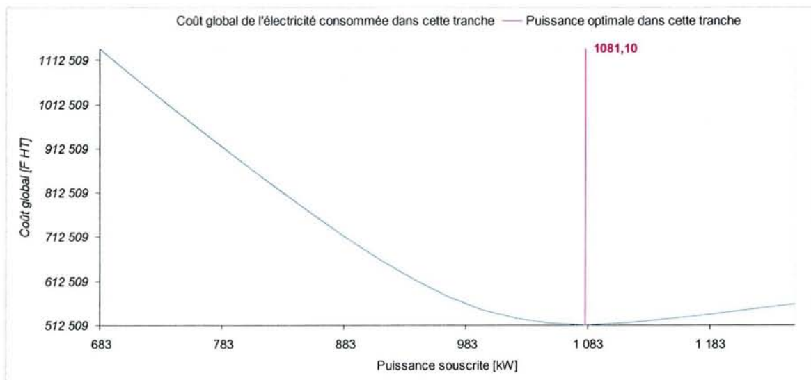
Figure 3-19 – Tarif A8 EJP Version TLU, puissance souscrite optimale dans la tranche PM
