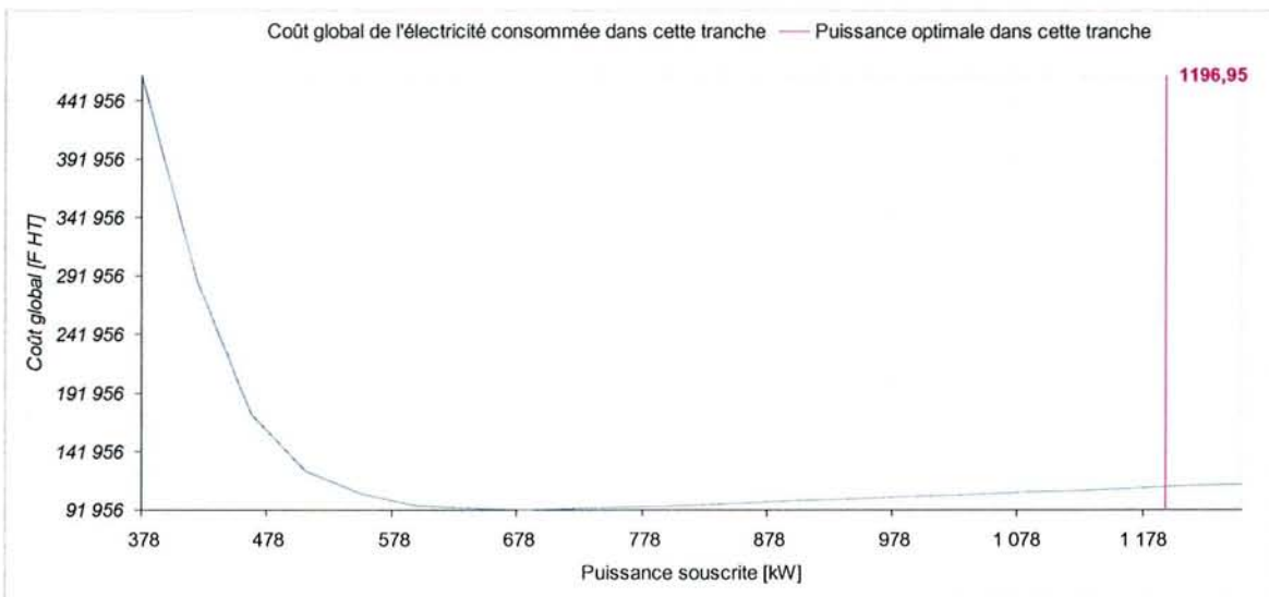
Figure 3-18 – Tarif A5 Base Version LU, puissance souscrite optimale dans la tranche HCE
