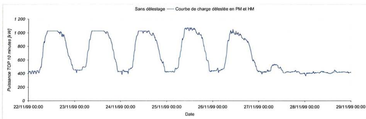
Figure 4-29 – Tarif A Mod TLU, optimisation par délestage dans les tranches PM & HM
