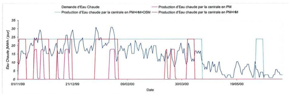
Figure 5-24 – Conduite de la centrale en A Mod, distribution des besoins et production d'Eau Chaude
