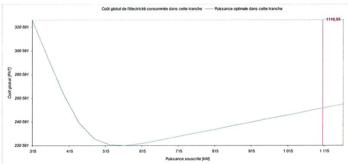
Figure 3-16 – Tarif A5 Base Version LU, puissance souscrite optimale dans la tranche HCH
