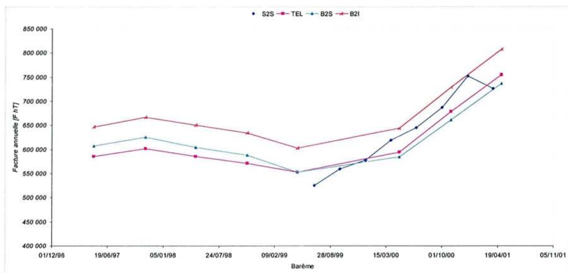
Figure 5-55 – Tarif A8 Base, centrale en conduite 1, évolution des factures gaz en fonction des barèmes
