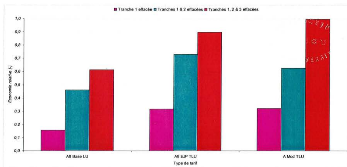
Figure 5-52 – Economie relative pour chaque tarif / chaque conduite en comparant avec et sans effacement
