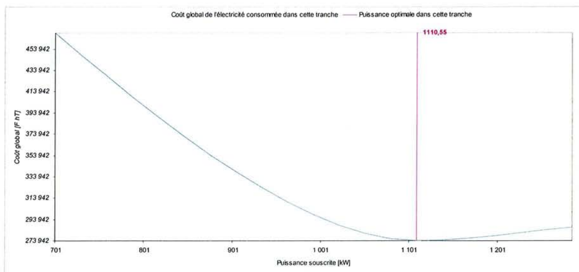
Figure 3-14 – Tarif A5 Base Version LU, puissance souscrite optimale dans la tranche PTE
