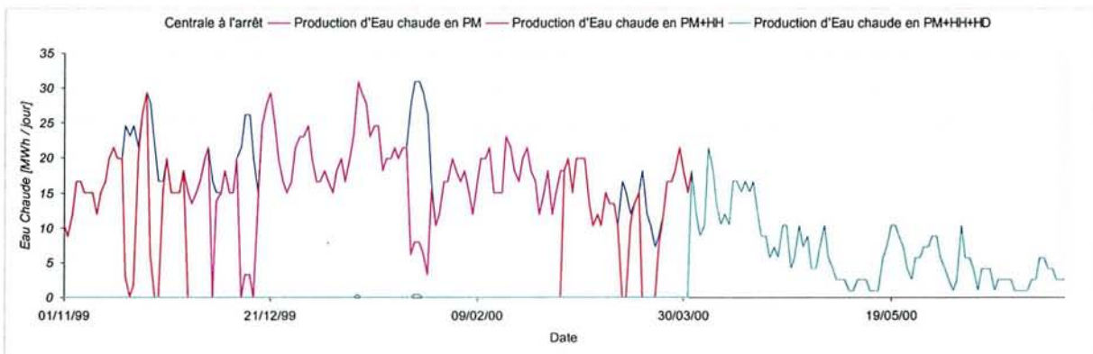
Figure 5-17 – Conduite de la centrale en A8 EJP, appoint de charge d'Eau Chaude demandée en chaufferie
