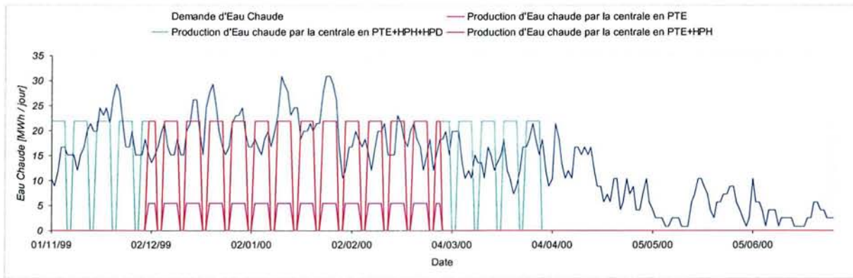
Figure 5-6 – Conduite de la centrale en A8 Base, distribution des besoins et production d'Eau Chaude
