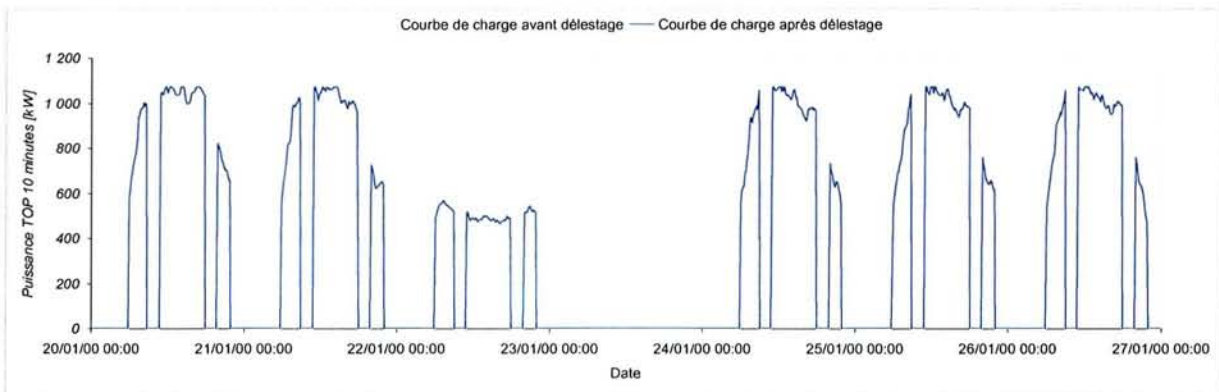
Figure 4-6 – Tarif A5 Base LU, tranche HPH délestée
