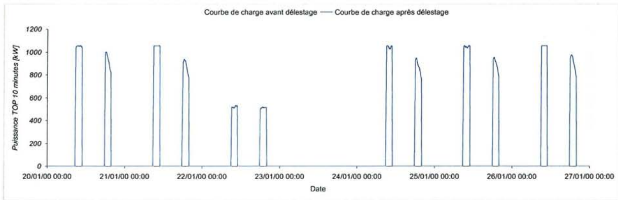
Figure 4-5 – Tarif A5 Base LU, tranche PTE délestée
