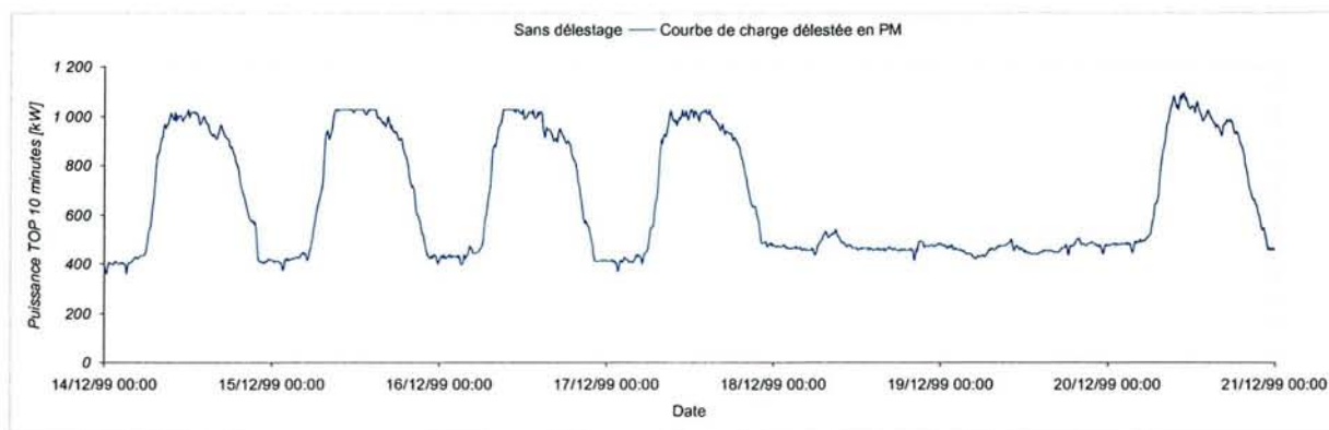
Figure 4-22 – Tarif A8 EJP TLU, optimisation par délestage dans la tranche PM
