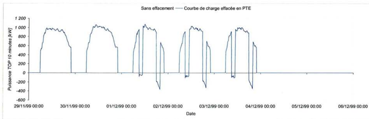
Figure 5-36 – Tarif A8 Base LU, optimisation par effacement selon la conduite 1
