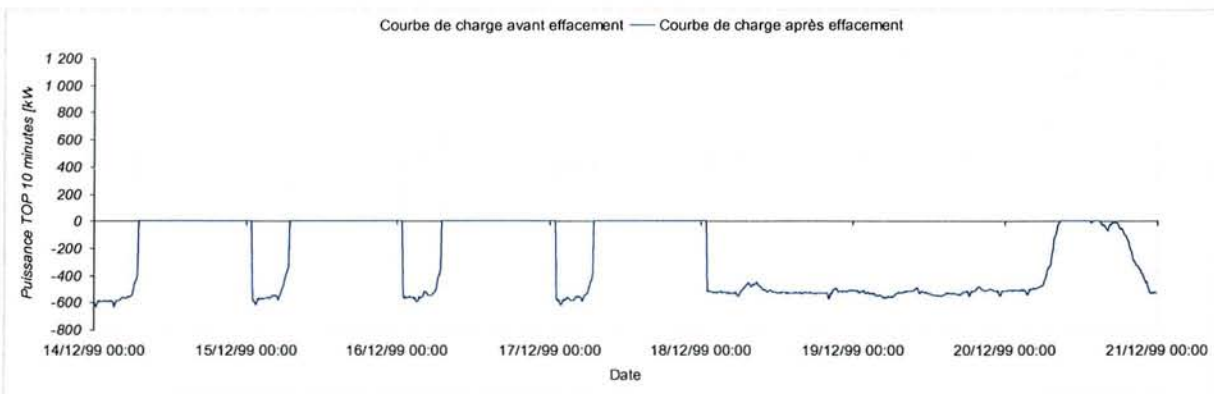
Figure 5-40 – Tarif A8 EJP TLU, tranche HH effacée
