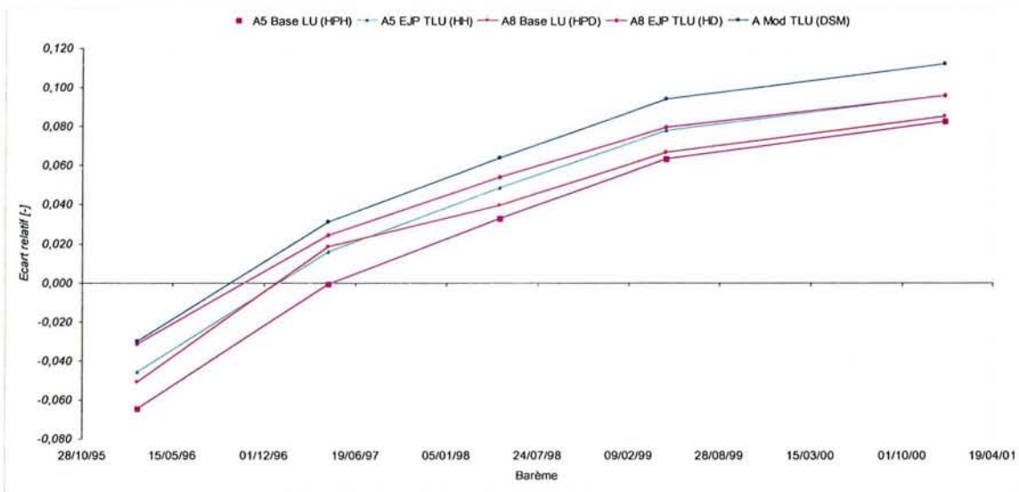
Figure 4-34 – Sensibilité des optimums délestés par rapport aux fluctuations des barèmes de prix
