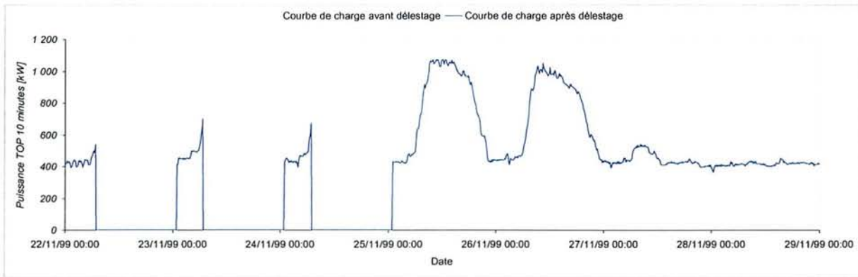
Figure 4-26 – Tarif A Mod TLU, tranche HM délestée
