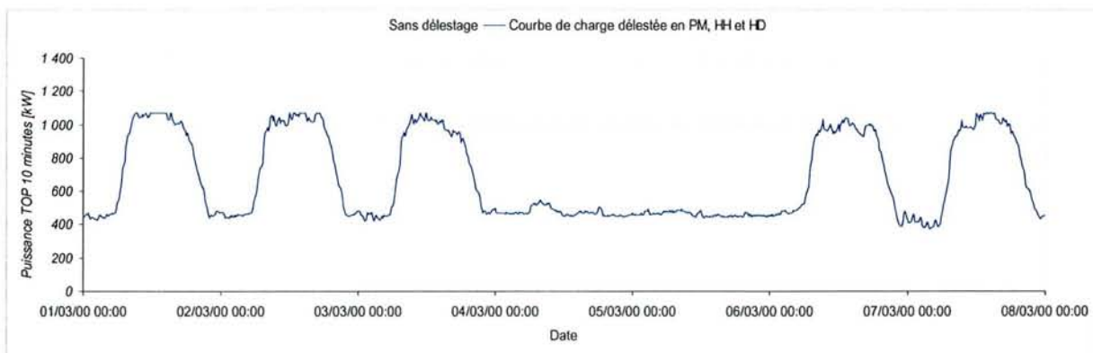
Figure 4-24 – Tarif A8 EJP TLU, optimisation par délestage dans les tranches PM, HH & HD
