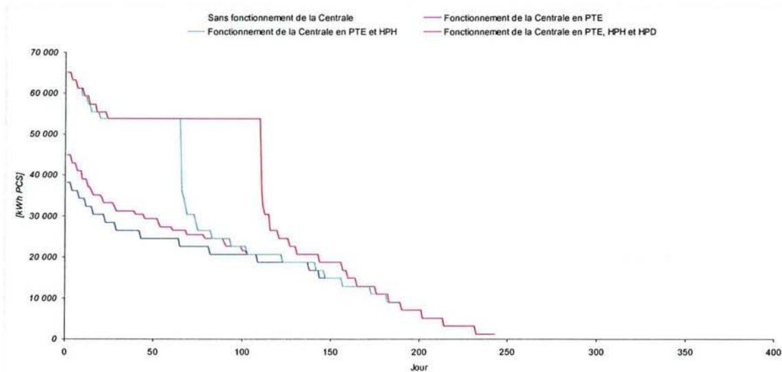
Figure 5-9 – Conduite de la centrale en A8 Base, monotone d'appel global de Gaz
