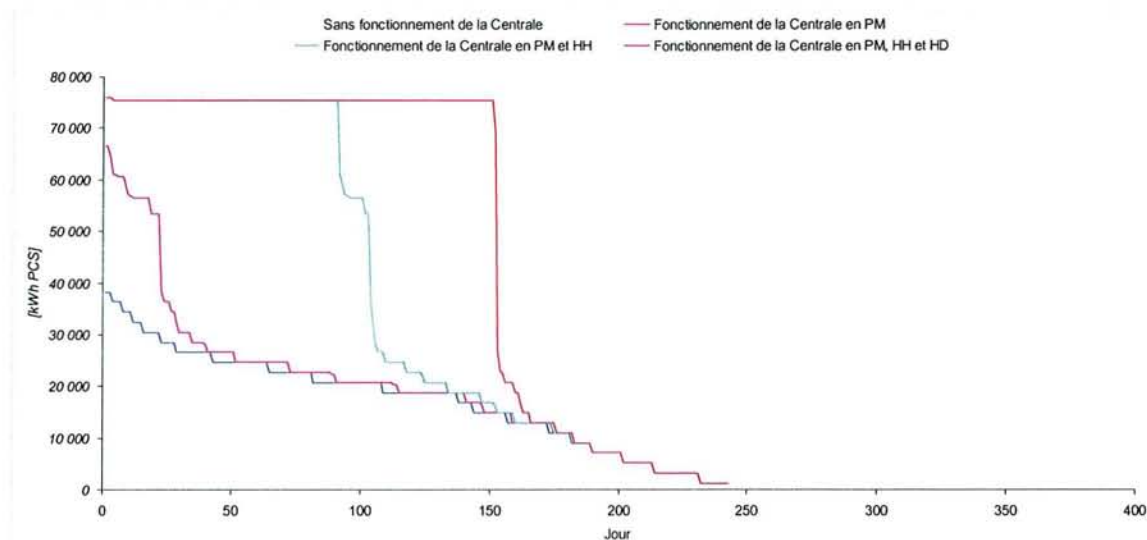
Figure 5-18 – Conduite de la centrale en A8 EJP, monotone d'appel global de Gaz
