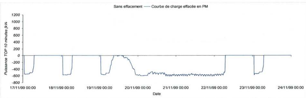
Figure 5-42 – Tarif A8 EJP TLU, tranche HD effacée
