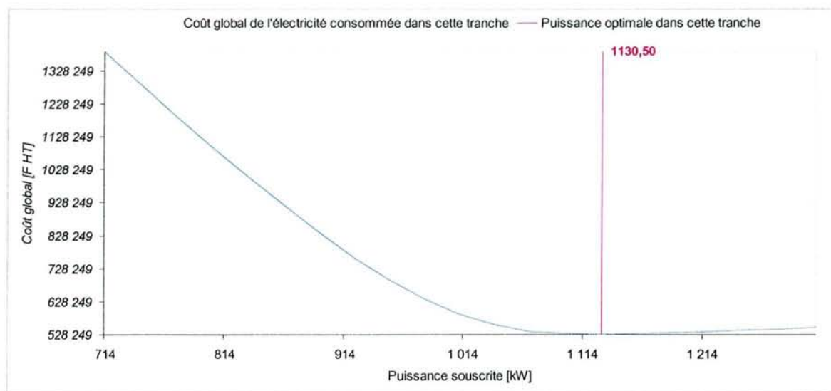
Figure 3-20 – Tarif A8 EJP Version TLU, puissance souscrite optimale dans la tranche HH
