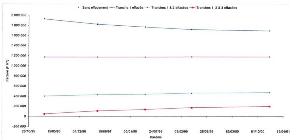
Figure 5-65 – Tarif A8 EJP TLU effacé, influence de l'évolution des barèmes sur la facture annuelle
