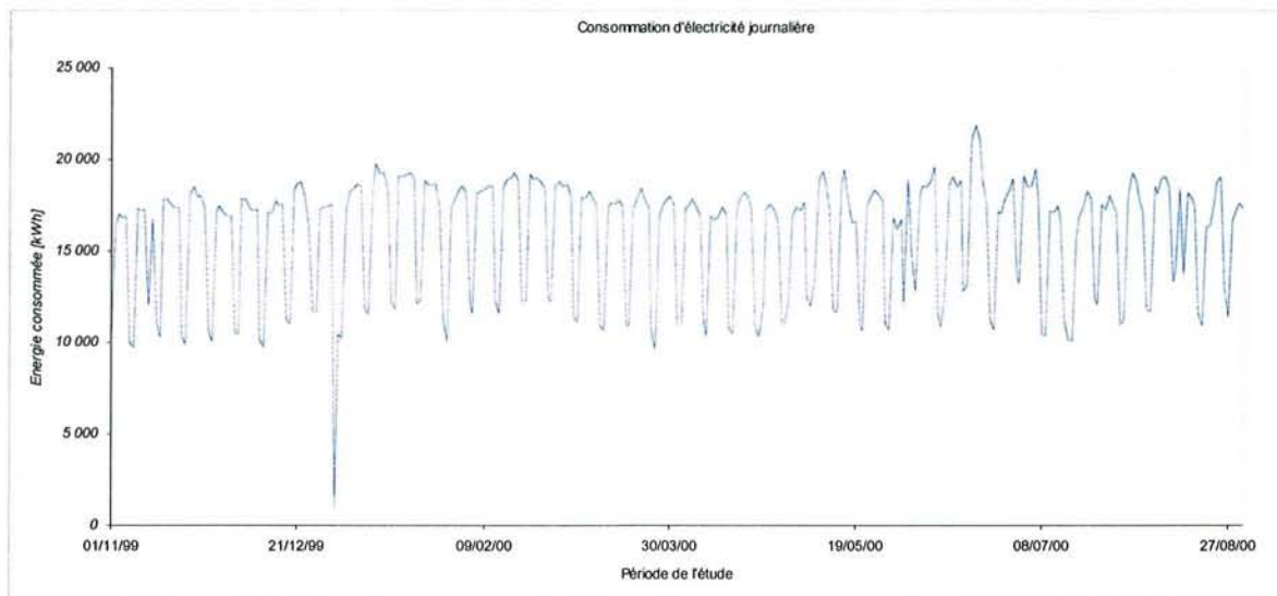
Figure 3-11– Distribution des consommations d'électricité journalières du 1/11/99 au 31/08/00
