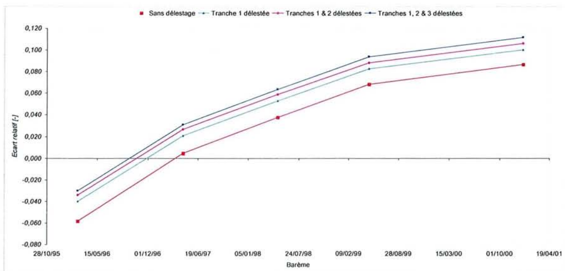
Figure 4-39 – A Mod TLU, sensibilité des factures délestées selon les fluctuations des barèmes de prix
