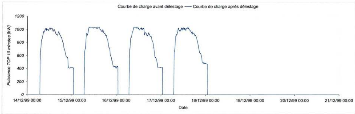
Figure 4-19 – Tarif A8 EJP TLU, tranche PM délestée
