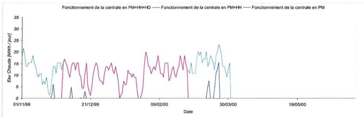
Figure 5-16 – Conduite de la centrale en A8 EJP, Eau Chaude excédentaire envoyée aux aérorefrigérants
