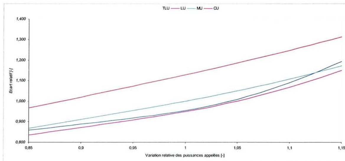
Figure 3-32 – A5 Base, sensibilité des factures globales par rapport aux fluctuations des consommations
