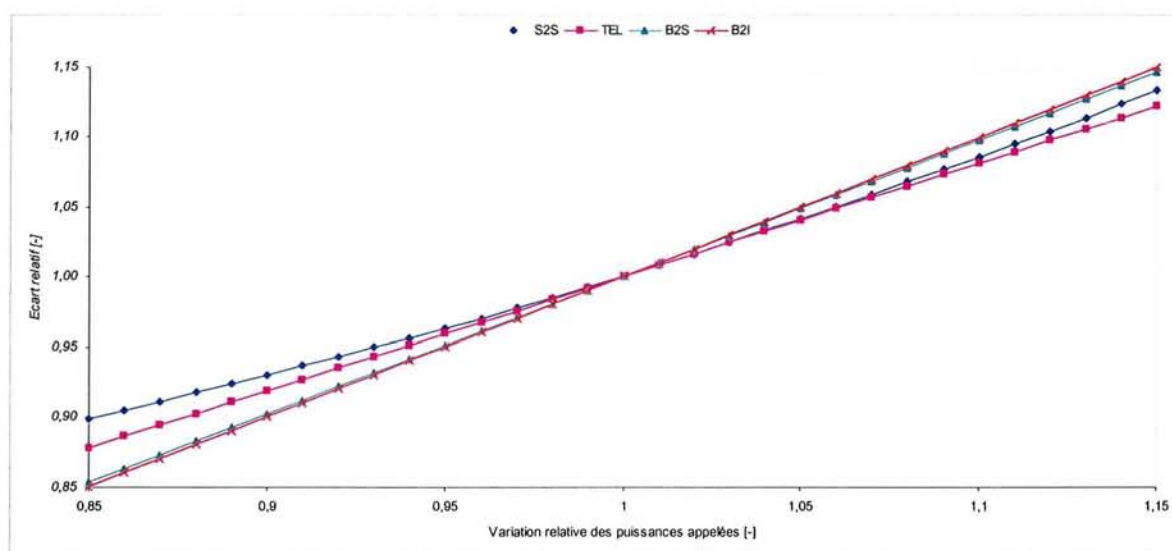
Figure 3-8 – Influence des puissances appelées sur la facture globale / écart relatif
