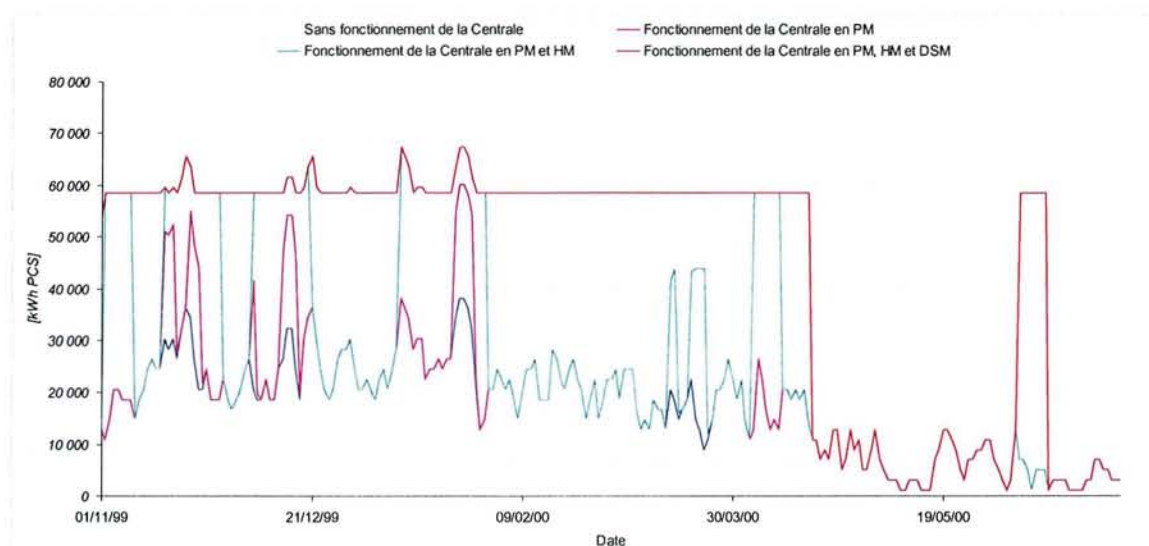
Figure 5-28 – Conduite de la centrale en A Mod, distribution des appels globaux journaliers de Gaz
