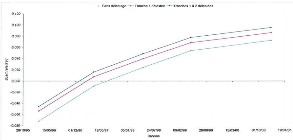
Figure 4-35 – A5 Base LU, sensibilité des factures délestées selon les fluctuations des barèmes de prix
