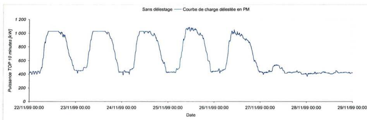
Figure 4-28 – Tarif A Mod TLU, optimisation par délestage dans la tranche PM
