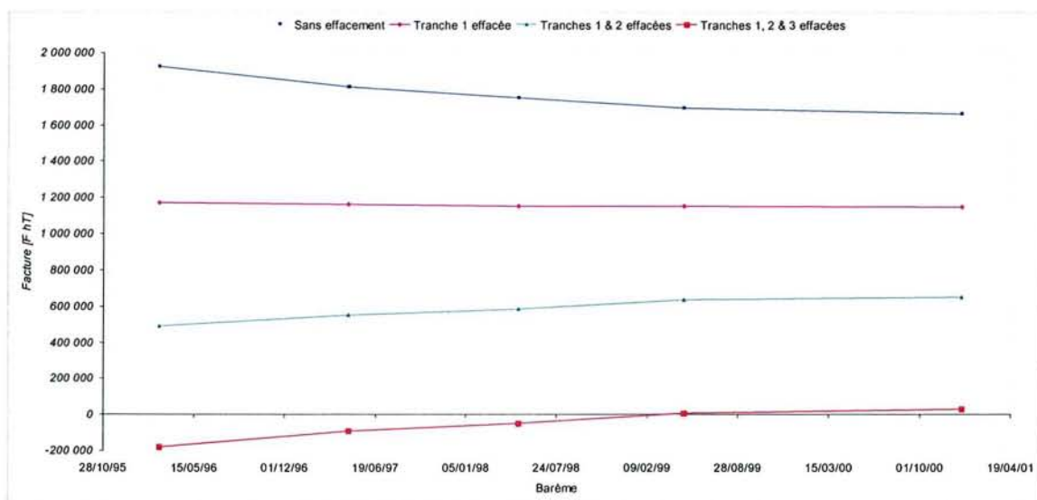
Figure 5-66 – Tarif A Mod TLU effacé, influence de l'évolution des barèmes sur la facture annuelle
