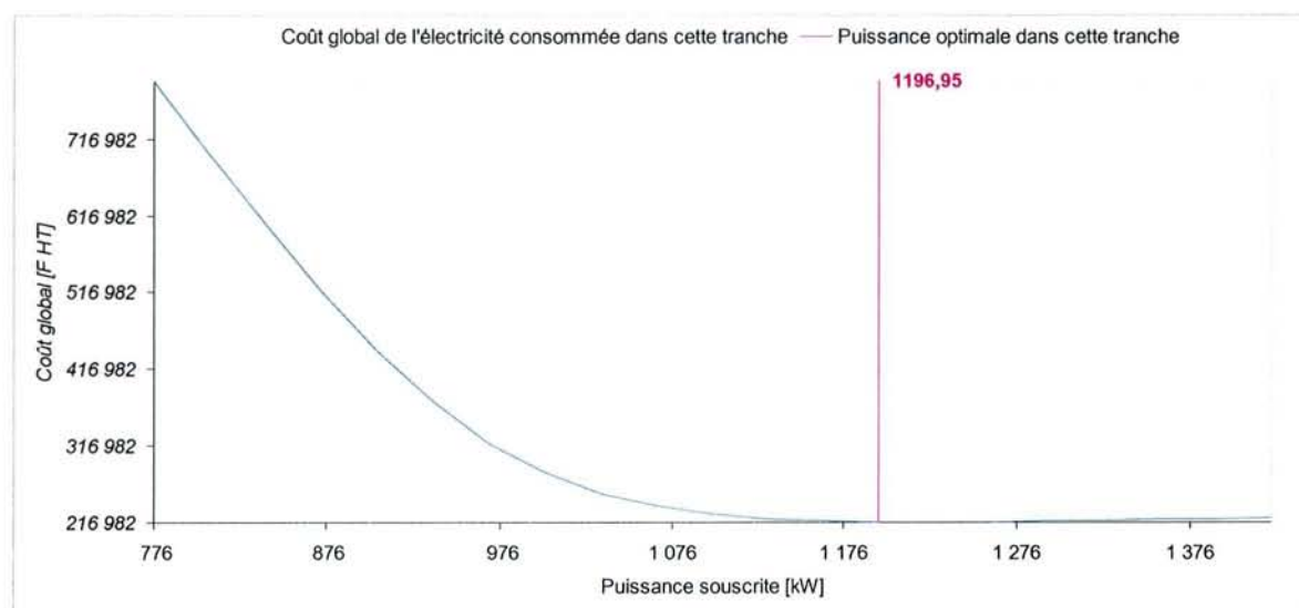
Figure 3-22 – Tarif A8 EJP Version TLU, puissance souscrite optimale dans la tranche HPE
