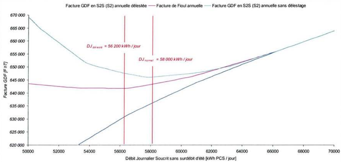
Figure 5-20 – A8 EJP conduite 1, facture S2S optimale avec et sans délestage du Gaz par le Fioul
