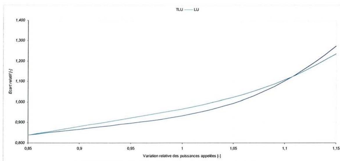
Figure 3-36 – A Mod, sensibilité des factures globales par rapport aux fluctuations des consommations
