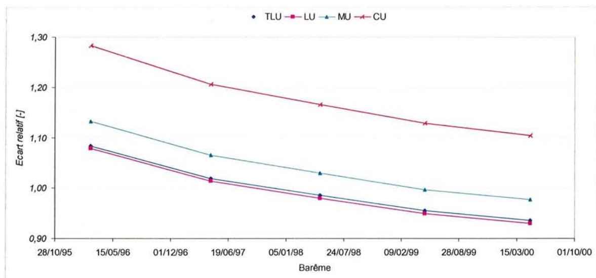
Figure 3-38 – A5 Base, sensibilité des factures globales par rapport aux fluctuations des barèmes de prix
