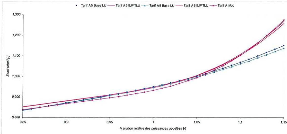
Figure 3-31 – Sensibilité des optimums trouvés par rapport aux fluctuations des consommations
