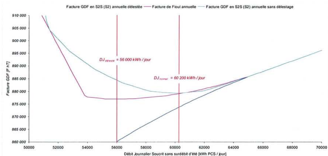
Figure 5-13 – A8 Base conduite 3, facture S2S optimale avec et sans délestage du Gaz par le Fioul
