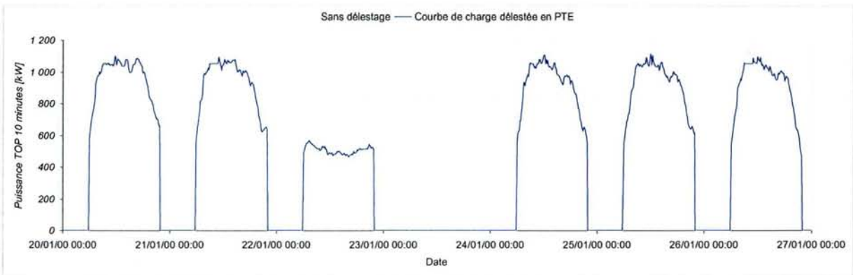
Figure 4-7 – Tarif A5 Base LU, optimisation par délestage dans la tranche PTE
