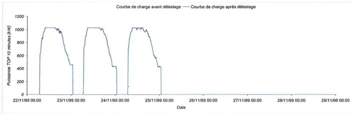
Figure 4-25 – Tarif A Mod TLU, tranche PM délestée
