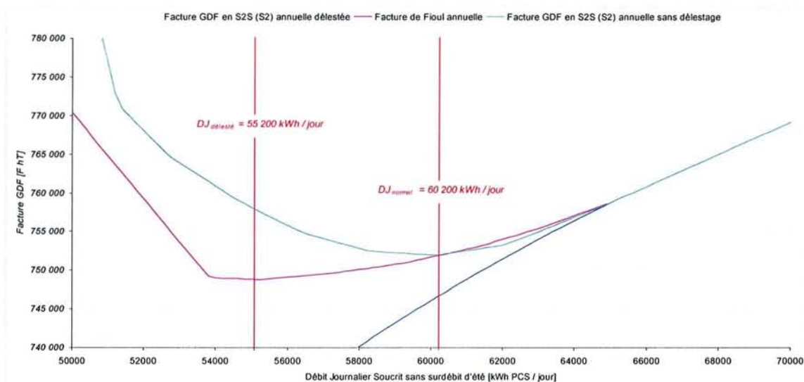
Figure 5-12 – A8 Base conduite 2, facture S2S optimale avec et sans délestage du Gaz par le Fioul
