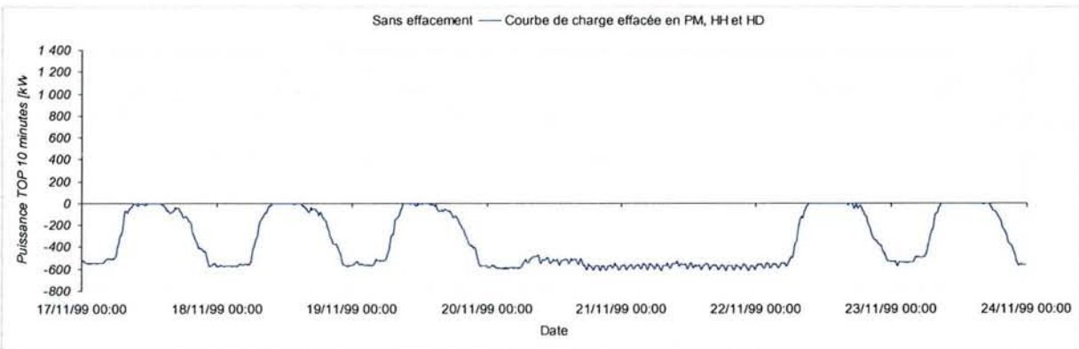
Figure 5-45 – Tarif A8 EJP TLU, optimisation par effacement selon la conduite 3
