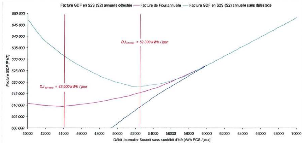
Figure 5-29 – A Mod conduite 1, facture S2S optimale avec et sans délestage du Gaz par le Fioul
