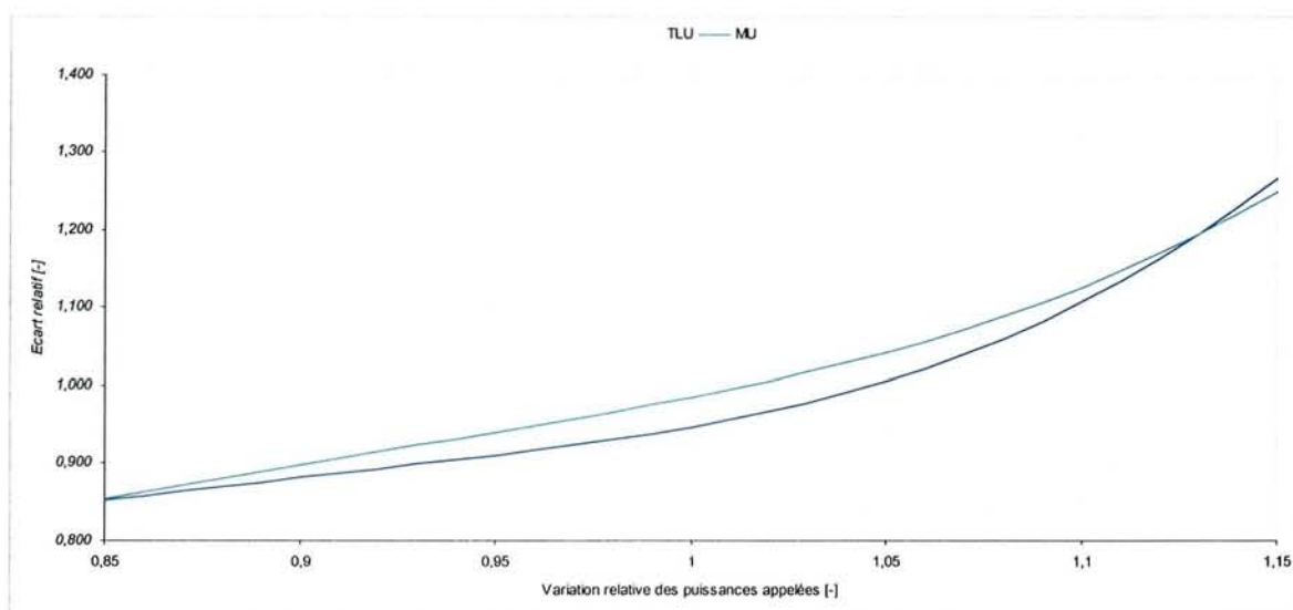
Figure 3-33 – A5 EJP, sensibilité des factures globales par rapport aux fluctuations des consommations
