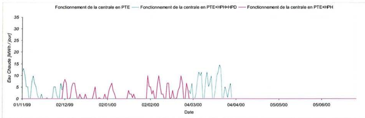
Figure 5-7 – Conduite de la centrale en A8 Base, Eau Chaude excédentaire envoyée aux aérorefrigérants
