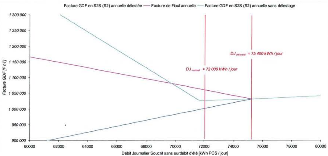
Figure 5-21 – A8 EJP conduite 2, facture S2S optimale avec et sans délestage du Gaz par le Fioul
