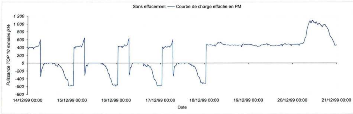
Figure 5-43 – Tarif A8 EJP TLU, optimisation par effacement selon la conduite 1
