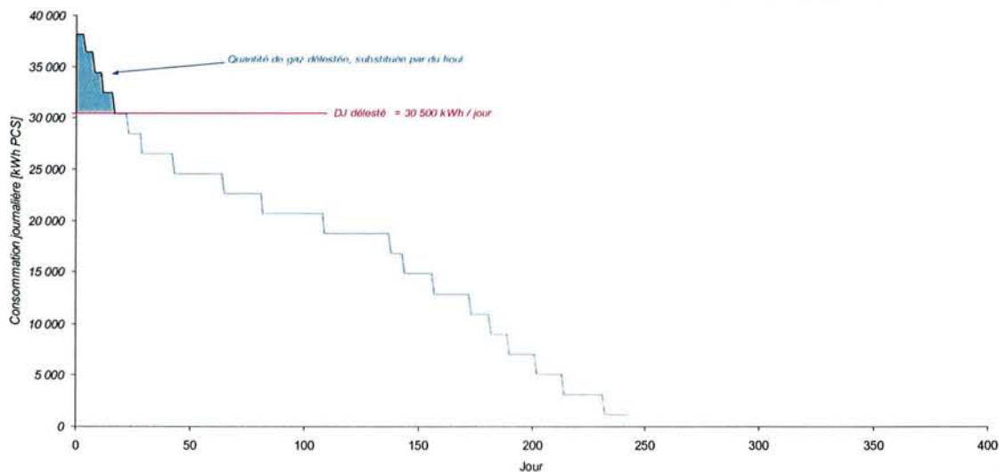
Figure 4-2 – Monotone de Gaz avec ou sans délestage
