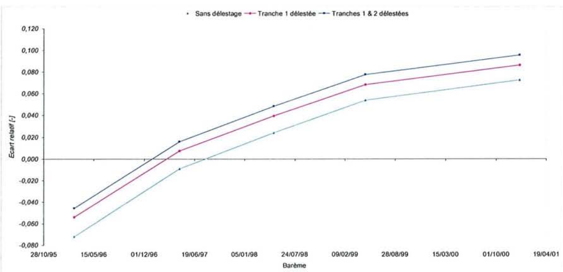
Figure 4-36 – A5 EJP TLU, sensibilité des factures délestées selon les fluctuations des barèmes de prix
