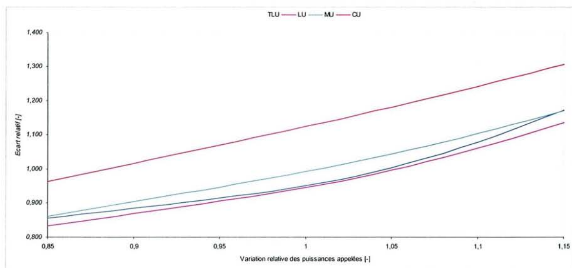
Figure 3-34 – A8 Base, sensibilité des factures globales par rapport aux fluctuations des consommations
