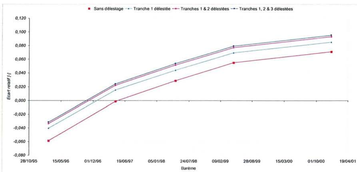
Figure 4-38 – A8 EJP TLU, sensibilité des factures délestées selon les fluctuations des barèmes de prix
