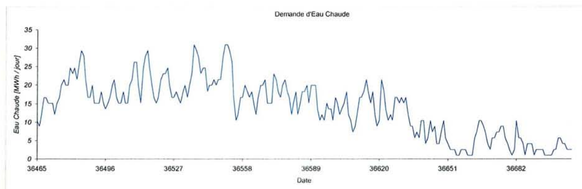
Figure 3-2 – Distribution des besoins d'Eau Chaude de l'établissement
