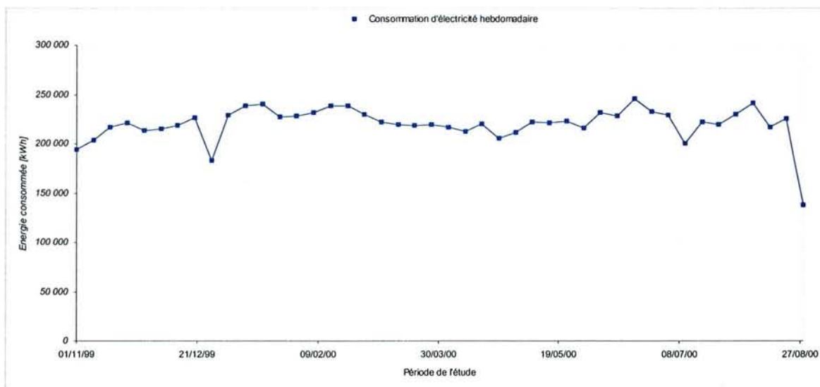
Figure 3-12– Distribution des consommations d'électricité hebdomadaires du 1/11/99 au 28/08/00
