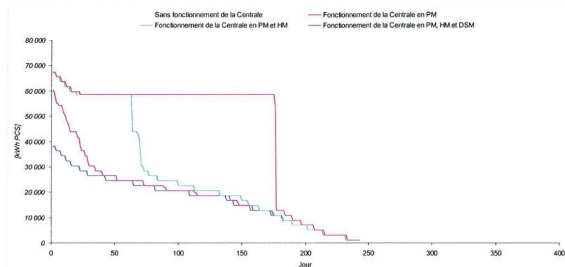
Figure 5-27 – Conduite de la centrale en A Mod, monotone d'appel global de Gaz
