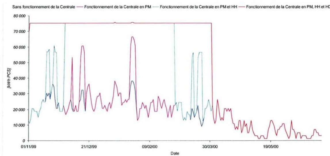
Figure 5-19 – Conduite de la centrale en A8 EJP, distribution des appels globaux journaliers de Gaz
