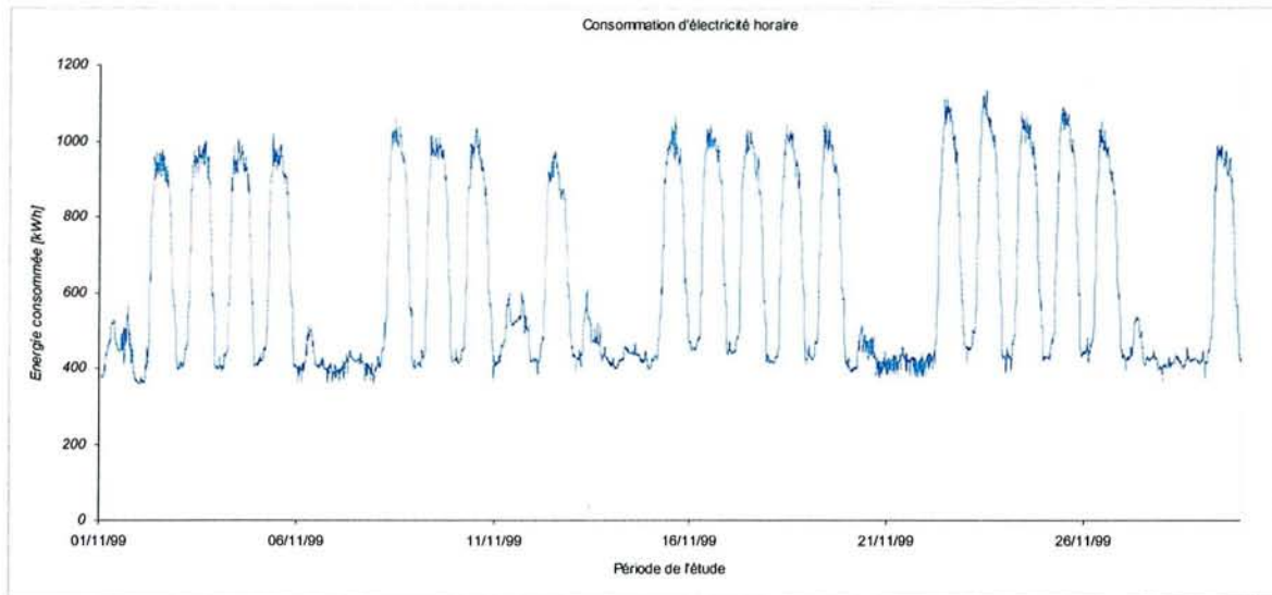
Figure 3-10 – Distribution des consommations d'électricité horaires du 1/11/99 au 30/11/99
