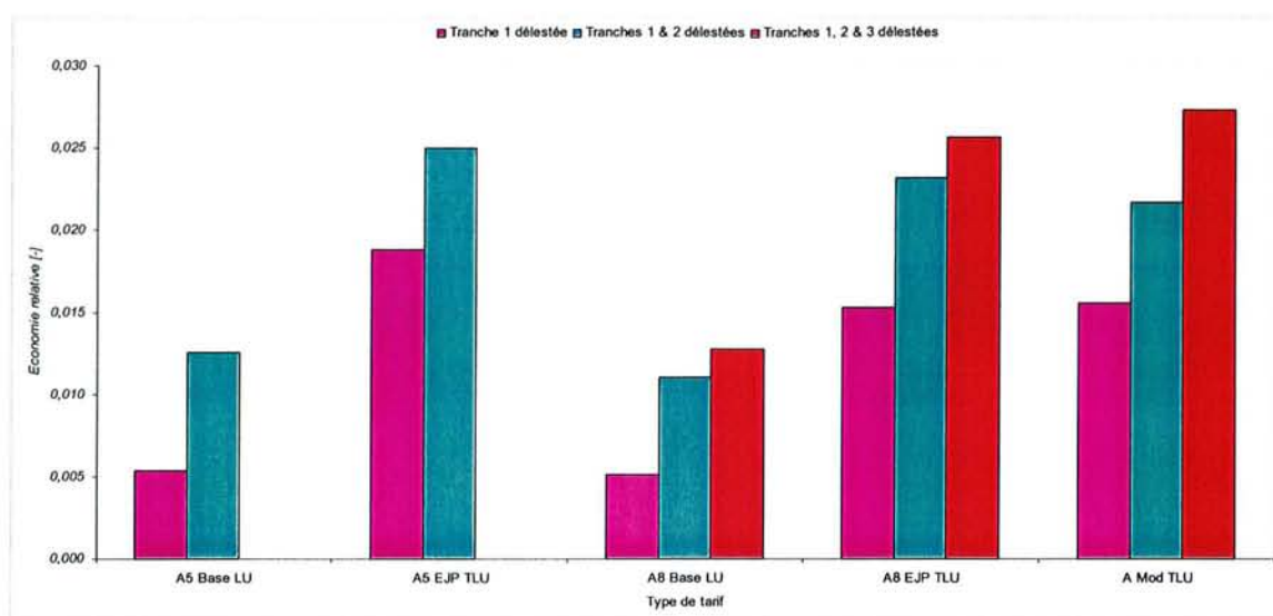
Figure 4-31 – Economie globale relative par type de contrat et selon le nombre de tranches délestées
