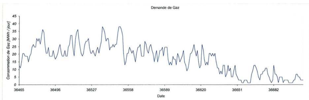
Figure 3-3 – Distribution des appels de Gaz de l'établissement
