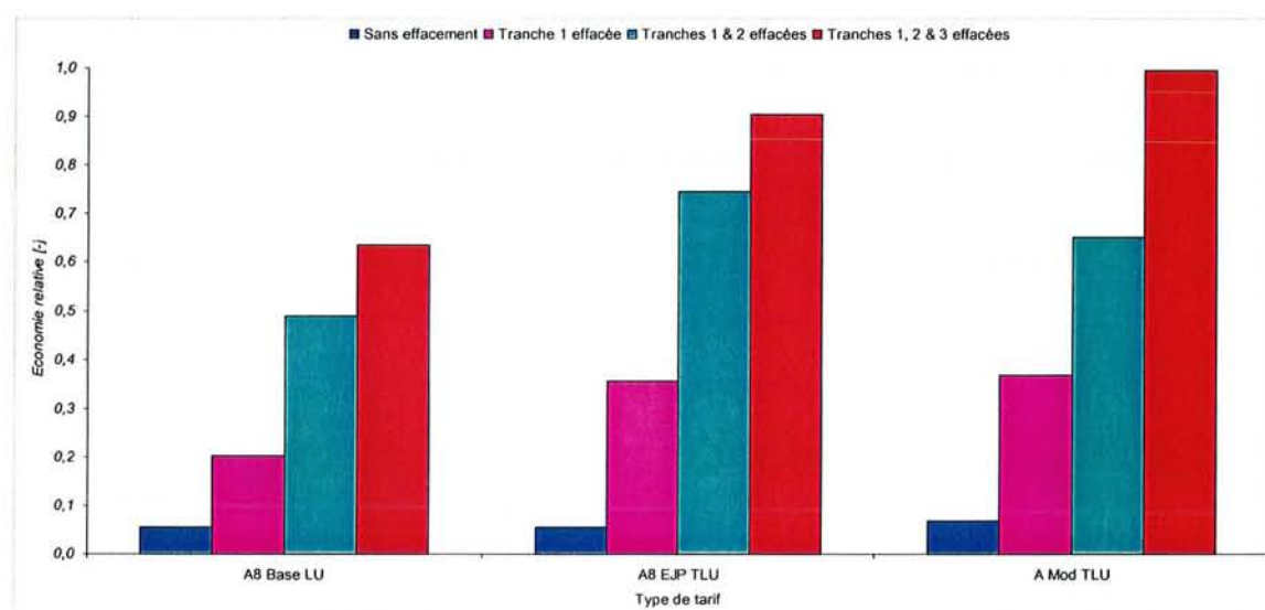
Figure 5-53 – Economie relative par rapport à la souscription actuelle du consommateur
