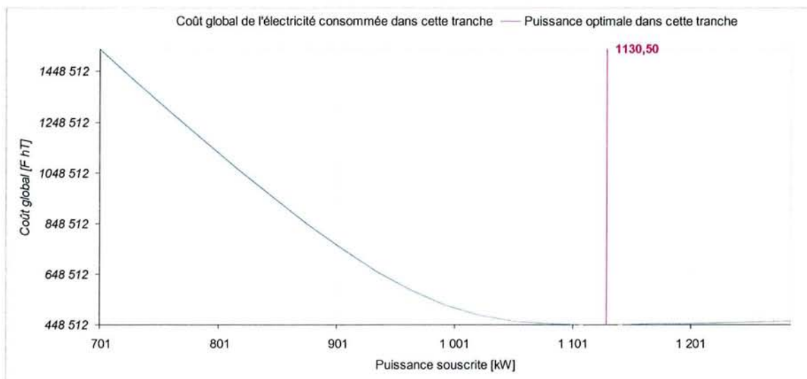
Figure 3-27 – Tarif A Mod. Version TLU, puissance souscrite optimale dans la tranche DSM
