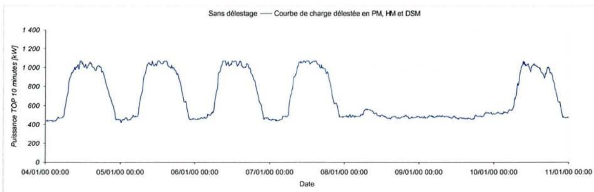
Figure 4-30 – Tarif A Mod TLU, optimisation par délestage dans les tranches PM, HM & DSM
