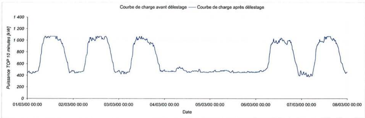
Figure 4-21 – Tarif A8 EJP TLU, tranche HD délestée
