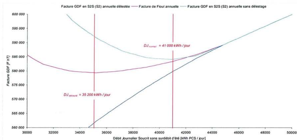
Figure 5-11 – A8 Base conduite 1, facture S2S optimale avec et sans délestage du Gaz par le Fioul
