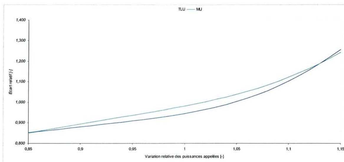
Figure 3-35 – A8 EJP, sensibilité des factures globales par rapport aux fluctuations des consommations
