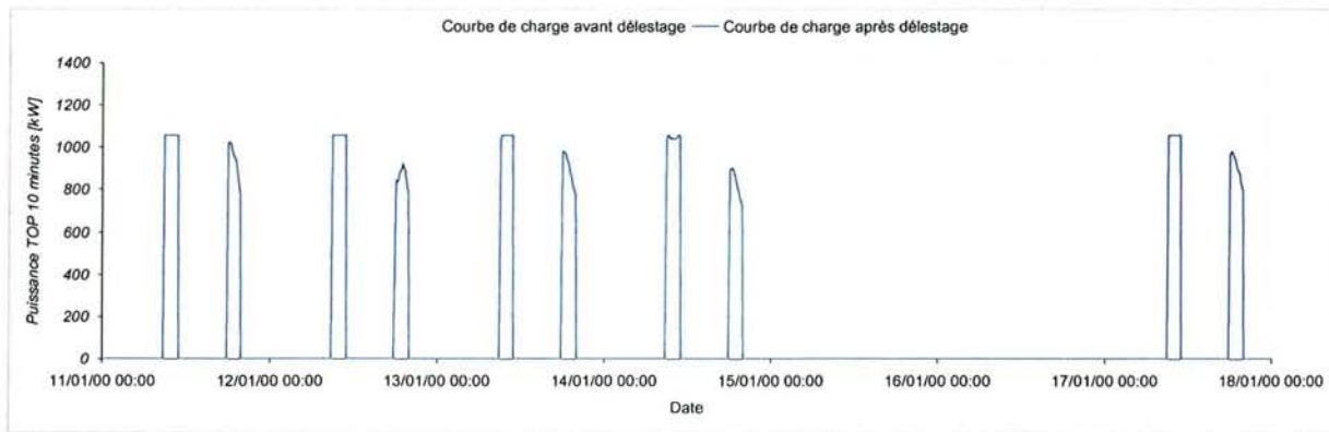
Figure 4-13 – Tarif A8 Base LU, tranche PTE délestée
