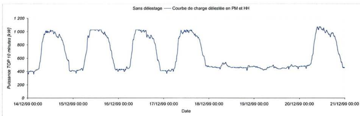
Figure 4-23 – Tarif A8 EJP TLU, optimisation par délestage dans les tranches PM & HH
