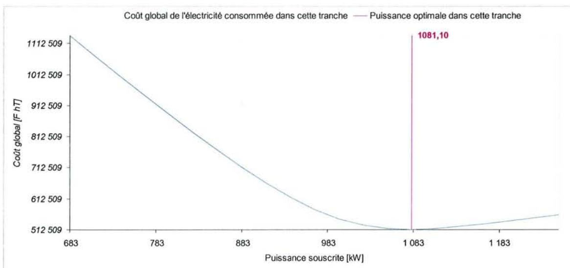
Figure 3-25 – Tarif A Mod. Version TLU, puissance souscrite optimale dans la tranche PM
