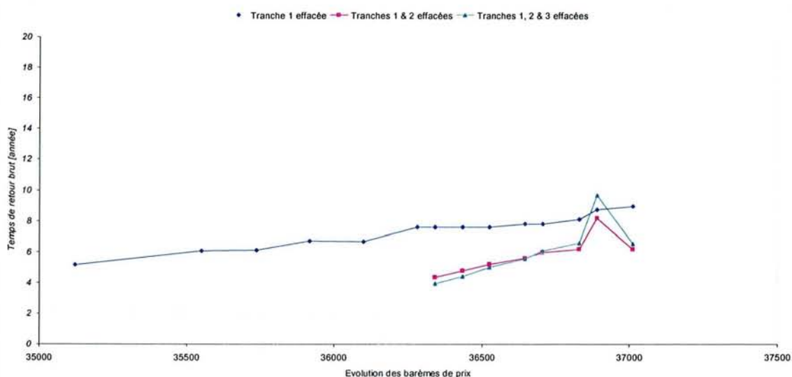
Figure 5-68 – Tarif A8 EJP TLU, sensibilité du temps de retour brut par rapport aux évolutions tarifaires
