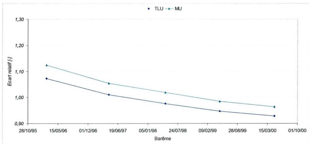
Figure 3-39 – A5 EJP, sensibilité des factures globales par rapport aux fluctuations des barèmes de prix
