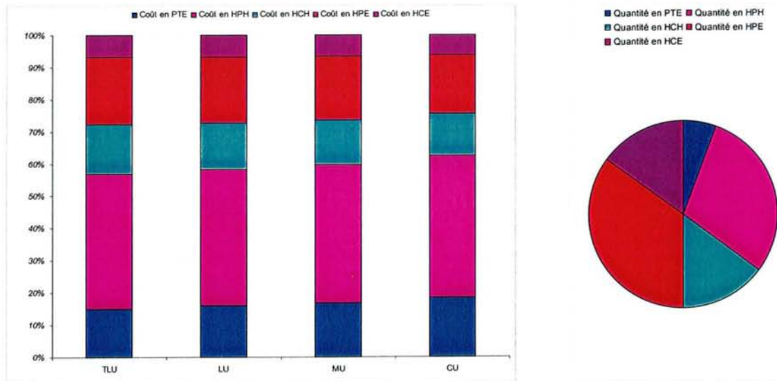
Figure 5-1 – Tarif A5 Base LU, contribution des différentes tranches dans la facture globale d'électricité
