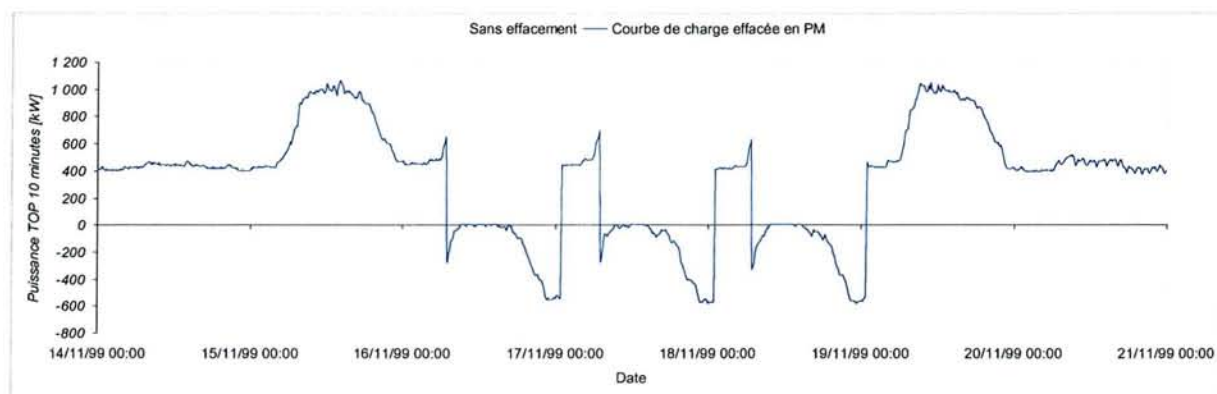
Figure 5-49 – Tarif A Mod TLU, optimisation par effacement selon la conduite 1
