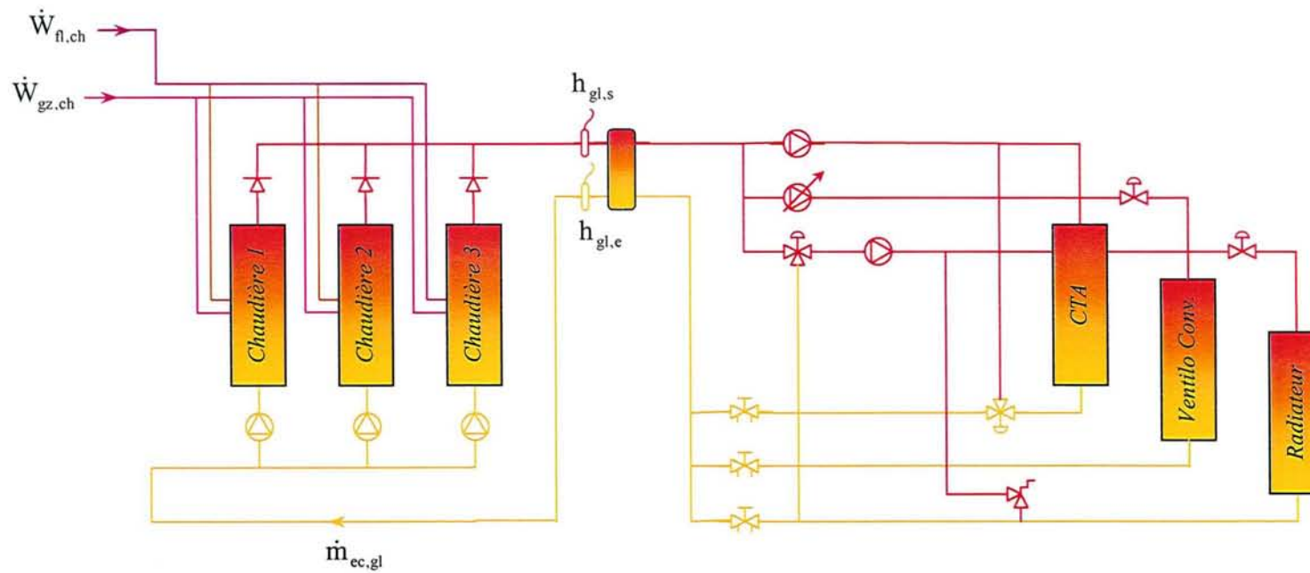
Figure 2-1 – Schéma de principe de chaufferie
