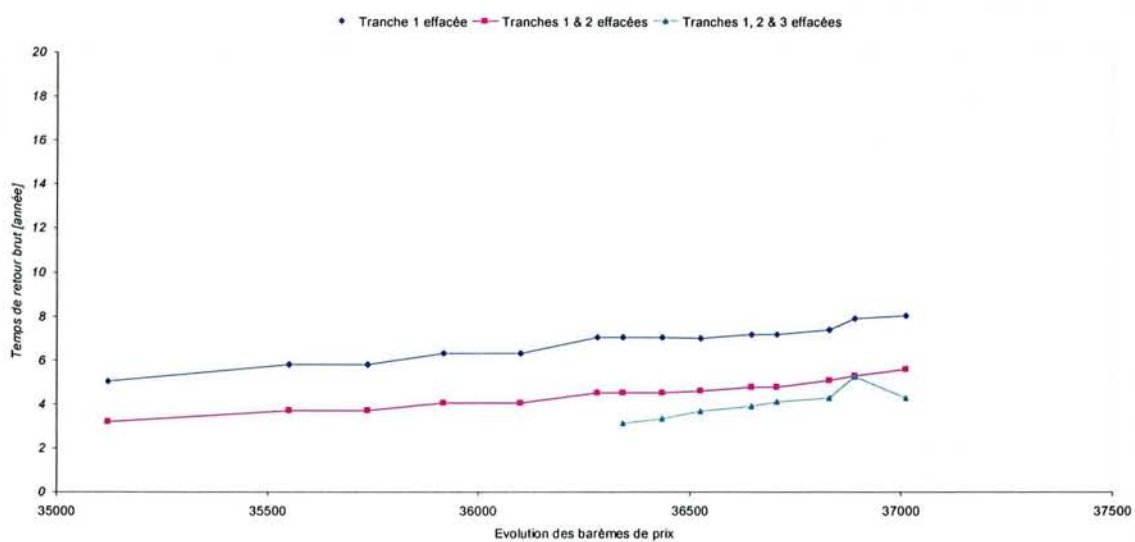
Figure 5-69 – Tarif A Mod TLU, sensibilité du temps de retour brut par rapport aux évolutions tarifaires
