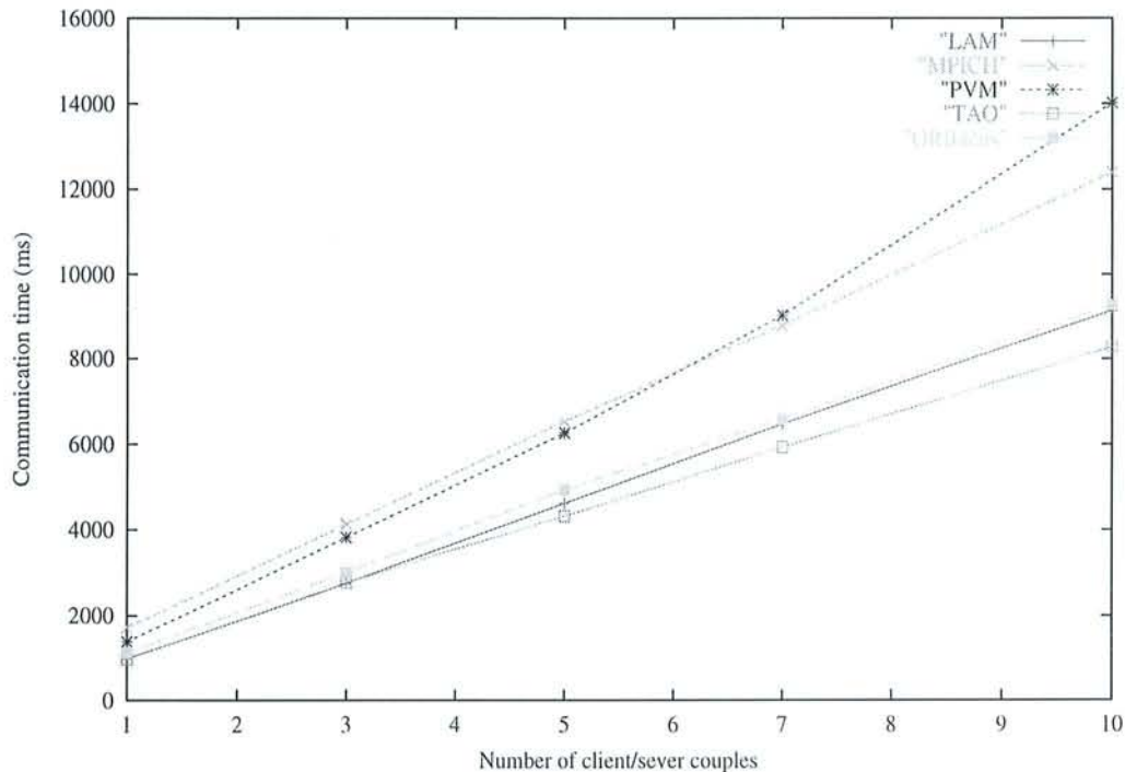
FIG. 8.11 – Temps de communication pour une taille de données de 1 Mo en fonction du nombre de couples client/serveur
