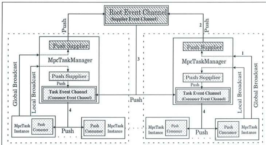
FIG. 10.16 – Le modèle de la diffusion globale
