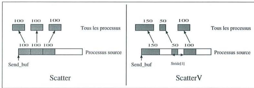
FIG. 6.2 – Différence entre Scatter et ScatterV
