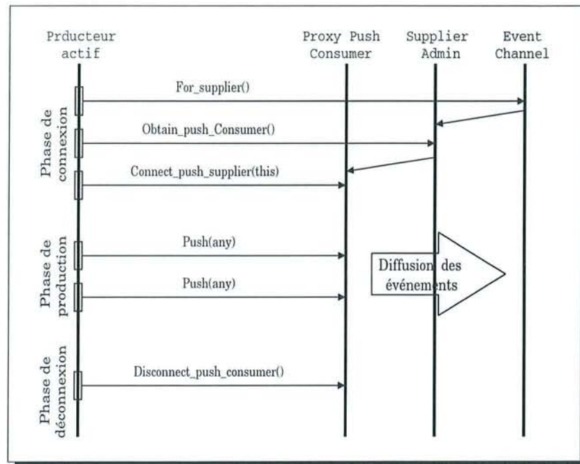
FIG. 10.12 – Le scénario d'un producteur actif
