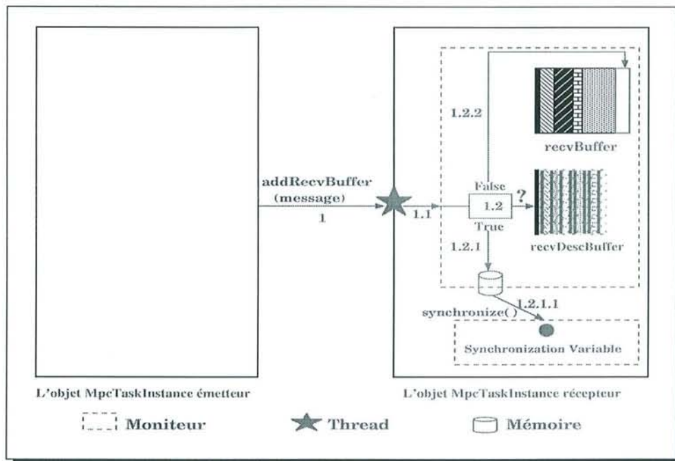
FIG. 10.4 – L'envoi asynchrone
