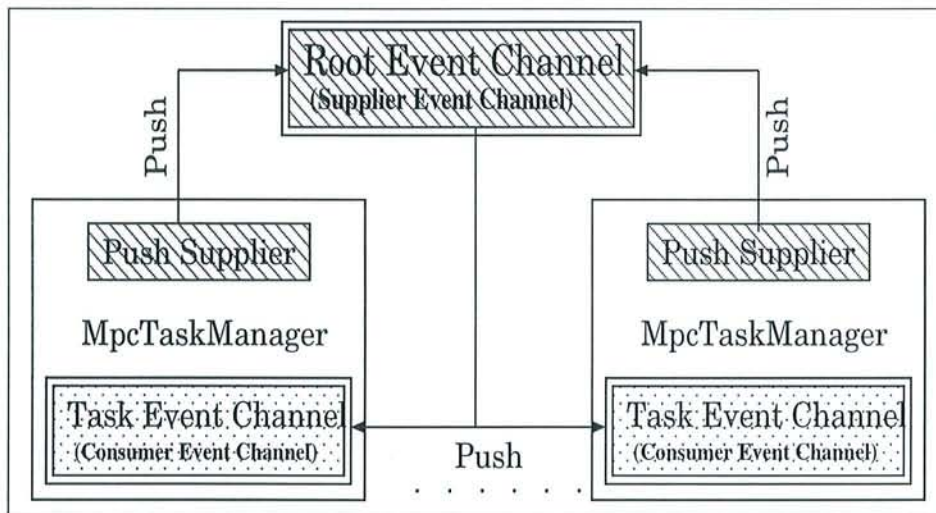
FIG. 10.15 – La connexion gestionnaire de groupe et MPCRoot
