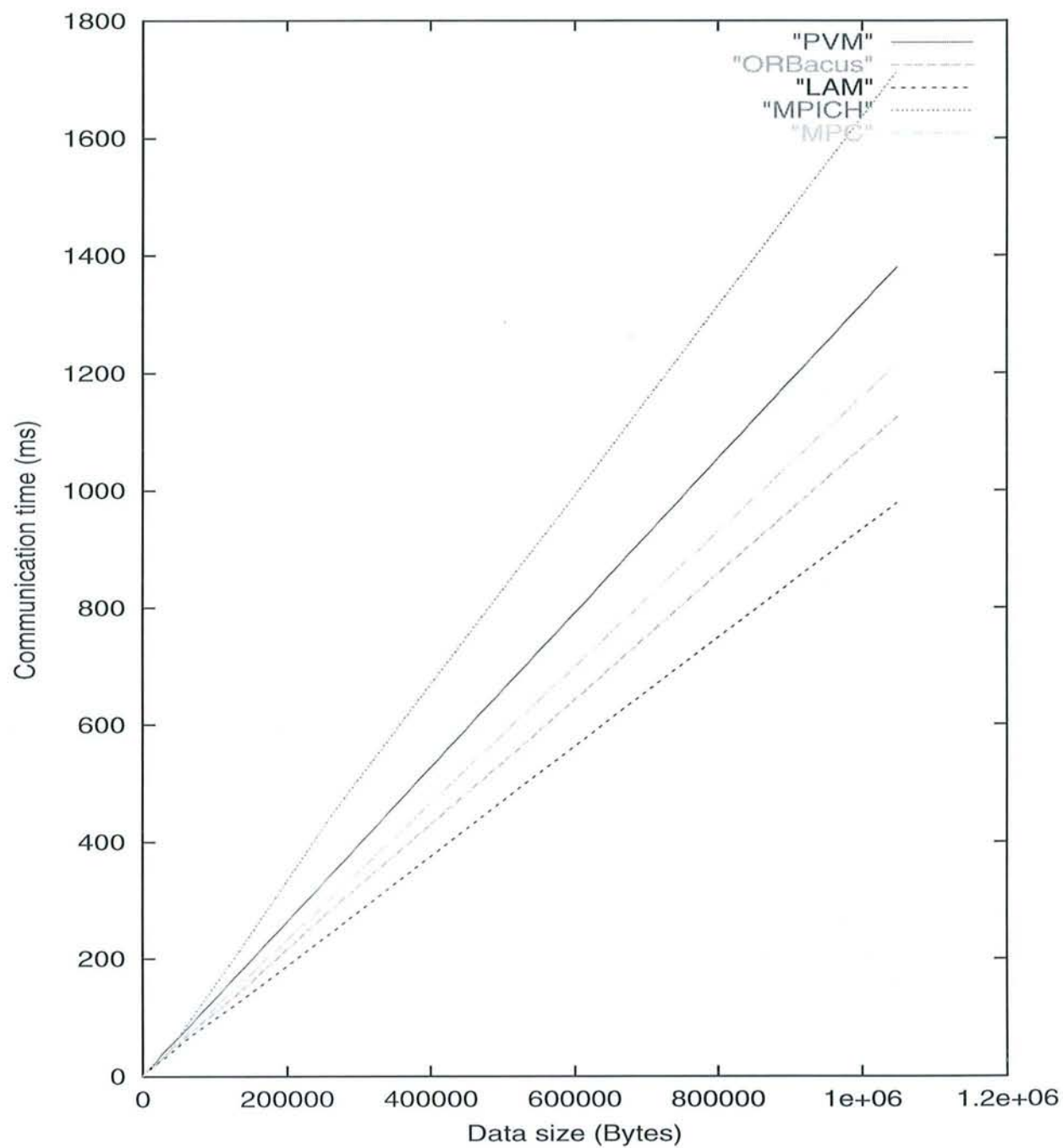
FIG. 10.8 – Comparaison des performances des communications entre ORBacus, MPC, MPICH, LAM et PVM
