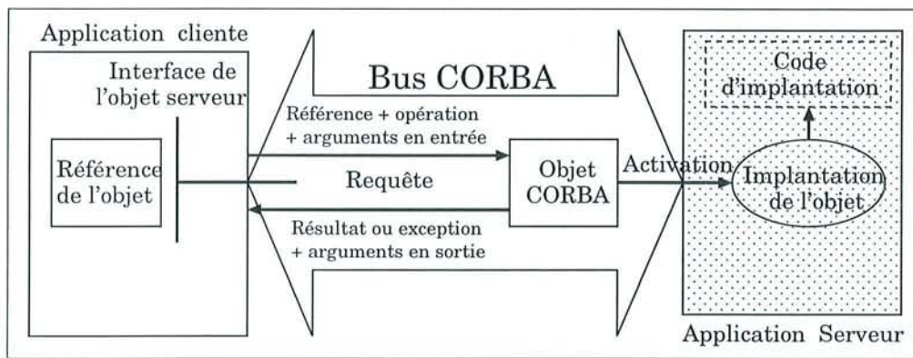
FIG. 3.2 – Le modèle objet client/serveur de CORBA
