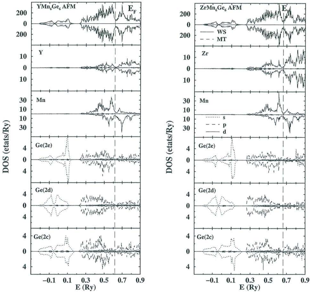
Figure 3.8 : Courbes de densité d'états des composés \text{YMn}_6\text{Ge}_6 et \text{ZrMn}_6\text{Ge}_6 dans l'état antiferromagnétique (+ - +).
