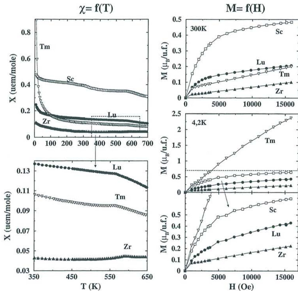
Figure 5.2 : Courbes magnétiques isochoamps ( H_{appl} = 0, 6 \text{ T} ) et isothermes (300 K et 4,2 K) des composés R_{1-\delta}\text{Fe}_6\text{Sn}_6 ( R = \text{Sc}, \text{Tm}, \text{Lu} et \text{Zr} ).
