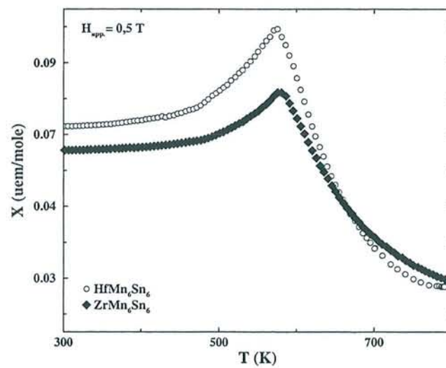
Figure 2.10 : Variation thermique de la susceptibilité magnétique de \text{ZrMn}_6\text{Sn}_6 et \text{HfMn}_6\text{Sn}_6 entre 300 K et 800 K ( H_{\text{appl}} = 0,5 \text{ T} ).
