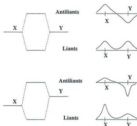
Figure 4.16 : Représentation schématique de l'effet du magnétisme covalent pour les composés RFe_6Ge_6 .
