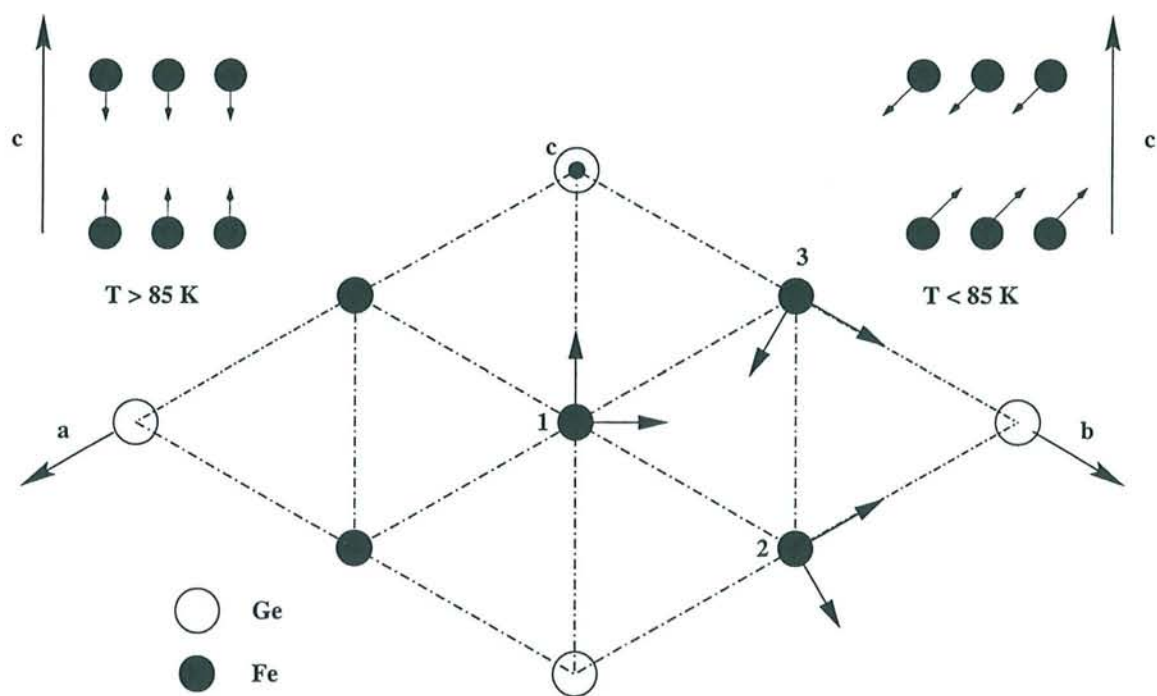
Figure 4.5.a : Orientation des axes du tenseur GCE dans les composés R\text{Fe}_6\text{Ge}_6 .
