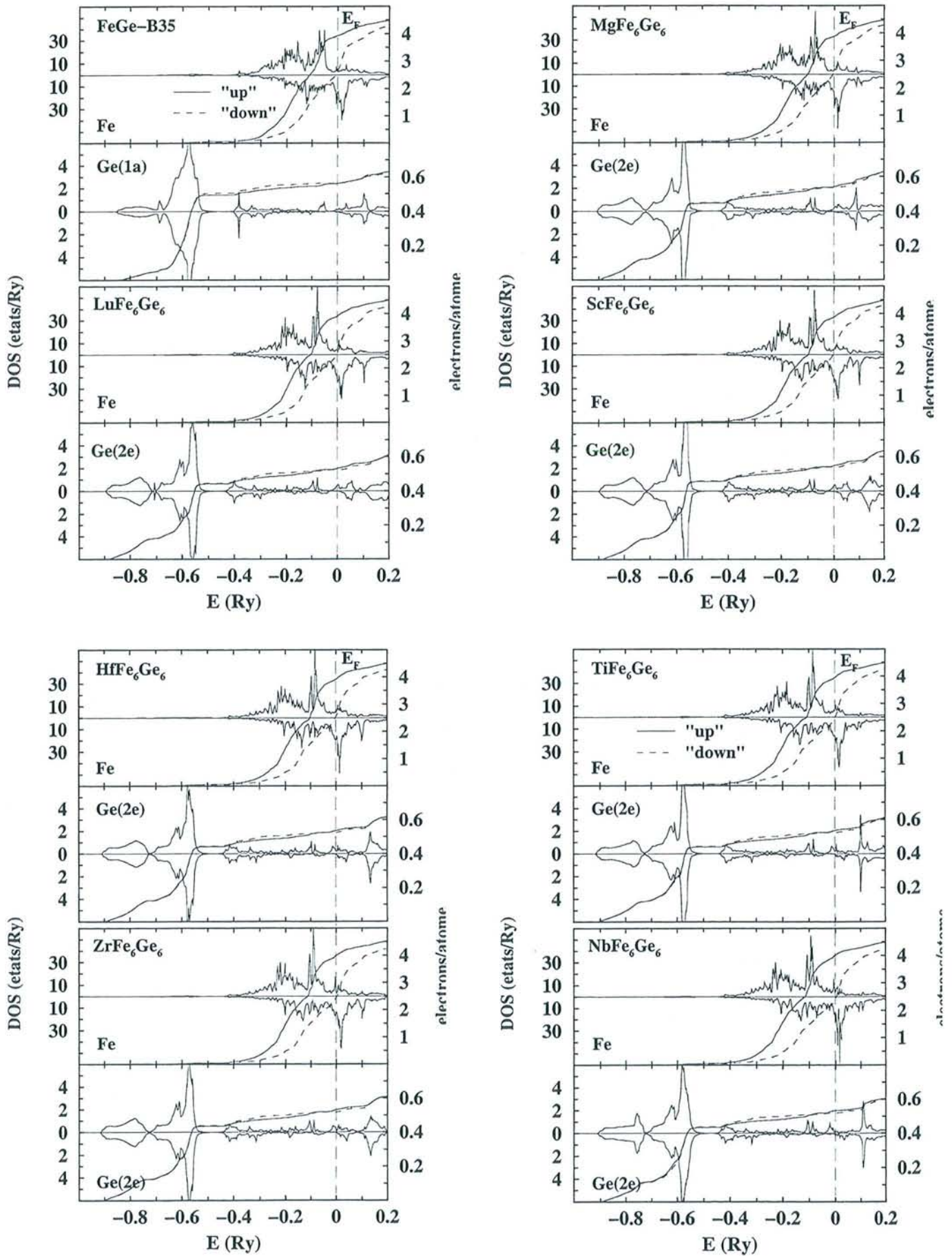
Figure 4.18 : Densité d'états d sur le site Fe et s sur le site Ge(2e) (Ge(1a)) pour FeGe-B35) dans les composés R\text{Fe}_6\text{Ge}_6 en compagnie des courbes correspondantes de remplissage des états électroniques pour les deux directions de spin.
