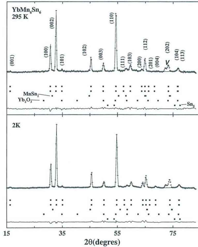
Figure 2.7 : Diagrammes de diffraction neutronique de \text{YbMn}_6\text{Sn}_6 à 300 K et 2 K ( \lambda = 2,52\text{ \AA} ).
