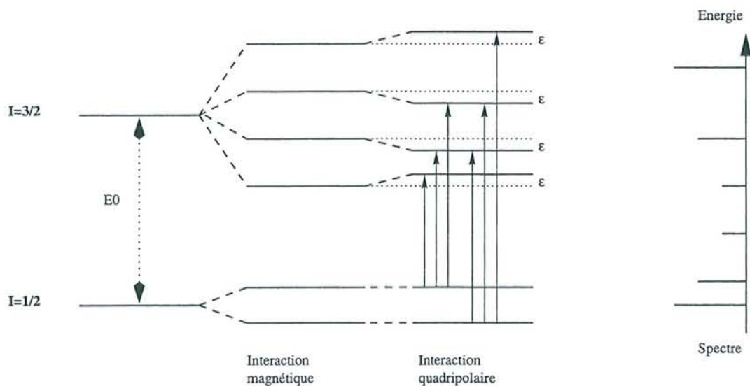
Figure A.3 : Interactions quadripolaire et magnétique combinées.
