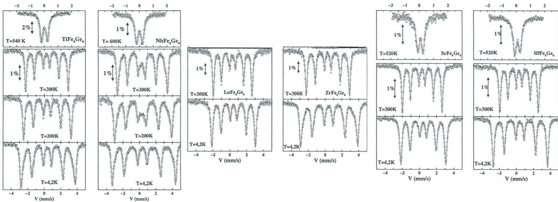
Figure 4.9 : Spectres Mössbauer ^{57}\text{Fe} des composés \text{RFe}_6\text{Ge}_6 ( \text{R} = \text{Sc}, \text{Lu}, \text{Ti}, \text{Zr}, \text{Hf} et \text{Nb} ).
