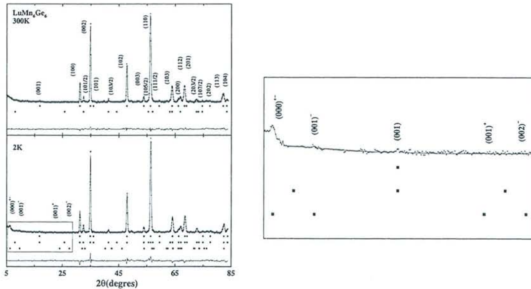
Figure 3.5 : Diffractogrammes neutroniques de \text{LuMn}_6\text{Ge}_6 à 300 K et 2 K ( \lambda = 2,487 Å).
