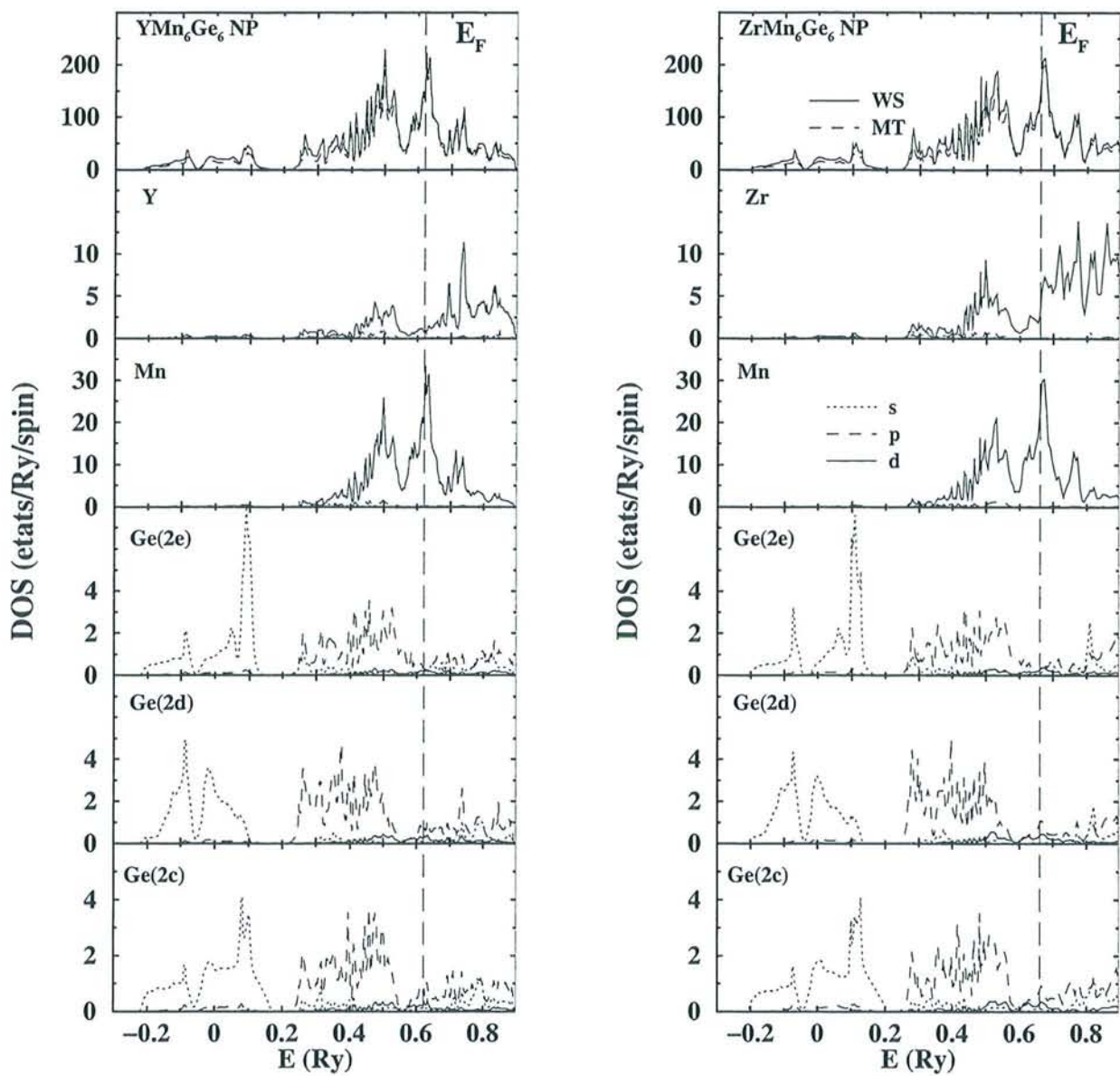
Figure 3.7 : Courbes de densité d'états des composés \text{YMn}_6\text{Ge}_6 et \text{ZrMn}_6\text{Ge}_6 dans l'état non polarisé (NP).
