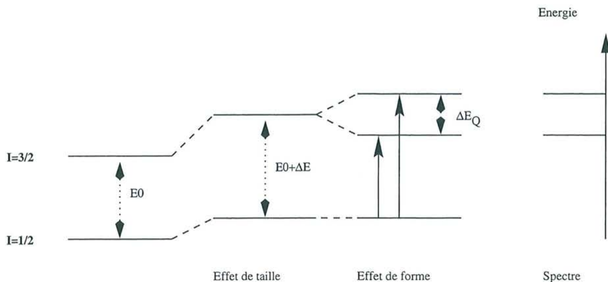
Figure A.1 : Interactions électriques monopolaire et quadripolaire.
