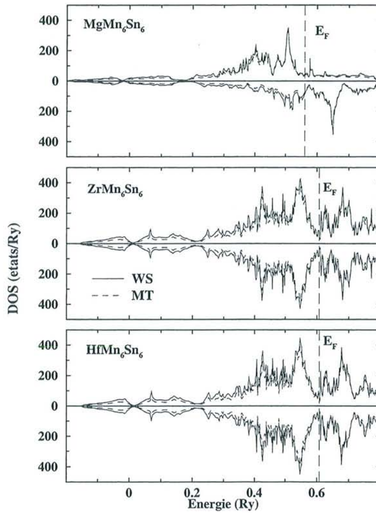
Figure 2.18 : Courbes de densité d'états totale dans l'état magnétique pour \text{MgMn}_6\text{Sn}_6 (FM), \text{ZrMn}_6\text{Sn}_6 (AFM) et \text{HfMn}_6\text{Sn}_6 (AFM).
