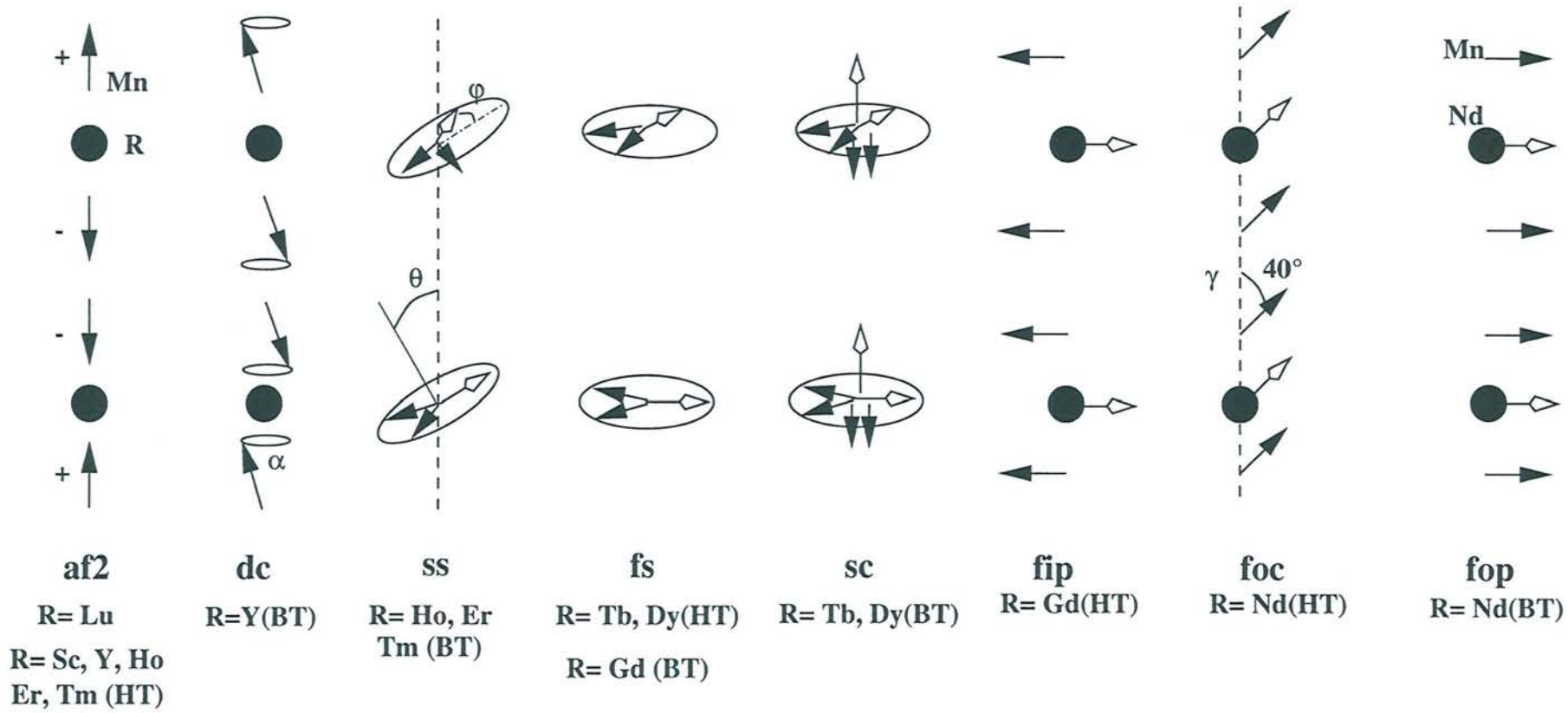
Figure 3.1 : Représentation schématique des différents arrangements magnétiques existant dans la série \text{RMn}_6\text{Ge}_6 ( \text{R} = \text{Sc}, \text{Y}, \text{Nd}, \text{Gd-Tm}, \text{Lu} ).
