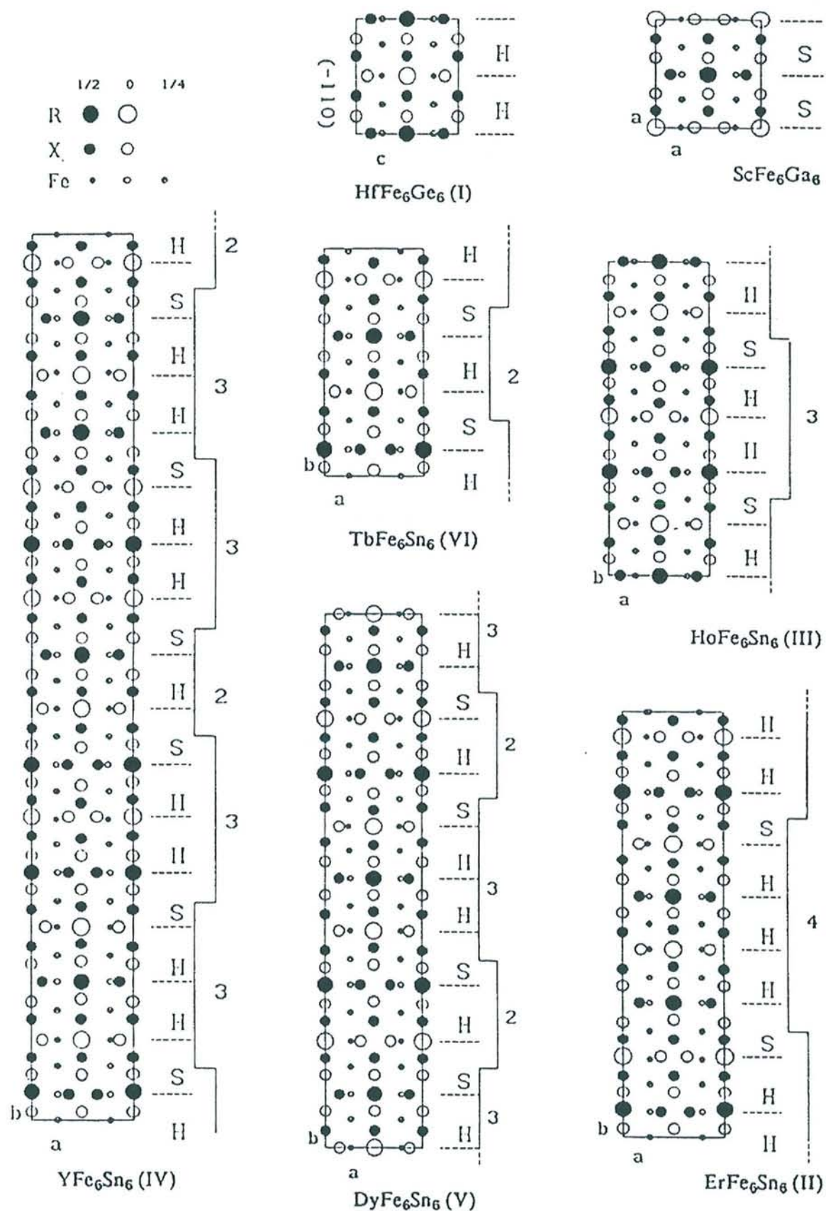
Figure 1.4 : Projections des différentes surstructures des types \text{YCo}_6\text{Ge}_6 et \text{SmMn}_6\text{Sn}_6 d'après [4] (H et S se réfèrent aux tranches \text{HfFe}_6\text{Ge}_6 et \text{ScFe}_6\text{Ga}_6 ).
