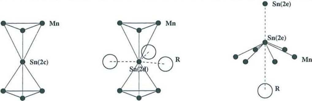
Figure 2.14 : Environnements des trois sites d'étain dans les composés \text{RMn}_6\text{Sn}_6 isotypes de \text{HfFe}_6\text{Ge}_6 .
