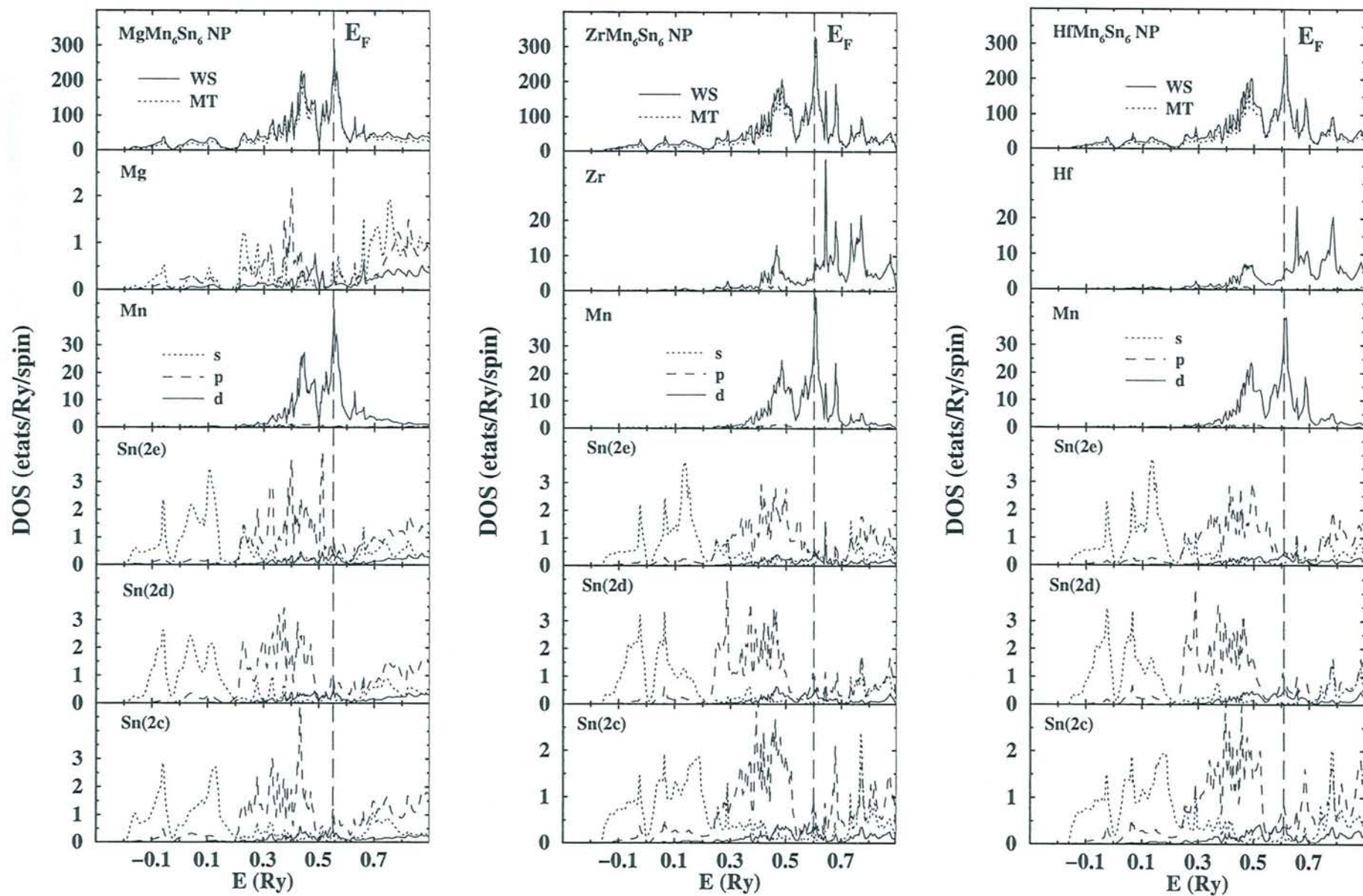
Figure 2.16 : Courbes de densité d'états des composés \text{RMn}_6\text{Sn}_6 ( \text{R} = \text{Mg}, \text{Zr} et \text{Hf} ) issues des calculs non polarisés (NP).
