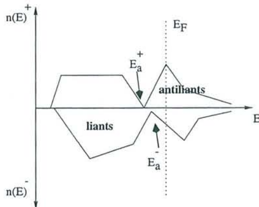
Figure C.3 : Représentation schématisée de la densité d'états s de l'impureté sp .
