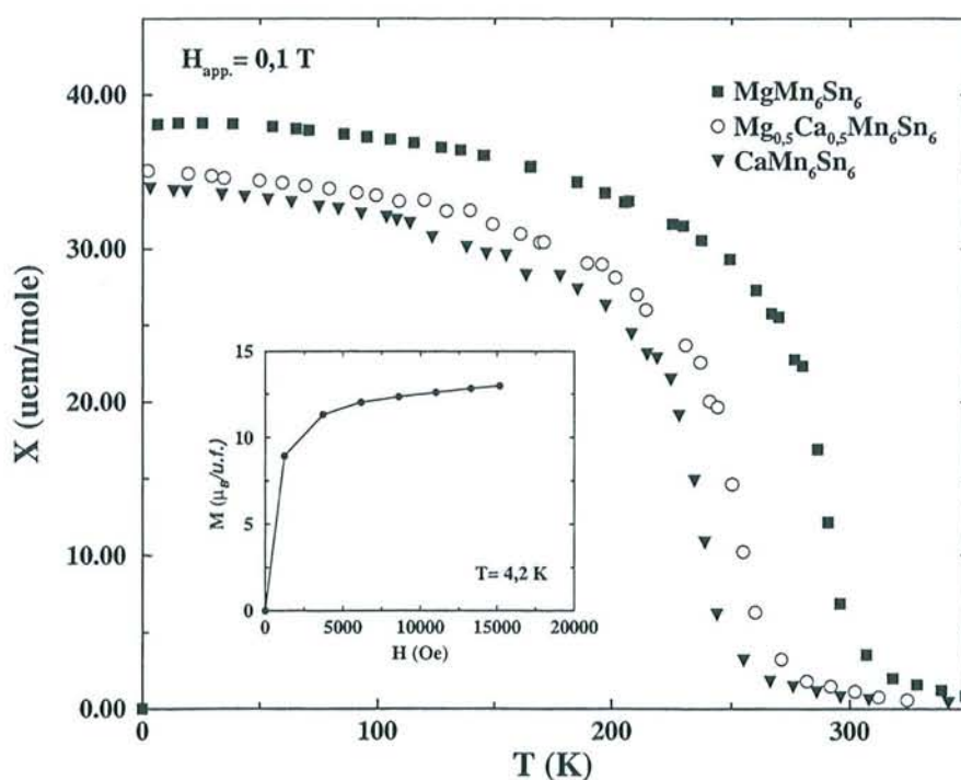
Figure 2.8 : Courbes magnétiques isochoamps ( H_{\text{appl}} = 0, 1 \text{ T} ) des composés \text{Mg}_{1-x}\text{Ca}_x\text{Mn}_6\text{Sn}_6 ( x=0 ; x=0,5 ; x=1 ). Courbe isotherme de \text{MgMn}_6\text{Sn}_6 .
