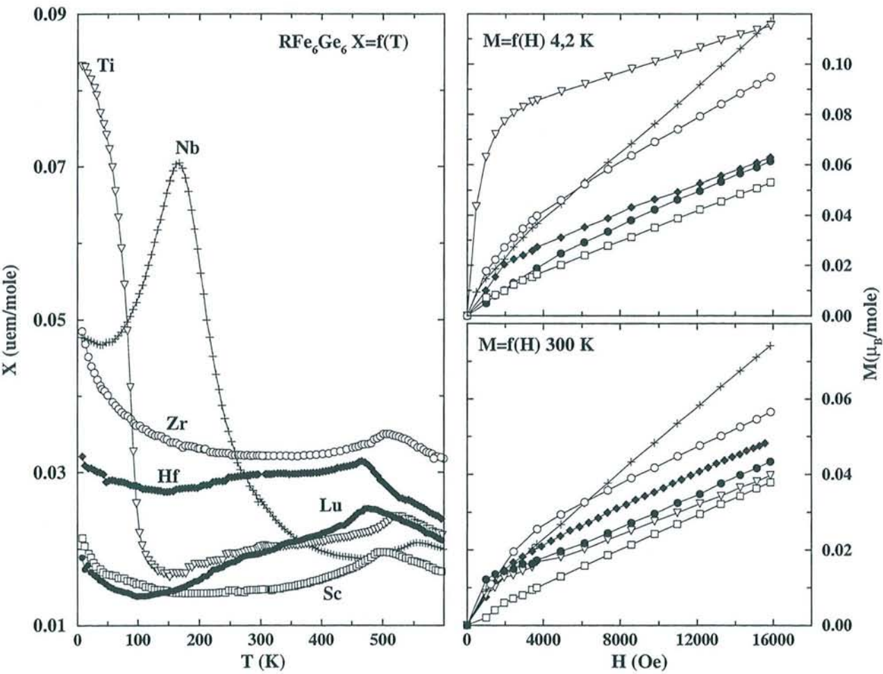
Figure 4.2 : Courbes magnétiques isochoamps ( H_{appl} = 0,6\ T ) et isothermes ( T= 300\ K et 4,2\ K ) des composés RFe_6Ge_6 ( R= Sc, Lu, Ti, Zr, Hf, Nb ).
