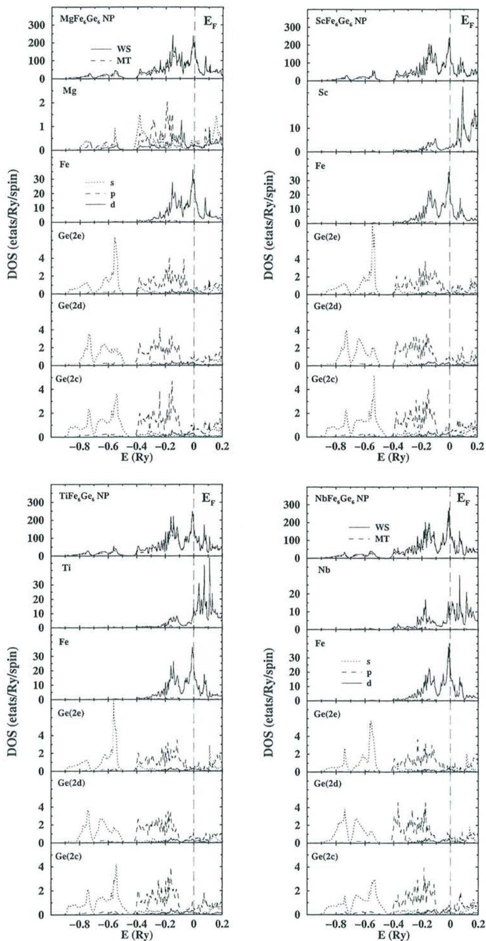
Figure 4.11.b : Courbes de densité d'états (calculs non polarisés) des composés R\text{Fe}_6\text{Ge}_6 ( R = \text{Mg}, \text{Sc}, \text{Ti} et \text{Nb} ).
