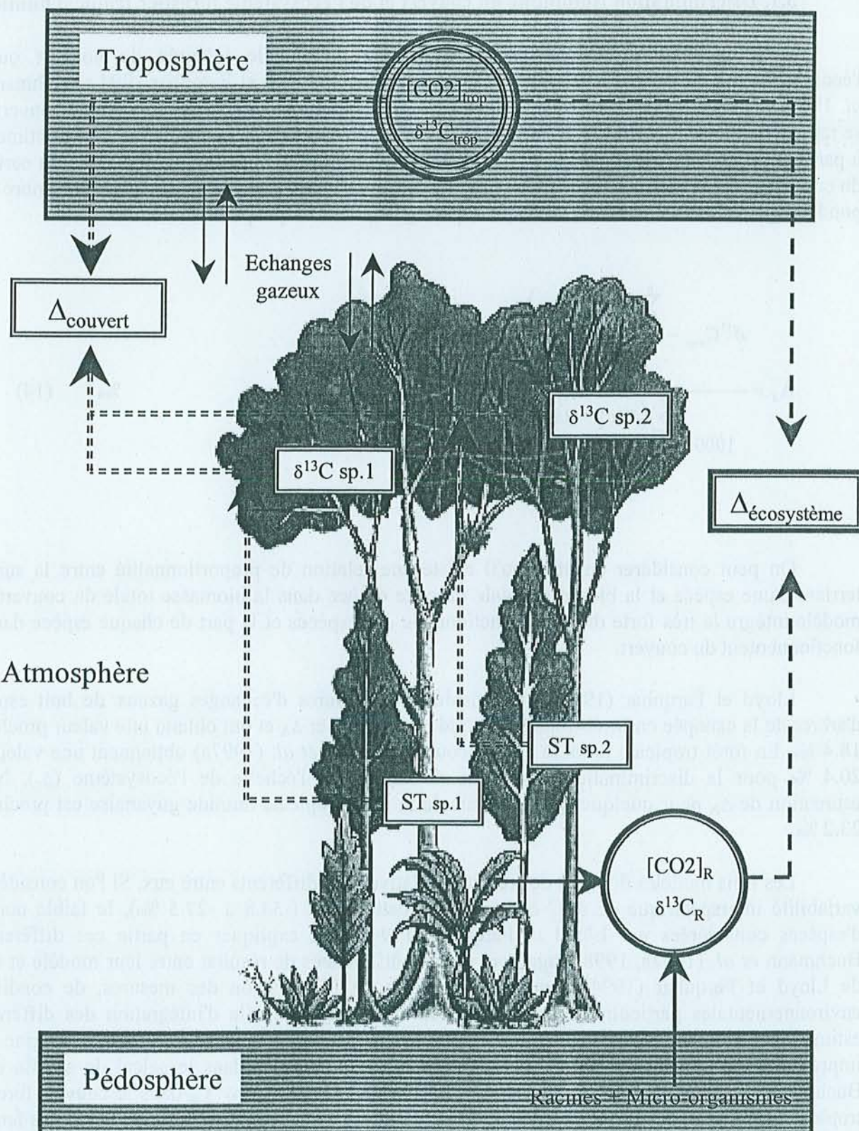
Fig. 11. Schéma conceptuel illustrant le modèle de discrimination isotopique du carbone de l'écosystème ( \Delta_e , Buchmann et al. 1997a) (trait simple pointillé) et de discrimination isotopique du carbone du couvert ( \Delta_A , A-I) (double trait pointillé). Pour la correspondance des symboles, voir la liste des abréviations ou le texte. Les flèches pleines correspondent aux échanges gazeux ; les flèches pointillés décrivent les mécanismes du modèle.
