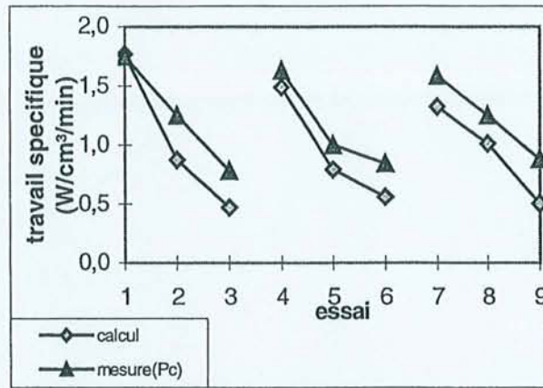
Figure 54 : Travail spécifique de coupe (W/cm³/min) mesurées et calculées avec e_{max} .
