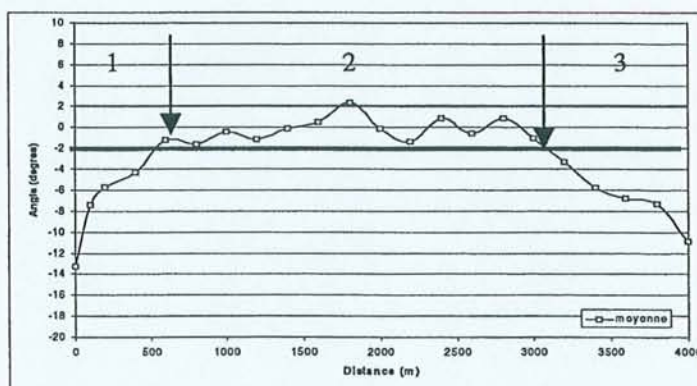
Figure 76 : Comportement de l'angle « F_c F_y » en fonction de la distance de bois usinée.
