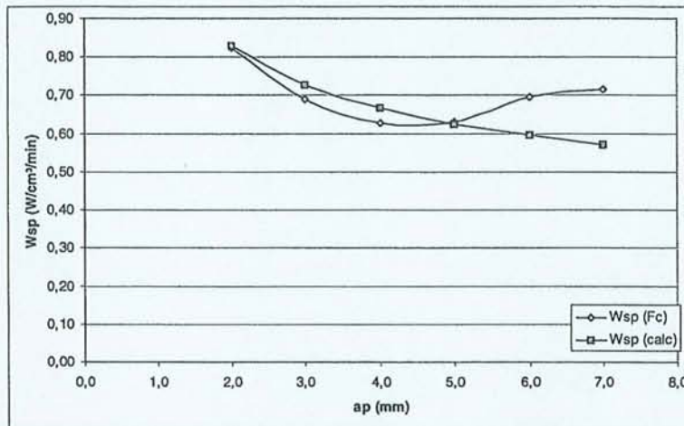
Figure 67 : Evolution du travail spécifique en fonction de l'engagement radial « a_p » par mesure d'efforts de coupe.
