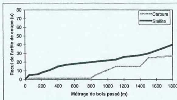
Figure 18: Comparaison entre le carbure de tungstène et le stellite, le recul de l'arête de coupe ( \mu ) d'après le mètre de bois passé (m) [DRE86].
