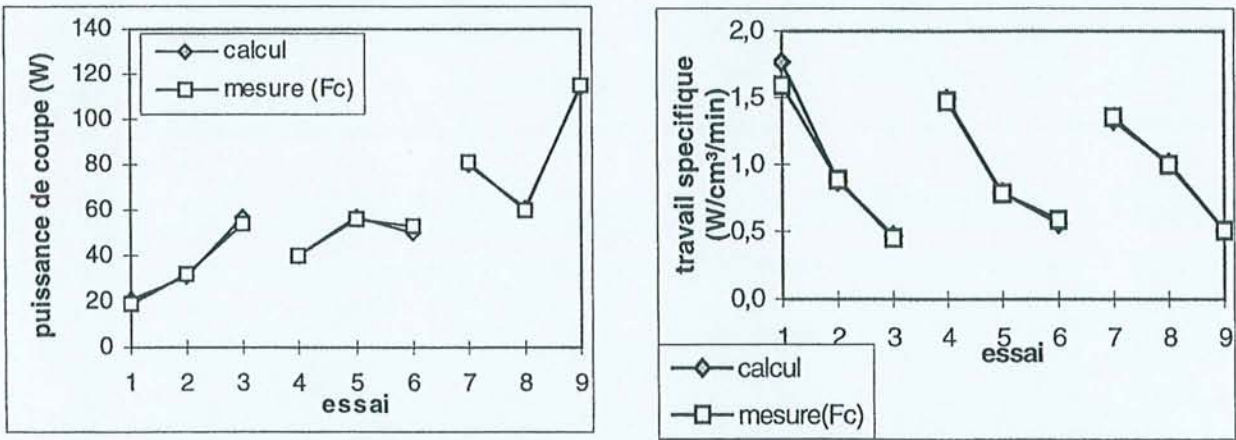
Figure 51: Rapport puissance de coupe (W) calculée et mesurée.
