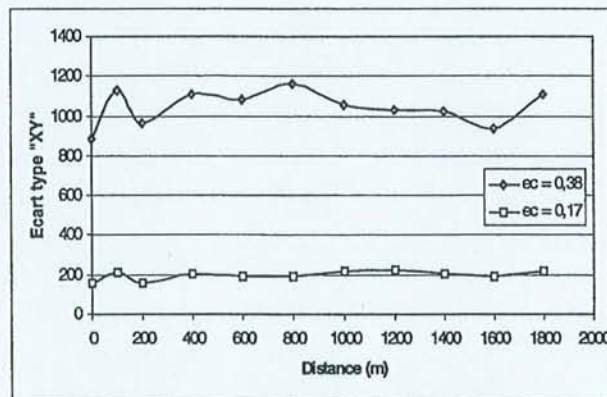
Figure 83 : Les états de surface par rapport à l'usure de l'outil et à l'épaisseur de copeau.
