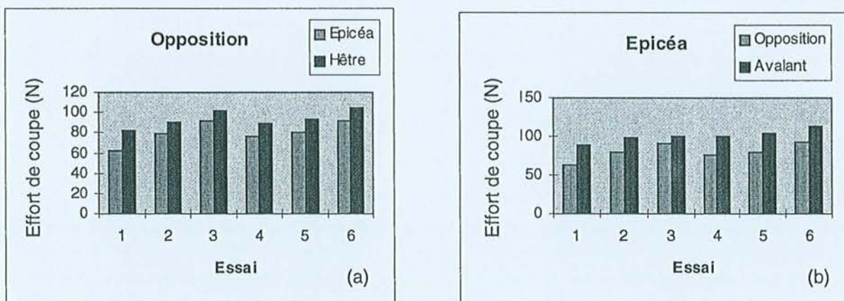
Figure 14 : Résultats des mesures des efforts de coupe dans l'épicéa et du hêtre, d'après un changement du niveau de la profondeur de passe (essais 1-3 ; 3 mm et 4-6 ; 5 mm), travail en opposition (a), et l'effet du mode d'usinage sur l'épicéa (b).
