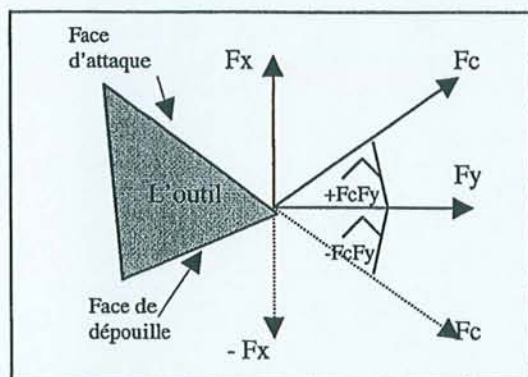
Figure 75 : L'angle « F_c F_y » pour mesurer l'usure.
