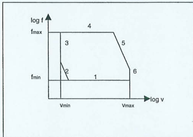
Figure 19 : Domaine des contraintes d'après [MAR80].
