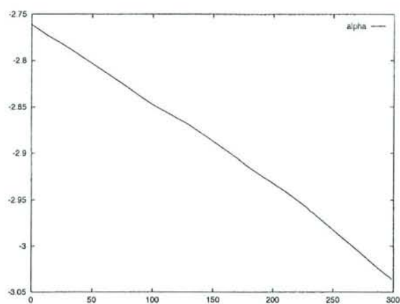
FIG. 6.9 – Évolution de l'angle \alpha sur la séquence du Pont-Neuf.
