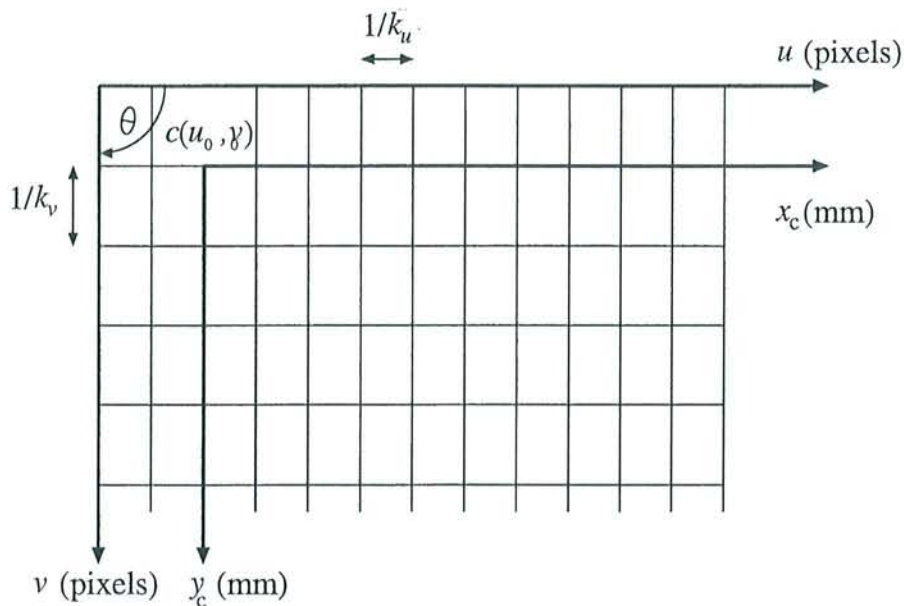
FIG. 2.2 – Les paramètres intrinsèques
