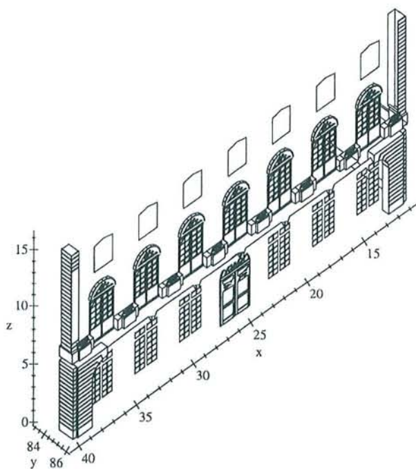
FIG. 5.25 – Modèle filaire de la façade de l'Opéra de Nancy.
