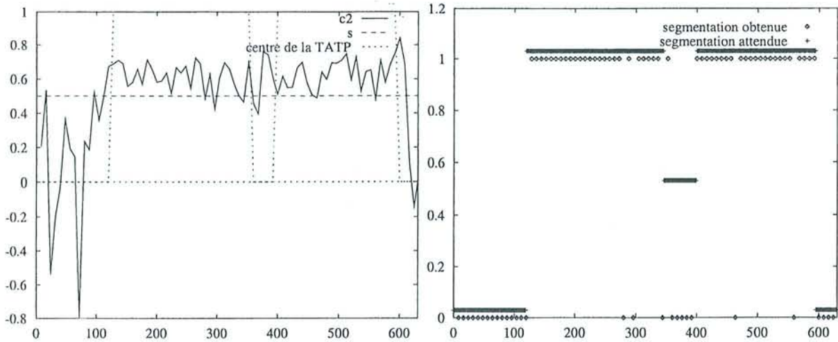
FIG. 7.22 – Valeurs du critère c_2 (à gauche) et résultat de la segmentation (à droite) sur la séquence du loria.
