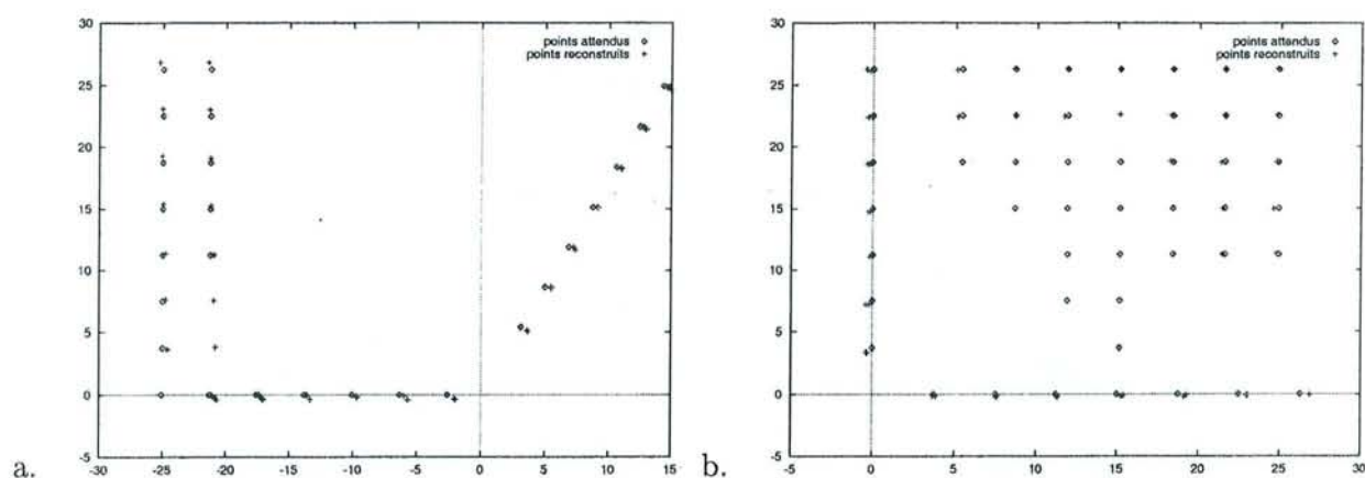
FIG. 7.17 – Projection des points reconstruits dans les plan (xy) et (yz) pour l'optimisation alternée. Les croix sont les points reconstruits et les cercles les points attendus.
