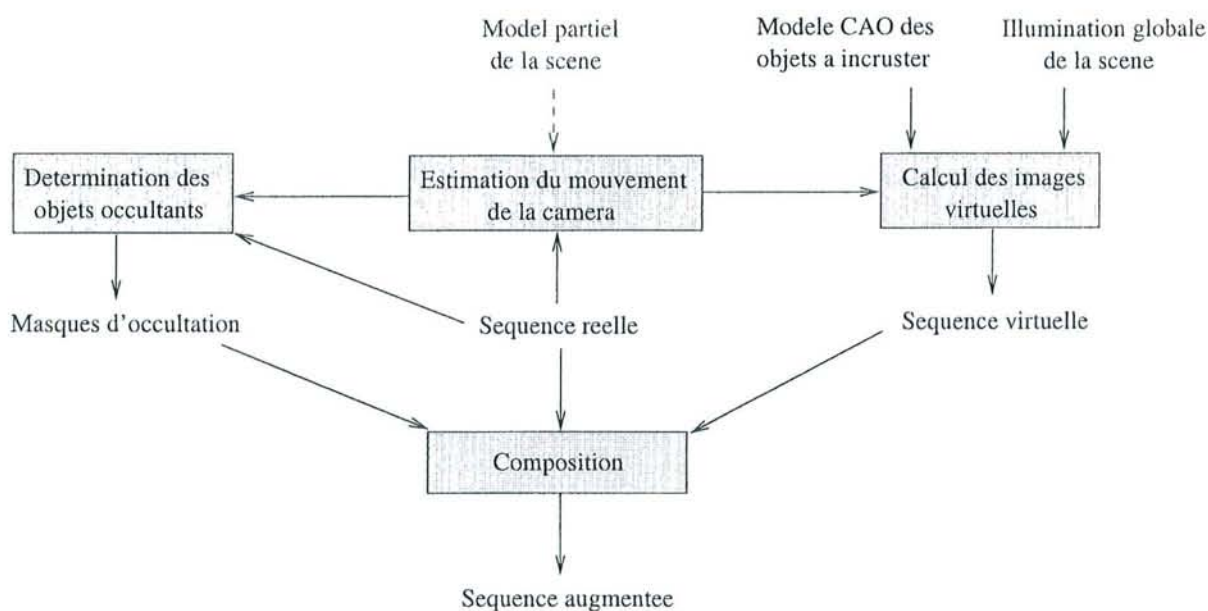
FIG. 3.1 – Schéma général d'un système de RA.
