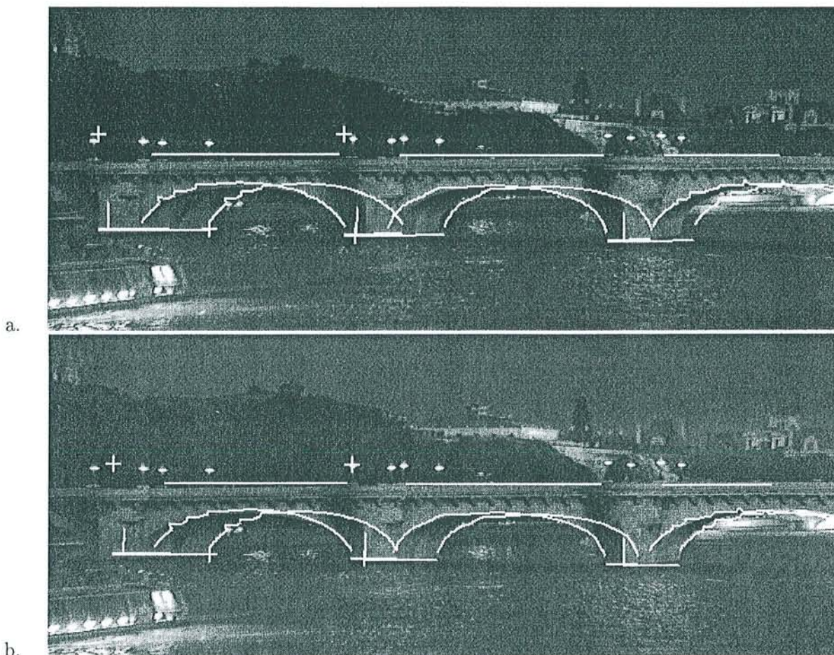
FIG. 4.5 – Initialisation. a. Estimation initiale par la méthode de Dementhon et Davis appliquée à quatre points non coplanaires. b. Estimation affinée obtenue après 23 itérations de l'algorithme de Powell.
