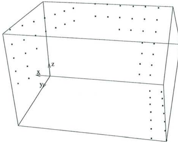
FIG. 7.3 – Les points de la mire reconstruits à partir des images 0 et 20 pour l'optimisation à neuf paramètres.
