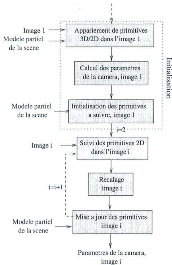
FIG. 3.2 – La boucle de recalage temporel pour un système de RA basé modèle.
