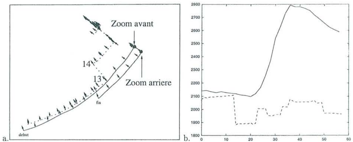
FIG. 7.2 – Paramètres de la caméra attendus (traits continus) et calculés (traits discontinus) pour une optimisation à neuf paramètres sur la séquence de la cabane. a. Projection de la trajectoire de la caméra dans le plan horizontal. b. Paramètre \alpha_u .
