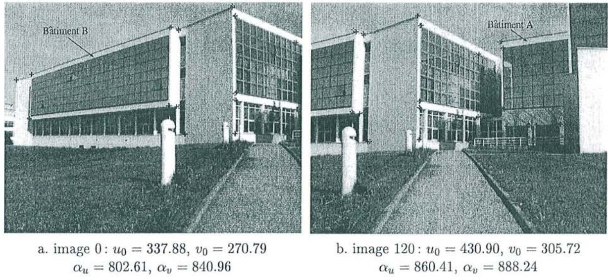
FIG. 7.21 – Points appariés et paramètres intrinsèques obtenus pour les images 0 et 120 de la séquence. Les croix continues indiquent les points 2-D extraits dans l'image et les croix discontinues la projection de leurs correspondants 3-D.
