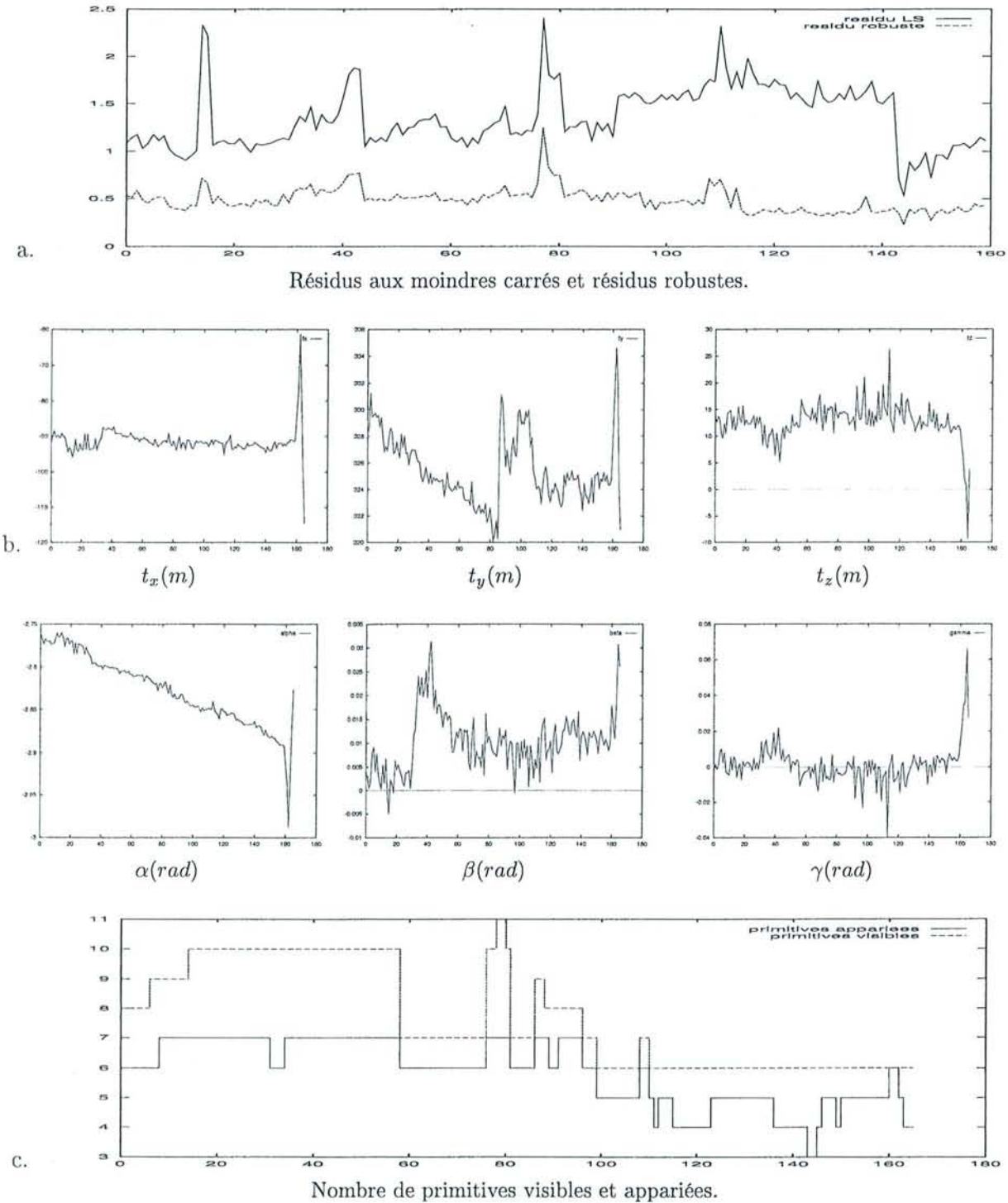
FIG. 5.15 – Résultats statistiques obtenus sur la séquence du Pont-Neuf.
