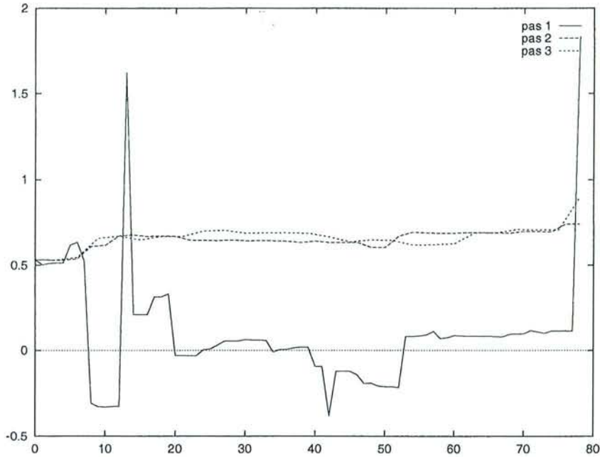
FIG. 6.4 – Influence du pas entre les images sur t_z pour la séquence de la place Stanislas.
