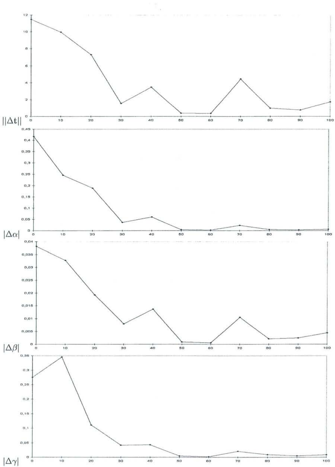
FIG. 5.23 – Erreur moyenne obtenue sur les paramètres du point de vue en fonction de la profondeur du modèle.
