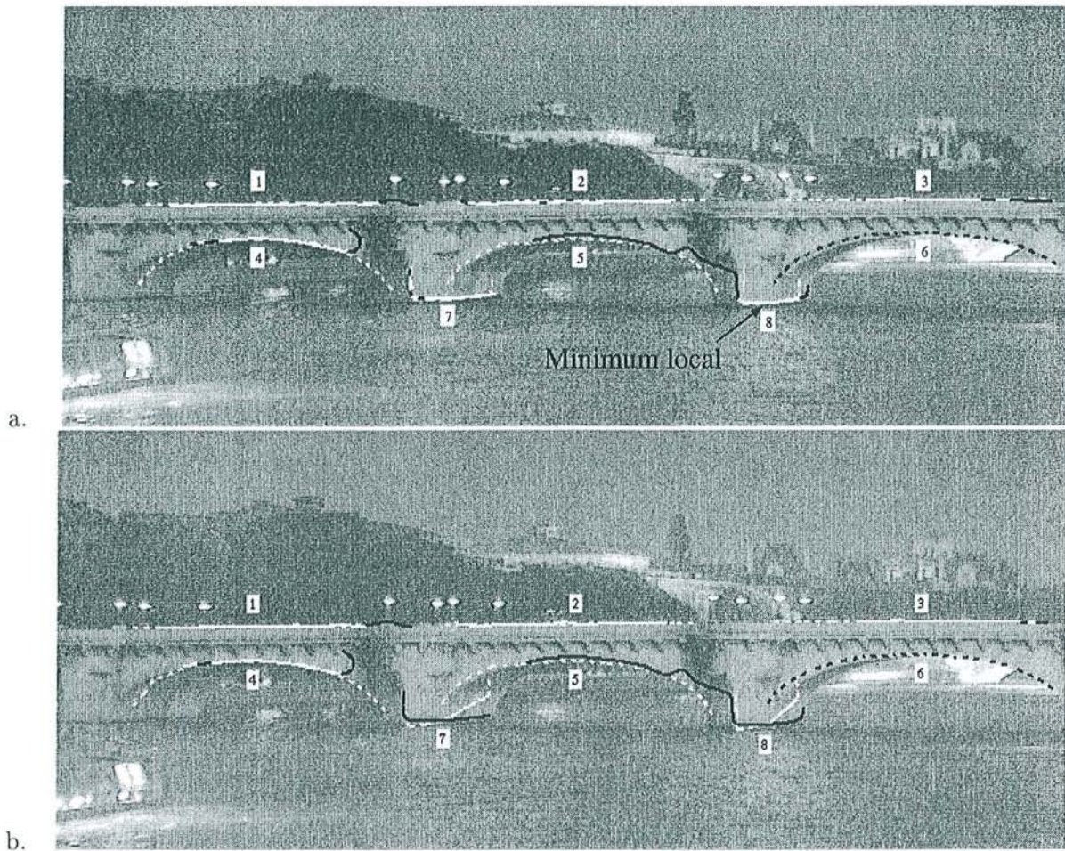
FIG. 5.13 – Exemples de problèmes inhérents à l'utilisation d'estimateurs médians dans l'image 13 de la séquence du Pont Neuf. a. Utilisation de l'estimateur LTS au niveau local : un minimum local est obtenu pour la primitive 8. b. Utilisation de l'estimateur LTS au niveau global : les primitives 7 et 8 comportant l'information de profondeur ne sont pas prises en compte.
