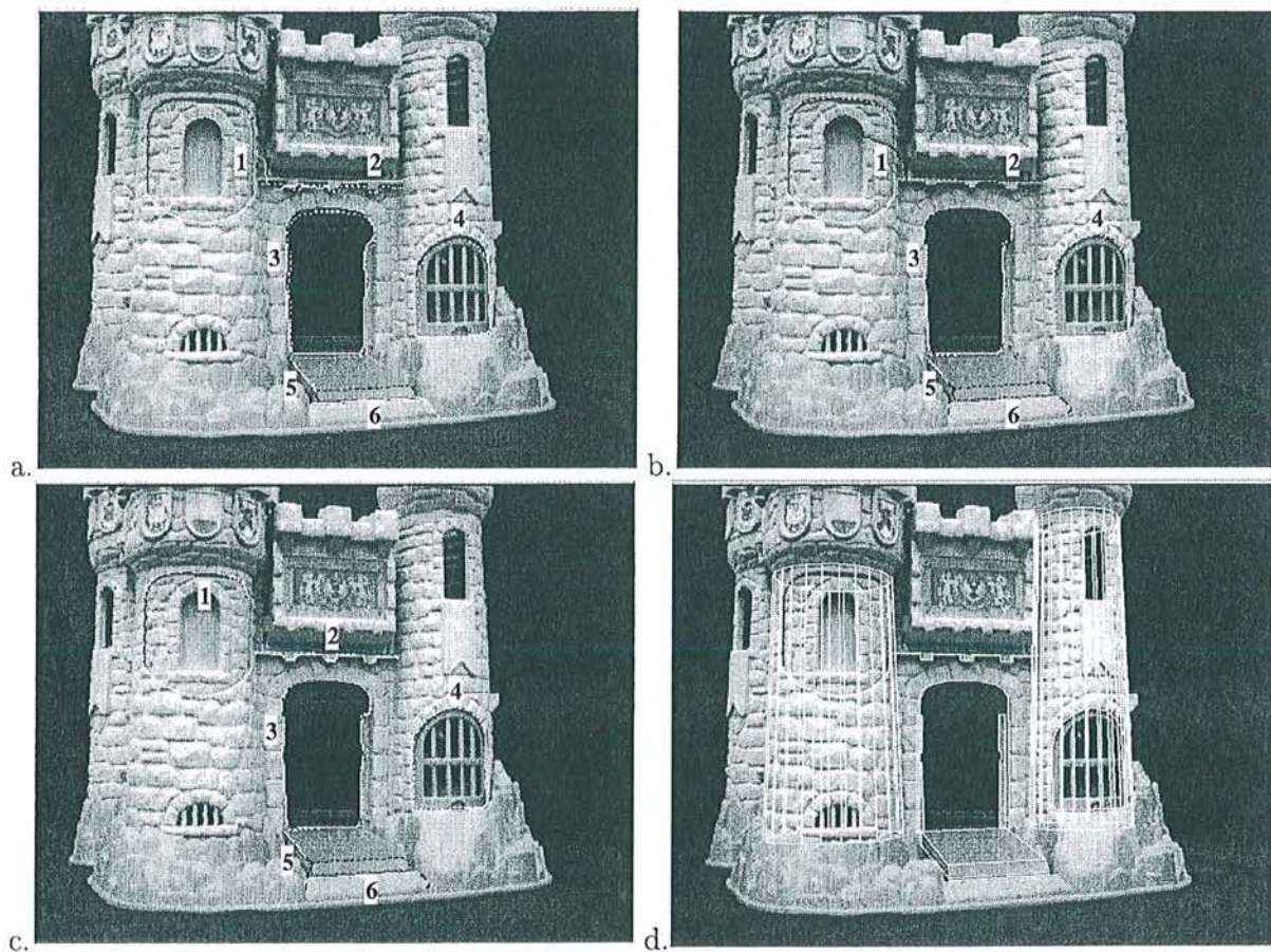
FIG. 5.19 – Recalage temporel dans une image de la séquence du château miniature. a. Suivi des primitives. b. Recalage. c. Mise à jour des primitives. d. Projection du modèle filaire du château.
