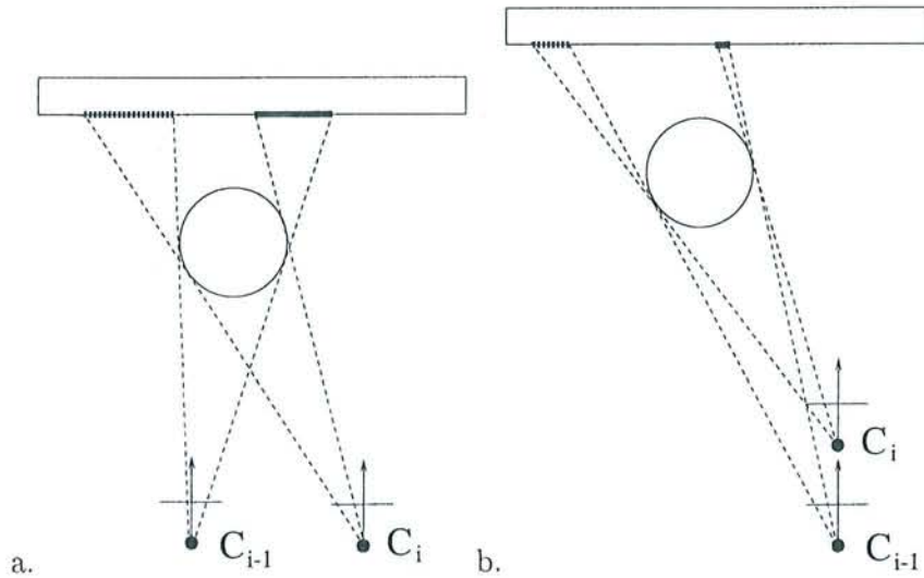
FIG. 7.8 – Dans le cas d'un mouvement général de la caméra (a), des éléments de la scène apparaissent (trait épais) ou disparaissent (trait épais discontinu) autour des contours d'occultation. Ce constat est aussi valable pour les translations le long de l'axe optique (b).
