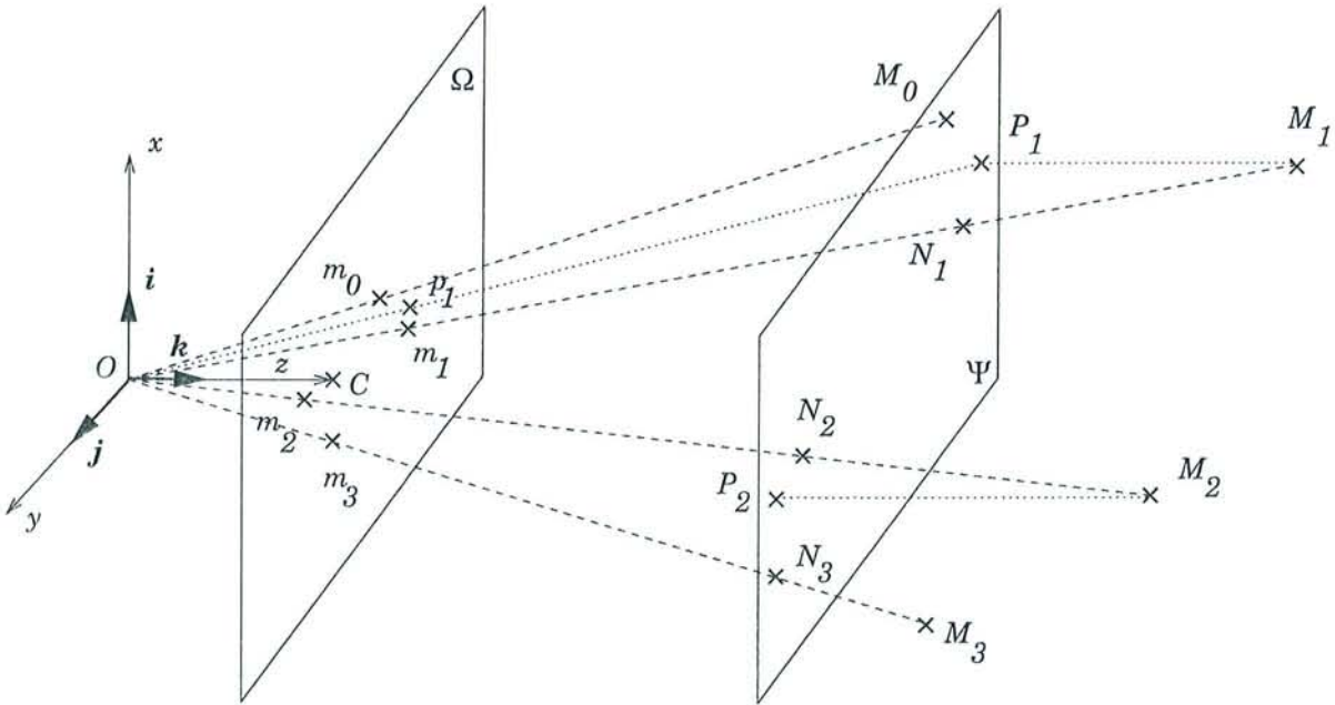
FIG. 4.2 – Illustration de la méthode de Dementhon et Davis.
