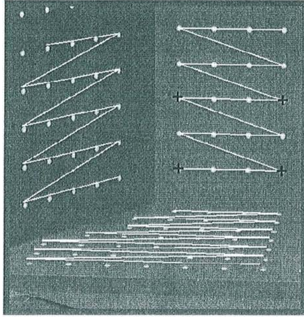
FIG. 4.1 – Calcul du point de vue par la méthode de Ferri et al., à partir de quatre points mesurés très précisément dans un même plan d'une mire de calibration.
