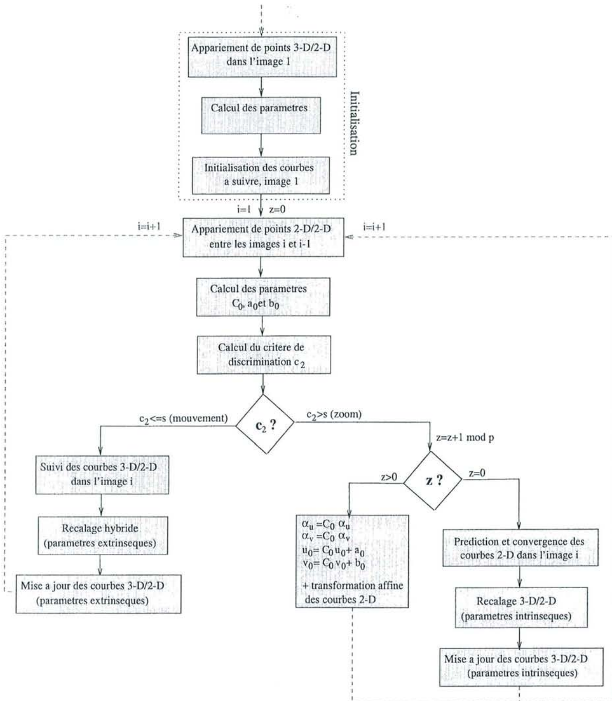
FIG. 7.10 – Boucle de recalage temporel pour une séquence à focale variable.
