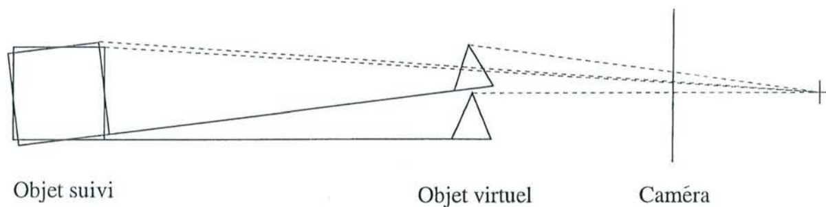
FIG. 5.24 – Une petite erreur de reprojection au niveau de l'objet suivi peut conduire à une incrustation complètement fausse pour un objet virtuel éloigné de l'objet ayant servi au calcul du point de vue.
