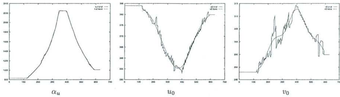
FIG. 7.29 – Paramètres intrinsèques de la caméra sur la séquence de la loria.
