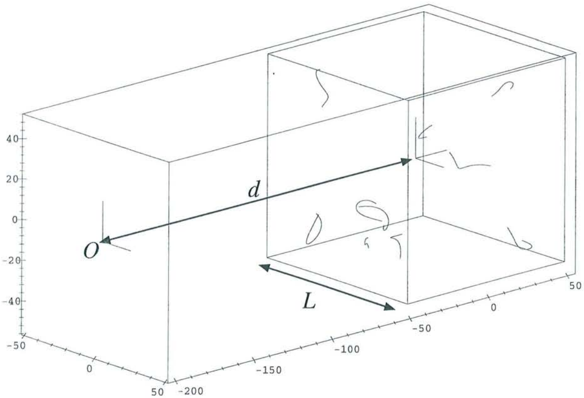
FIG. 5.3 – n courbes 3-D générées aléatoirement dans un cube de côté L , dont le centre est situé à une distance d du centre optique de la caméra ( n = 10 ; L = 100 ; d = 200 ).
