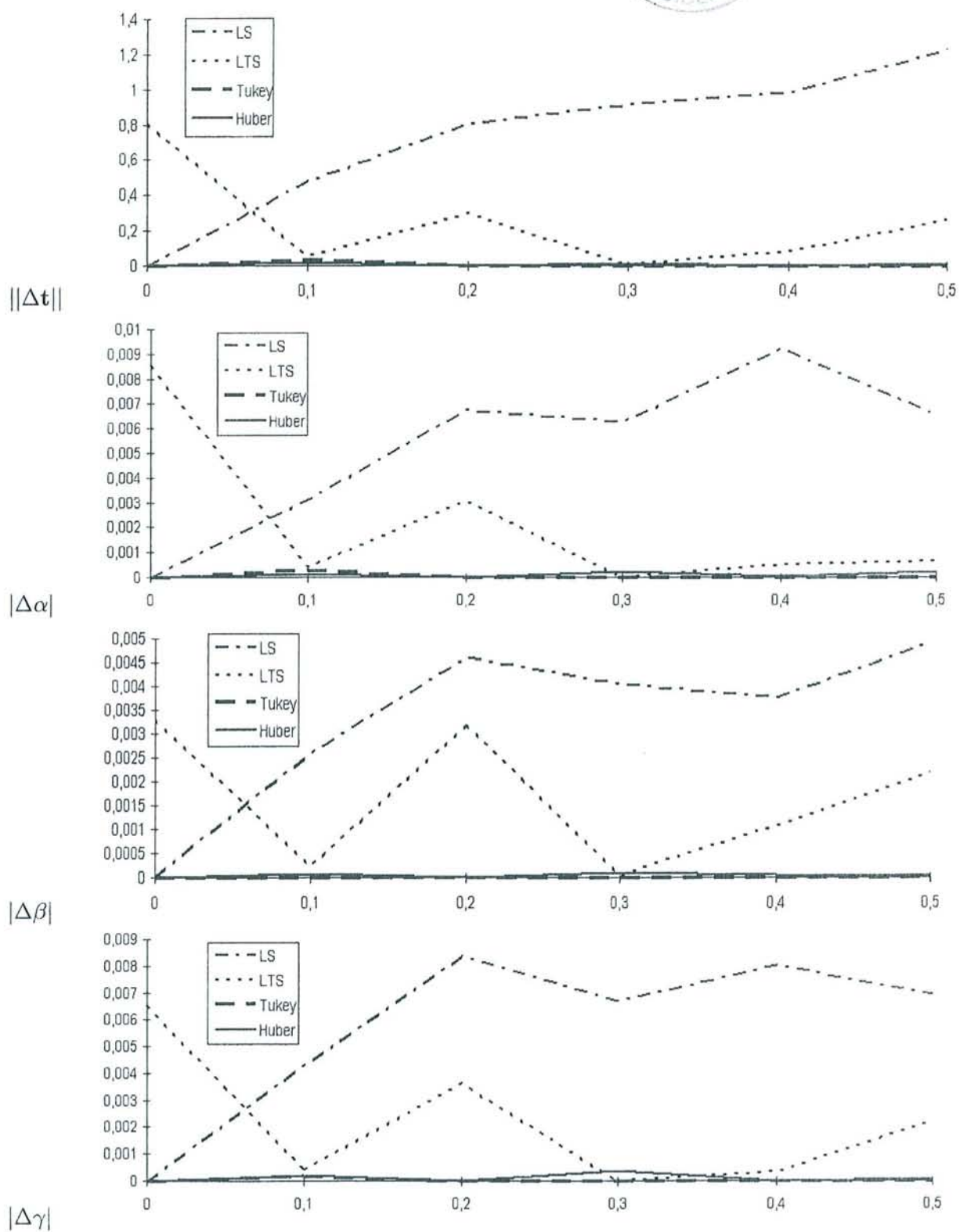
FIG. 5.7 – Influence des erreurs locales sur l'optimisation, pour différents estimateurs utilisés au niveau local.
