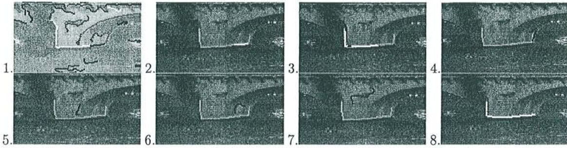
FIG. 5.10 – Exemple d'initialisation dans la séquence du Pont Neuf. 1 : carte des contours autour de la primitive projetée. 2 à 7 : test de rejet par la procédure R-courbe+ pour les 6 contours les plus proches de la projection. La projection de la primitive 3-D est dessinée en gris, les sections de contours conservées apparaissent en blanc et les sections rejetées ainsi que les contours globalement rejetés sont en noir. 8 : résultat final : la primitive retenue est la réunion des sections conservées.
