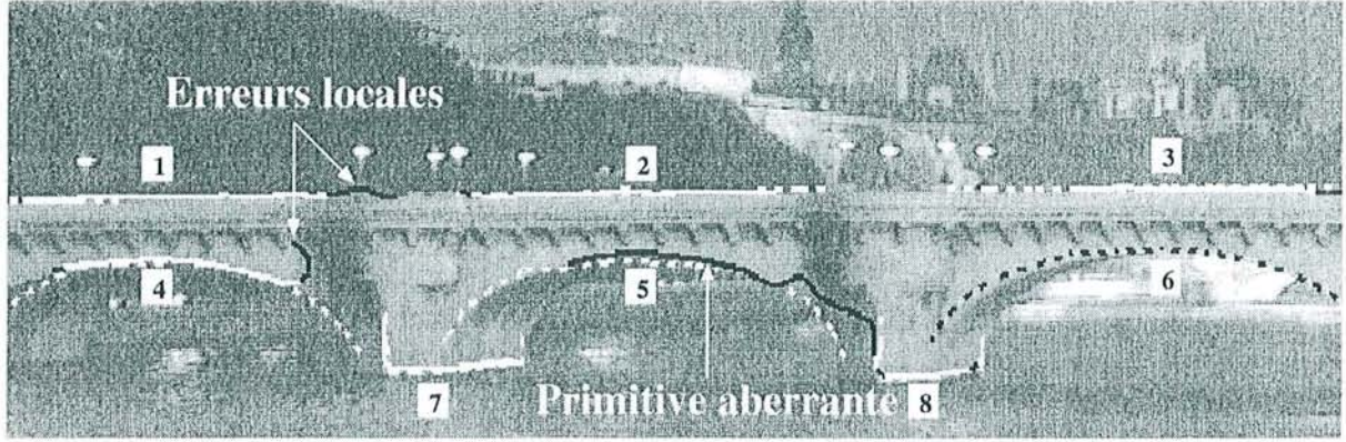
FIG. 5.1 – Exemple d'erreurs de suivi obtenues sur la séquence du Pont Neuf (une erreur local est obtenue pour les primitives primitives 1 et 4 et une erreur aberrante pour la primitive 5). Les conventions sont les suivantes : lignes blanches continues : primitives images (les sections en noir sont les parties dont l'influence est réduite lors de la minimisation, c'est-à-dire les points pour lesquels le résidu d_{i,j} est supérieur à c , donné en table 4.1) ; lignes blanches discontinues : projection des primitives 3-D correspondantes ; lignes noires continues : primitives aberrantes ; lignes noires discontinues : primitives non initialisées.
