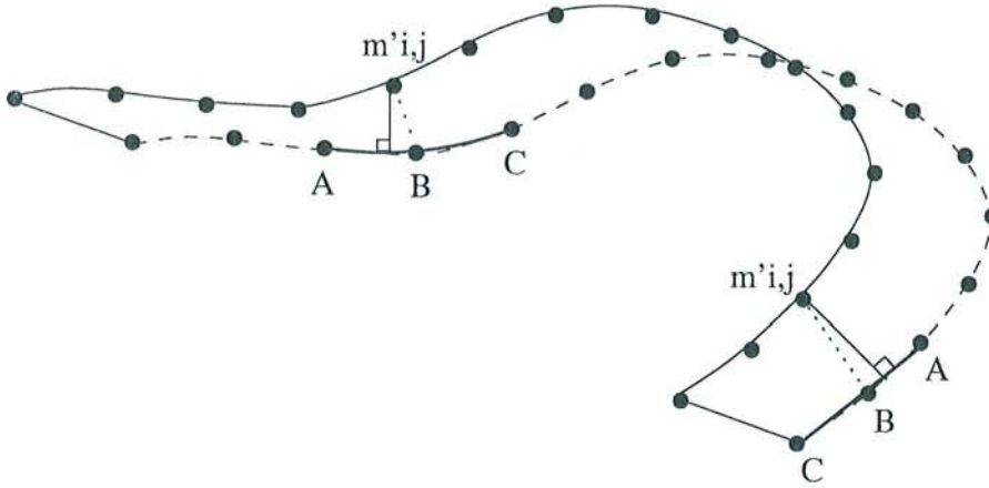
FIG. 5.2 – Approximation de la distance d'un point à une courbe. La distance est d'abord approximée par la longueur du segment discontinu, puis affinée par celle du segment continu.
