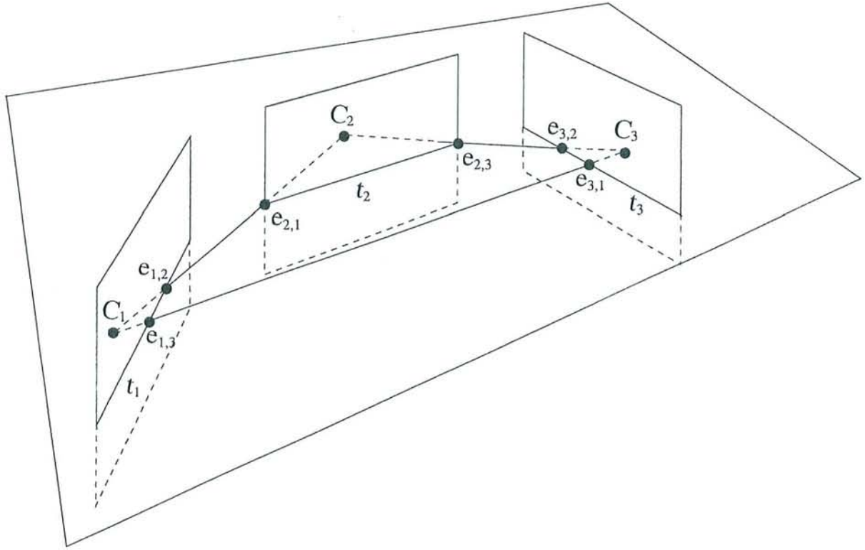
FIG. 2.6 – La géométrie trifocale.
