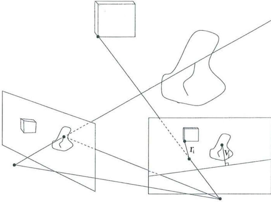
FIG. 6.1 – la méthode hybride consiste à minimiser simultanément les résidus modèle/image et les distances des points images aux droites épipolaires. Dans cet exemple, le cube est un objet dont le modèle est connu, alors que le second objet n'est pas nécessairement modélisé.
