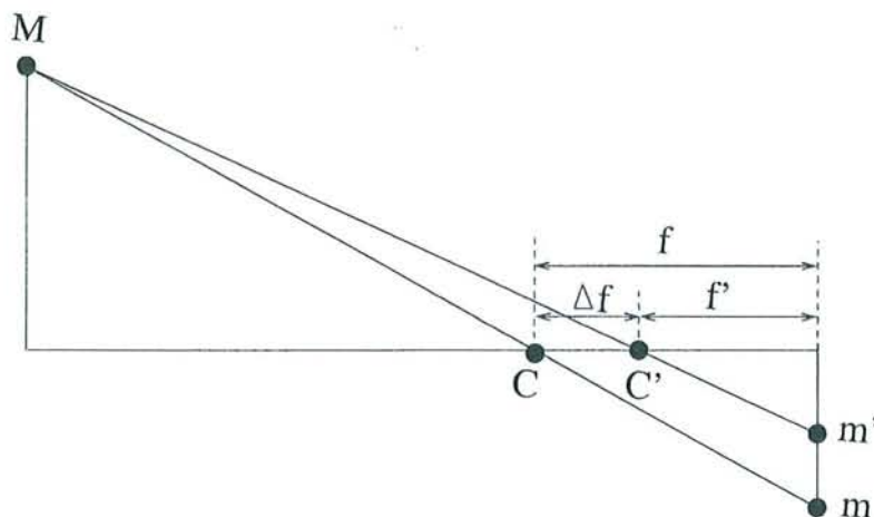
FIG. 2.7 – Déplacement du centre optique par changement de focale.
