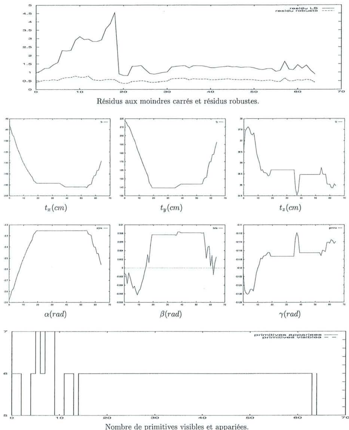
FIG. 7.14 – Résultats statistiques obtenus sur la séquence de la cabane.
