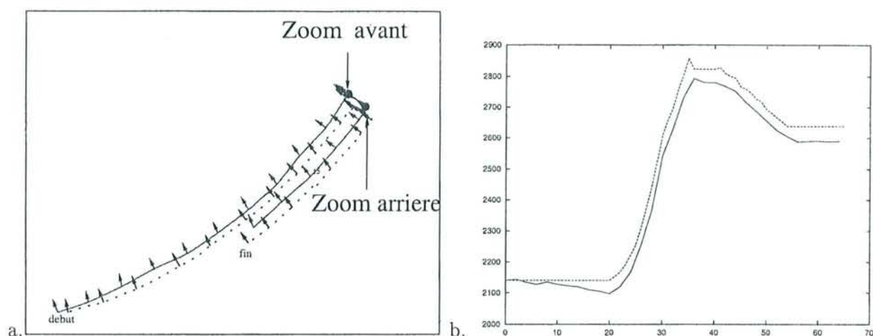
FIG. 7.13 – Paramètres de la caméra attendus (traits continus) et calculés (traits discontinus) pour l'optimisation alternée sur la séquence de la cabane. a. Projection de la trajectoire de la caméra dans le plan horizontal. b. Paramètre \alpha_u .
