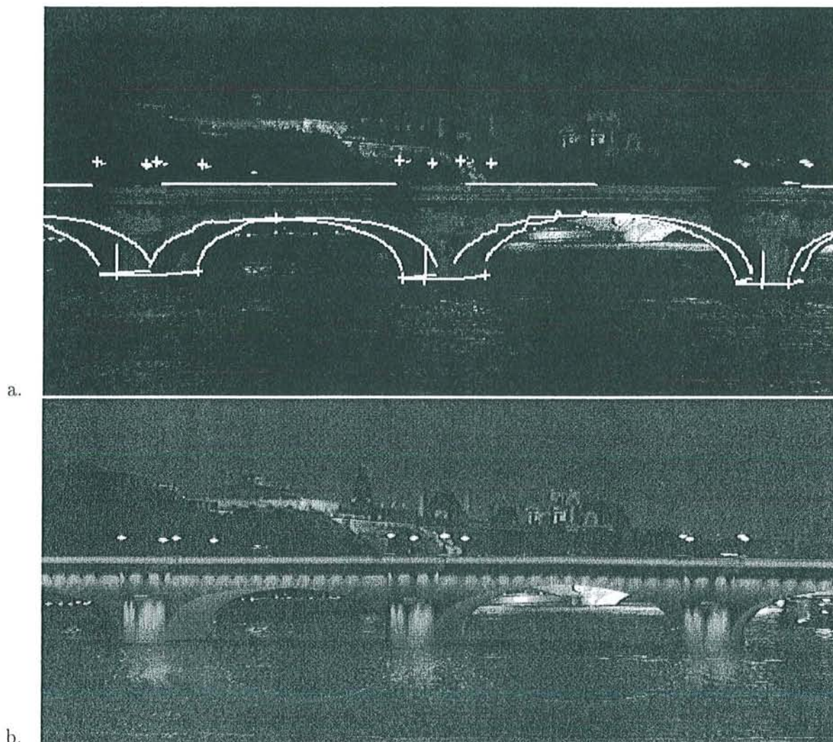
FIG. 4.8 – Résultats pour la 60 ème image de la séquence. a. Projection du modèle filaire et des points utilisés pour le calcul du point de vue. b. Résultat de la composition.
