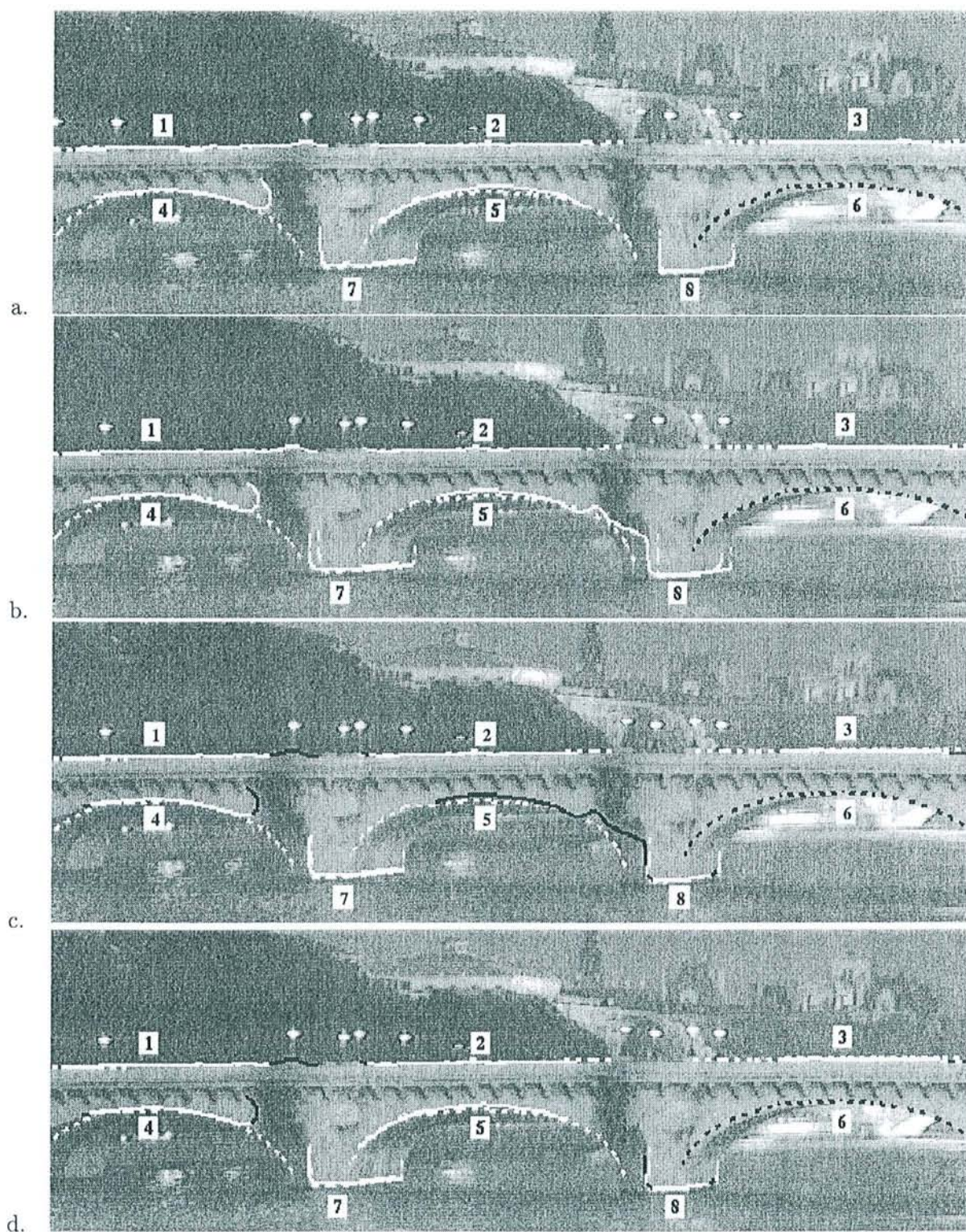
FIG. 5.12 – Itération dans l'image 13. a. Appariements obtenus dans l'image 12. b. Suivi des courbes dans l'image 13 (les projections des primitives 3-D sont celles de l'image 12). c. Recalage du modèle. d. Mise à jour des primitives.
