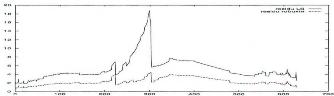
FIG. 7.26 – Résidus aux moindres carrés et résidus robustes sur la séquence du loria.
