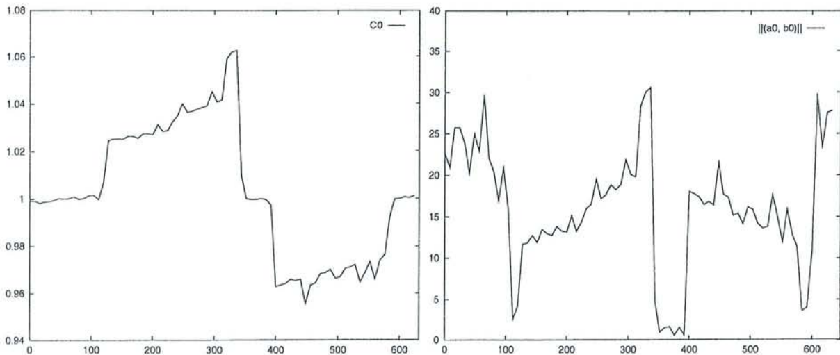
FIG. 7.23 – Évolution de C_0 et de la norme du vecteur (a_0 \ b_0)^T sur la séquence du loria.
