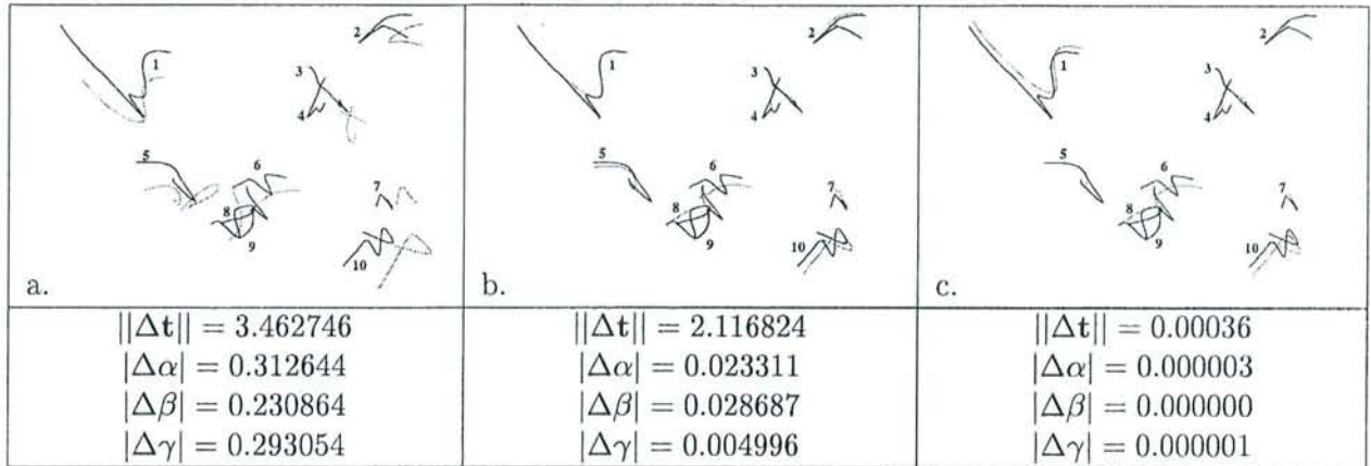
FIG. 5.9 – Exemple de recalage. a. position initiale (les primitives 1, 6 et 10 sont aberrantes). b. Résultat obtenu après l'optimisation à un seul niveau. c. Résultat obtenu après l'optimisation à deux niveaux.
