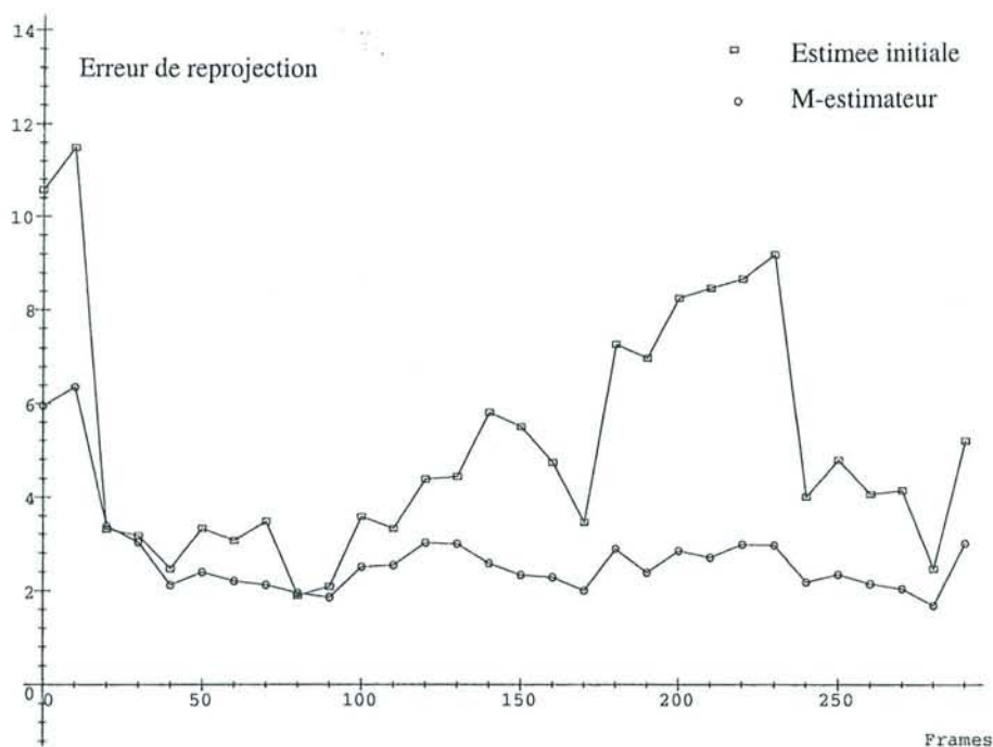
FIG. 4.7 – Erreur de reprojection en pixels après la première estimation (carrés) et après raffinement par l'estimation robuste (cercles).
