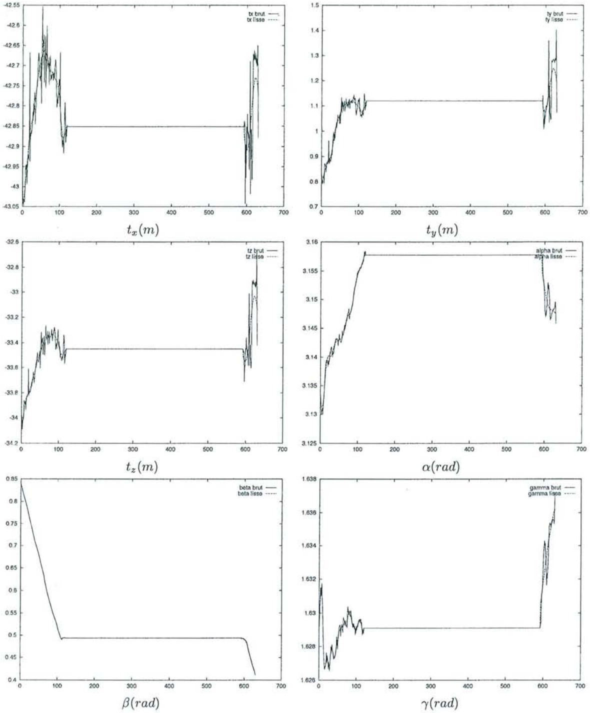
FIG. 7.28 – Paramètres du point de vue obtenus sur la séquence du loria.
