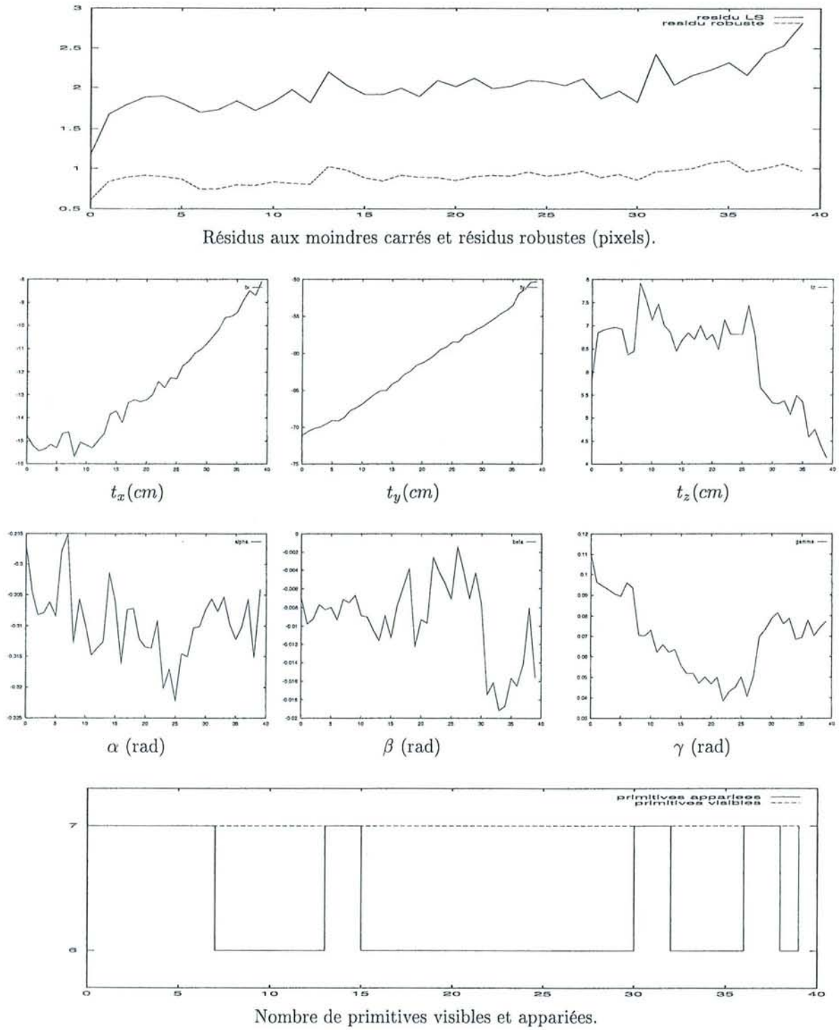
FIG. 5.21 – Résultats statistiques obtenus sur la séquence du chateau.
