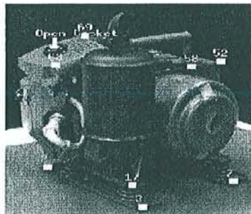
FIG. 3.4 – Recalage temporel par la méthode de Ravela et al. Les fenêtres suivies par corrélation sont indiquées par des rectangles blanc.
