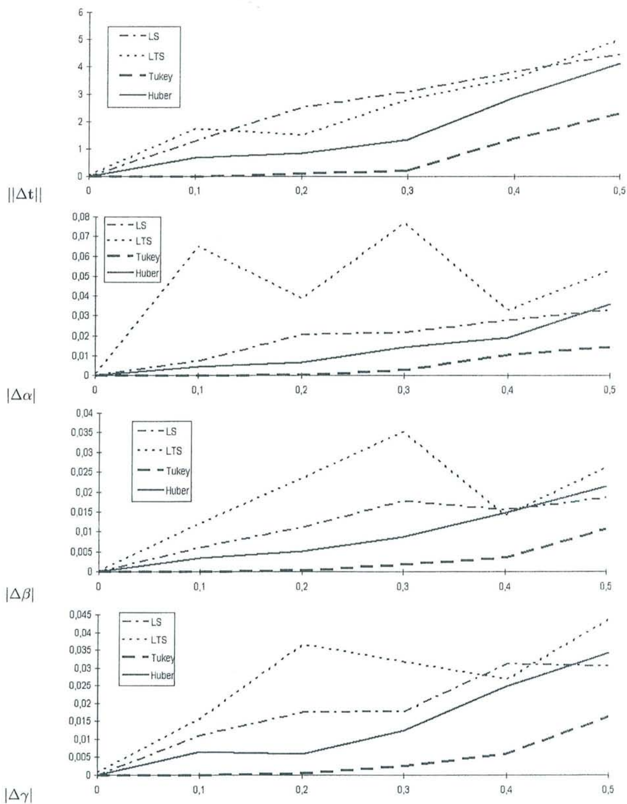
FIG. 5.5 – Influence des erreurs aberrantes sur le calcul du point de vue, en fonction du taux d'erreurs présentes dans les données et pour différents estimateurs utilisés au niveau global ( n = 10 ).
