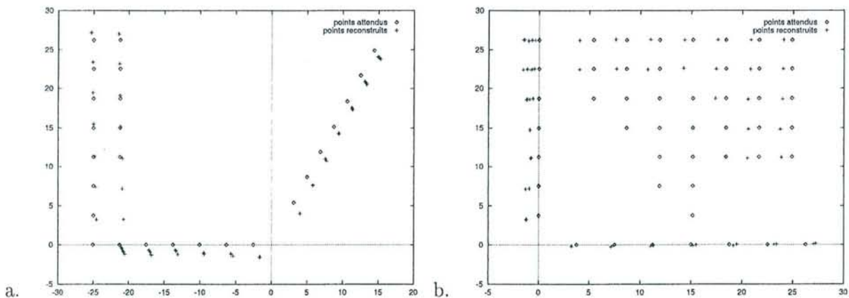
FIG. 7.4 – Projection des points reconstruits dans le plan (xy) (a) et (yz) (b). Les croix sont les points reconstruits et les losanges les points attendus.
