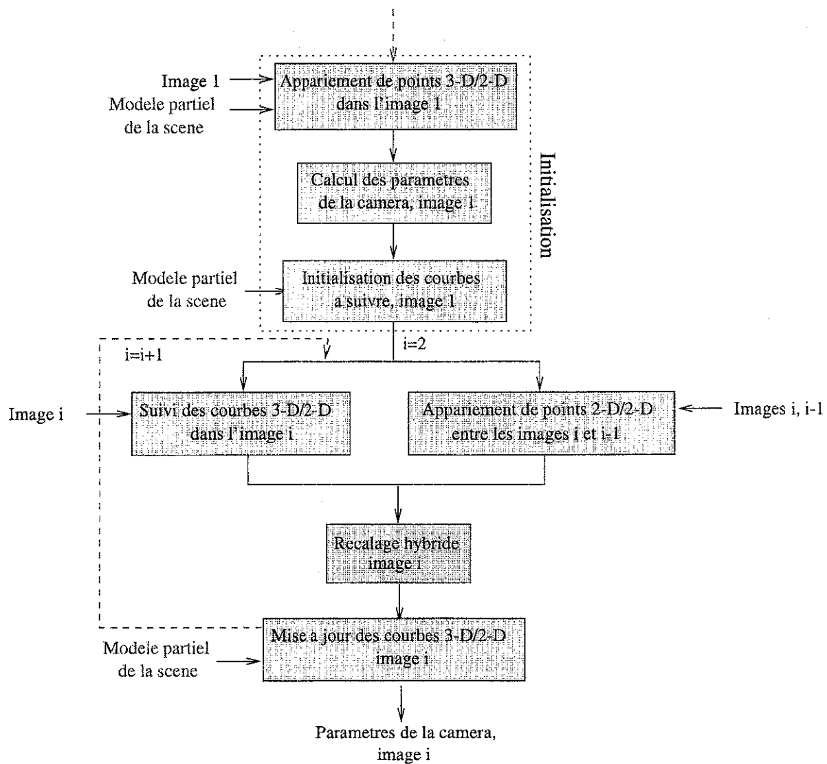
FIG. 6.2 – Boucle de recalage temporel pour la méthode hybride.
