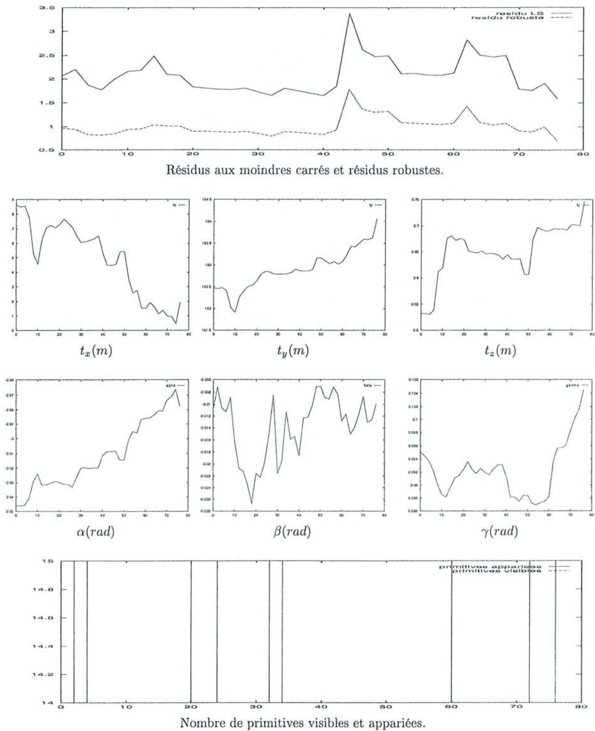
FIG. 6.5 – Résultats statistiques obtenus sur la séquence de la place Stanislas.
