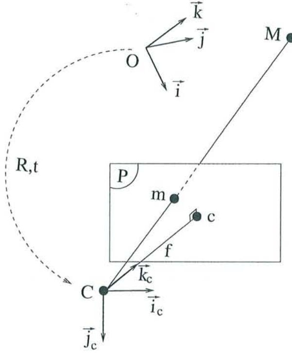
FIG. 2.1 – Le modèle sténopé de caméra.
