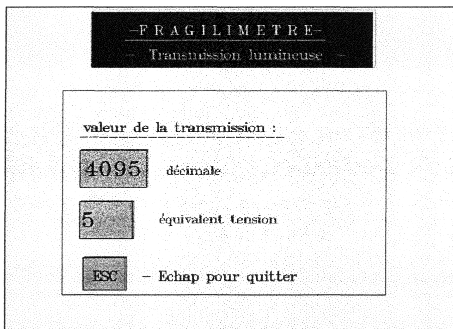
Figure 67 : fenêtre graphique proposée pour visualiser les valeurs en continu du paramètre intensité de transmission lumineuse captée.
