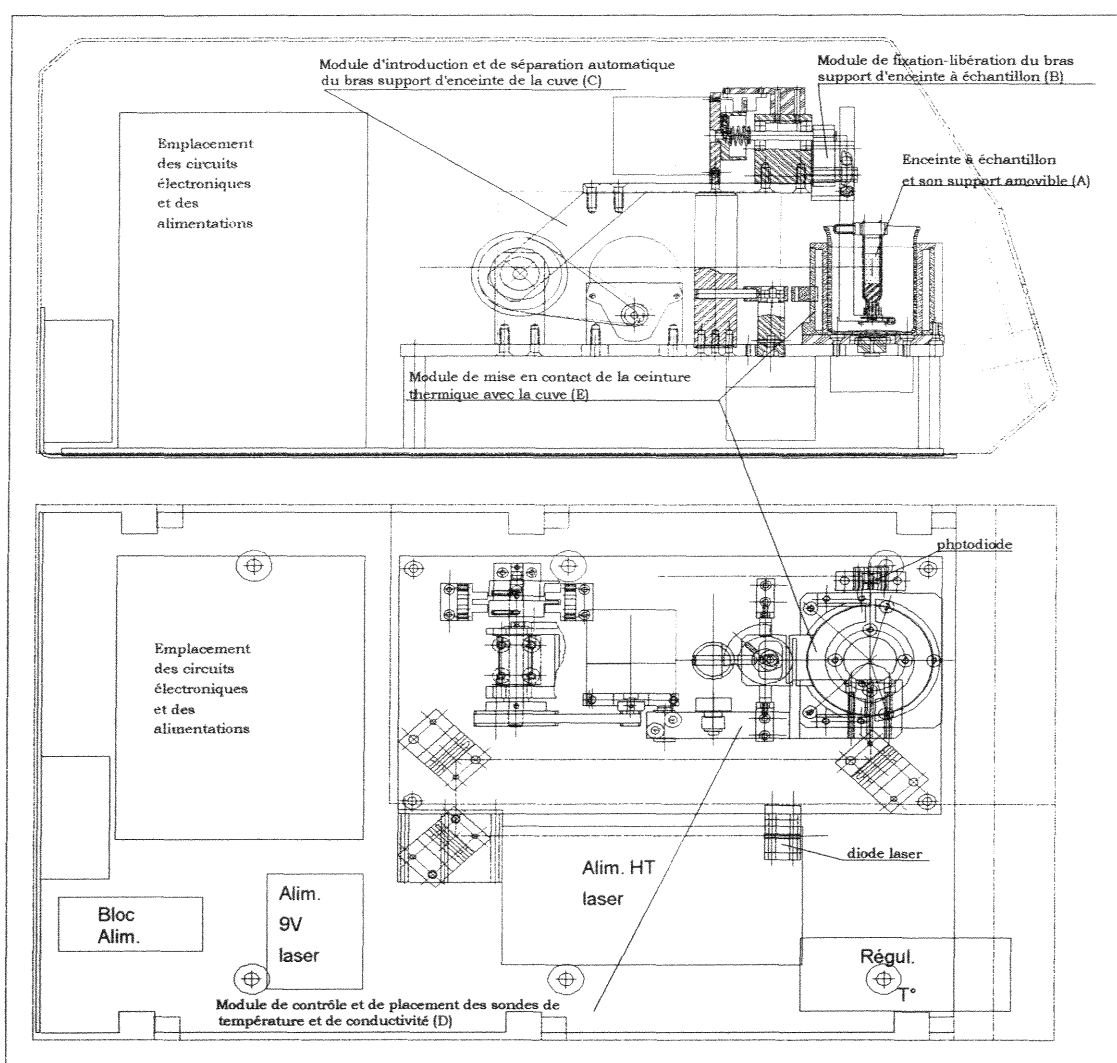
Figure 63 : schémas mécaniques correspondant aux vues d'ensemble du Fragilimètre prototype (vue de dessus : partie inférieure de la figure, vue de côté : partie supérieure de la figure).
