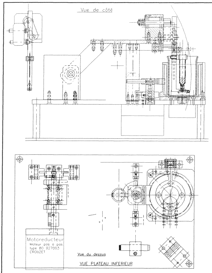
Figure 64 : exemple de vue d'ensemble pour le montage du Fragilimètre version industrielle.
