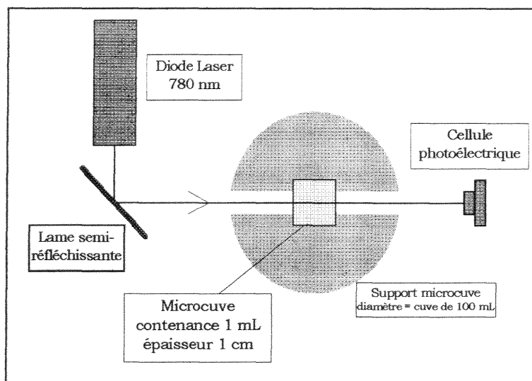
Figure 39 : dispositif de mesure pour analyser le test RCH
