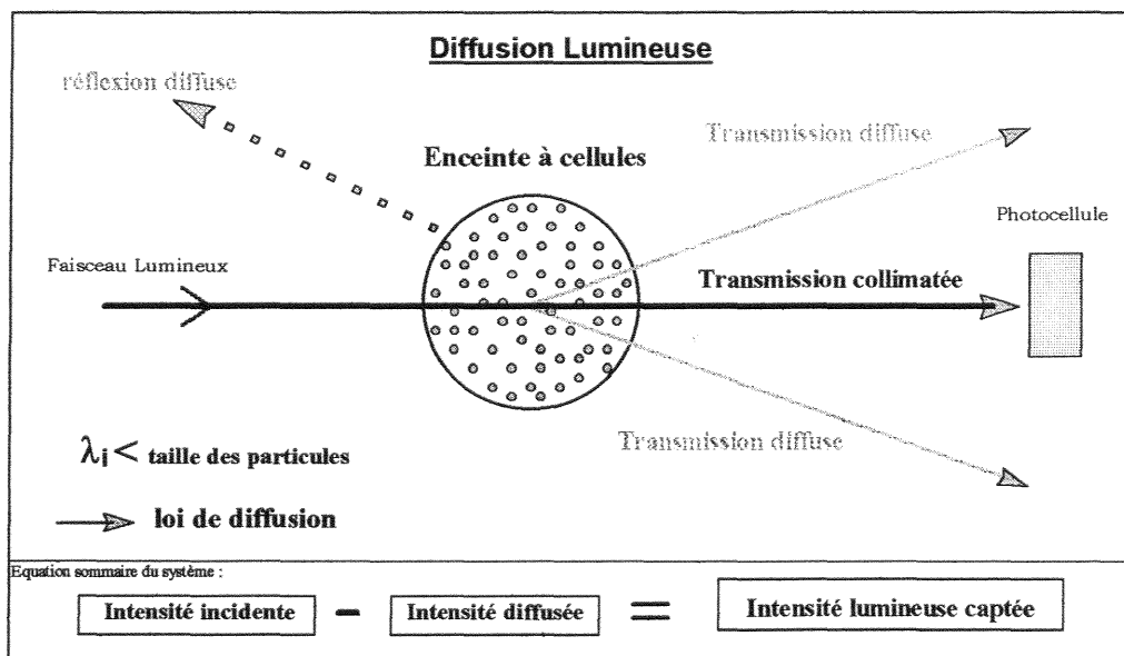
Figure 17 : représentation des trois transmissions caractéristiques de la diffusion pour un faisceau lumineux illuminant une suspension de particules de taille > \lambda_i .
