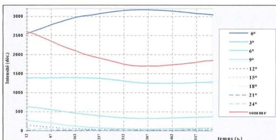
Figure 30 : courbes d'intensité de diffusion autour de la cuve en fonction du temps et pour un même PRP.
