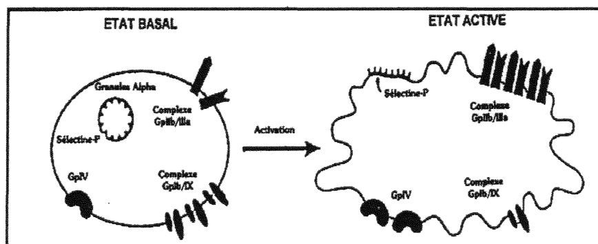
Figure 10 : représentation des principales glycoprotéines (Gp) sur les plaquettes au repos et après activation, d'après Nurden P. (21)
