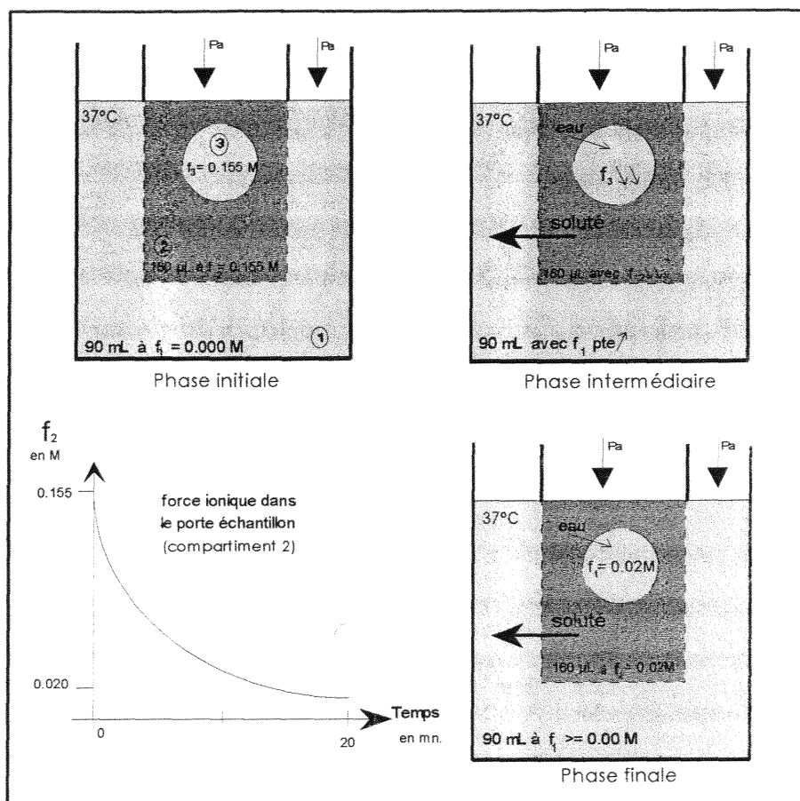
Figure 15 : représentation schématique des différentes étapes correspondant aux variations de pression osmotique engendrées dans le dispositif de mesure du Fragilimètre.
