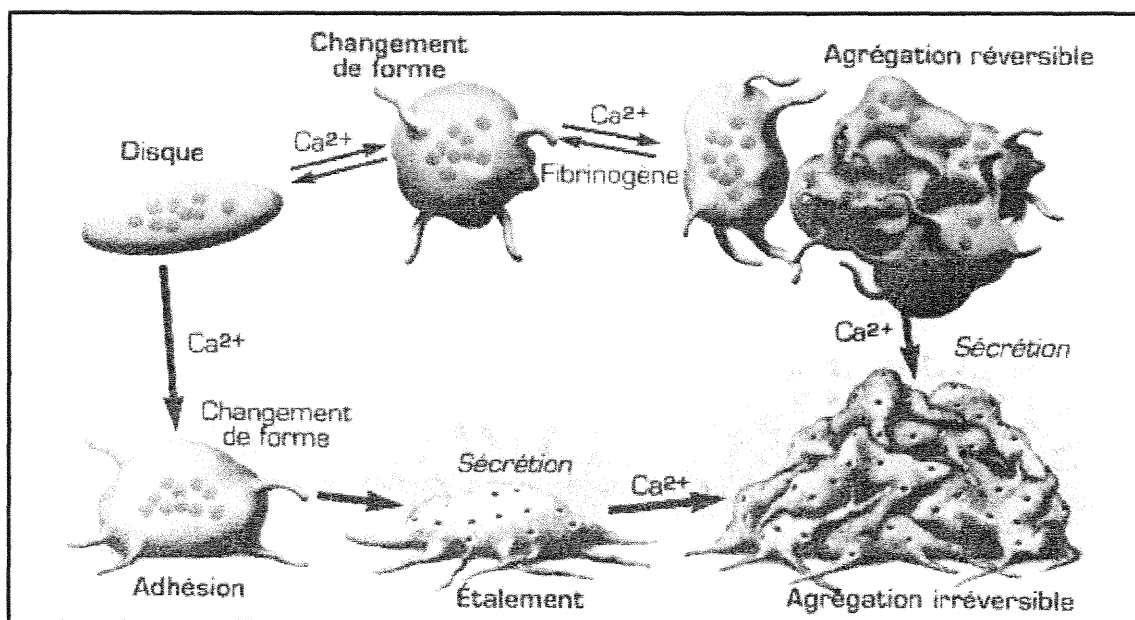
Figure 5 : réactions de base de l'activation plaquettaire, d'après Boneu B. (1)
