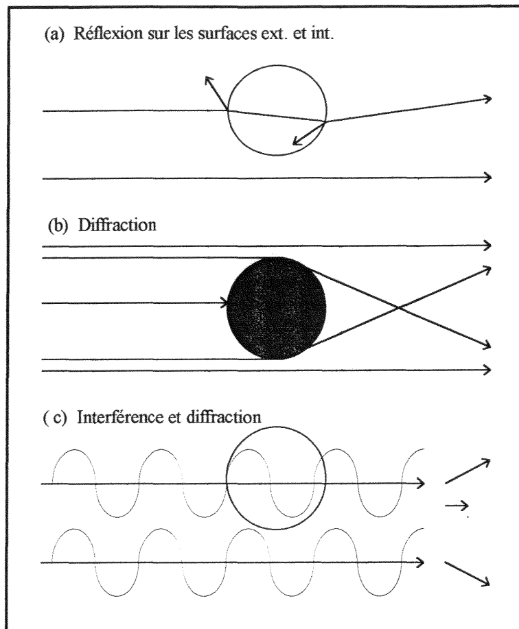
Figure 16 : mécanismes de diffusion sur une particule dont la taille est supérieure à \lambda , et dont la valeur de l'indice de réfraction est proche de celle du centre.
