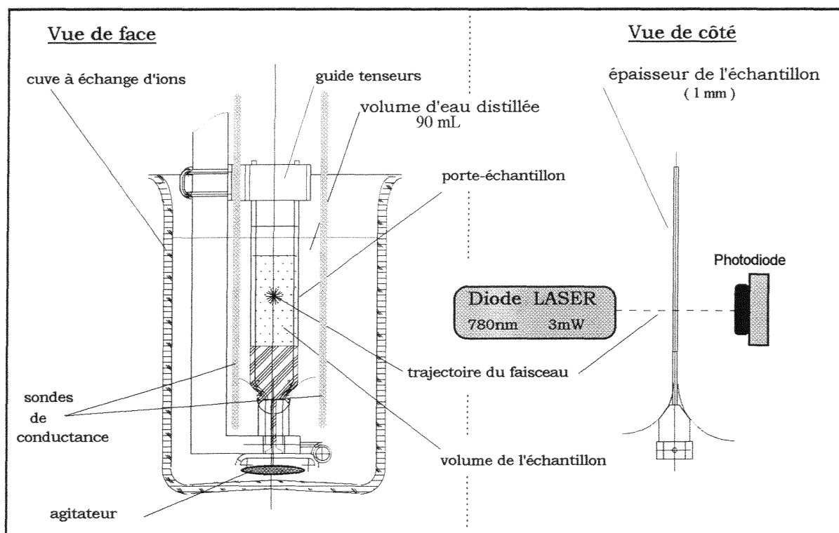
Figure 21 : représentation du dispositif de mesure du Fragilimètre.
