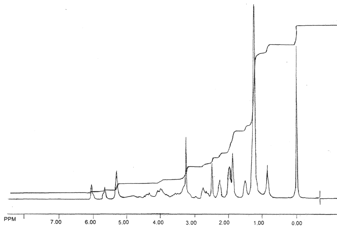
Figure 82 : spectre RMN en 1 H du mélange dérivé 1,5 (C18-OH)PG10 et GMA (1 éq.) après 15 minutes de chauffage à 90°C en présence de DMAP (dans CDCl 3 ).
