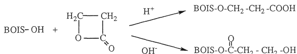
Figure 12 : réaction entre le bois et la \beta propiolactone.
