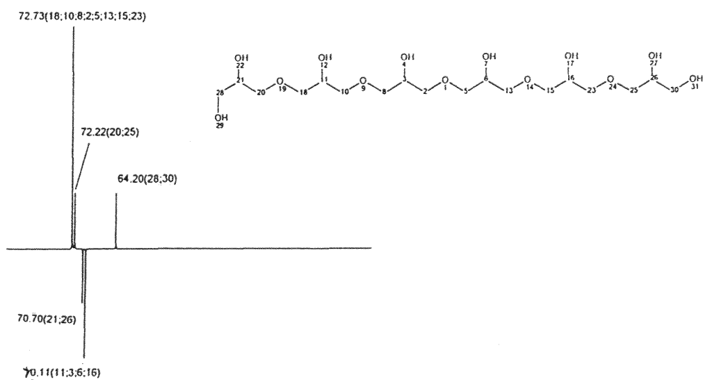
Figure 77 : données RMN 13 C simulés dans DMSO D6 de GMA, glycidol et PG6.
