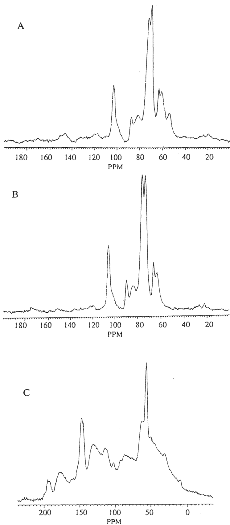
Figure 35 : spectres RMN ^{13}\text{C} de la sciure non modifiée et de ses fractions holocellulose et lignine.
