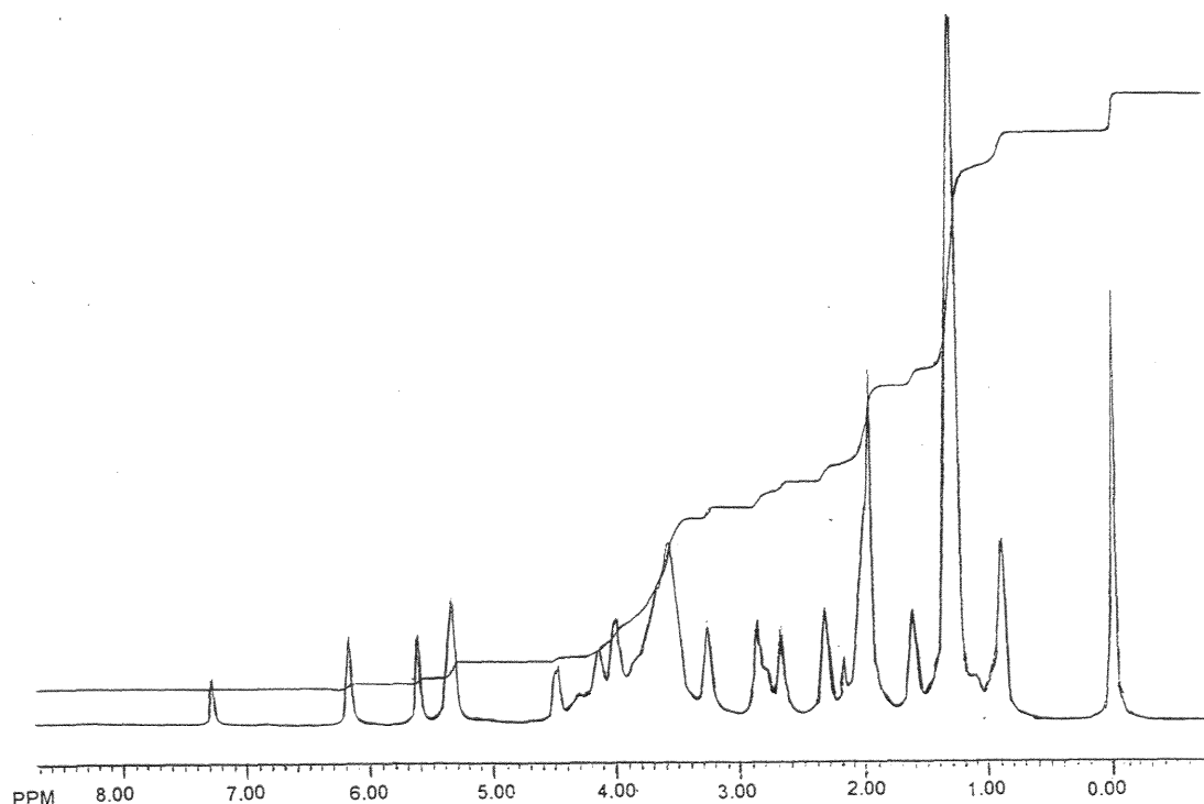
Figure 80 : spectre RMN en ^1\text{H} du mélange dérivé 1 (C6-C18)PG2 / GMA (1 éq.) après 15 minutes de chauffage à 90°C en présence de DMAP (dans \text{CDCl}_3 ).
