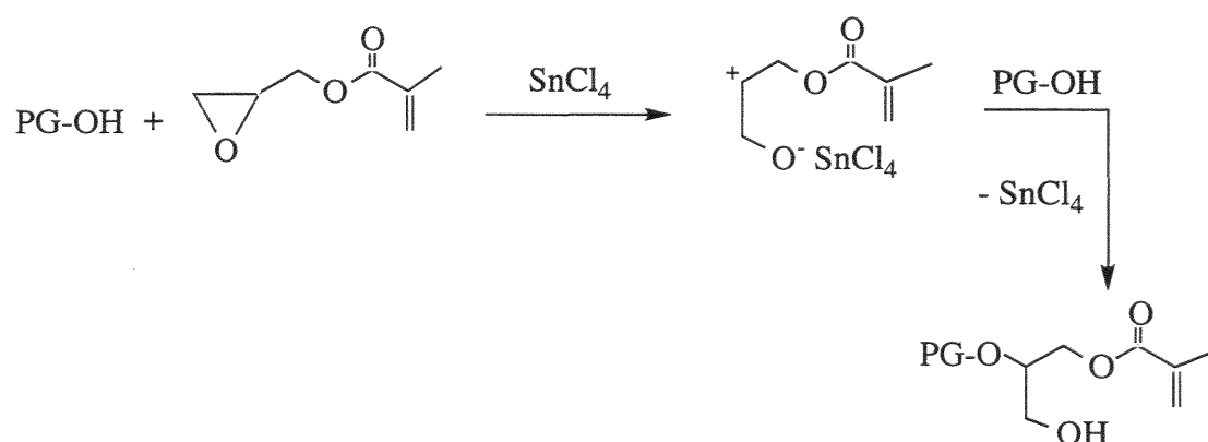
Figure 74 : ouverture du cycle époxyde du GMA par le PG en présence de \text{SnCl}_4 .
