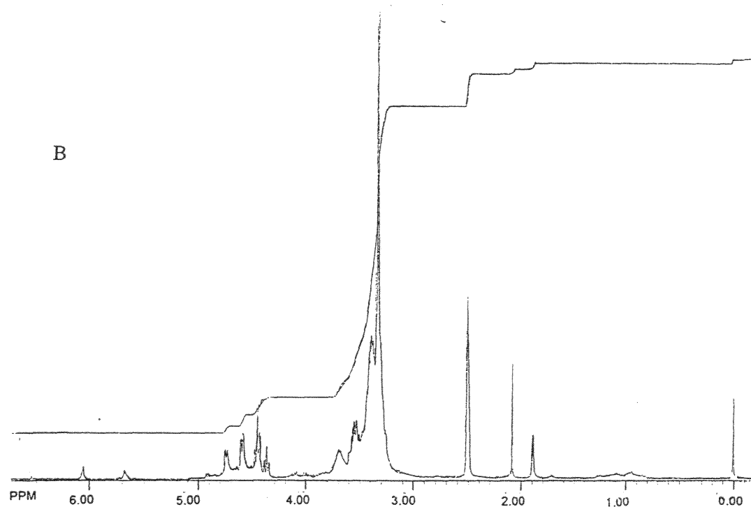
Figure 73 : spectres RMN ^1\text{H} du mélange PG6 / GMA après 15 minutes (A) et 1 heure (B) de chauffage à 90^\circ\text{C} en présence de \text{SnCl}_4 (dans DMSO D6).
