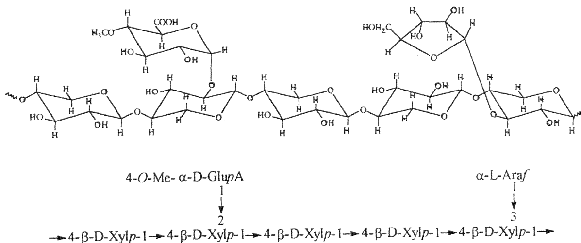
Figure 5: structure partielle d'un arabino-4-o-méthylglucuronoxylane chez les conifères.
