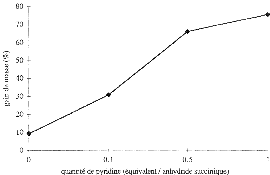
Figure 16 : influence de la quantité de pyridine sur le gain de masse de la sciure estérifiée.
