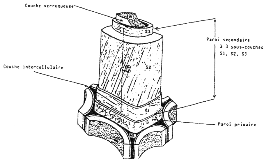
Figure 3: représentation schématique des différentes couches constituant la paroi cellulaire (Core, 1979).
