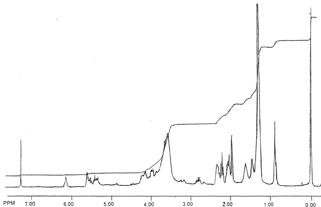
Figure 83 : spectre RMN en ^1\text{H} du mélange monoglycéride de colza et GMA (1 éq.) après 15 minutes de chauffage à 90^\circ\text{C} en présence de DMAP (dans \text{CDCl}_3 ).
