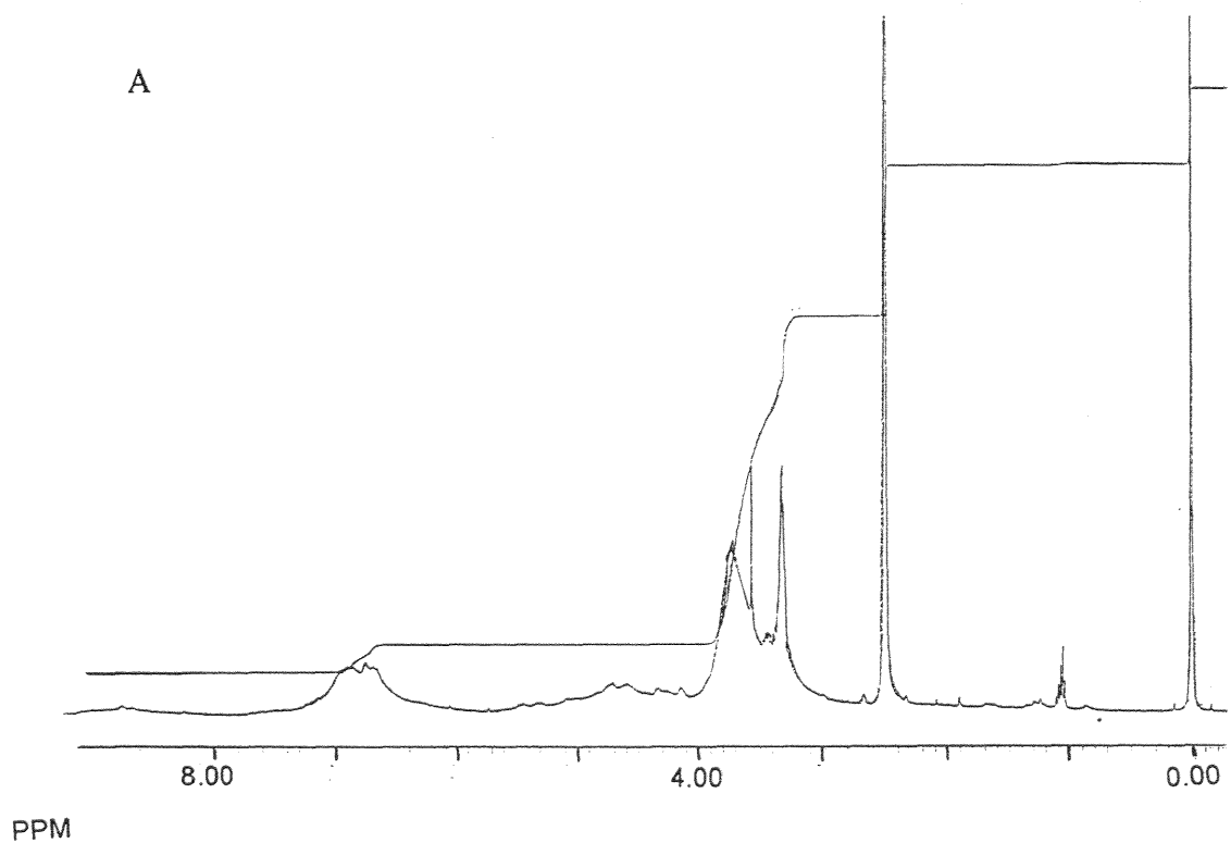
Figure 41 : spectres RMN ^1\text{H} de lignines (dans DMSO D6) A = lignine du bois brut extraite à pH7; B = lignine du bois greffé extraite à pH4.
