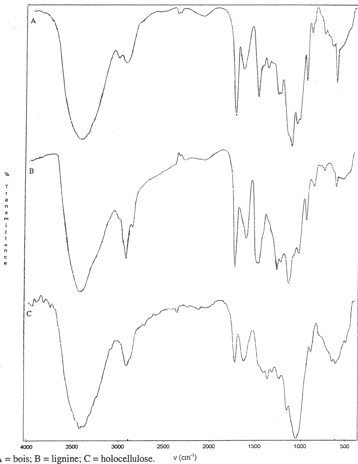
Figure 44 : spectres IR du bois greffé avec le chlorure de 2-(méthacryloyloxyéthyl)triméthylammonium et de ses fractions holocellulose et lignine
