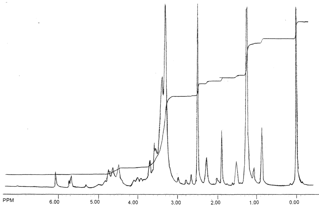
Figure 81 : spectre RMN en 1 H du mélange dérivé 1,5 (C6-C18)PG10 / GMA (1 éq.) après 15 minutes de chauffage à 90°C en présence de DMAP (dans CDCl 3 ).
