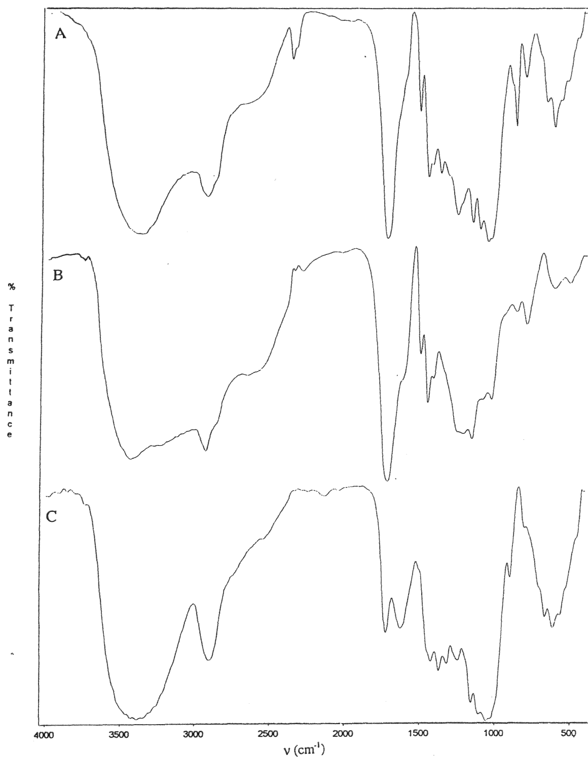
Figure 34 : spectres IR du bois modifié avec l'acide acrylique et de ses fractions holocellulose et lignine.
