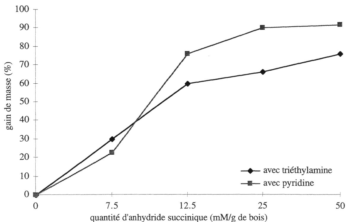
Figure 15 : influence de la quantité d'anhydride succinique sur le gain de masse de la sciure estérifiée.
