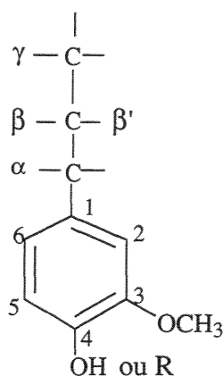
Figure 38 : unité guaïacyle de la lignine d'épicéa.
