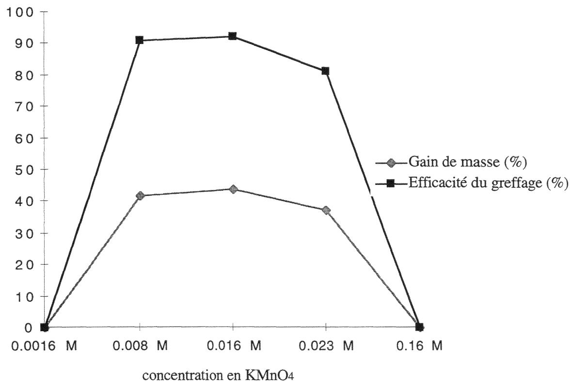
Figure 20 : influence de la concentration en \text{KMnO}_4 de la solution de prétraitement sur le greffage de l'acide acrylique avec la sciure.
