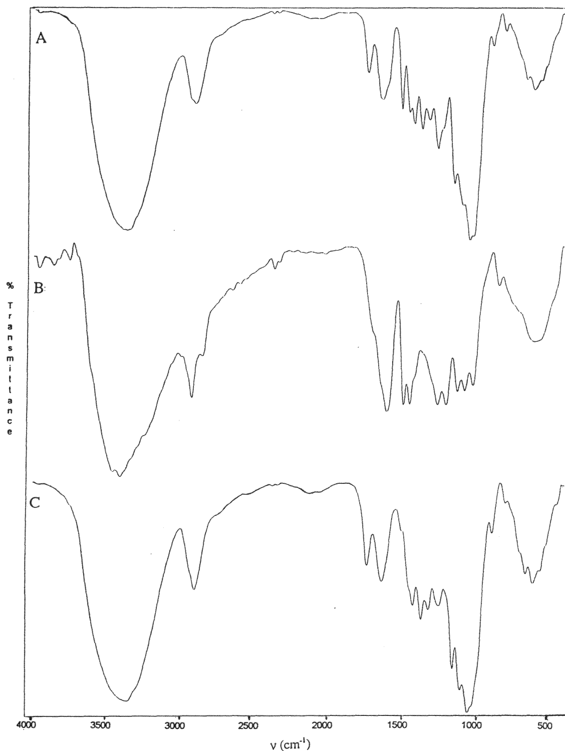
Figure 32 : spectres IR du bois non modifié et de ses fractions holocellulose et lignine.
