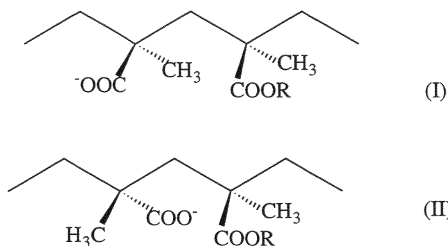
Figure 19 : représentation structurale de deux chaînes de polyméthacrylate de méthyle.
