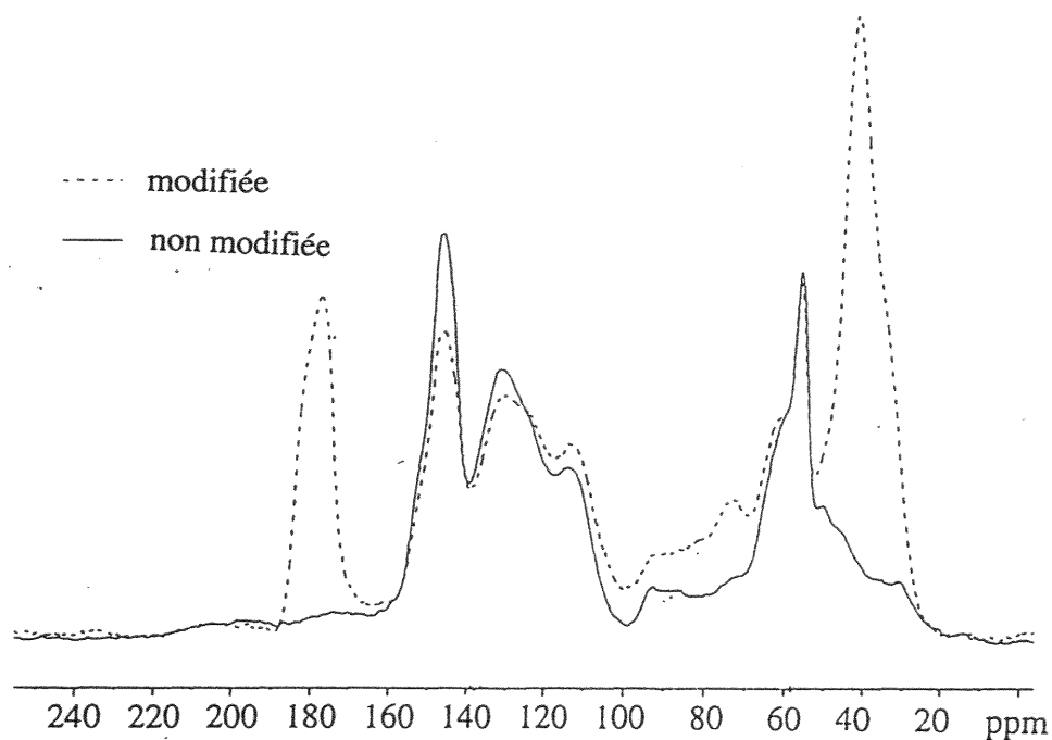
Figure 39 : spectres RMN ^{13}\text{C} avec suppression des bandes de rotation de la lignine dans la sciure non modifiée et modifiée (gain de masse de 11 %).
