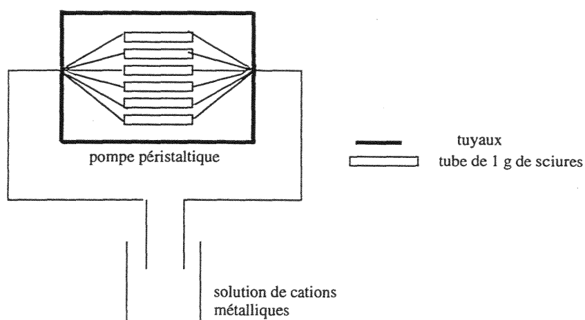
Figure 51 : montage expérimentale.
