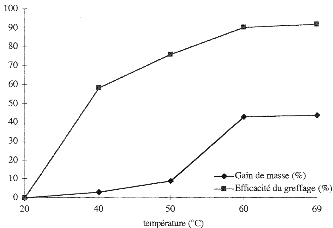
Figure 21: influence de la température sur le greffage de l'acide acrylique avec la sciure. (0,5 g de sciure prétraitée avec \text{KMnO}_4 0,016 M puis modifiée avec 0,5 ml d'acide acrylique dans 16 ml d'hexane pendant 2 heures).
