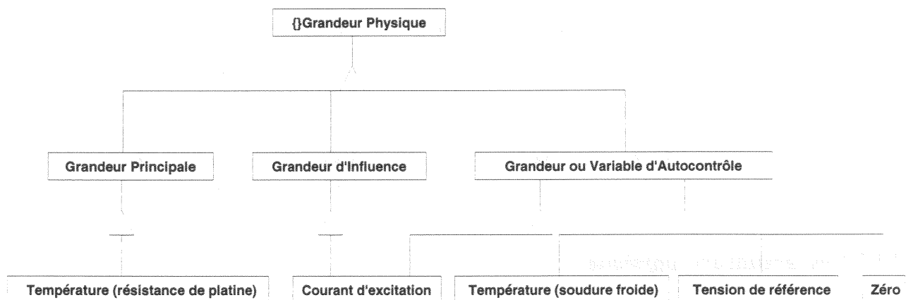
Figure VI.3 : Diagramme d'objets comportant un héritage multiple montrant les différentes grandeurs physiques intervenant pour la mesure de température avec une résistance de platine.
