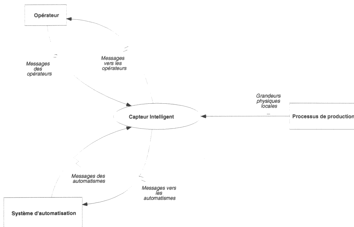
Figure IV.10 : Diagramme de flots de données montrant les interactions du capteur intelligent avec son environnement.
