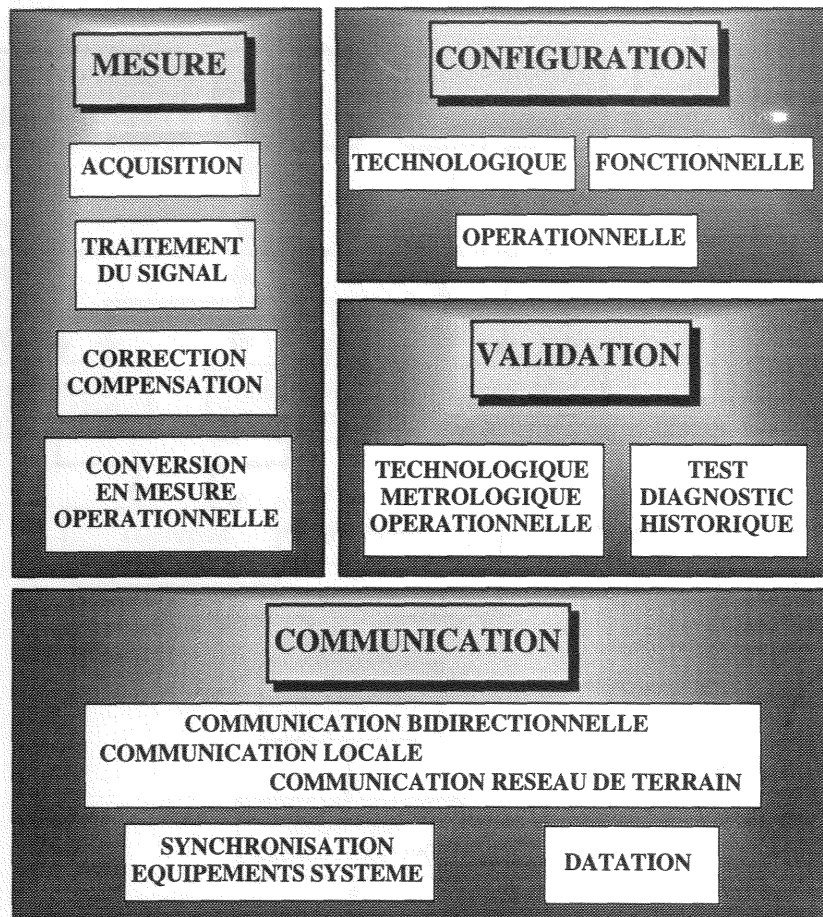
Figure I.11 : Fonctionnalités internes du capteur intelligent.
