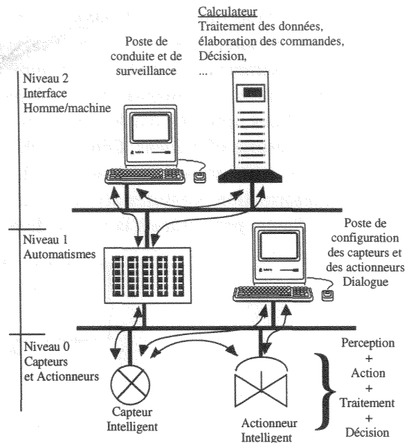
Figure I.10 : L'utilisation d'équipements intelligents permet de décentraliser les traitements.
