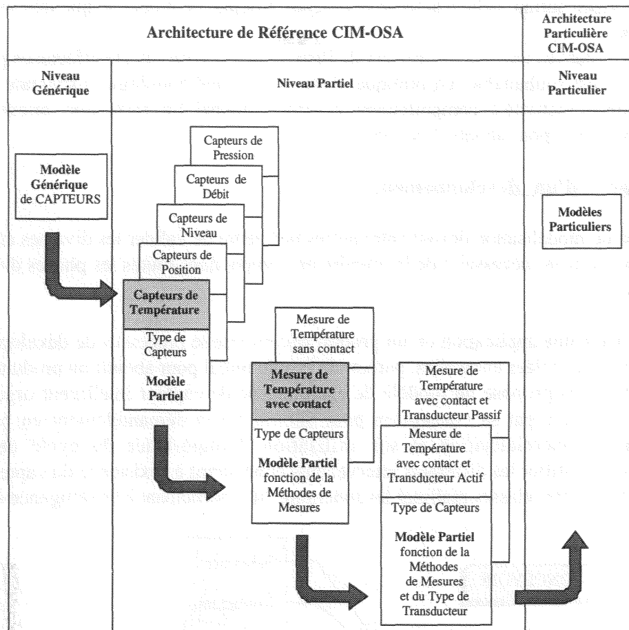
Figure III.2 : Instanciation des constructions génériques de capteurs intelligents en modèles partiels et modèles particuliers [RIVI-94].
