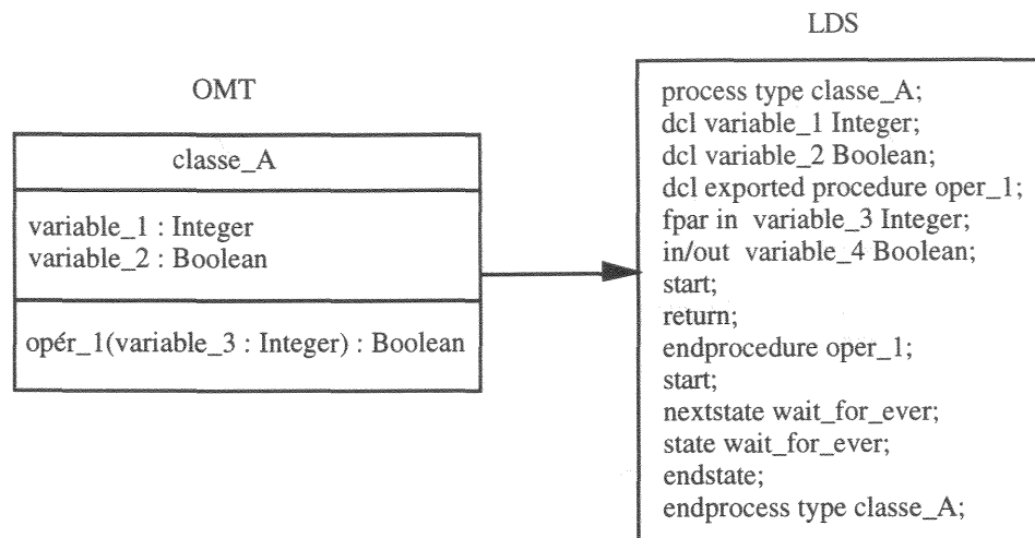
Figure VI.20 : Exemple de passage d'un objet passif en notation OMT vers la notation LDS.
