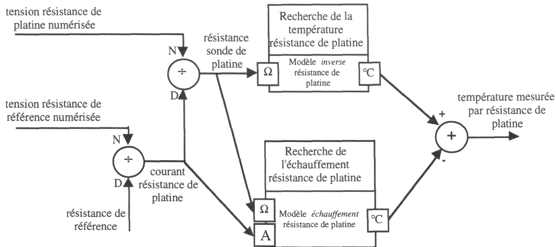
Figure VI.13 : Modèles et grandeurs utilisés pour le calcul d'une température mesurée par une résistance de platine.
