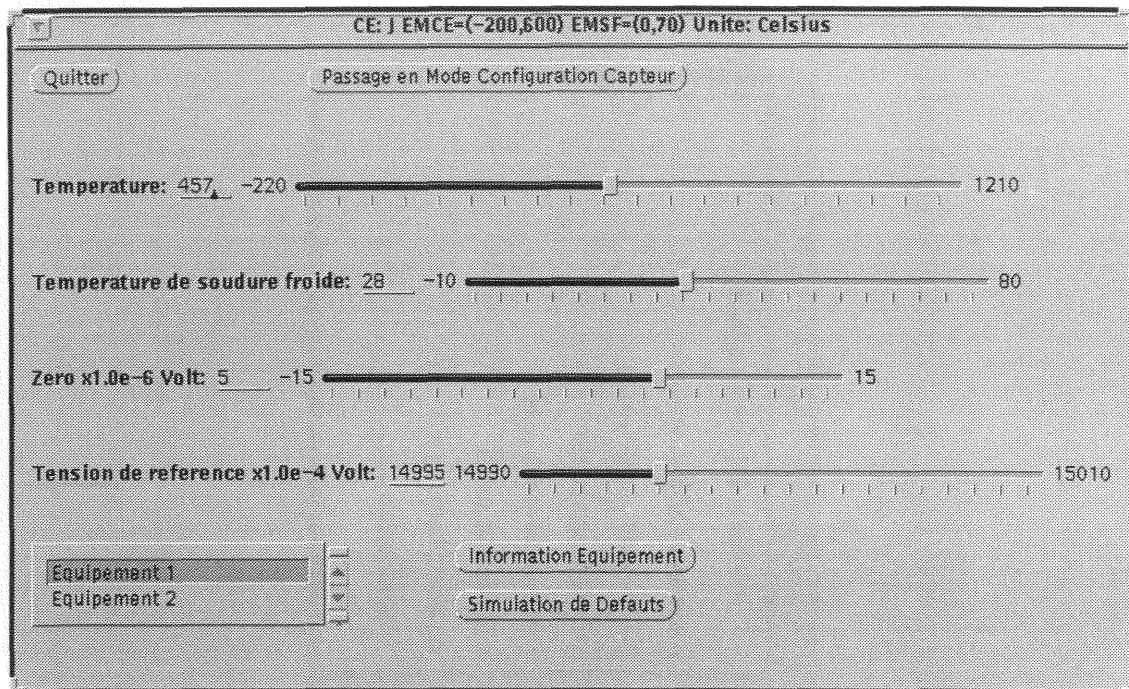
Figure AIV.2 : Tableau de bord de simulation pour les grandeurs physiques.
