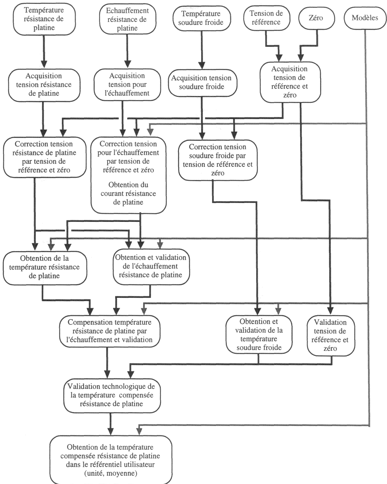
Figure VI.5 : Hiérarchie d'obtention d'une mesure opérationnelle pour une résistance de platine.
