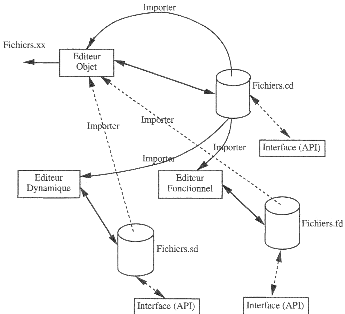
Figure IV.20 : Organisation de l'outil LOV/OMT.
