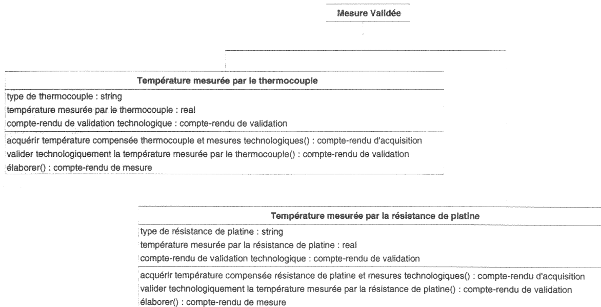
Figure VI.12 : Portion du diagramme d'objet de la hiérarchie de mesure montrant la hiérarchie d'héritage pour la classe "Mesure Validée".
