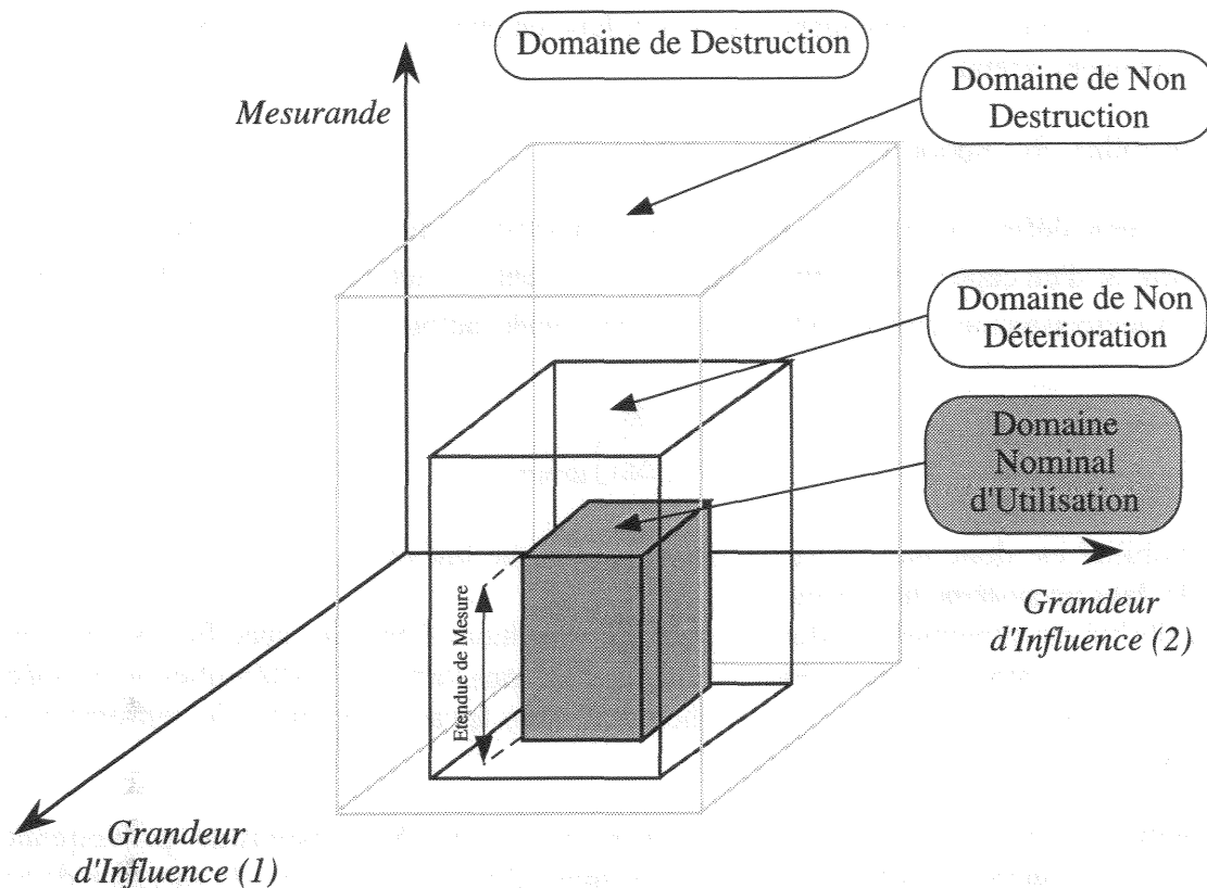
Figure I.5 : Limite d'emploi du capteur.
