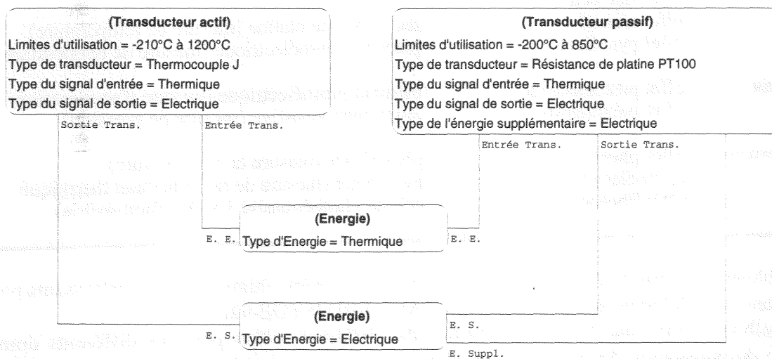
Figure V.10 : Diagramme d'instance d'un thermocouple et d'une résistance de platine
