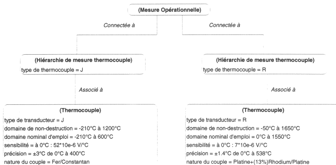
Figure VI.7 : Diagramme d'instances partiel pour une mesure opérationnelle.
