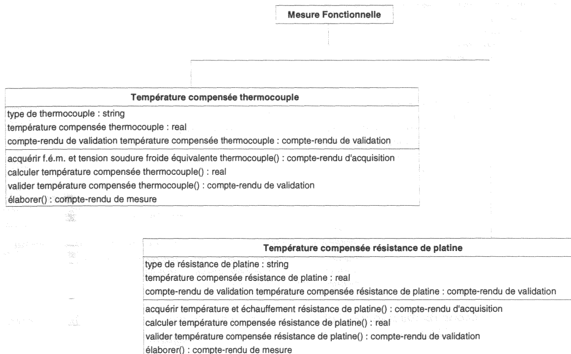
Figure VI.10 : Portion du diagramme d'objet de la hiérarchie de mesure montrant la hiérarchie d'héritage pour la classe "Mesure Fonctionnelle".
