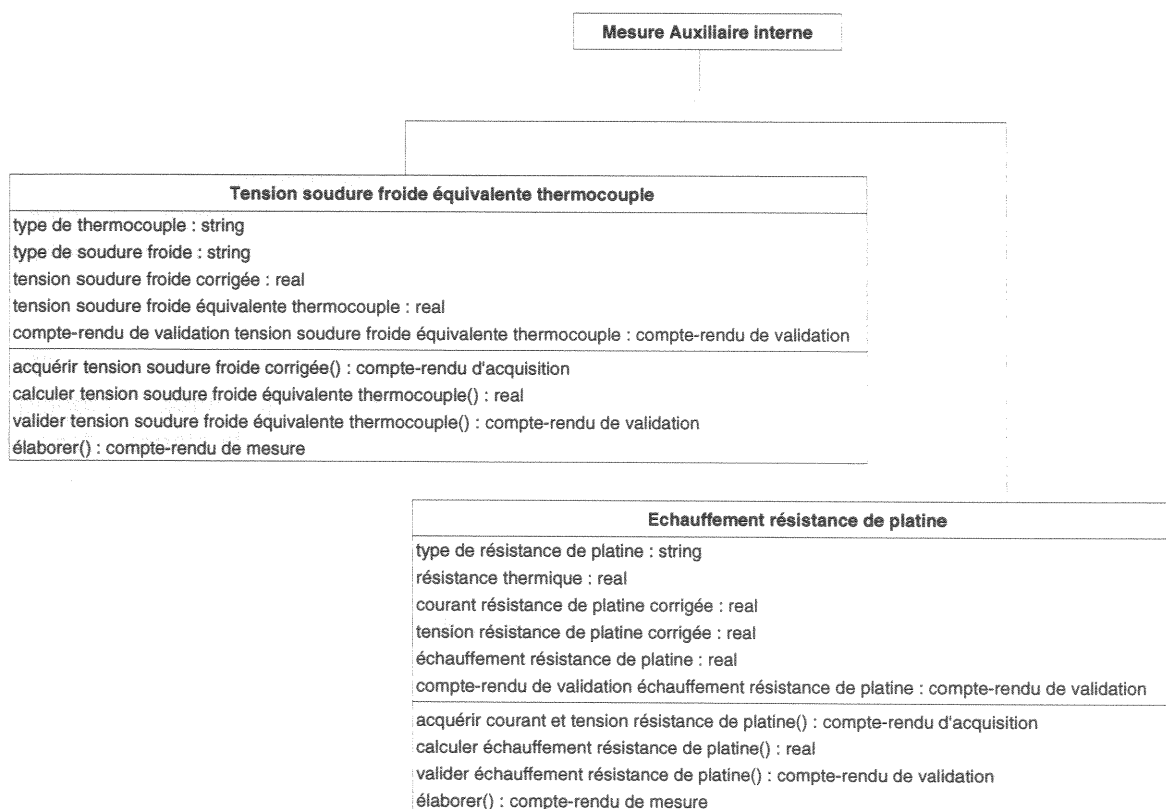
Figure VI.9 : Portion du diagramme d'objet de la hiérarchie de mesure montrant la hiérarchie d'héritage pour la classe "Mesure Auxiliaire Interne".
