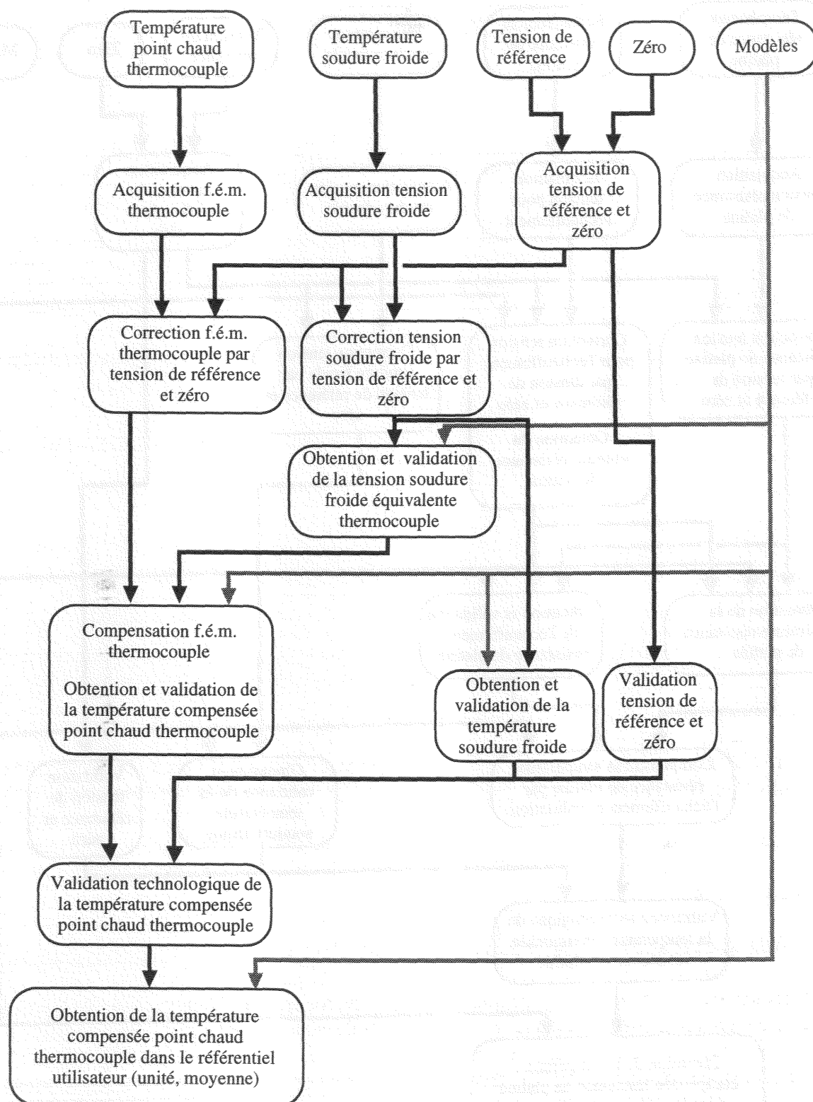
Figure VI.4 : Hiérarchie d'obtention d'une mesure opérationnelle pour un thermocouple.
