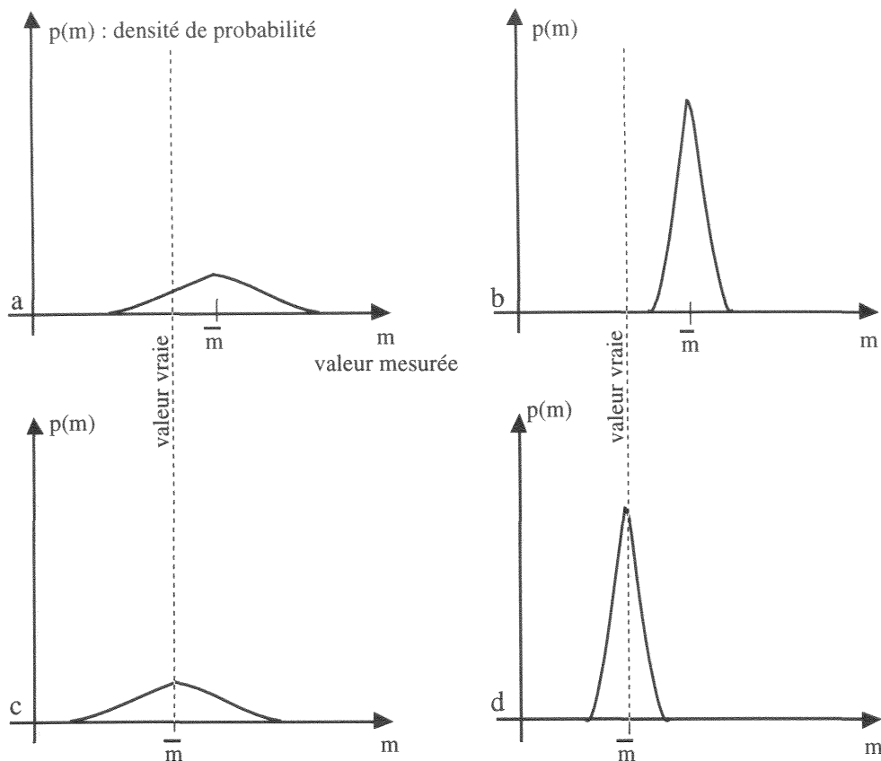
Figure I.4 : Analyse des mesures caractérisant la précision d'un capteur [ASCH-91].
