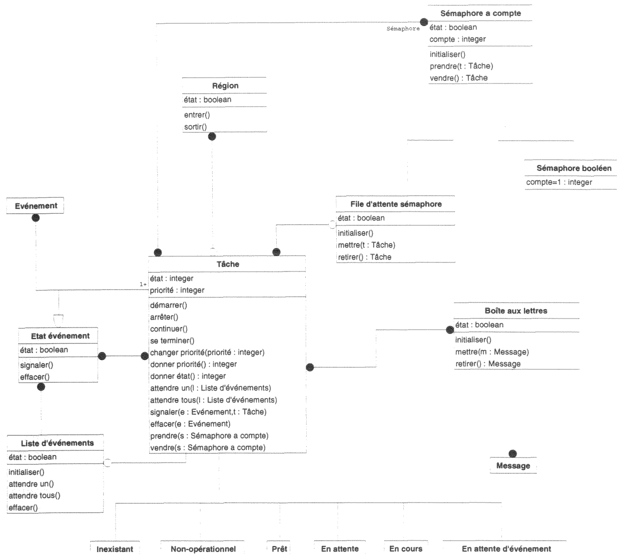
Figure C.1 : Diagramme d'objets montrant les classes dédiées au temps réel [DORS-91] [PERE-90].
