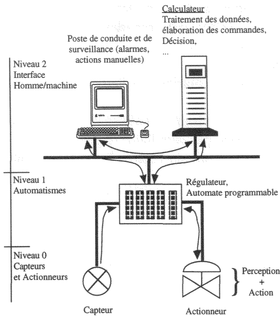
Figure I.9 : Le traitement est centralisé sur un régulateur ou automate programmable avec des capteurs et actionneurs analogiques.
