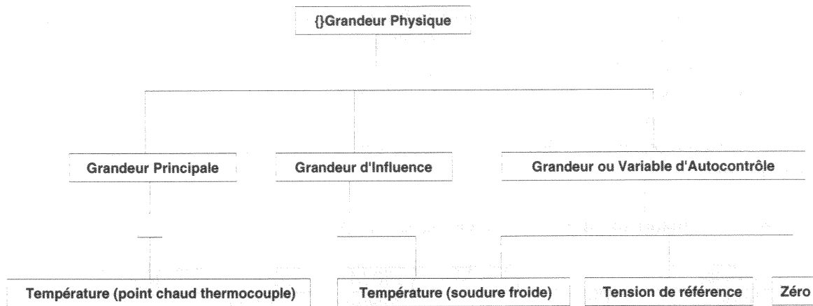
Figure VI.2 : Diagramme d'objets comportant un héritage multiple montrant les différentes grandeurs physiques intervenant pour la mesure de température avec un thermocouple.
