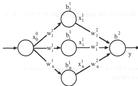
Figure VI.15 : Réseau de neurones à 3 couches.
