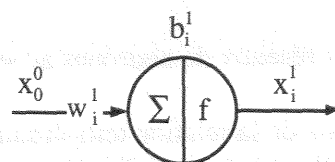
Figure VI.16 : Neurone i de la couche cachée.
