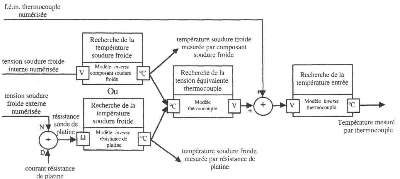
Figure VI.14 : Modèles et grandeurs utilisés pour le calcul d'une température mesurée par un thermocouple.
