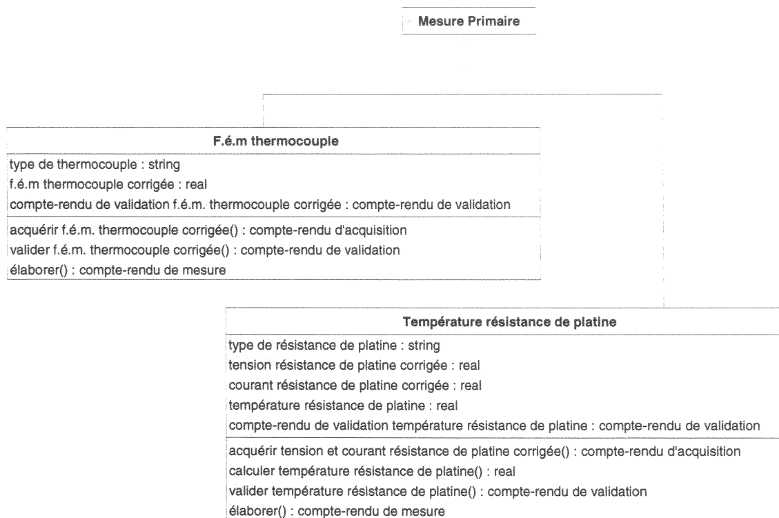
Figure VI.8 : Portion du diagramme d'objet de la hiérarchie de mesure montrant la hiérarchie d'héritage pour la classe "Mesure Primaire".
