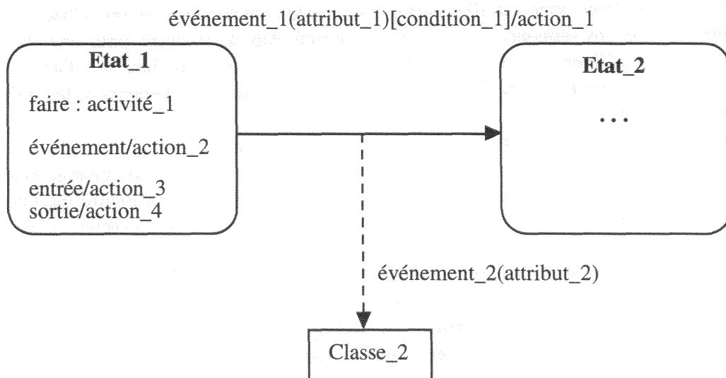
Figure AII.4 : Notation du diagramme d'états.
