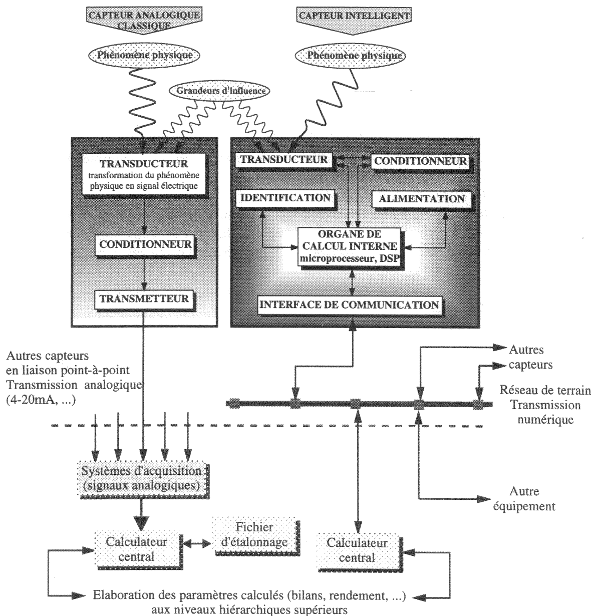
Figure I.6 : Comparaison des deux types de chaînes de mesures (analogique à gauche, numérique "intelligent" à droite)[BEAU-91].
