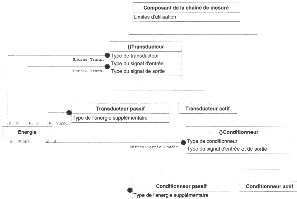
Figure V.7 : Modèle objet pour les composants de la chaîne de mesure en fonction des domaines d'énergie.
