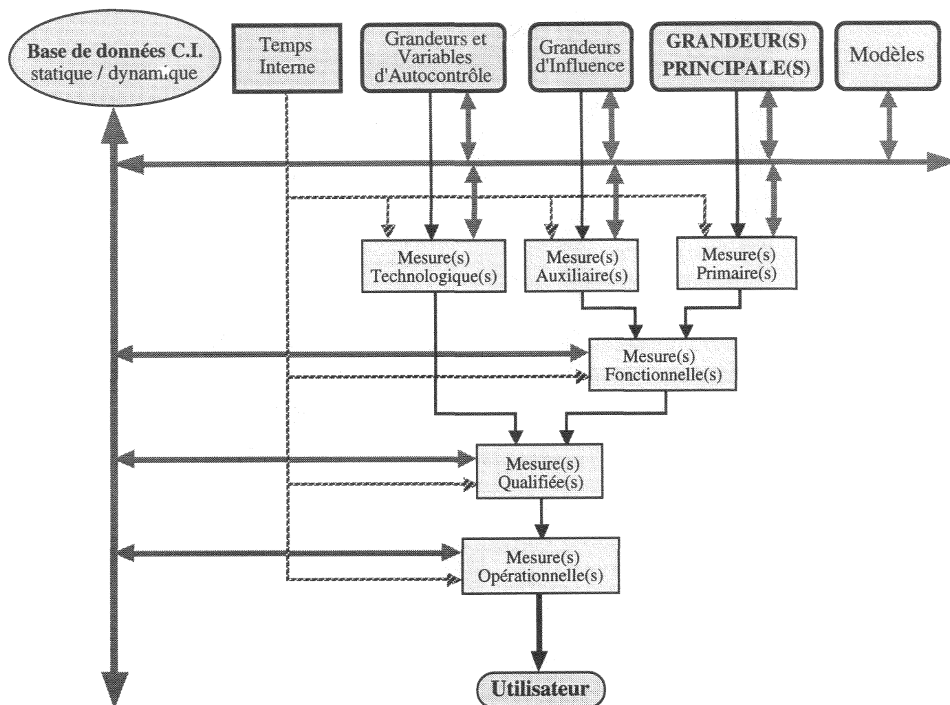
Figure I.12 : Hiérarchie conduisant à la mesure opérationnelle.
