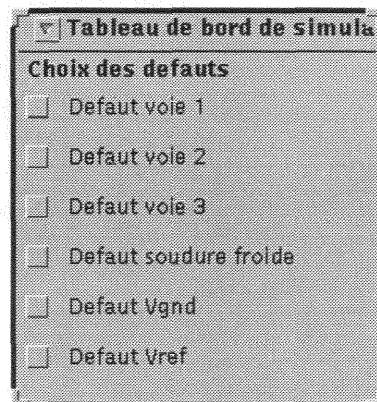
Figure AIV.3 : Tableau de bord de simulation pour les défauts.
