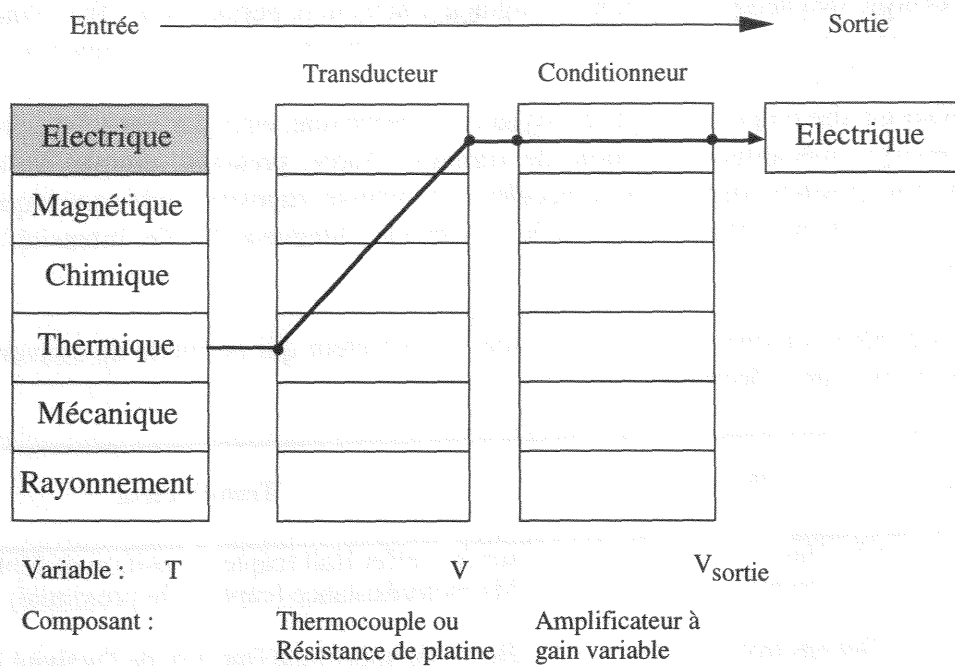
Figure V.9 : Exemple d'une chaîne de mesure d'un capteur de température utilisant un thermocouple ou une résistance de platine.
