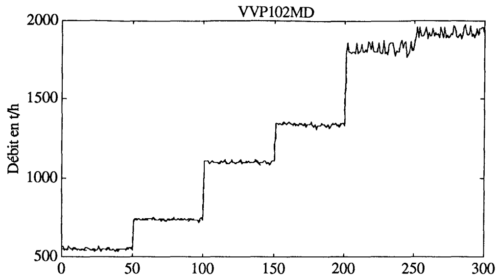
Fig. IV.15 : Mesures débit vapeur.
