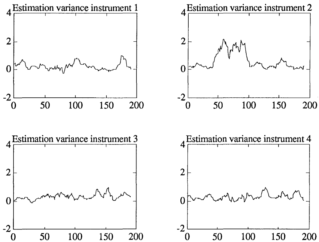
Fig. II.3 : Estimations des variances des erreurs de mesure sur une fenêtre de longueur 10.
