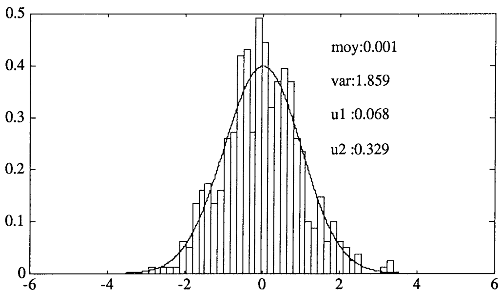
Fig. III.5a : Comparaison à une loi normale du résidu 1.
