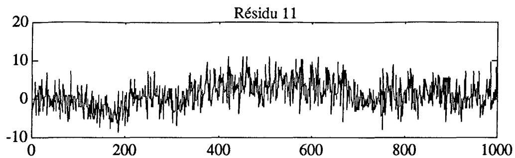
Fig. IV.11 : Résidus des équations de bilan.
