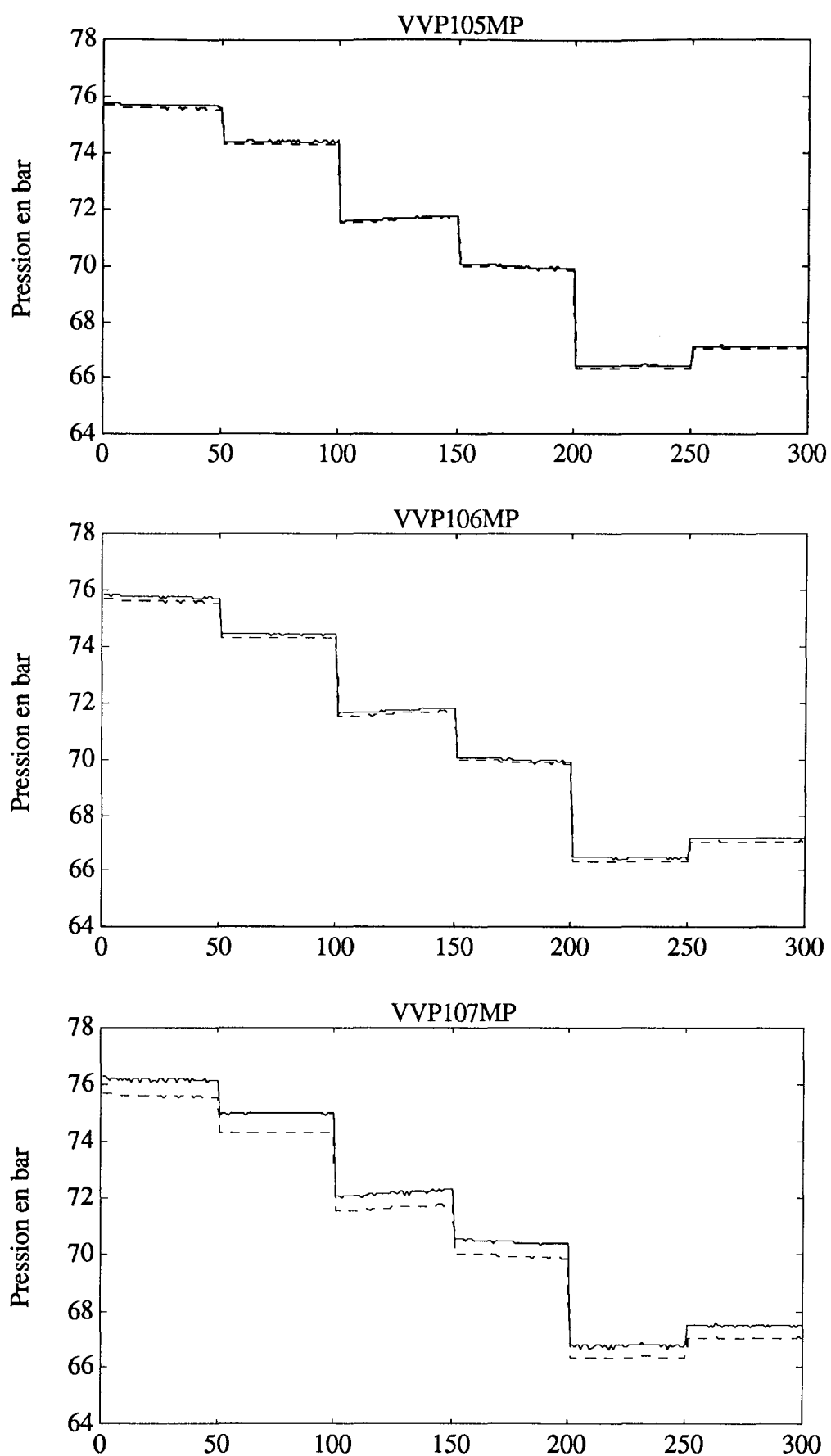
Fig. IV.13 : Mesures pression vapeur.
