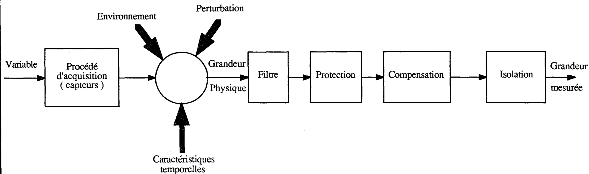
Fig. I.1 : Chaîne d'instrumentation.
