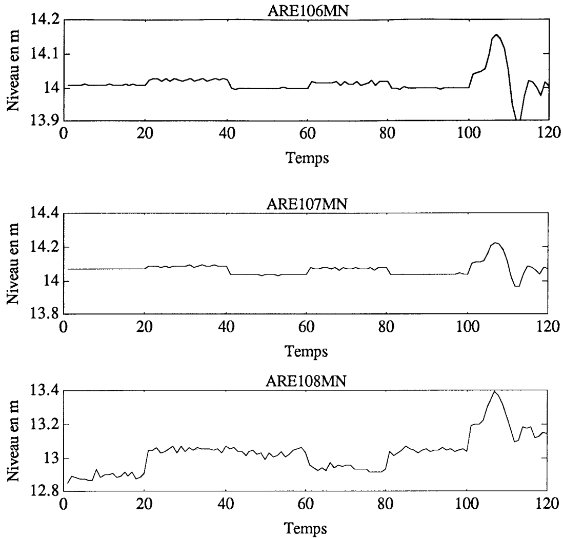
Fig. IV.7 : Mesures niveaux.
