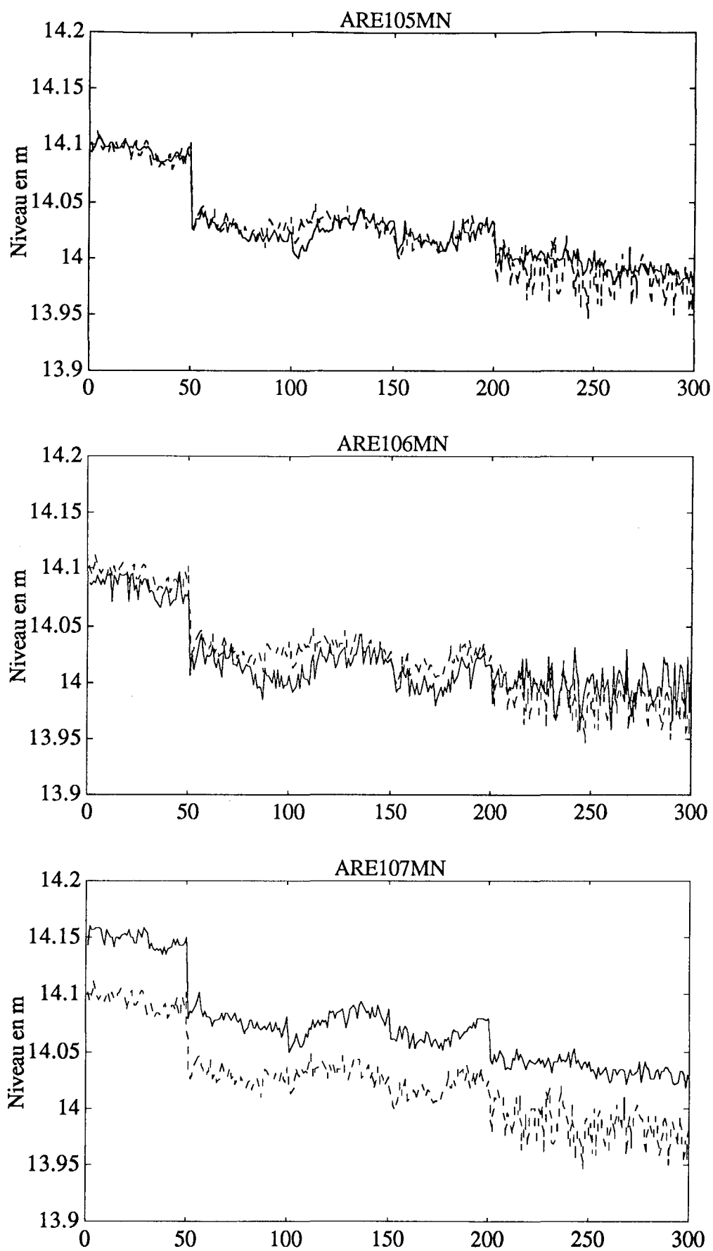
Fig. IV.17 : Mesures niveau gamme étroite.
