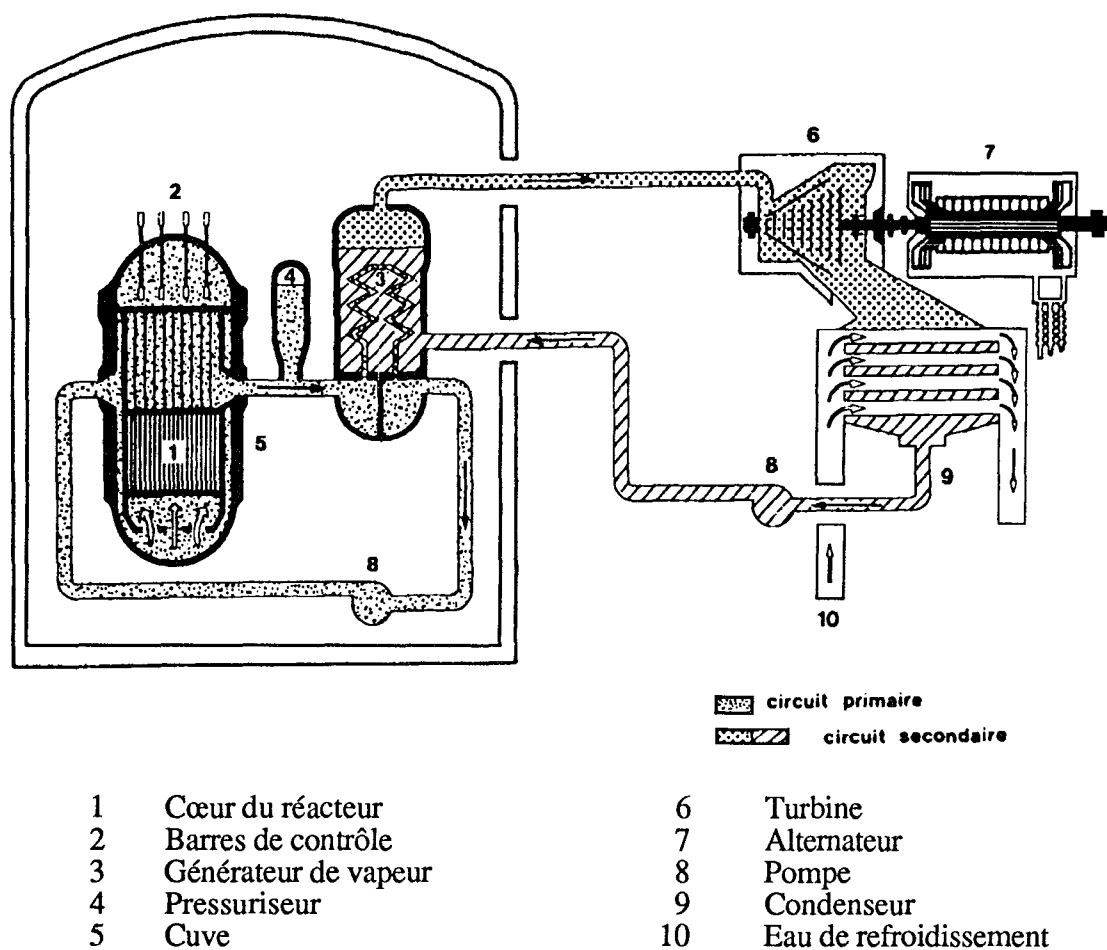
Fig. IV.1 : Schéma de principe du fonctionnement d'une centrale nucléaire à eau sous pression.
