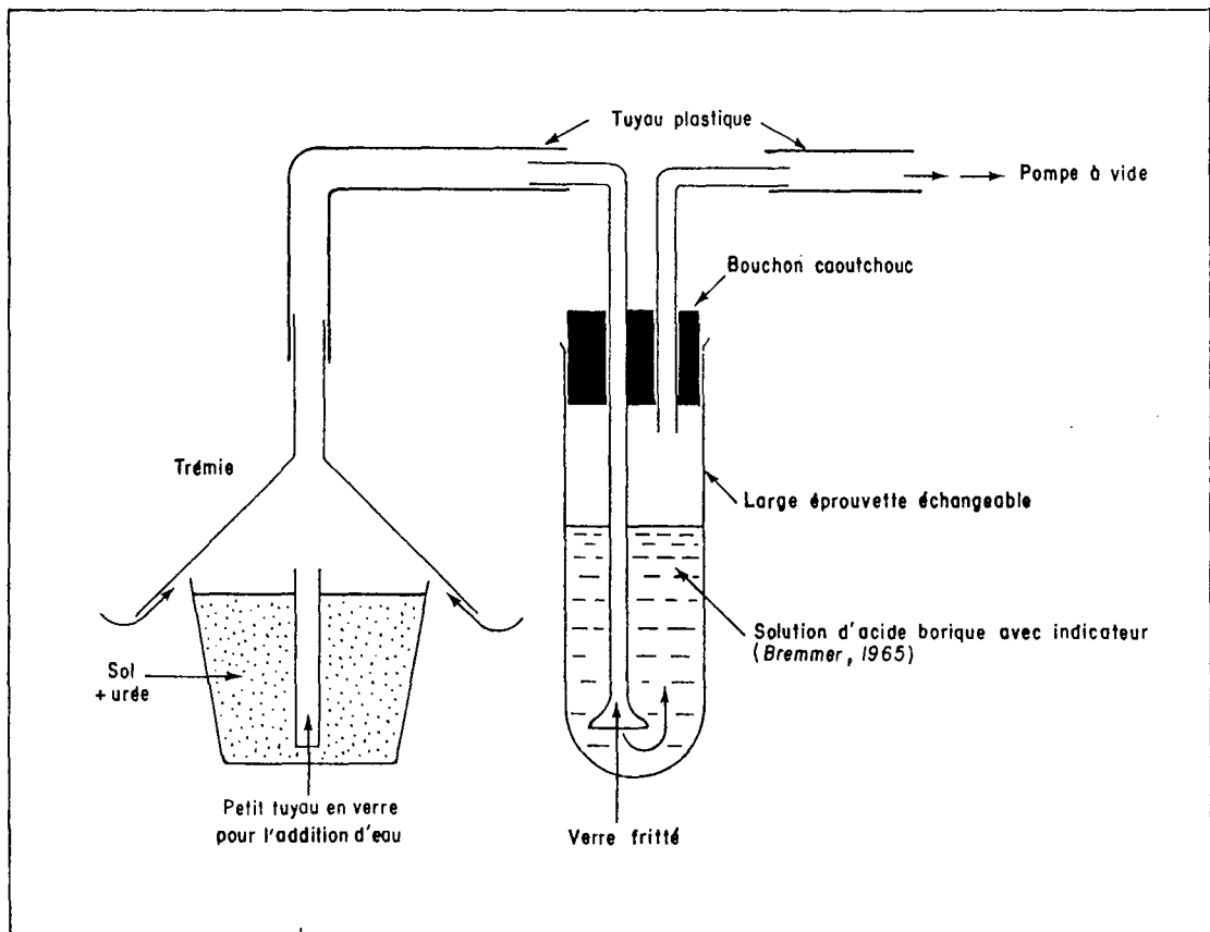
Figure 21 : Schéma du système utilisé en milieu contrôlé pour la détermination des pertes par volatilisation d'ammoniac à partir de l'urée ajoutée.
