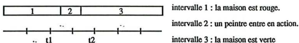
Figure 2.20 : Un univers indécis pour le prédicat : TRUE( t_1, t_2, \text{COLOR}(\text{HOUSE17}, \text{RED}) )
