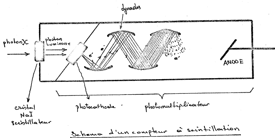
FIG. 14-15 COMPTeur A SCINTILLATION
