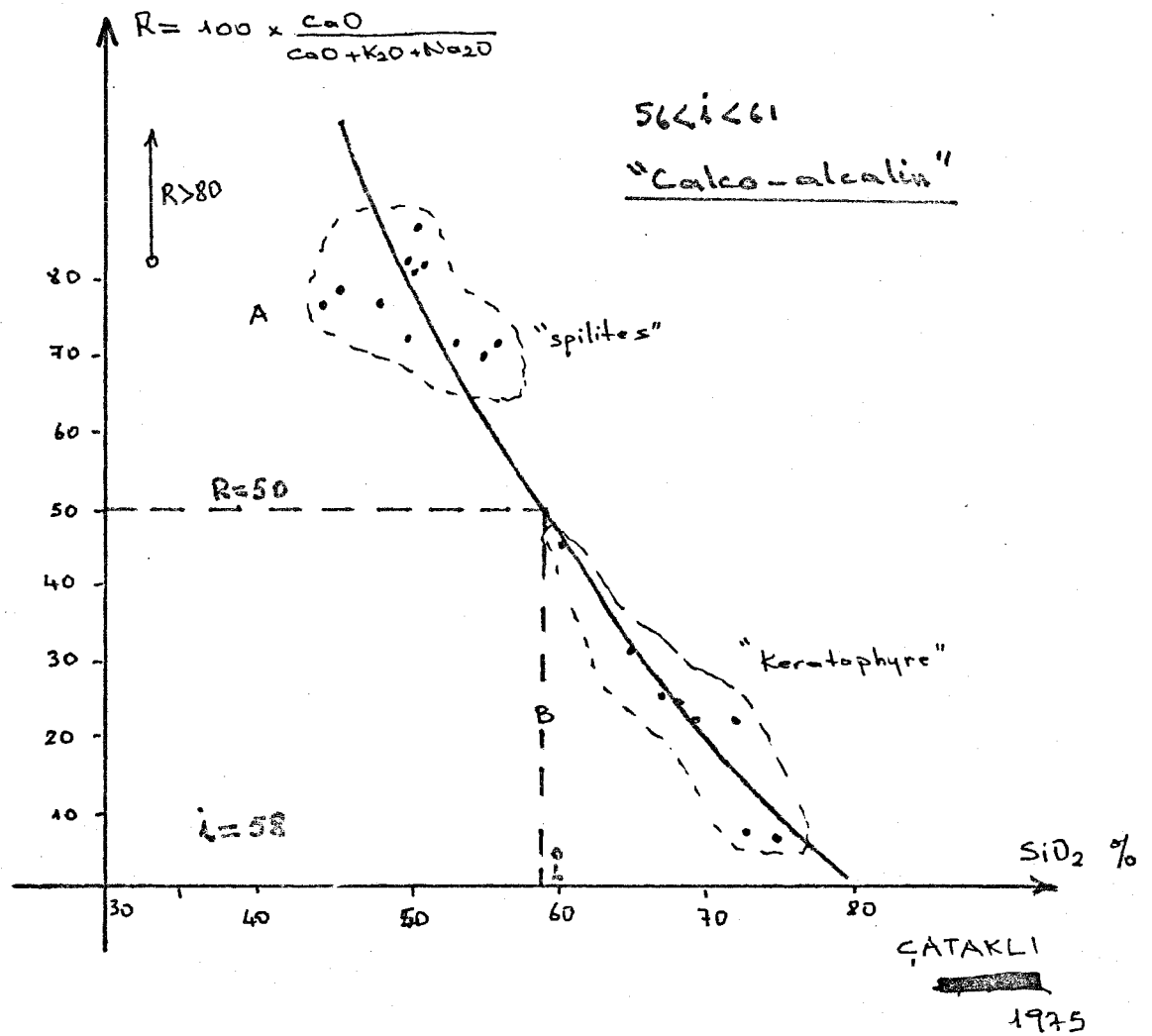
FIG. 44 - Diagramme de calco-alcalinité de YONG pour la série volcanique "probablement spilité-keratophyrique" de Tsalobia El Khedra (Mauritanie).
