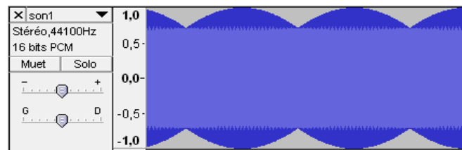
Figure 15 bis : Représentation temporelle d'un son pur de 11025 Hz, F_{ECH}=44100 Hz
