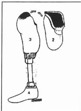
Figure 30 : emboîture tibiale "contact" orientée à collet PTS et manchon en cuir.
