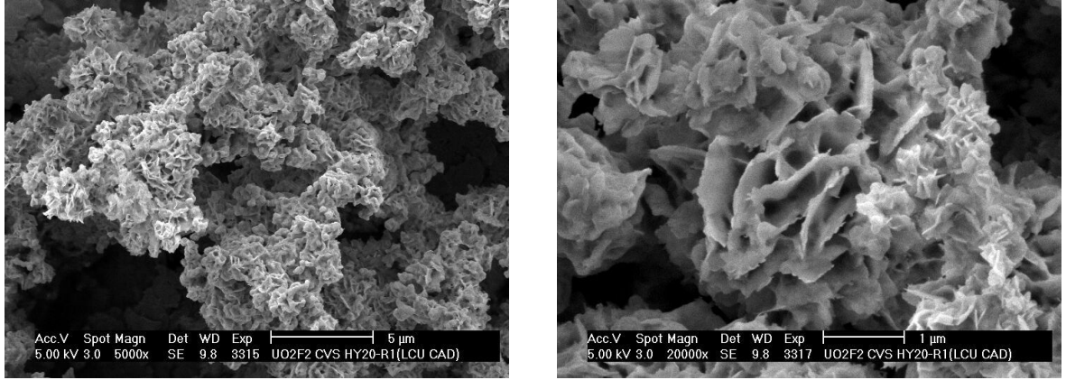
FIG. 11 – Clichés MEB d'une poudre d' \text{UO}_2\text{F}_2 [Ablitzer et al. 2002]
