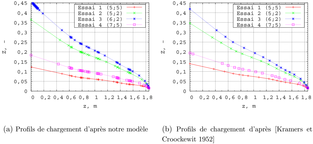
FIG. 4.4 – Comparaison des profils de chargement du four LCU calculés pour les conditions supposées du tableau 4.4.
