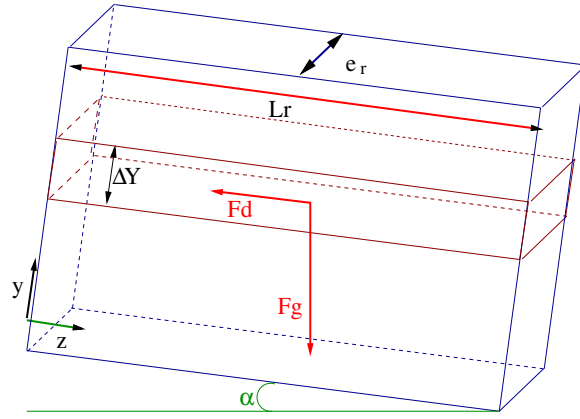
FIG. 2.1 – Représentation schématique du rideau de poudre
