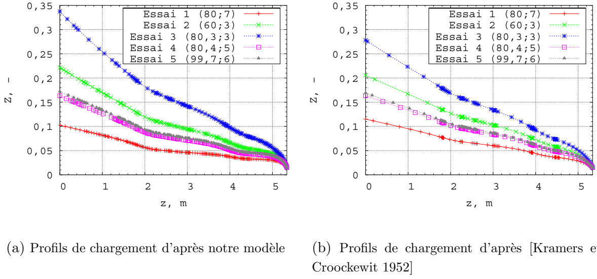
FIG. 4.3 – Comparaison des profils de chargement du four FBFC calculés pour les conditions des essais expérimentaux du tableau 4.3.
