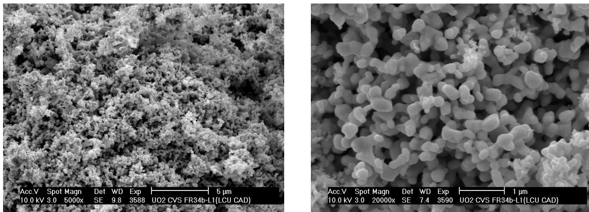
FIG. 12 – Clichés MEB d'une poudre d' \text{UO}_2 [Ablitzer et al. 2002]
