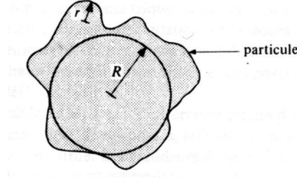
FIG. 8 – Arrondissement d'une particule
