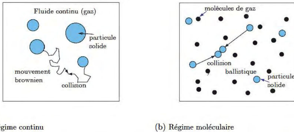
FIG. 3.1 – Schéma de principe des collisions entre particules pour les différents régimes de l'agglomération par mouvement brownien
