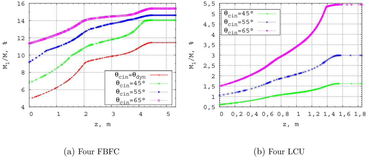
FIG. 4.13 – Quantité de poudre en phase dispersée le long des fours de conversion dans le cas d'un fonctionnement nominal
