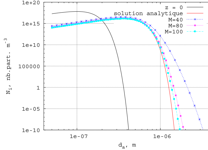
FIG. 2.2 – Comparaison des solutions analytiques et numériques pour différents nombres de sections dans la cas d'un noyau d'agglomération constant
