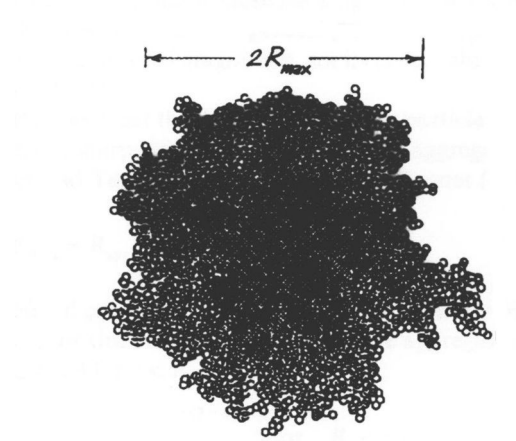
FIG. 9 – Exemple d'agrégat fractal de dimension fractale D_f = 2,5
