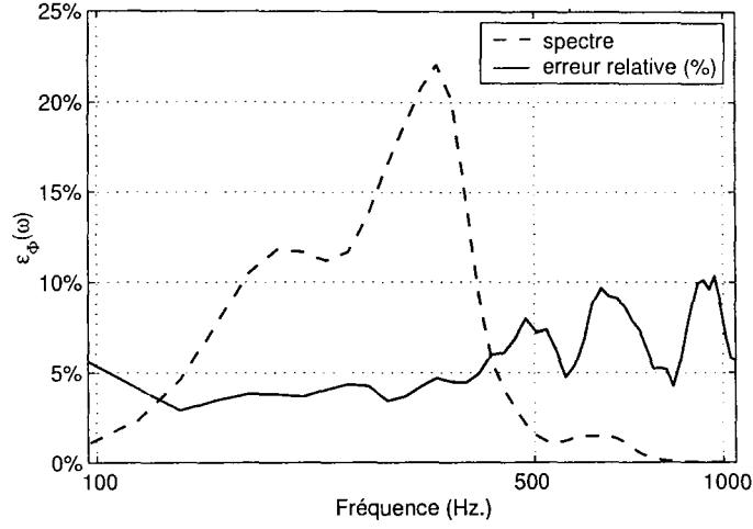
FIG. 2.10 – Variation de l'erreur de stationnarité fréquentielle \epsilon_\Phi(\omega) . L'erreur est superposée au spectre estimé moyen \hat{\Phi}_{S_1,m}(\omega) de la source S_1 . La fréquence d'échantillonnage choisie pour les mesures est de 5000 Hz.
