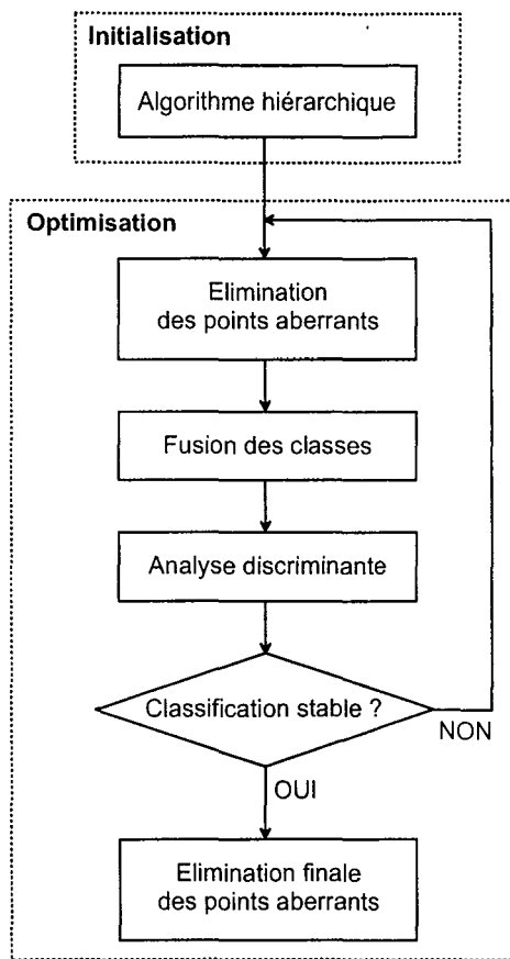
FIG. 5.18 – Organigramme de l'algorithme de classification non-supervisée.
