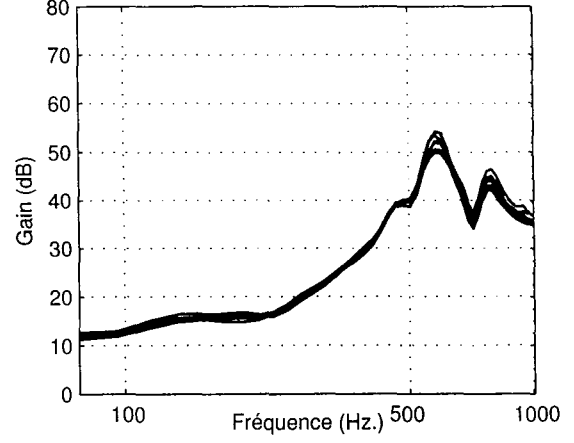
FIG. 2.17 – Superposition des réponses fréquentielles du système équipé du capteur C_2 (Littmann), estimées pour différentes pressions d'appui.
