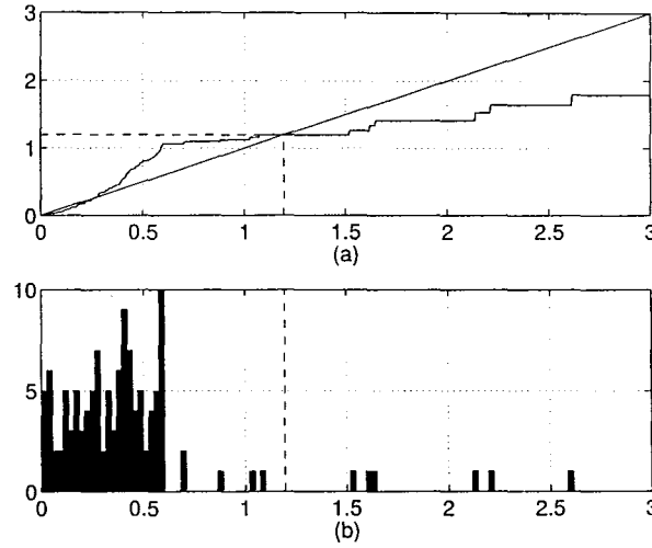
FIG. 3.8 – Pour une distribution empirique de w_x^{j,p} et un j donné : (a) les fonctions y = f_j(x) (pour F_a^j = 3 ) et y = x , montrant l'interprétation de point fixe et la valeur finale x_0 = S_L^j donnée par l'algorithme ; (b) l'histogramme des valeurs absolues des coefficients d'ondelette w_x^{j,p} . La ligne en pointillé représente le seuil de séparation entre le bruit (les petites valeurs) et le signal informatif.
