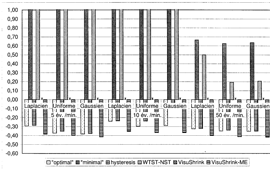
FIG. B.6 – Valeurs détaillées du critère ES pour les 6 algorithmes testés, pour un bruit additif coloré, en fonction du type de signal et de la distribution du bruit.
