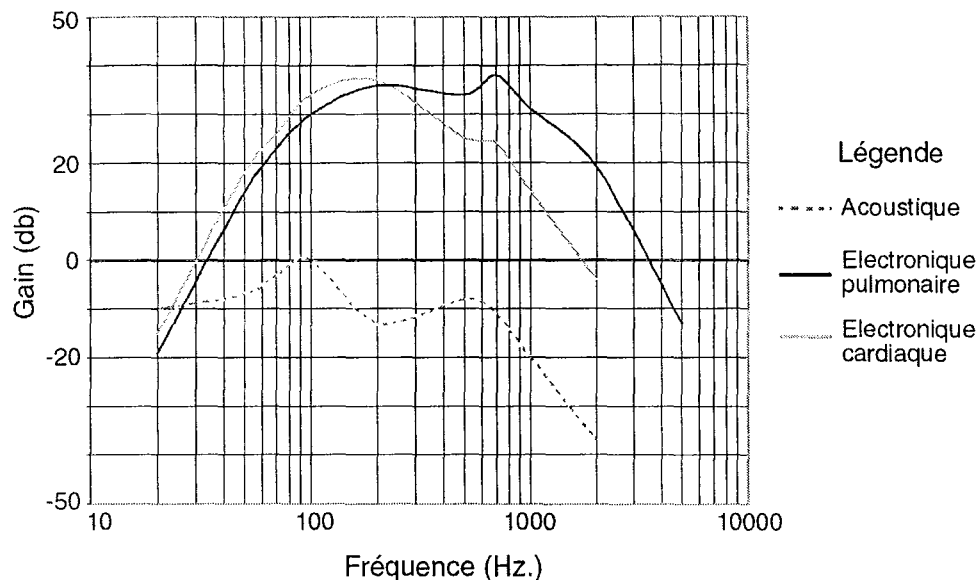
FIG. 2.5 – Exemple de réponses fréquentielles des stéthoscopes acoustiques et électroniques (les courbes présentées font partie de la documentation technique du stéthoscope électronique E-Scope produit par Cardionics Inc. http://www.cardionics.com , qui a deux modes de fonctionnement : cardiaque et pulmonaire).
