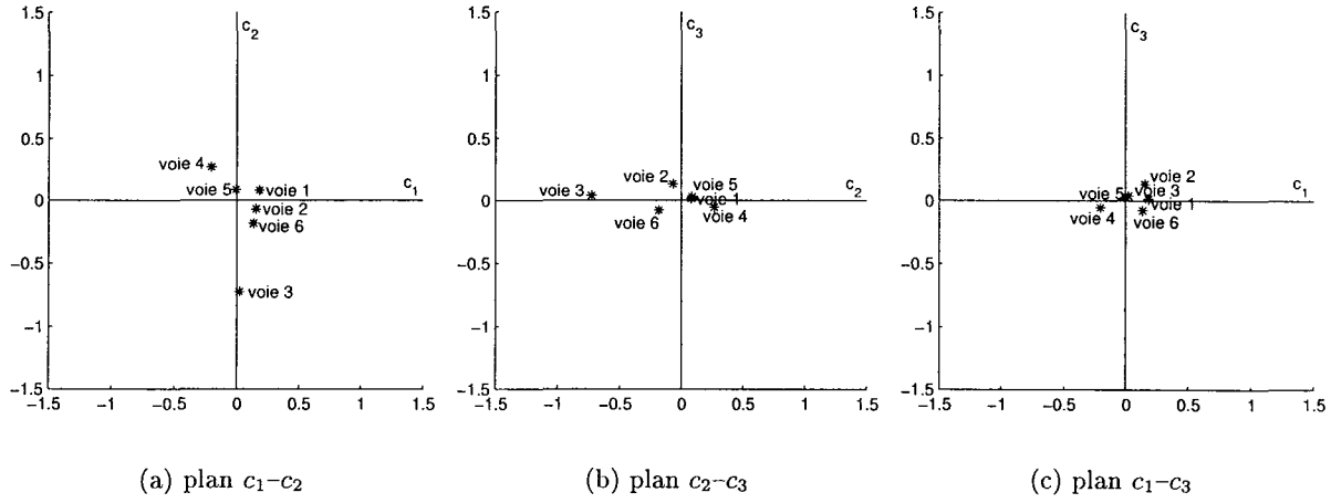
FIG. 5.15 – Projections des voies v_1 à v_6 sur les plans principaux de l'espace des sons individuels.
