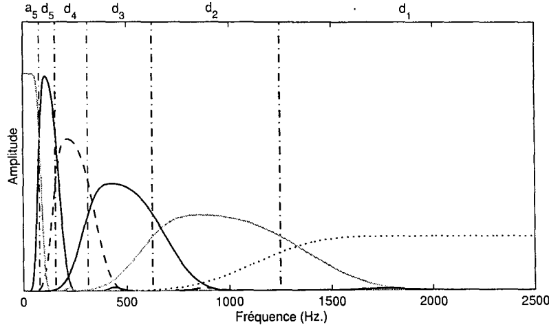
FIG. 4.1 – Spectres des ondelettes Daubechies no. 9 pour l'échelle de l'approximation et les 5 échelles des détails.
