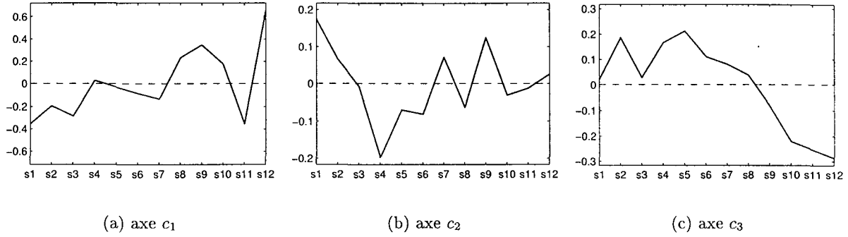
FIG. 5.10 – Évolution temporelle des séquences selon les axes principaux. c_1 \approx niveau sonore, c_2 \approx richesse/pauvreté en événements, c_3 \approx fréquence moyenne.
