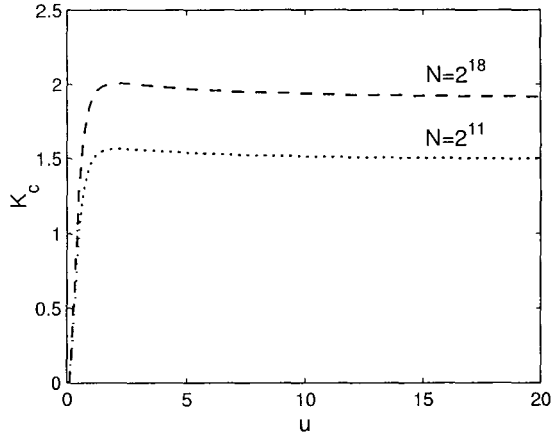
FIG. 3.13 – Variation de la constante K_c en fonction du paramètre u et de la taille du signal N .
