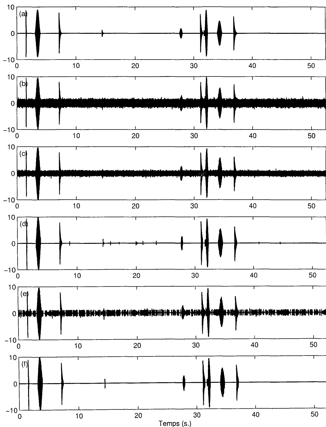
FIG. 3.23 – Résultats comparatifs du débruitage pour un bruit additif blanc, de distribution gaussienne : (a) signal d'origine ; (b) signal bruité ; signaux débruités par (c) algorithme "minimal", (d) algorithme par hystérésis, (e) WTST-NST, (f) VisuShrink . Le résultat fourni par l'algorithme "optimal" n'est pas présenté ici, car le signal est visuellement indistinct de (d). Le même argument est valable pour l'algorithme VisuShrink-ME , étant donné qu'il s'agit d'un bruit additif blanc.
