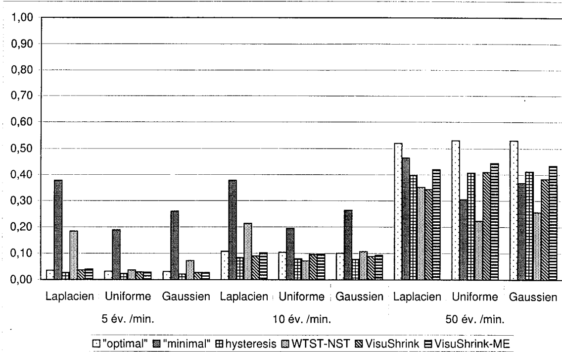
FIG. B.1 – Valeurs détaillées du critère EQM pour les 6 algorithmes testés, pour un bruit additif blanc, en fonction du type de signal et de la distribution du bruit.
