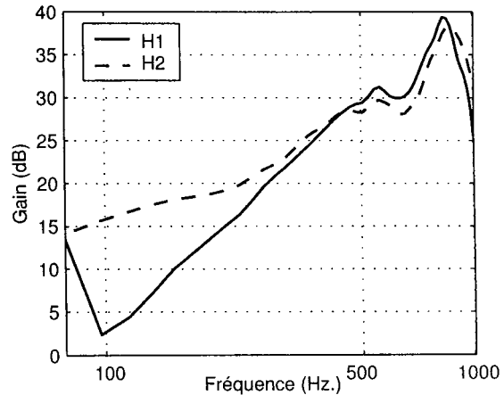
FIG. 2.15 – Réponse fréquentielle des systèmes identifiés (stéthoscope Colson = H_1 , stéthoscope Littmann = H_2 ).
