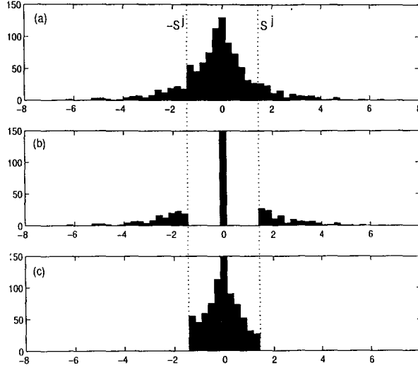
FIG. 3.7 – Histogramme des coefficients d'ondelette à l'échelle j (a) de l'estimation courante du bruit résiduel à l'itération l \Omega_{r,l}^j , (b) du signal informatif \Omega_{\Delta c,l+1}^j , (c) de la nouvelle estimation du bruit résiduel \Omega_{r,l+1}^j . Pour cet exemple, les coefficients d'ondelette du signal simulé suivent une loi de Laplace (l'axe des ordonnées n'est pas complètement représenté en (b) et (c)).
