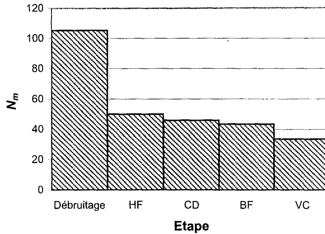
FIG. 4.6 – Évolution de l'indice N_m – nombre d'événements par minute. Les étapes de l'algorithme d'élimination d'artéfacts sont marquées en abscisse : HF = annulation des coefficients de haute-fréquence, CD = élimination des événements de courte durée, BF = élimination des événements de basse-fréquence, VC = validation croisée. L'ordonnée représente la valeur de l'indice après l'étape respective.
