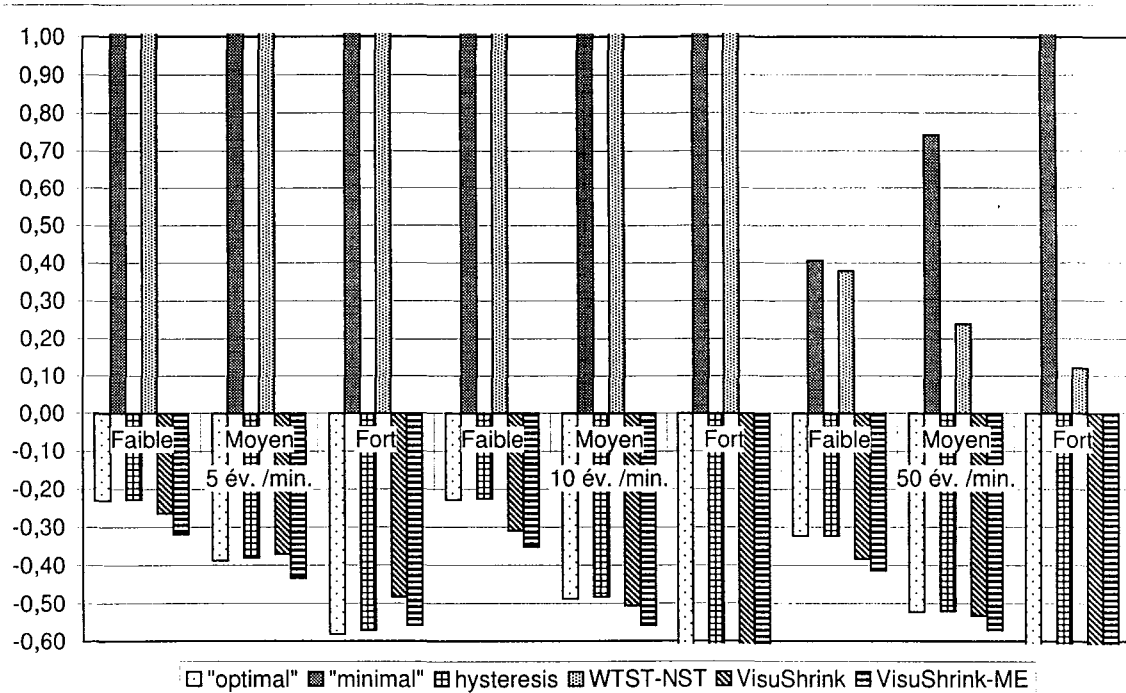
FIG. B.7 – Valeurs détaillées du critère ES pour les 6 algorithmes testés, pour un bruit additif blanc, en fonction du type de signal et de la puissance du bruit (Faible : \sigma = 0.5 , Moyen : \sigma = 1 , Fort : \sigma = 2 ).
