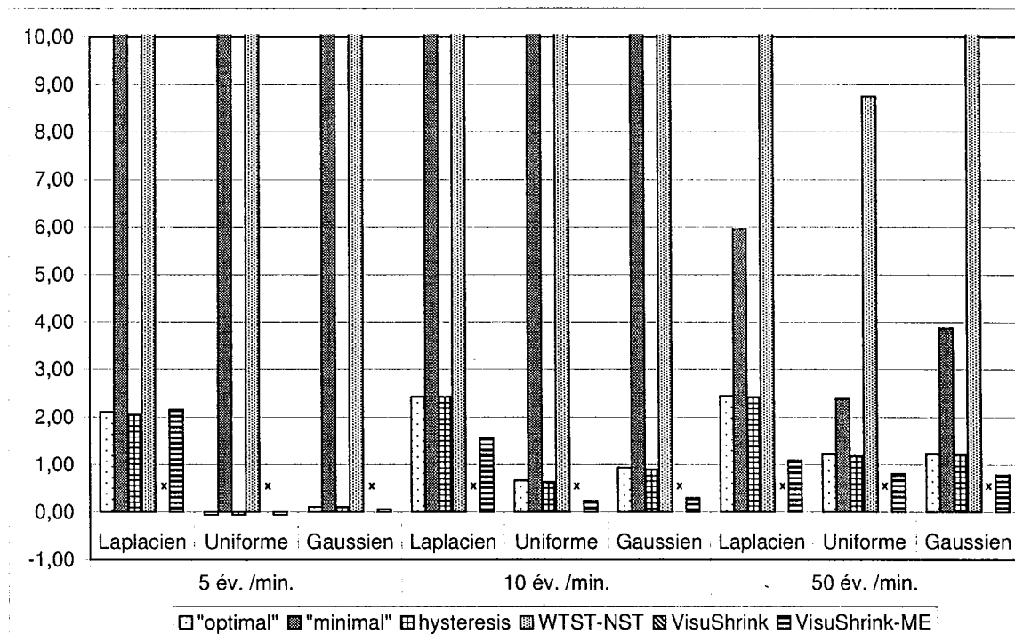
FIG. B.10 – Valeurs détaillées du critère ED pour les 6 algorithmes testés, pour un bruit additif coloré, en fonction du type de signal et de la distribution du bruit. L'algorithme VisuShrink n'est évidemment pas adapté au bruit coloré et il ne segmente pas le signal.
