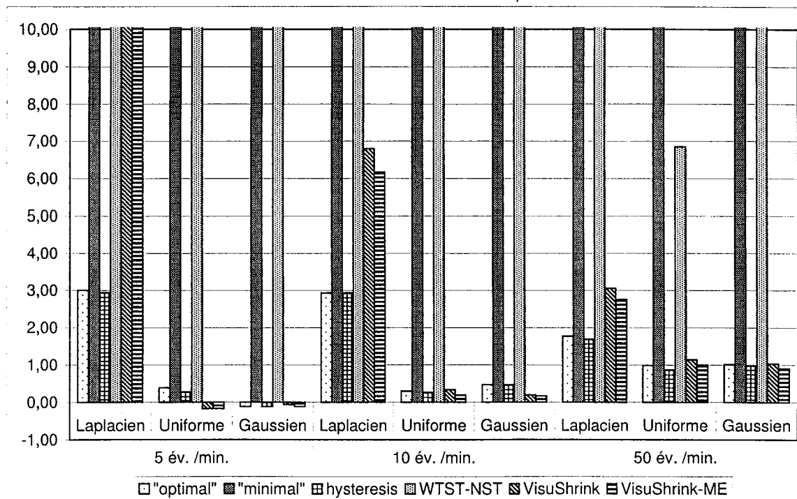
FIG. B.9 – Valeurs détaillées du critère ED pour les 6 algorithmes testés, pour un bruit additif blanc, en fonction du type de signal et de la distribution du bruit.
