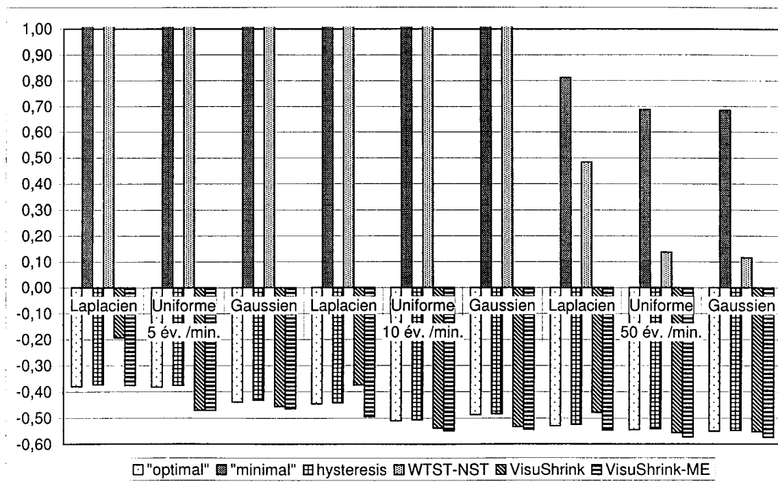
FIG. B.5 – Valeurs détaillées du critère ES pour les 6 algorithmes testés, pour un bruit additif blanc, en fonction du type de signal et de la distribution du bruit.
