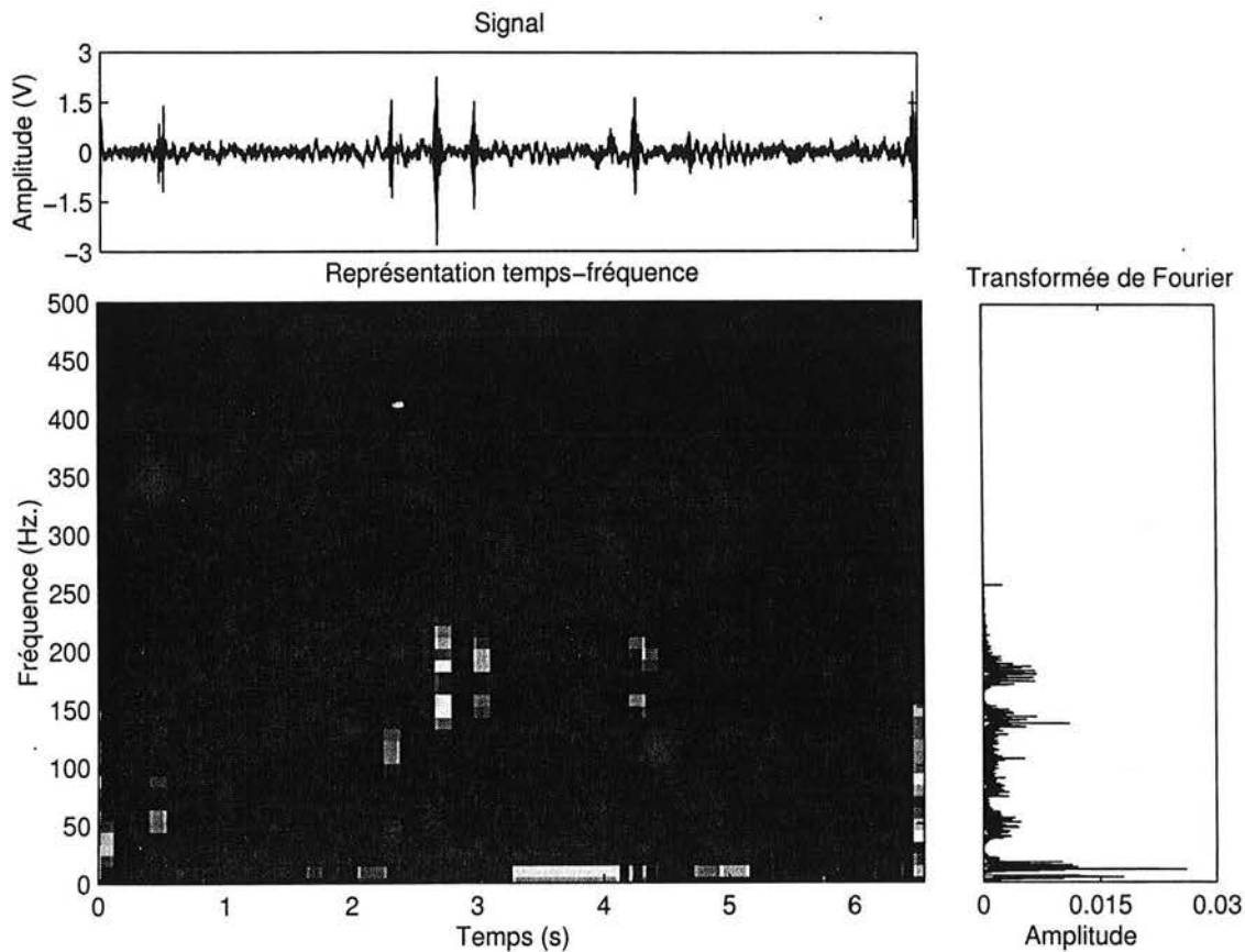
FIG. 3.3 – Représentation temps-fréquence
