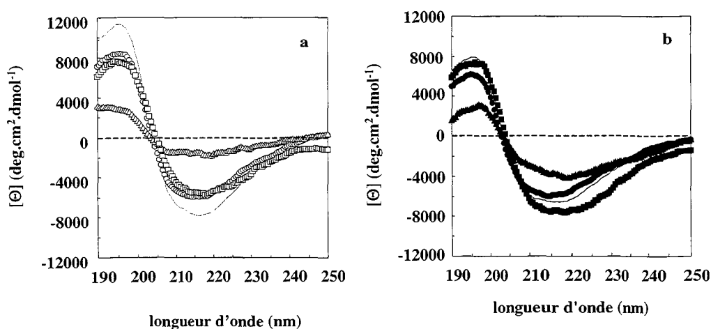
Figure 3.23 : Spectres UV obtenus par dichroïsme circulaire à 20°C pour des dispersions protéiques et des mélanges \beta -lg/gomme d'acacia/eau à une concentration totale en biopolymères de 0,05% et pH 4,2 et 20°C. (a) BLG (—) ; BLG/gomme d'acacia/eau, ratio Pr : Ps ( \circ ) 8 : 1 ; ( \triangle ) 2 : 1 ; ( \square ) 1 : 1. (b) BLG agr (—) ; BLG agr /gomme d'acacia/eau, ratio Pr : Ps ( \bullet ) 8 : 1 ; ( \blacktriangle ) 2 : 1 ; ( \blacksquare ) 1 : 1.
