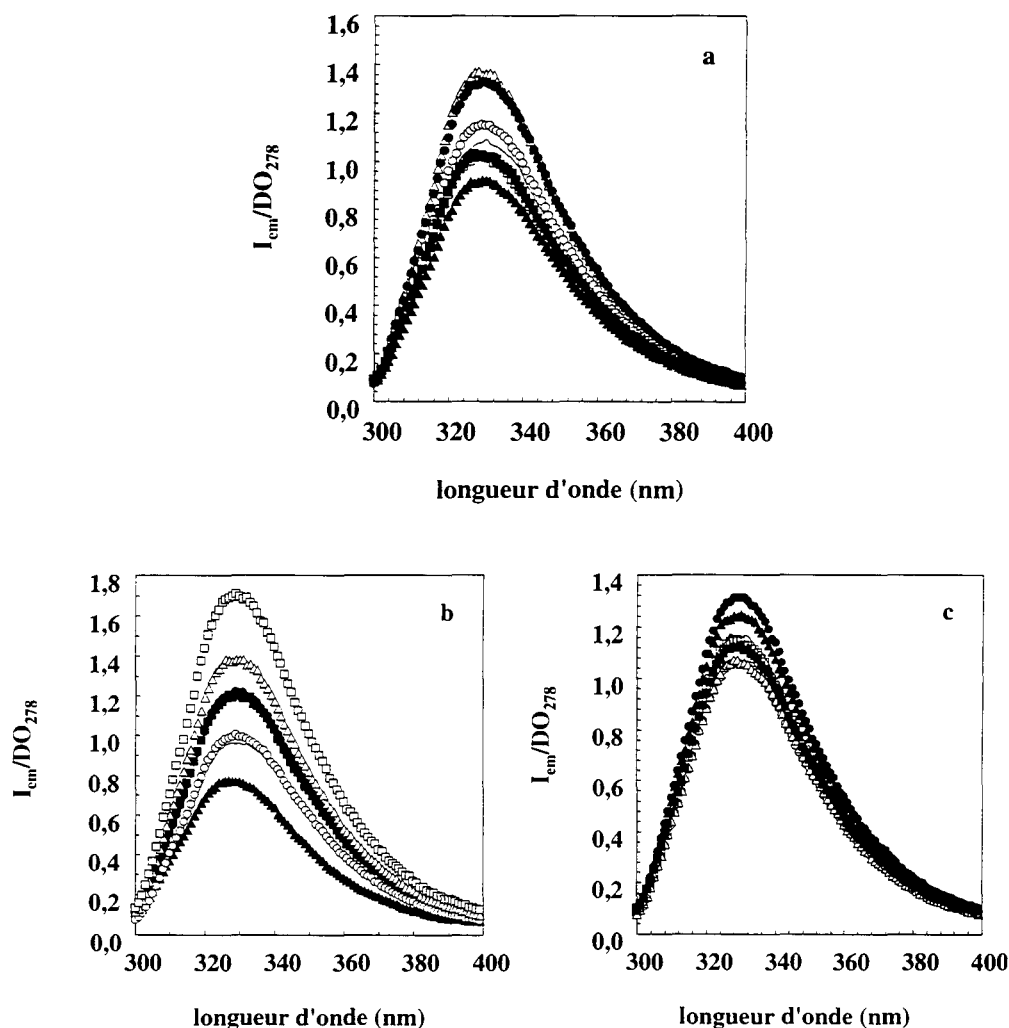
Figure 3.24 : Spectres de SFF à 20°C, normalisés par la concentration protéique ( DO_{278} ), des dispersions de BLG, BLG_{agr} et des mélanges BLG/gomme d'acacia/eau et BLG_{agr} /gomme d'acacia/eau à une concentration totale en biopolymères de 3%. BLG et BLG_{agr} (—). BLG/gomme d'acacia/eau, ratio Pr : Ps (○) 8 : 1; (△) 2 : 1; (□) 1 : 1. BLG_{agr} /gomme d'acacia/eau, ratio Pr : Ps (●) 8 : 1; (▲) 2 : 1; (■) 1 : 1. (a) pH 3,6; (b) pH 4,2; (c) pH 5,0.
