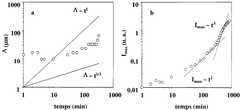
Figure 4.22 : Variation de (a) la longueur de corrélation \Lambda , (b) l'intensité maximale diffusée au cours du temps à 20°C dans un mélange BLG agr (8)/gomme d'acacia(1)/eau à pH 3,6 et une concentration totale en biopolymères de 0,1%. Les droites représentent les modèles de croissance en puissance.
