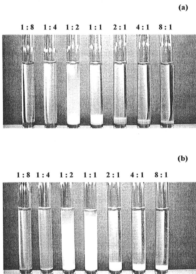
Figure 3.6 : Séparation de phase obtenue à différents ratios Pr : Ps de mélange, après 2 jours à pH 3,6 et 20°C. (a) mélange BLG /gomme d'acacia/eau à 4,5% ; (b) mélange BLG_{agr} /gomme d'acacia/eau à 5%.
