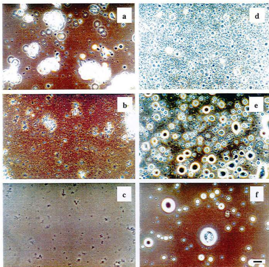
Figure 3.12 : Micrographies obtenues par MOCP à 20^{\circ}\text{C} de la structure des mélanges \text{BLG}_{\text{agr}}/\text{gomme d'acacia}/\text{eau} (a-c) et \text{BLG}/\text{gomme d'acacia}/\text{eau} (d-f) à pH 4,2 à une concentration totale en biopolymères de 1%. Ratio Pr : Ps : 8 : 1 (a-d) ; 2 : 1 (b-e) ; 1 : 1 (c-f). La barre d'échelle représente 20\ \mu\text{m} .
