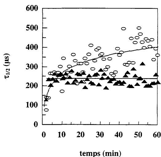
Figure 4.3 : Evolution du temps de demi-décroissance de la fonction de corrélation ( \tau_{1/2} ) calculé à 20°C pour des mélanges \beta -lg/gomme d'acacia/eau à pH 4,2 et une concentration totale en biopolymères de 1%. (○) Mélange BLG_{agr}(2)/ gomme d'acacia(1)/eau. (▲) Mélange BLG(1)/ gomme d'acacia(1)/eau. Les lignes continues constituent uniquement un repère visuel.
