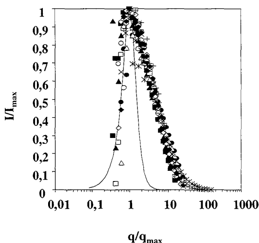
Figure 4.23 : Courbes de mise à l'échelle de l'intensité diffusée à 20°C dans un mélange BLG agr (8)/gomme d'acacia(1)/eau à pH 3,6 et une concentration totale en biopolymères de 0,1 % en fonction du vecteur d'onde normalisé. Temps après mélange des biopolymères : (○) 1 min ; (●) 2 min ; (△) 3 min ; (▲) 4 min ; (□) 5 min ; (■) 10 min ; (◇) 30 min ; (◆) 45 min ; (×) 60 min ; (※) 450 min ; (+) 840 min. La courbe pleine représente le modèle de Furukawa, caractéristique des phases tardives de la décomposition spinodale.
