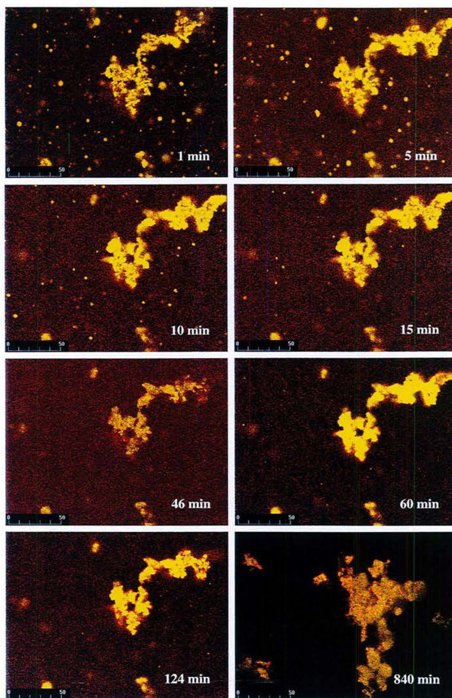
Figure 4.7 : Cinétique de séparation de phase à 20°C obtenue par MCBL dans le mélange BLG agr (8)/gomme d'acacia(1)/eau à pH 4,2 et à une concentration totale en biopolymères de 1%. La barre d'échelle représente 50 μm.
