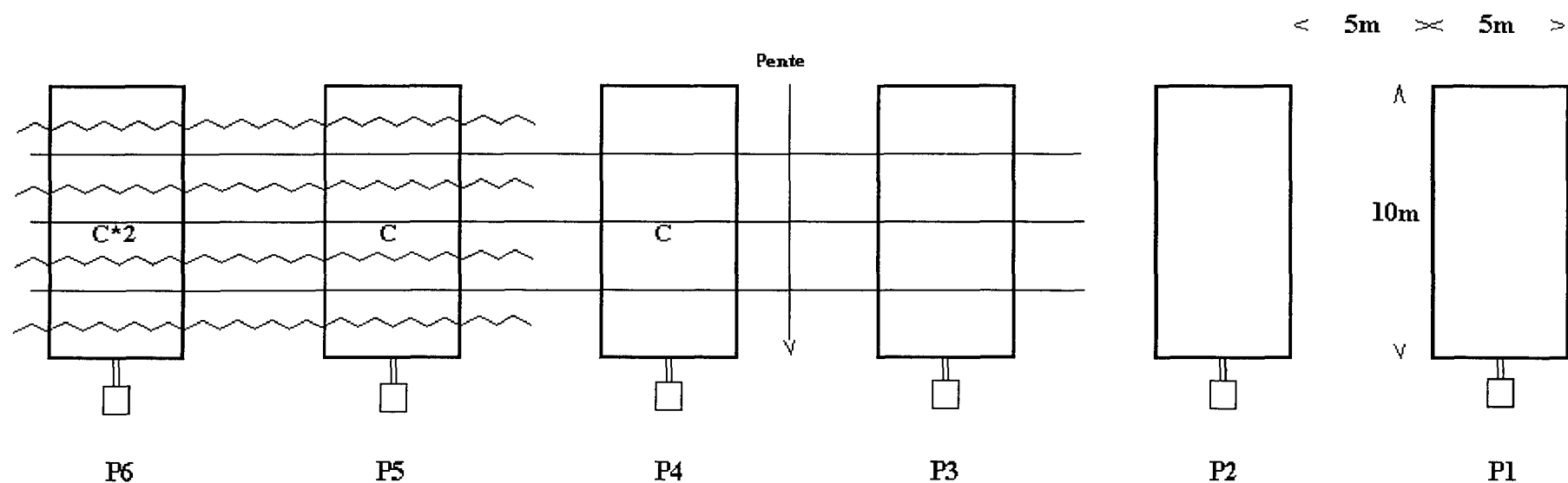
Figure 4 : Essai "Travail du sol * compost" de Thyssé-Kaymor mis en place en 1990 par Sène (1993)
