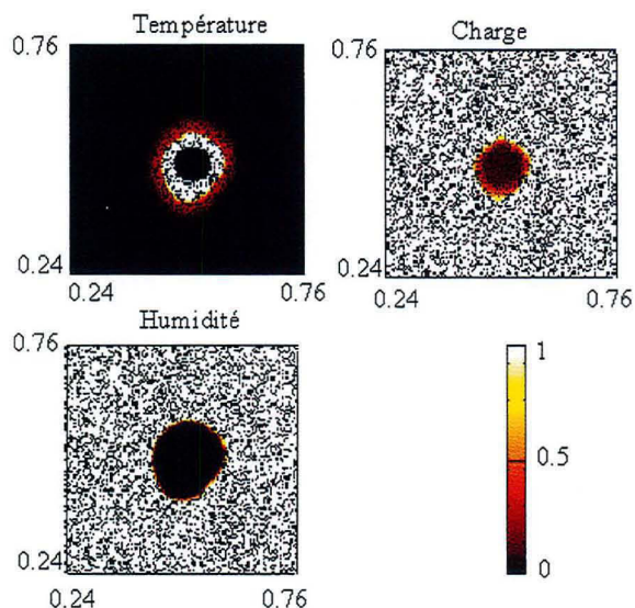
FIG. 5.15 – Profils de température, de charge et d'humidité
