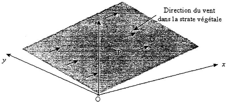
FIG. 4.7 – Surface plane avec vent dans le plan (Oxz)
