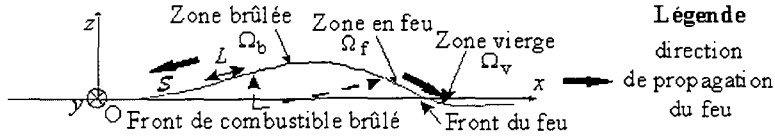
FIG. 1.11 – Coupe de la strate de broussaille à l'échelle gigascopique
