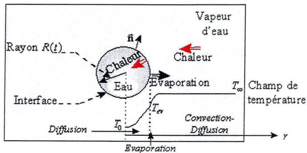
FIG. 4.2 – Evaporation d'une goutte dans sa vapeur
