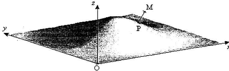
FIG. 4.4 – Coordonnées curvilignes associées à une surface
