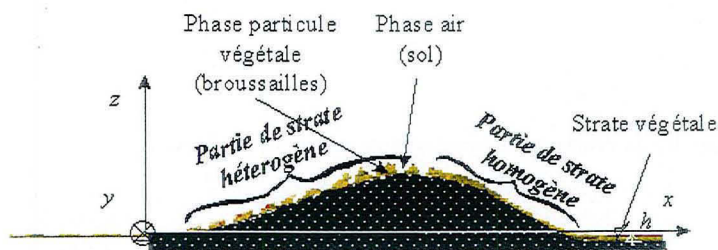
FIG. 3.3 – Hétérogénéité horizontale d'une strate de végétation
