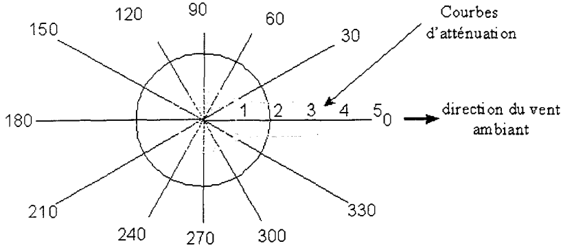
FIG. 4.13 - Courbes d'atténuation anisotrope
