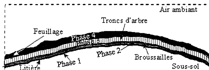
FIG. 3.1 – Différentes phases végétales
