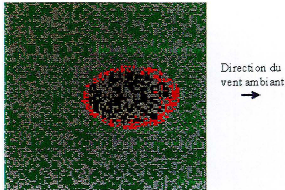
FIG. 5.7 – Rôle d'un vent ambiant global (Etape 32)
