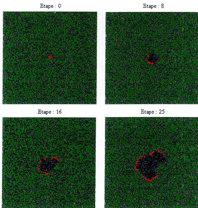
FIG. 5.4 – Exemple de propagation du feu ( d=0.6 )
