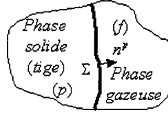
FIG. 3.13 – Interface séparant deux milieux
