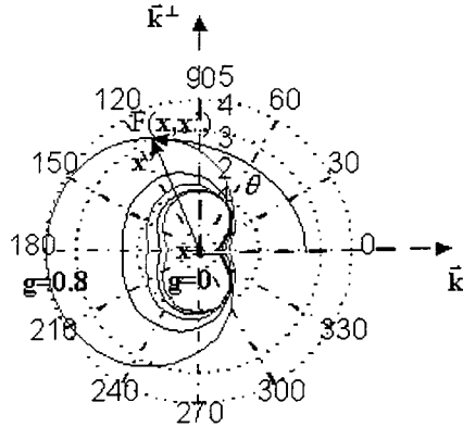
FIG. 2.6 - Fonctions indicatrices pour f = 1 , h = 0.5 et g variant de 0 à 1
