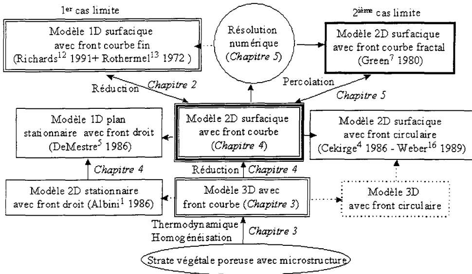
FIG. 1.20 – Classification des modèles par échelles
