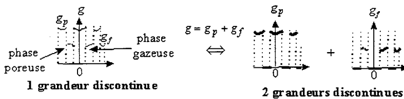
FIG. 3.11 – Grandeurs mésoscopiques associées aux différentes phases
