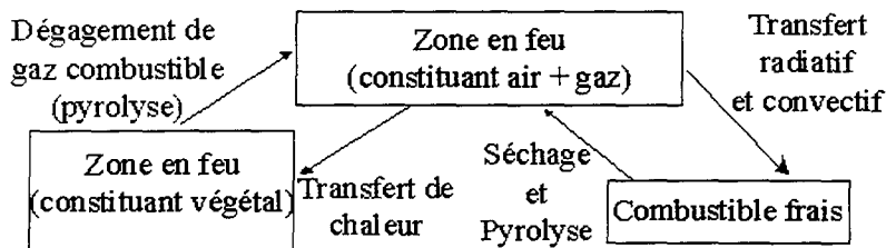
FIG. 1.15 – Transferts d'énergie et de masse
