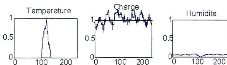
FIG. 5.16 – Profils dans la section y = 0.5
