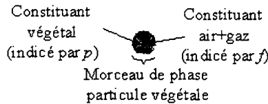
FIG. 3.4 - Morceau de phase particule végétale
