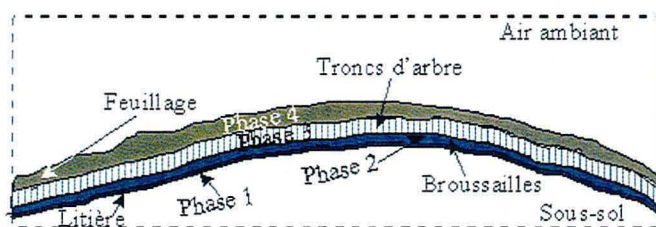
FIG. 1.9 – Différentes phases végétales
