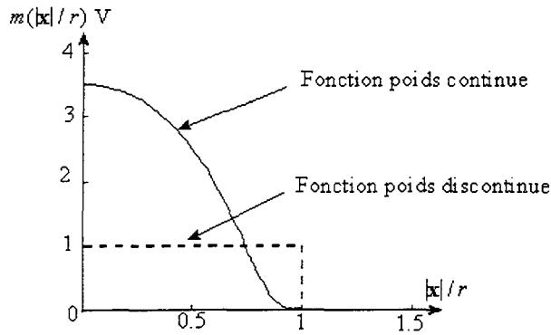
FIG. 3.10 – Exemple de fonctions poids
