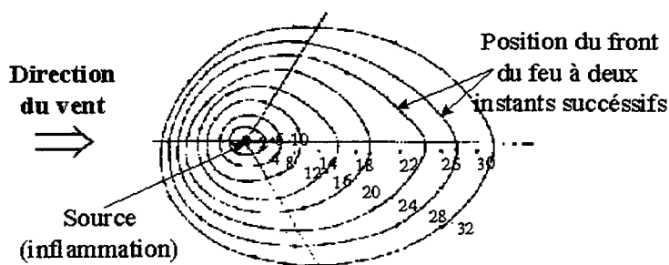
FIG. 5 - Expérience d'évolution du front du feu, dans une forêt homogène, uniforme, à partir d'un point source (Peet 1971)
