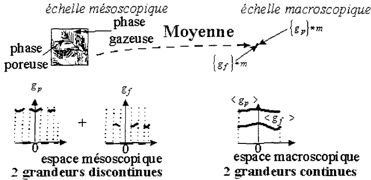
FIG. 3.12 – Grandeurs mésoscopiques et grandeurs macroscopiques associées
