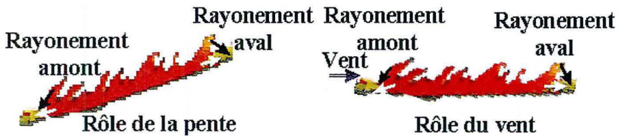
FIG. 1.19 – Influence de la pente et du vent sur le transfert radiatif
