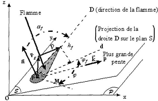
FIG. 4.11 - Forme de la flamme
