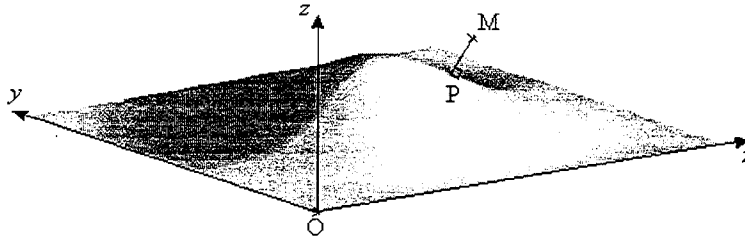
FIG. 4.3 – Paramétrage curviligne de la surface \mathcal{S}
