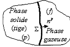
FIG. 3.9 – Interface séparant deux milieux
