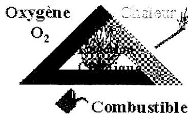
FIG. 1 - Triangle du feu
