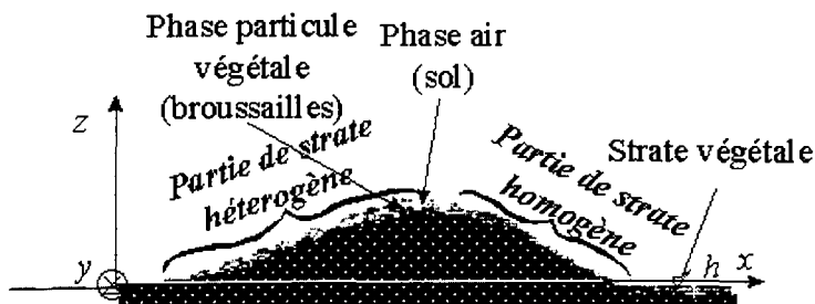
FIG. 1.10 - Hétérogénéité horizontale d'une strate de végétation
