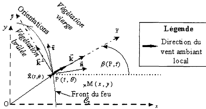
FIG. 2.3 - Paramétrage du front de feu
