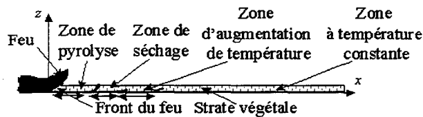
FIG. 1.16 – Différentes zones en avant du front du feu
