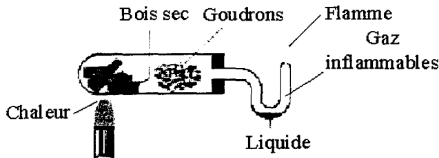
FIG. 1.17 – Pyrolyse du bois
