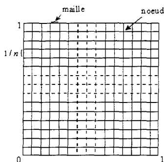
FIG. 5.1 - Réseau carré
