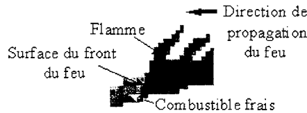
FIG. 1.7 - Coupe de la surface représentant le front du feu
