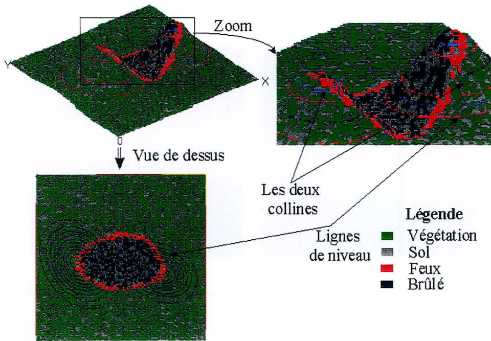
FIG. 5.9 – Rôle d'une pente locale
