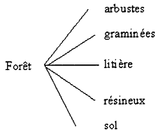
FIG. J.1 – Hiérarchie de l'objet forêt
