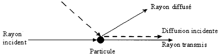
FIG. 3.6 - Diffusion et diffusion incidente
