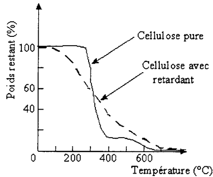
FIG. 1.18 – Courbes de pyrolyse avec et sans retardant
