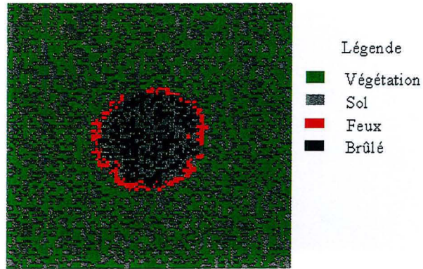
FIG. 5.5 - Densité d'occupation importante ( d=0.8 , Etape 32)
