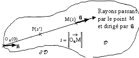
FIG. 4.9 - Domaine \mathcal{D} entourant un point M
