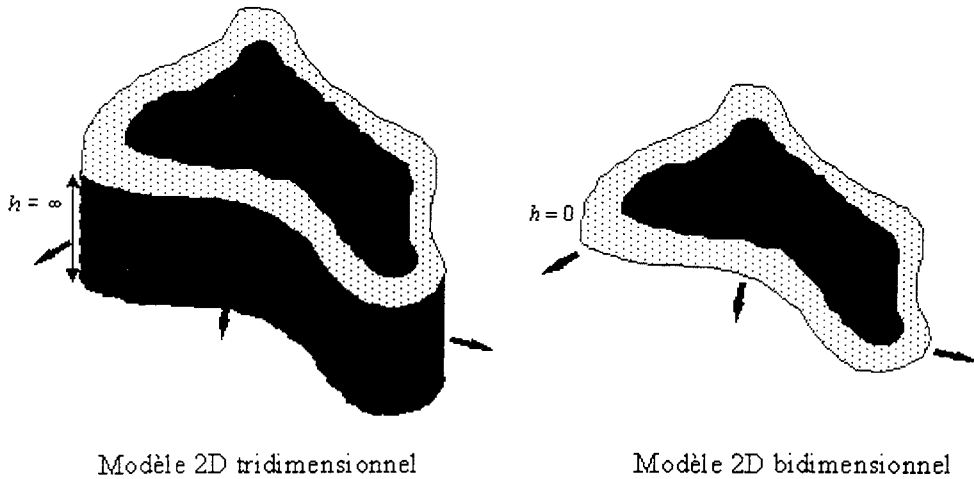
FIG. 1.21 – Différents espaces d'étude
