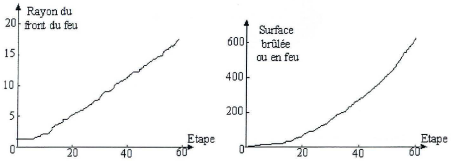
FIG. 5.6 - Evolution du rayon du front du feu et de la surface en feu
