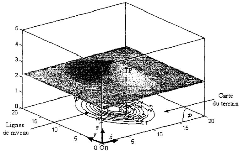
FIG. 4.5 - Lignes de niveau associées à la surface S
