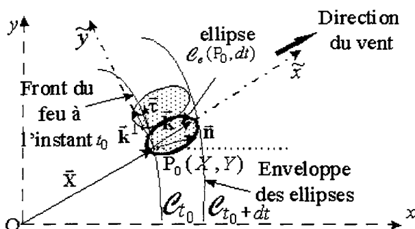
FIG. 2.4 – Principe de Huygens
