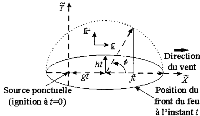
FIG. 2.2 – Evolution du front du feu (vue de dessus de la strate végétale à l'échelle gigantesque)
