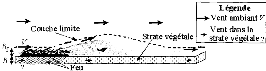
FIG. 1.11 – Coupe de la strate de broussaille à l'échelle gigascopique
