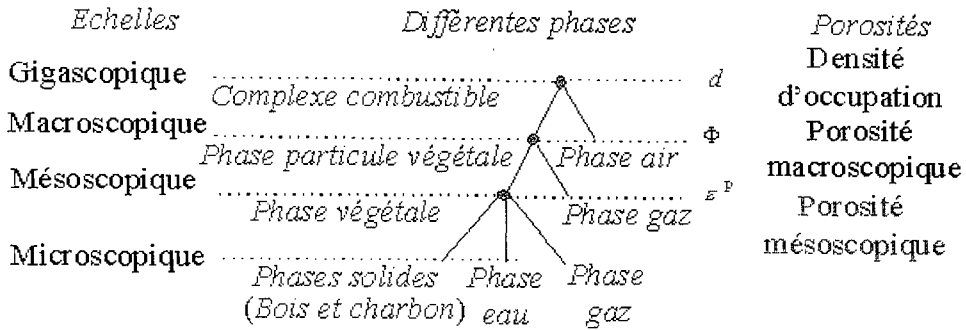
FIG. 1.14 - Les différentes échelles et les phases associées
