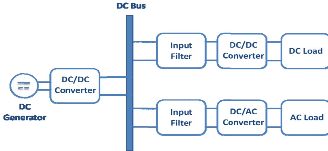
Figure 1.2: Système à Puissance Distribué (SPD)
