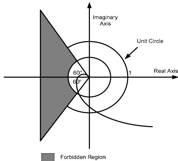
Figure 1.7: Région interdite par la méthode GMPM
