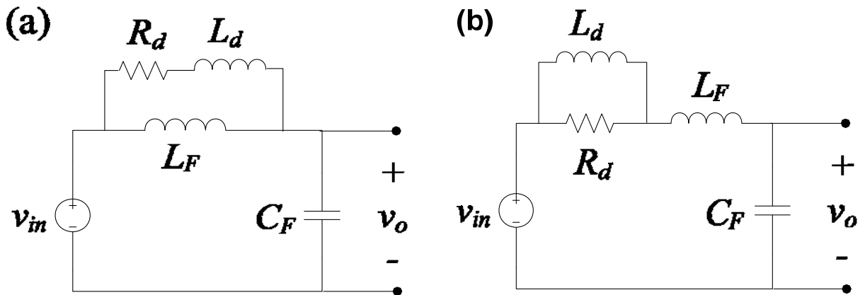
Figure 1.11: méthode pratique pour régler l'amortissement du filtre d'entrée sur les réseaux alternatifs; (a): circuit R_d - L_d en série; (b): circuit R_d - L_d parallèle.
