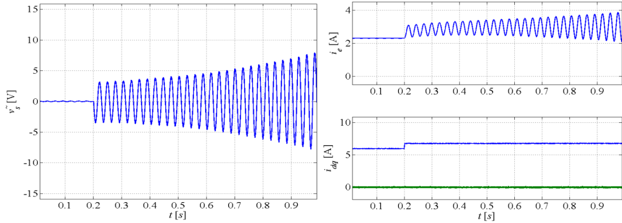
Fig. 2.7- Instabilité des variation de tension du bus DC ( \tilde{v}_s ) et du courant du bus DC ( i_e ) après un échelon de puissance ( C=500\mu F , K=0 )
