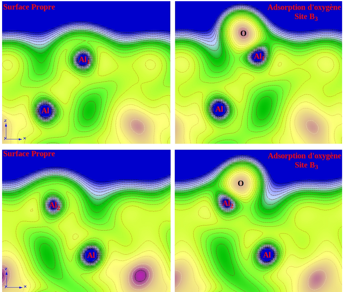
Figure 9 : Densité de charge du site B 3 (composé par les atomes Al 1 et Al 2 ) avant et après l'adsorption de l'atome d'oxygène.
