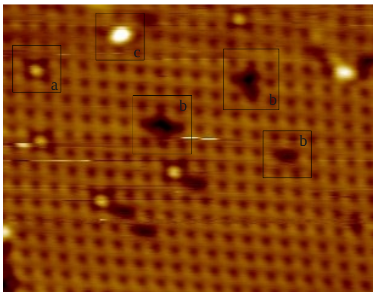
Figure 10 : Image STM expérimentale enregistrée à 300K et pour un taux de couverture égal à 0,5 MLE (9,58x12,13 nm 2 , V_{bias} = -2 V). Différents types de motifs observés dans les STM sont entourés par un cadre noir.
