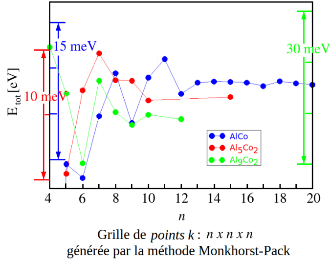
Figure 2 : Énergie totale E_{tot} vs grille de points k pour les systèmes massifs B2-AlCo ( \sigma = 0,1 eV, E_{cut} = 450 eV), Al_5Co_2 et Al_9Co_2 ( \sigma = 0,1 eV, E_{cut} = 350 eV).
