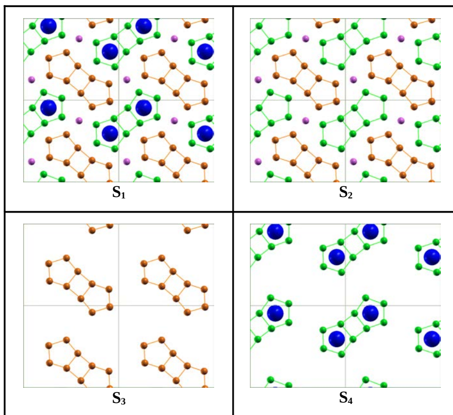
Figure 1 : Les 4 modèles de la surface (100)o- Al_{13}Co_4 (cellule unité de surface de 2 \times 2 ). Les petites sphères (vertes, oranges et roses) correspondent aux atomes d'aluminium, et grandes sphères (bleues) aux atomes de cobalt. Deux types de motifs bipentagonaux apparaissent sur les modèles : les atomes d'aluminium des motifs en vert (resp. orange) sont situés légèrement au dessus (au dessous) de la position moyenne du plan dans le cas du plan complet P . Les atomes d'aluminium représentés en rose sont les atomes ciments ou « glue atoms ».
