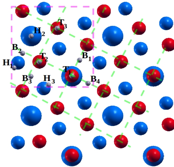
Figure 2 : Sites d'adsorption des atomes d'oxygène (petites sphères grises) sur la surface (001)Al 9 Co 2 (cellule unité de surface de 2x2 – maille élémentaire de surface en ligne pointillée rouge). Les sphères rouges correspondent aux atomes d'aluminium d'extrême surface. Les sphères bleues correspondent aux atomes de la sous-surface : les sphères de taille moyenne correspondent aux atomes d'aluminium et les grandes sphères aux atomes de cobalt.
