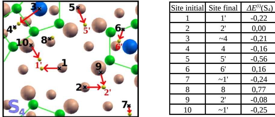
Figure 6 : À gauche : Positions initiales (croix) et finales (sphères jaunes) des atomes de Pb déposés sur le modèle de surface S 4 . Les atomes de la sous-surface sont également montrés (sphères crème-orange). Les grandes sphères représentent les atomes de cobalt et les sphères de taille moyenne représentent les atomes d'aluminium. À droite : Énergies relatives d'adsorption \Delta E^{(i)} = E_{Slab+Pb}^{(i)} - E_{Slab+Pb}^{(2')} (unités en eV) des différents sites finaux (initialement déposés sur le site i ) occupés par les atomes de Pb.
