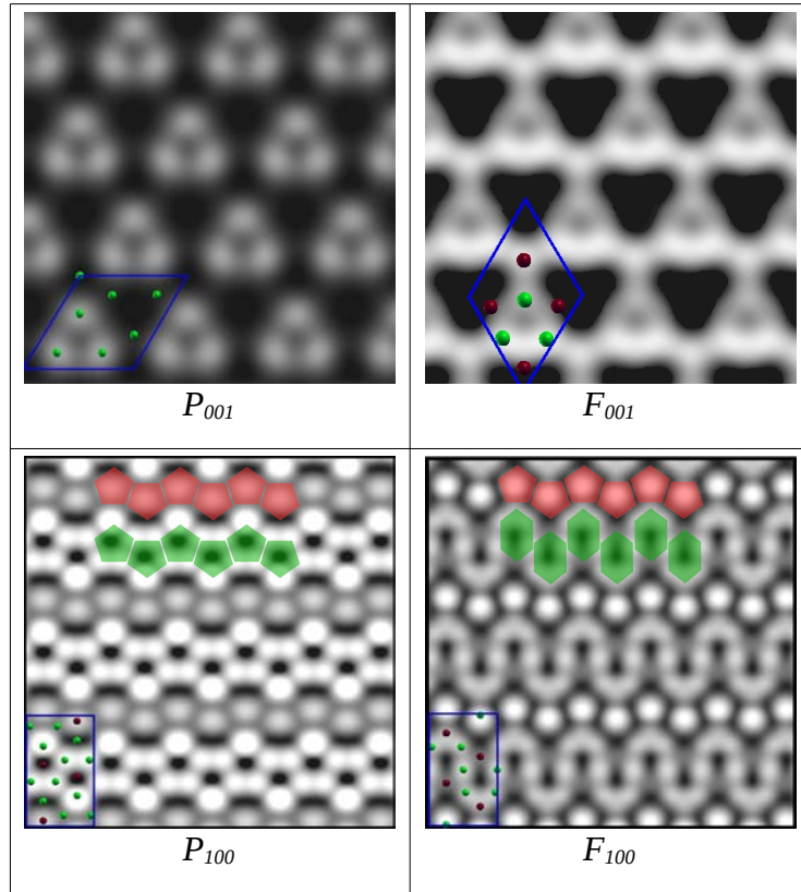
Figure 3 : Images STM simulées à partir de différents modèles de surface du cristal \text{Al}_5\text{Co}_2 , en utilisant h = 3 \text{ Å} et V_{PS} = 0,7 \text{ V} . Une maille élémentaire de surface est superposée : les sphères rouges correspondent aux atomes de cobalt et les sphères vertes représentent les atomes d'aluminium.
