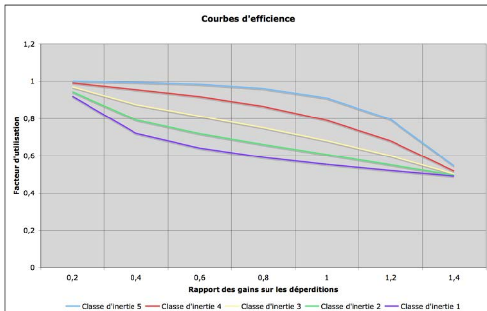
Figure 34. Courbes d'efficacité.
