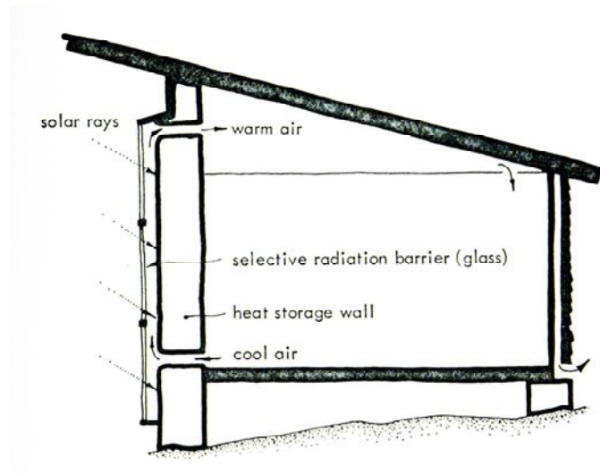
Figure 24. Coupe schématique de la maison d'Odeillo : principe du mur Trombe-Michel. (Mazria 2005)
