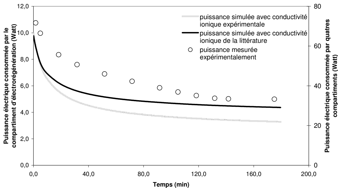
Figure 4-10: Comparaison expérience et modèle : puissance électrique consommée
