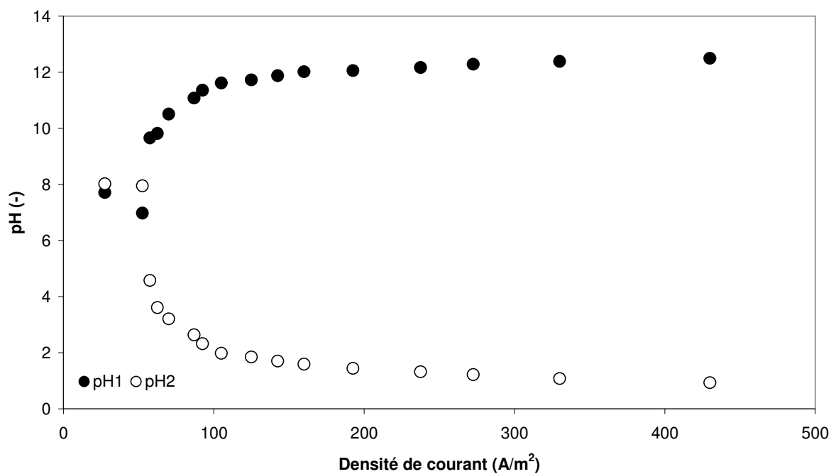
Figure 3-31: Variation de pH ( \text{pH}_1 et \text{pH}_2 ) en régime stationnaire en fonction de la densité de courant dans le cas de la dissociation de l'eau dans un couplage de la membrane échangeuse de cations et de résine échangeuse d'anions (MC+RA)
