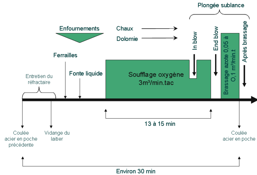
Figure 1.3 – Processus d’élaboration d’une coulée en poche
