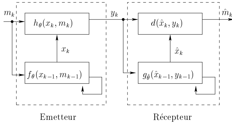
FIGURE 1.4 – Chiffrement par inclusion
