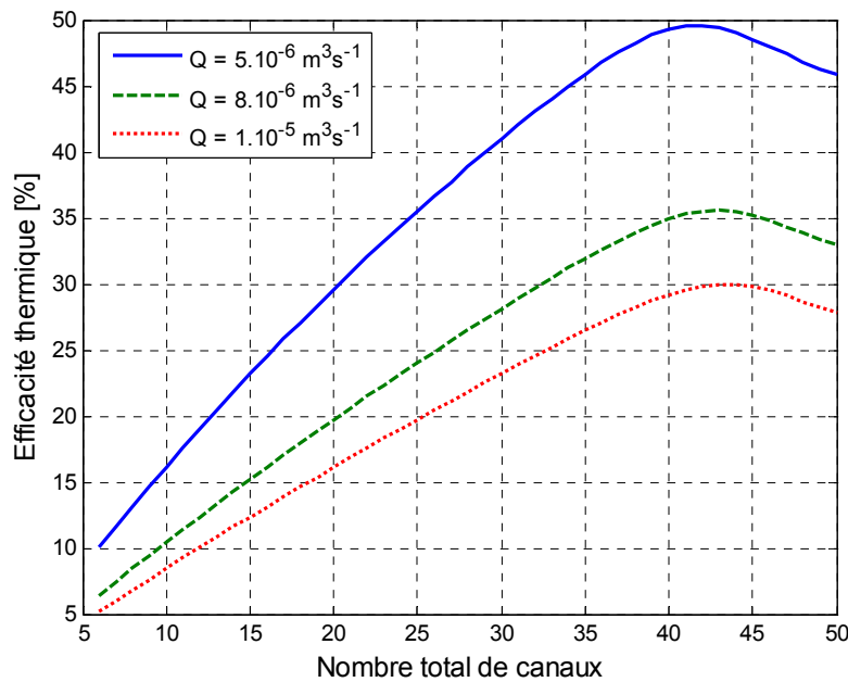
Figure IV.5. Effacité globale calculée pour différentes configurations à deux échelles présentant la même surface d'échange à différents débits d'entrée.
