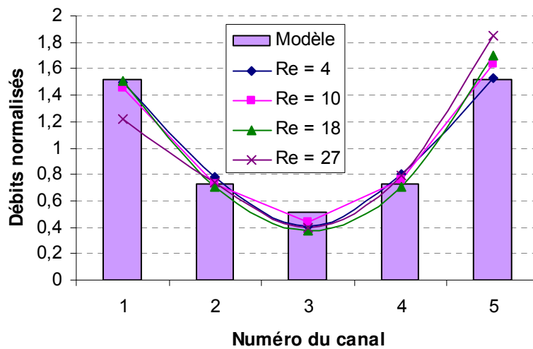
Figure III.9. Comparaison des distributions du fluide normalisées par la moyenne correspondante.
