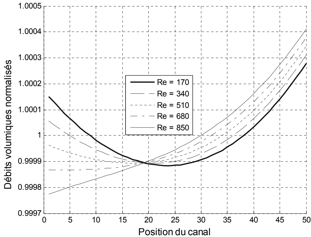
Figure II.7. Distribution des débits pour différents nombres de Reynolds et en introduisant les effets des pertes de charge singulières.
