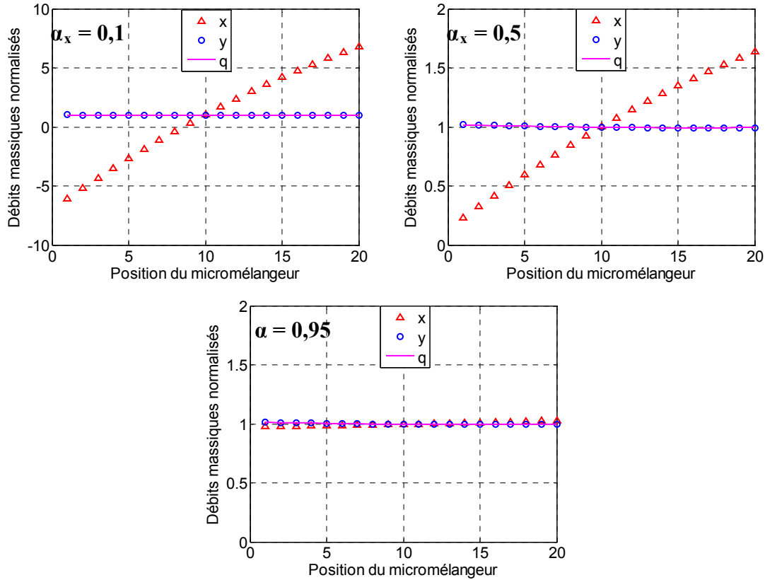
Figure VI.8. Distribution des débits massiques normalisés pour différentes fractions volumiques, dans un système azote/eau modélisé par un modèle de perte de charge linéaire ( \alpha_x = 0,1 à gauche, \alpha_x = 0,5 à droite et \alpha_x = 0,95 en bas).
