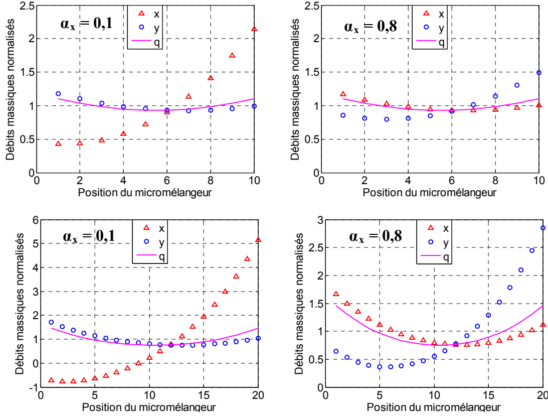
Figure VI.4.A. Distribution des débits normalisés pour deux fractions volumiques différentes ( \alpha_x = 0,1 à gauche et \alpha_x = 0,8 à droite) et deux valeurs du nombre total de canaux en parallèle ( n = 10 en haut et n = 20 en bas) : Cas A dans le Tableau VI.1.
