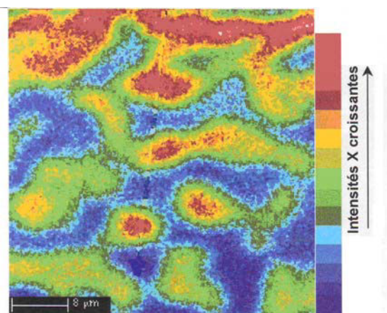
Figure A3.IV.8. Cartographie de distribution de Mn pour l'acier Fe-0.07C-1.5Mn-0.32Si-0.59Cr, maintien à 775°C pendant 33 min et la trempe [PETI99].
