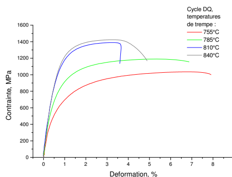
Figure A3.II.5. Courbes de traction pour les cycles DQ.
