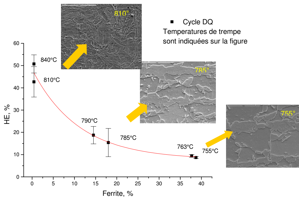
Figure A3.V.2. Evolution de HE avec l'accroissement du taux de ferrite.
