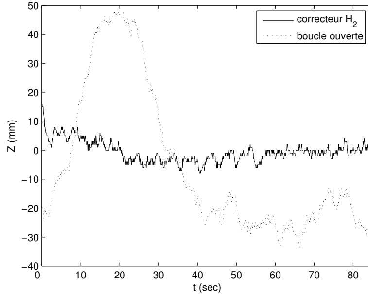
Figure 10: Évolution du décentrement de bande
