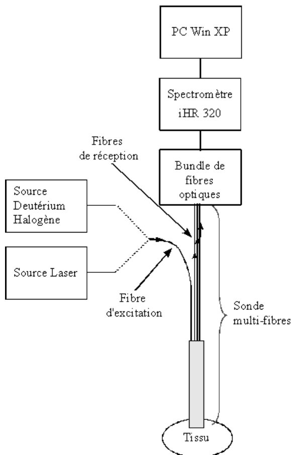
FIGURE 2.2 – Schéma de principe du système mis en œuvre pour l'expérimentation [Péry, 2007], système constitué de : deux sources de lumière (lampe Deutérium-Halogène et diode laser), une sonde multi-fibres optiques et un spectrographe.
