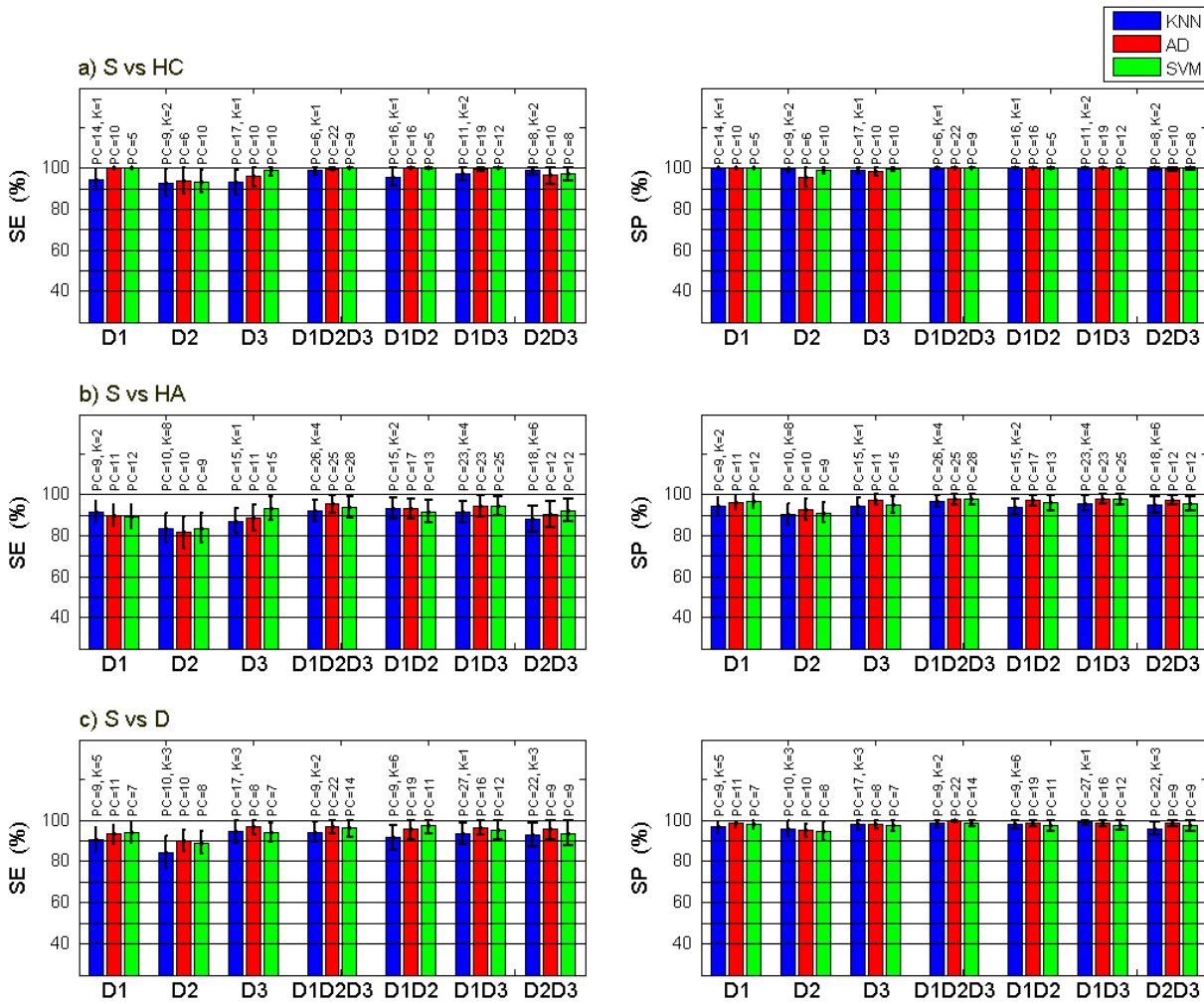
FIGURE 3.33 – Sensibilités (SE) et Spécificités (SP) en utilisant les caractéristiques qui discriminent exclusivement HA (Hyperplasie Atypique) vs D (Dysplasie) + moyennes calculées à partir d'un jeu de 13 caractéristiques spectrales (D1=6, D2=2 et D3=5) capables de discriminer les 6 paires de classes histologiques : a) S (Sain) vs. HC (Hyperplasie Compensatoire), b) S vs. HA (Hyperplasie Atypique), c) S vs. D (Dysplasie), HC vs. HA, HC vs. D et HA vs. D. Sur chaque histogramme, les résultats sont donnés pour toutes les combinaisons possibles des 3 distances inter-fibres (D1=271 \mu\text{m} , D2 = 536 \mu\text{m} et D3 = 834 \mu\text{m} ) et pour chacune des trois méthodes de classification. PC et K indiqués sur chaque histogramme correspondent aux nombres des composantes principales (PC) et de plus proches voisins (k) permettant d'obtenir les résultats optimaux montrés ici. Les barres d'erreur représentent les écart-types obtenus pour les moyennes de Se et Sp calculées sur 100 valeurs (itérations).
