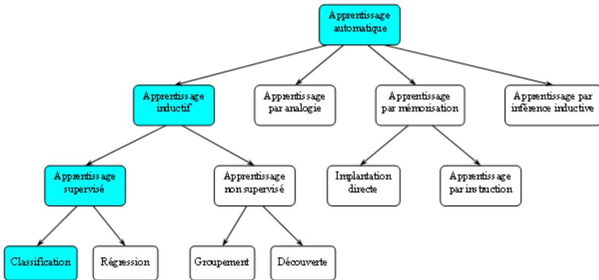
FIGURE 3.16 – Organisation hiérarchique des techniques d'Apprentissage Automatique, [Lorenzo-Navarro, 2001].
