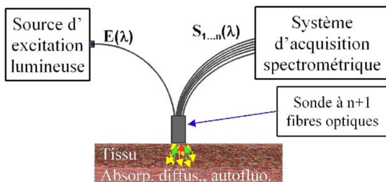
FIGURE 1.6 – Schéma de principe de base pour la spectroscopie tissulaire résolue spatialement (1 fibre d'excitation, n fibres d'acquisition).
