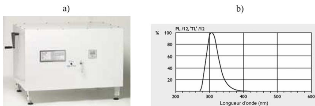
FIGURE 2.19 – Photographie de l'appareil d'irradiation ultraviolette (Research Irradiation Unit, Daavlin, Belgique), b) Spectre d'émission des tubes TL/12 Philips en place.
