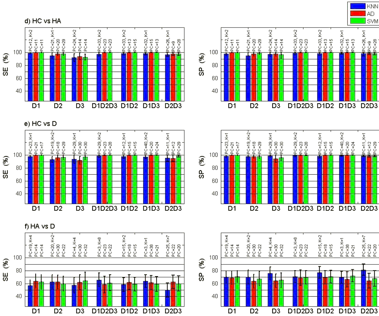
FIGURE 3.32 – Sensibilités (SE) et Spécificités (SP), moyennes calculées à partir d'un jeu de 306 caractéristiques spectrales (D1=83, D2=98 et D3=125) capables de discriminer au moins 4 des 6 paires de classes histologiques : S (Sain) vs. HC (Hyperplasie Compensatoire), S vs. HA (Hyperplasie Atypique), S vs. D (Dysplasie), d) HC vs. HA, e) HC vs. D et f) HA vs. D. Sur chaque histogramme, les résultats sont donnés pour toutes les combinaisons possibles des 3 distances inter-fibres (D1=271 \mu\text{m} , D2 = 536 \mu\text{m} et D3 = 834 \mu\text{m} ) et pour chacune des trois méthodes de classification. PC et K indiqués sur chaque histogramme correspondent aux nombres des composants principaux (PC) et de plus proches voisins (k) permettant d'obtenir les résultats optimaux montrés ici. Les barres d'erreur représentent les écart-types obtenus pour les moyennes de Se et Sp calculées sur 100 valeurs (itérations).
