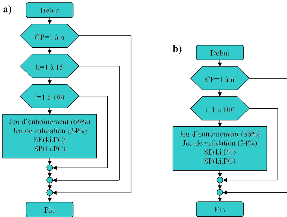
FIGURE 3.23 – Algorithmes de classification développés. a) pour l’algorithme k-NN et b) pour les algorithmes LDA et SVM.
