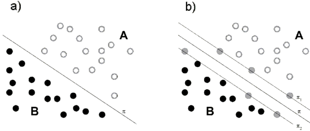
FIGURE 3.21 – a) Ensemble de points séparables et hyperplan dans l'espace dimensionnel \mathbb{R}^2 , les points vides représentent les données avec l'étiquette y = 1 et les points noirs les données avec l'étiquette y = -1 ; b) hyperplans parallèles \pi , \pi_1 et \pi_2 et les vecteurs de support possibles sont indiqués en gris. La marge est la distance entre les hyperplans \pi et \pi_1 (ou \pi_2 ).
