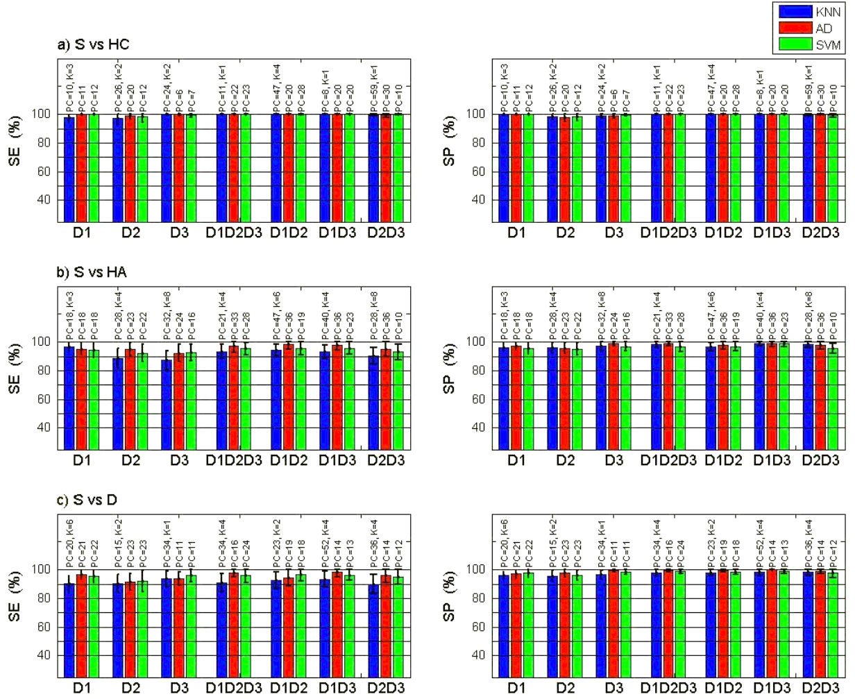
FIGURE 3.31 – Sensibilités (SE) et Spécificités (SP), moyennes calculées à partir d'un jeu de 306 caractéristiques spectrales (D1=83, D2=98 et D3=125) capables de discriminer au moins 4 des 6 paires de classes histologiques : a) S (Sain) vs. HC (Hyperplasie Compensatoire), b) S vs. HA (Hyperplasie Atypique), c) S vs. D (Dysplasie), HC vs. HA, HC vs. D et HA vs. D. Sur chaque histogramme, les résultats sont donnés pour toutes les combinaisons possibles des 3 distances inter-fibres (D1=271 \mu\text{m} , D2 = 536 \mu\text{m} et D3 = 834 \mu\text{m} ) et pour chacune des trois méthodes de classification. PC et K indiqués sur chaque histogramme correspondent aux nombres des composants principaux (PC) et de plus proches voisins (k) permettant d'obtenir les résultats optimaux montrés ici. Les barres d'erreur représentent les écart-types obtenus pour les moyennes de Se et Sp calculées sur 100 valeurs (itérations).
