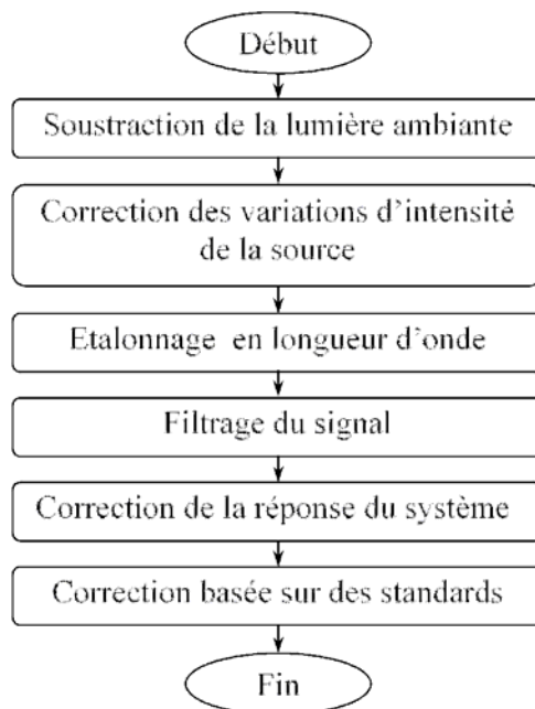
FIGURE 3.1 – Organigramme du prétraitement des données en spectroscopie de fluorescence proposé par [Marín et al. , 2006].
