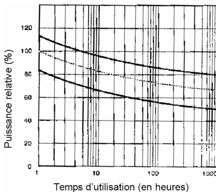
FIGURE 2.17 – Courbes typiques moyenne (trait pointillé), minimale et maximale (traits pleins) de variation de la puissance relative au cours du temps d'utilisation de la lampe Xénon 300 W ( http://www.eurosep.com ).
