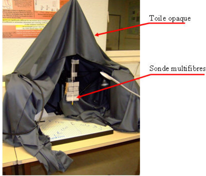
FIGURE 3.5 – Cache mis en place pour couvrir et isoler le site de mesure de toute source ou perturbation lumineuse ambiante.
