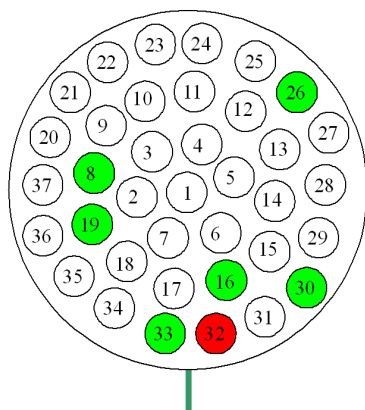
FIGURE 2.21 – Configuration géométrique de l'extrémité distale de la sonde multi-fibres. Pour notre étude in vivo la fibre 32 a servi pour l'excitation et les fibres 8, 16, 19, 26, 30 et 33 pour la réception.
