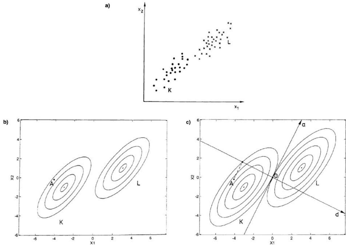
FIGURE 3.19 – Approche géométrique de la méthode ADL. a) Les deux classes K et L à discriminer ; b) limites de confiance autour des centroïdes des classes K et L ; c) représentation des limites de confiance, O est le point d'intersection de ces iso-probabilités, la droite ( a ) est la tangente aux deux ellipses et ( d ) la direction de discrimination optimale, A un individu.
