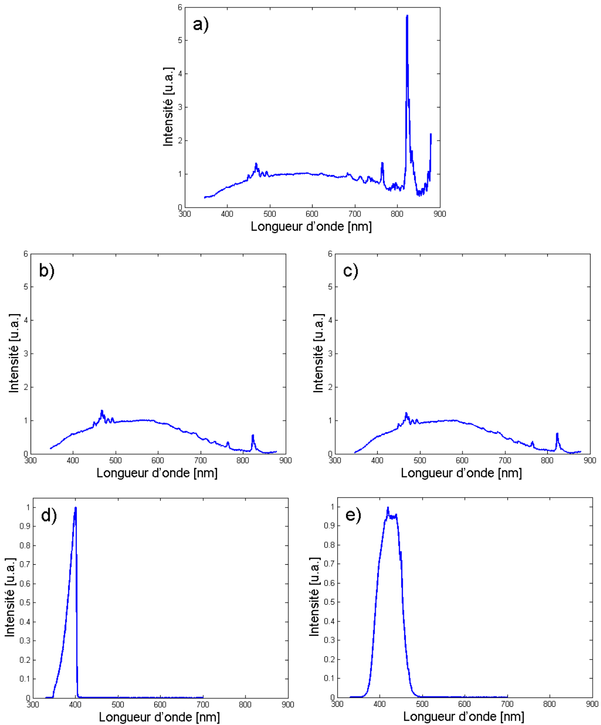
FIGURE 2.10 – Spectres mesurés à la sortie de chaque élément du système d'excitation ; a) en sortie de la lampe ; b) derrière le filtre anticalorique KG1 ; c) derrière la lentille de focalisation ; d) derrière le filtre passe-bande utilisé pour les excitations en AF à 360 et 368 nm ; e) derrière le filtre passe-bande utilisé pour les excitations en AF à 390, 400, 410, 420 et 430 nm.
