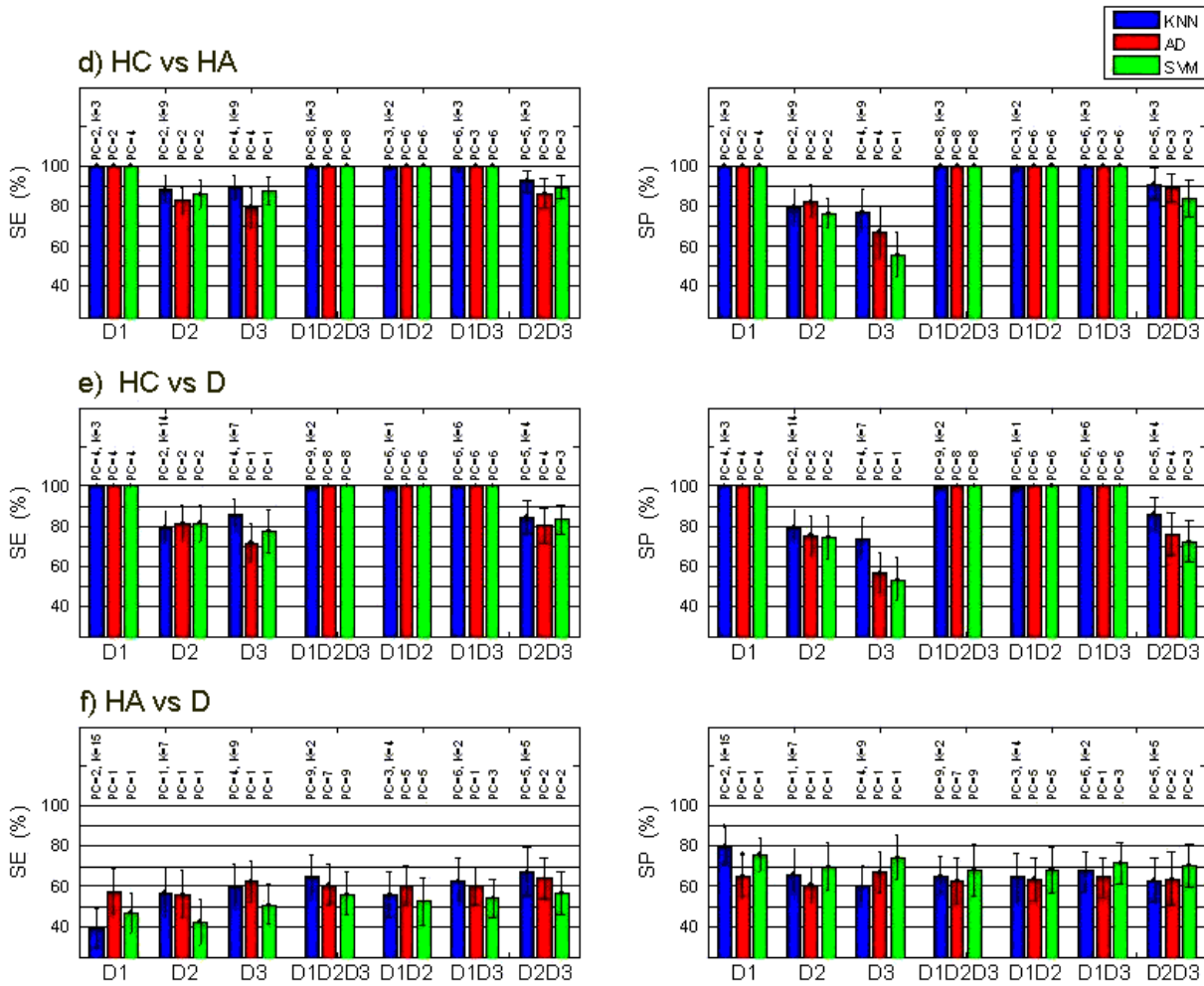
FIGURE 3.28 – Sensibilités (SE) et Spécificités (SP), moyennes calculées à partir d'un jeu de 13 caractéristiques spectrales (D1=6, D2=2 et D3=5) capables de discriminer les 6 paires de classes histologiques : S (Sain) vs. HC (Hyperplasie Compensatoire), S vs. HA (Hyperplasie Atypique), S vs. D (Dysplasie), d) HC vs. HA, e) HC vs. D et f) HA vs. D. Sur chaque histogramme, les résultats sont donnés pour toutes les combinaisons possibles des 3 distances inter-fibres (D1=271 \mu\text{m} , D2 = 536 \mu\text{m} et D3 = 834 \mu\text{m} ) et pour chacune des trois méthodes de classification. PC et K indiqués sur chaque histogramme correspondent aux nombres de composantes principales (PC) et de plus proches voisins (k) permettant d'obtenir les résultats optimaux montrés ici. Les barres d'erreur représentent les écart-types obtenus pour les moyennes de Se et Sp calculées sur 100 valeurs (itérations).
