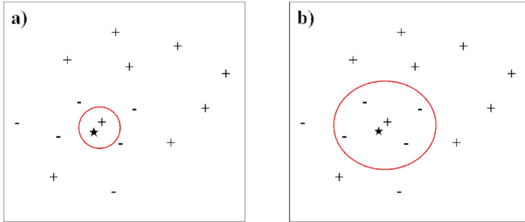
FIGURE 3.18 – Exemples de la classification k-NN. a) k=1 ; b) k=5
