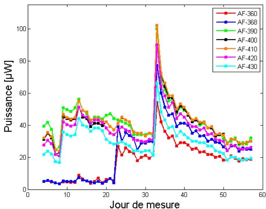
FIGURE 2.18 – Courbes des mesures quotidiennes de puissance d'excitations d'AF au cours du protocole expérimentale in vivo mené au laboratoire de avril 2007 à octobre 2007.
