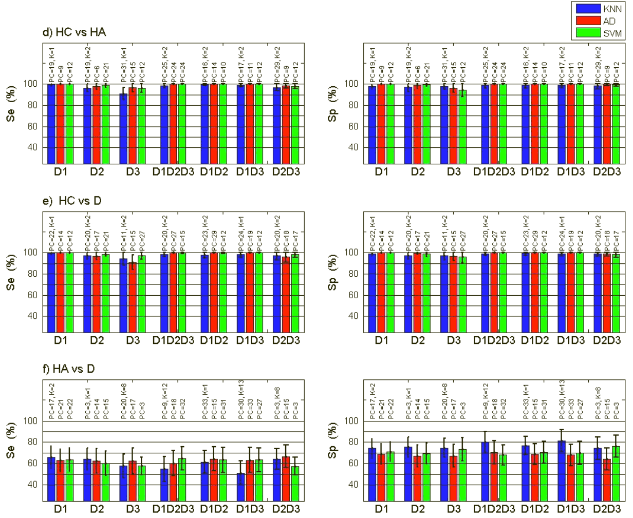
FIGURE 3.36 – Sensibilité (SE) et Spécificité (SP) en utilisant les caractéristiques qui discriminent exclusivement HA (Hyperplasie Atypique) vs D (Dysplasie) + moyennes calculées à partir d'un jeu de 186 caractéristiques spectrales (D1=44, D2=59 et D3=83) capables de discriminer au moins 5 des 6 paires de classes histologiques : S (Sain) vs. HC (Hyperplasie Compensatoire), S vs. HA (Hyperplasie Atypique), S vs. D (Dysplasie), d) HC vs. HA, e) HC vs. D et f) HA vs. D. Pour chaque histogramme, les résultats sont donnés pour toutes les combinaisons possibles des 3 distances inter-fibres (D1=271 \mu\text{m} , D2 = 536 \mu\text{m} et D3 = 834 \mu\text{m} ) et pour chacune des trois méthodes de classification. PC et K indiqués sur chaque histogramme correspondent aux nombres de composantes principales (PC) et de plus proches voisins (k) permettant d'obtenir les résultats optimaux montrés ici. Les barres d'erreur représentent les écart-types obtenus pour les moyennes de Se et Sp calculées sur 100 valeurs (itération).
