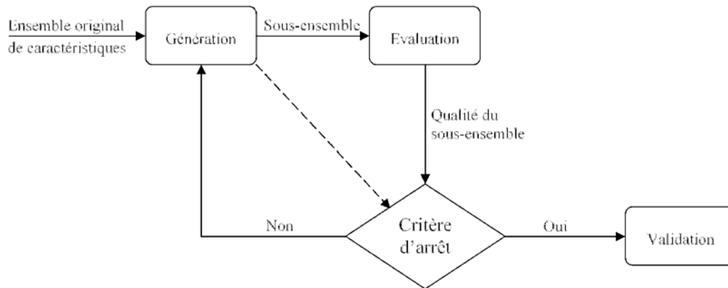
FIGURE 3.3 – Organigramme d'un processus de sélection de caractéristiques selon [Dash and Liu, 1997].
