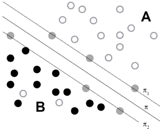
FIGURE 3.22 – Exemple des hyperplans séparateurs pour le cas de données non linéairement séparables.
