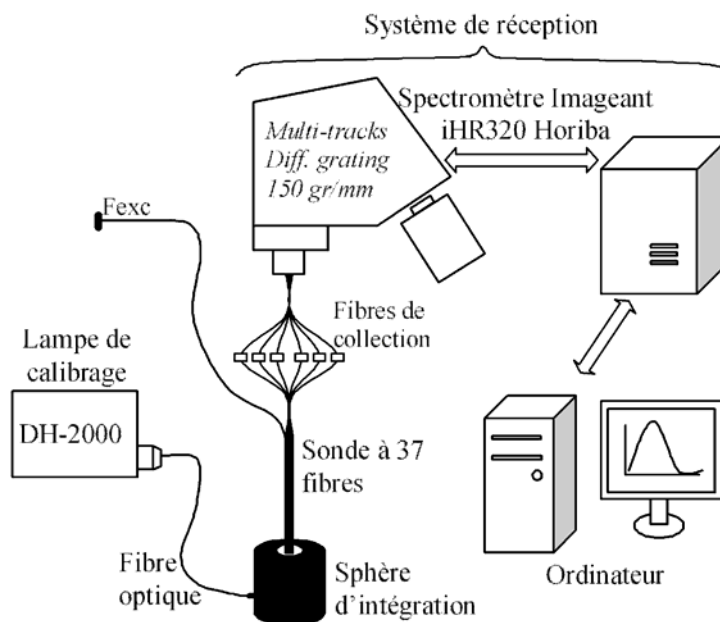
FIGURE 2.13 – Schéma de la configuration expérimentale mise en œuvre pour réaliser les mesures de calibration de la réponse spectrale du système d'acquisition.
