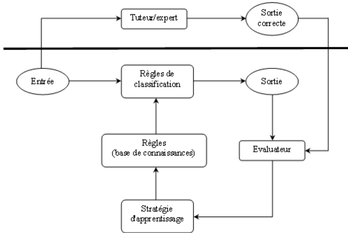
FIGURE 3.17 – Schéma de l'apprentissage supervisé [Forsyth, 1989][Lorenzo-Navarro, 2001].
