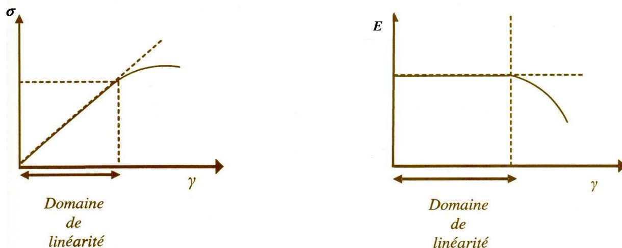
Figures 2.25. Le domaine de linéarité mis en évidence lors d'un balayage en déformation.
