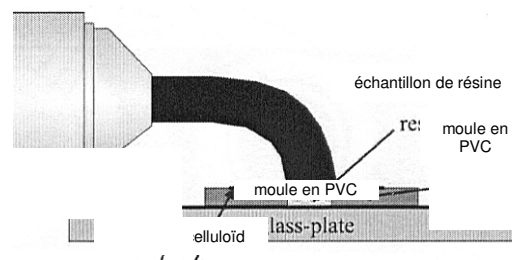
Figure 2.23. Système de fabrication des échantillons pour les essais en DMTA.
