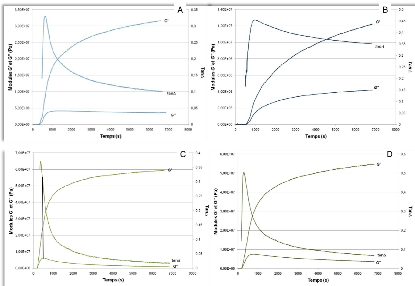
Figures 4.4. Courbes représentatives de l'évolution de G' , G'' et tangente \delta au cours de la réticulation des différents mélanges de comonomères : B-T 50/50 (A), B-T 70/30 (B), U-T 66/33 (C) et U-T 88/11 (D).
