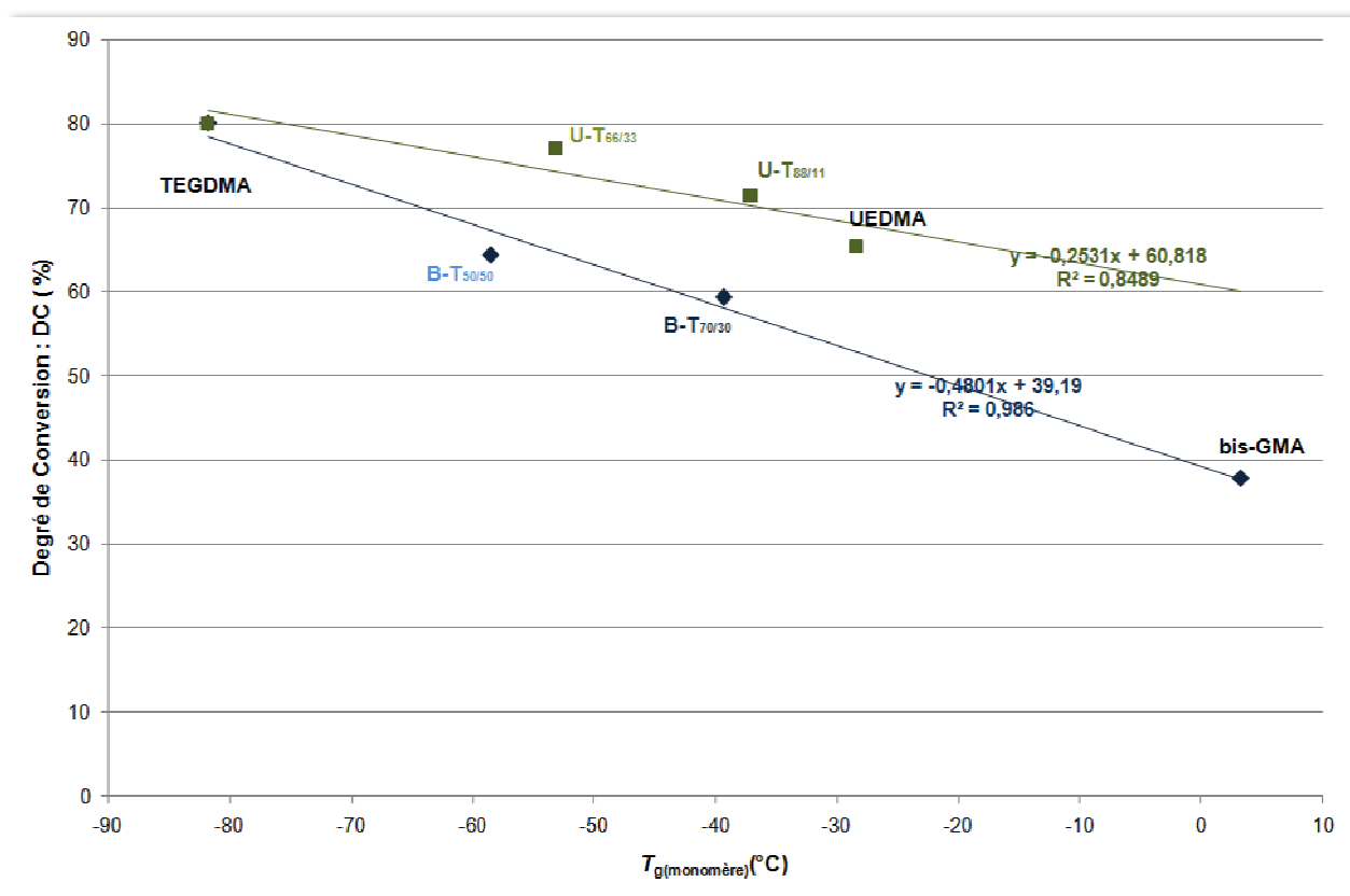
Figure 3.9. Variation du degré de conversion ( DC : %) des matrices obtenues par IRTF en fonction de la T_{g(\text{monomère})} (°C) des monomères et des mélanges de comonomères correspondants
