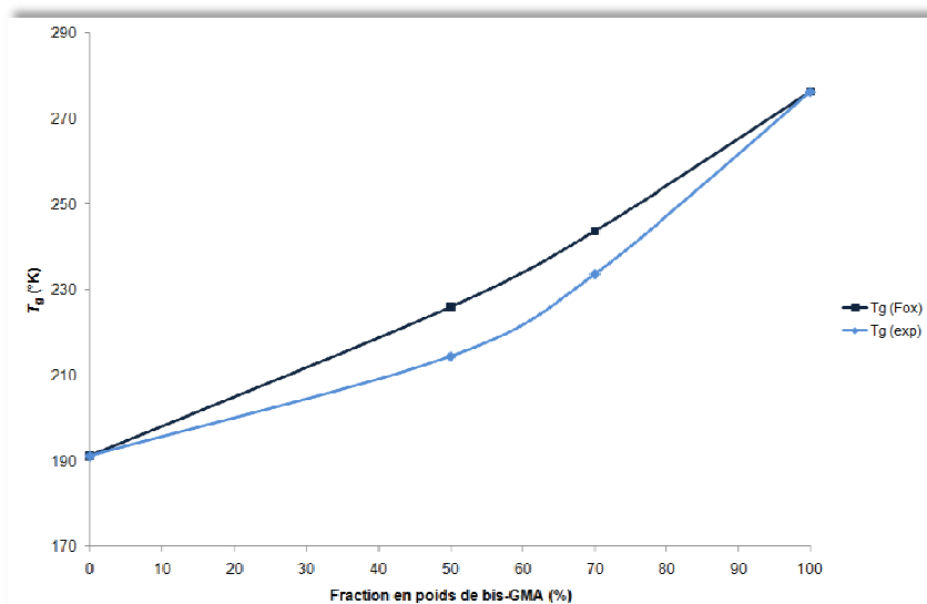
Figure 3.7.a. Variation des T_{g(\text{Fox})} et T_{g(\text{exp})} des mélanges à base de Bis-GMA en fonction de la fraction massique de Bis-GMA
