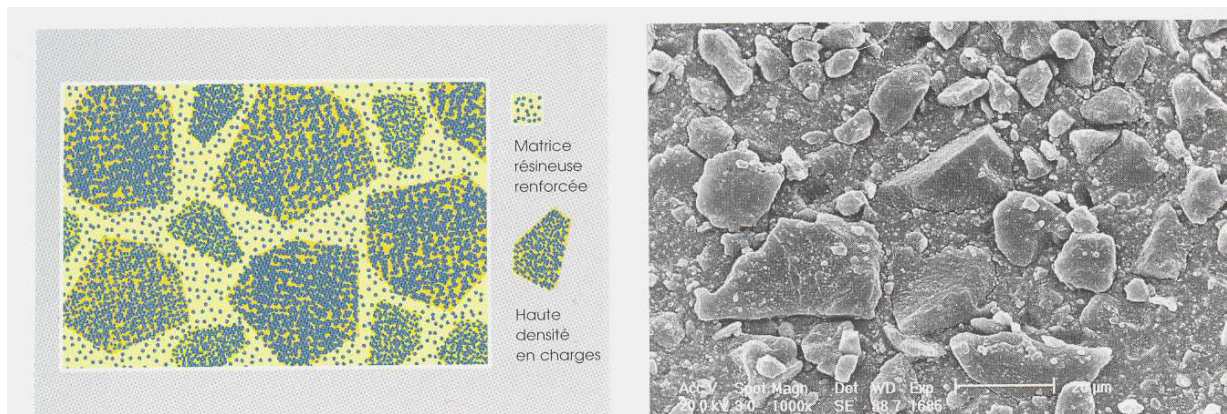
Figure 1.7.a. Schéma de la structure d'un composite microchargé hétérogène. Les complexes prépolymérisés, présentant une haute densité en charges, sont noyés dans une matrice renforcée, d'après Dietschi D. et Spreafico R. [18].
