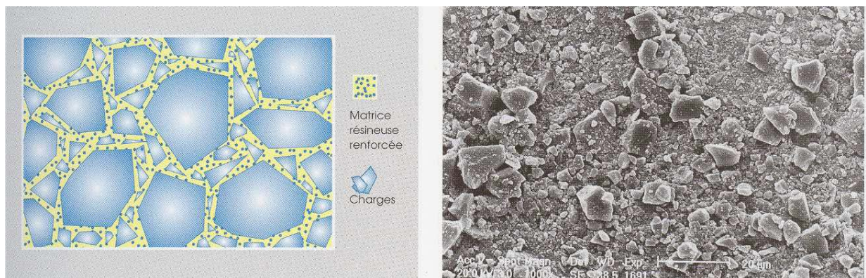
Figure 1.8.a. Schéma de la structure d'un composite hybride. Les particules, obtenues par concassage ( > 1 \mu\text{m} ), sont incluses dans une matrice renforcée par des microparticules, d'après Dietschi D. et Spreafico R. [18].
