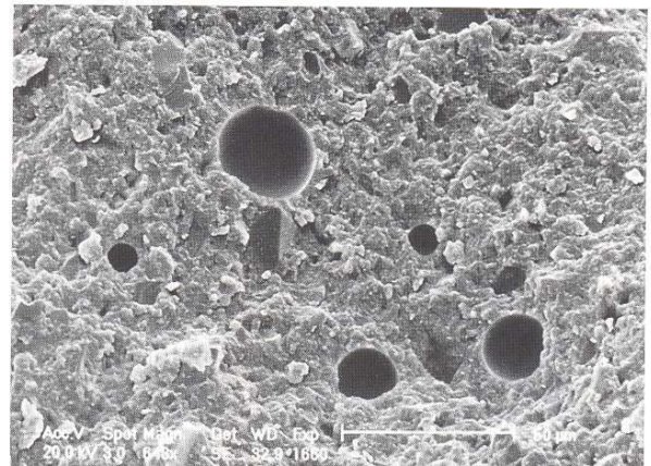
Figure 1.3.b. Cliché MEB d'un échantillon de composite chimopolymérisable : présence de porosités liées au malaxage, d'après Dietschi D. et Spreafico R. [18].
