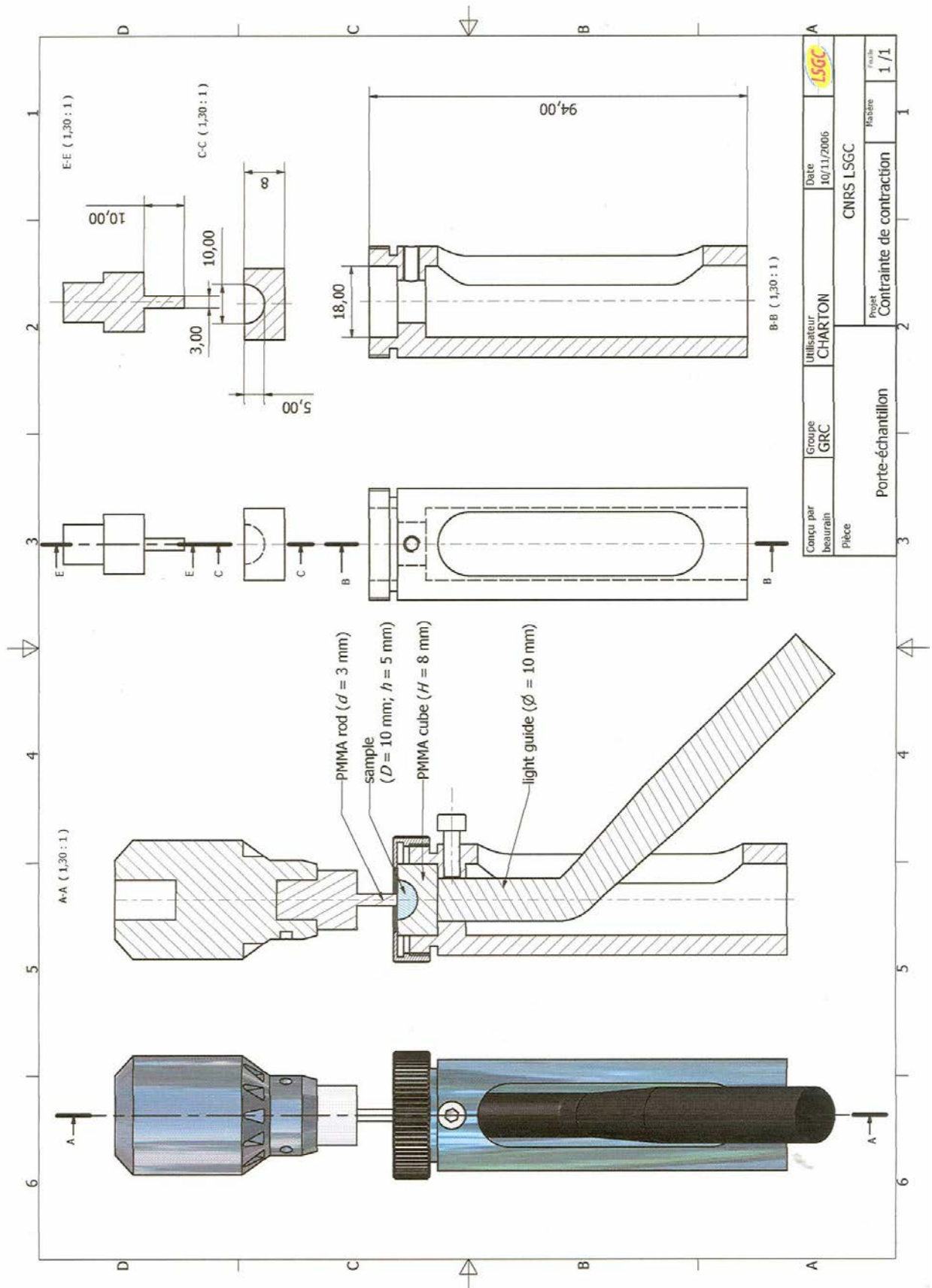
Figure 2.14. Gros plan du porte-échantillon, de la sonde d'enregistrement et du canon à photons de l'unité de photopolymérisation Demetron Optilux 501® (Kerr-Hawe). Facteur C : 2,3.
