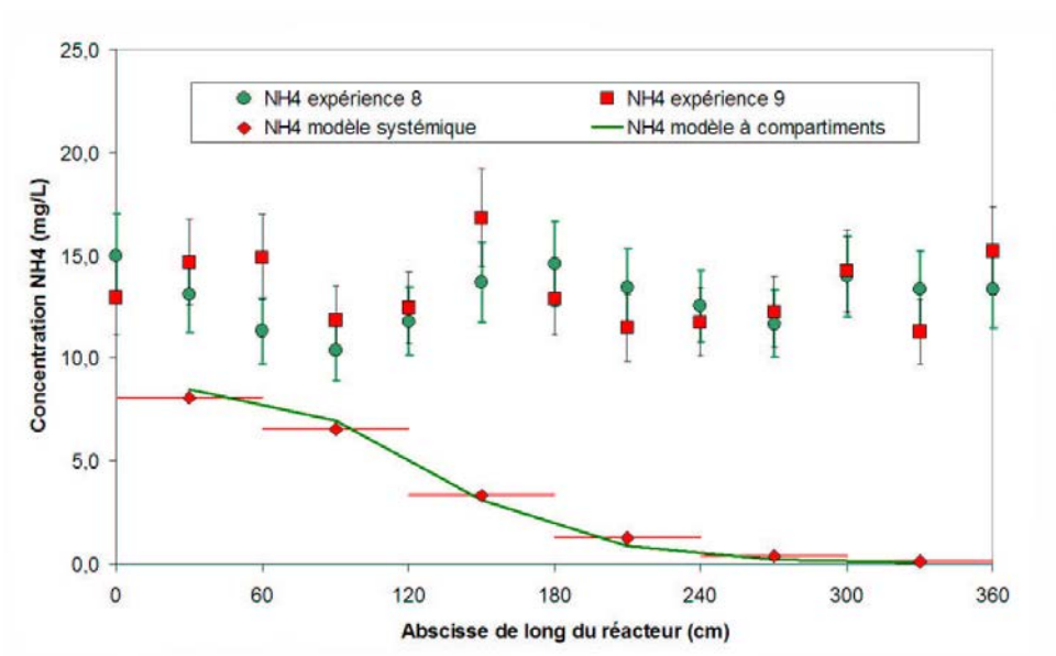
FIG. 5.22 – Comparaison de l'évolution de la concentration en ammonium pour les expériences 8 à 9
