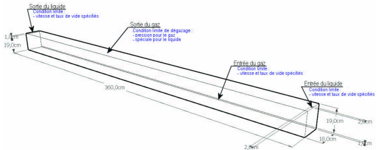
FIG. B.4 – Schéma coté du réacteur avec les conditions aux limites
