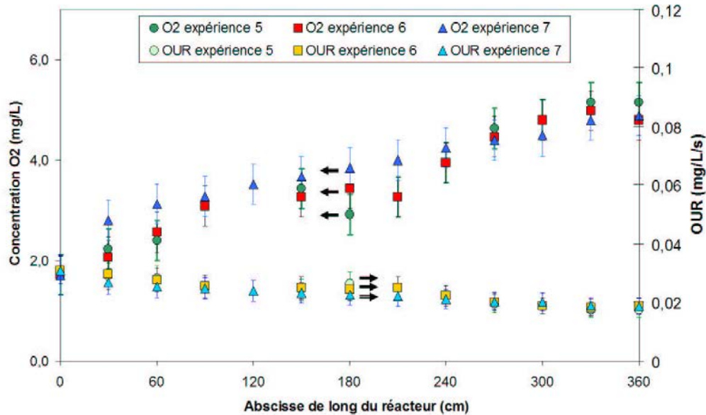
FIG. 2.17 – Evolution de l’oxygène dissous et du OUR le long du réacteur pour les expériences 5 à 7
