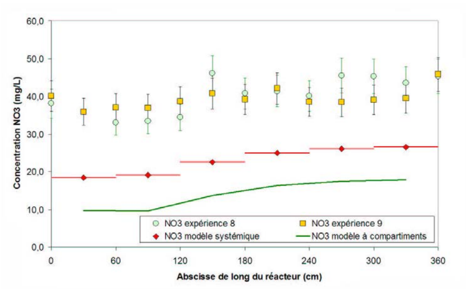
FIG. 5.21 – Comparaison de l'évolution de la concentration en nitrates pour les expériences 8 à 9
