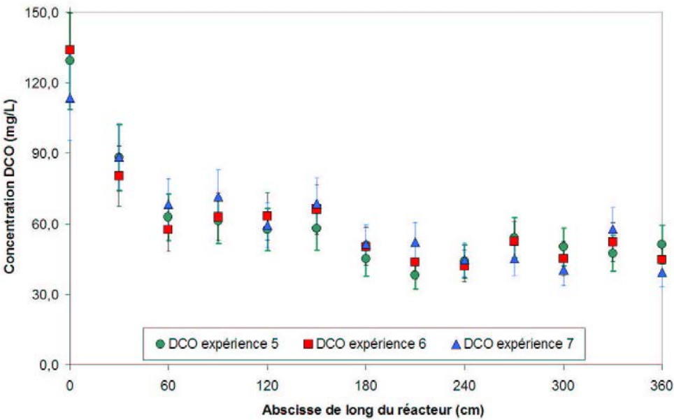
FIG. 2.16 – Evolution de la DCO le long du réacteur pour les expériences 5 à 7
