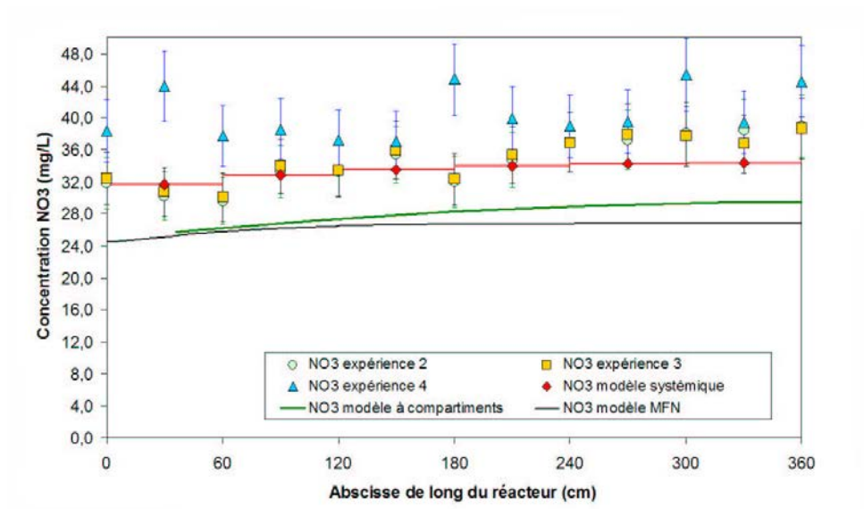
FIG. 5.13 – Comparaison de l'évolution de la concentration en nitrates pour les expériences 2 à 4
