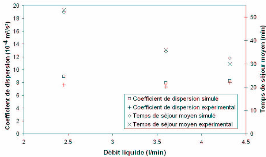
FIG. 1.18 – DTS expérimentales et simulées, avec le modèle RSM, pour différents débit de liquide et un débit de gaz égal à 65 \text{ L.min}^{-1}
