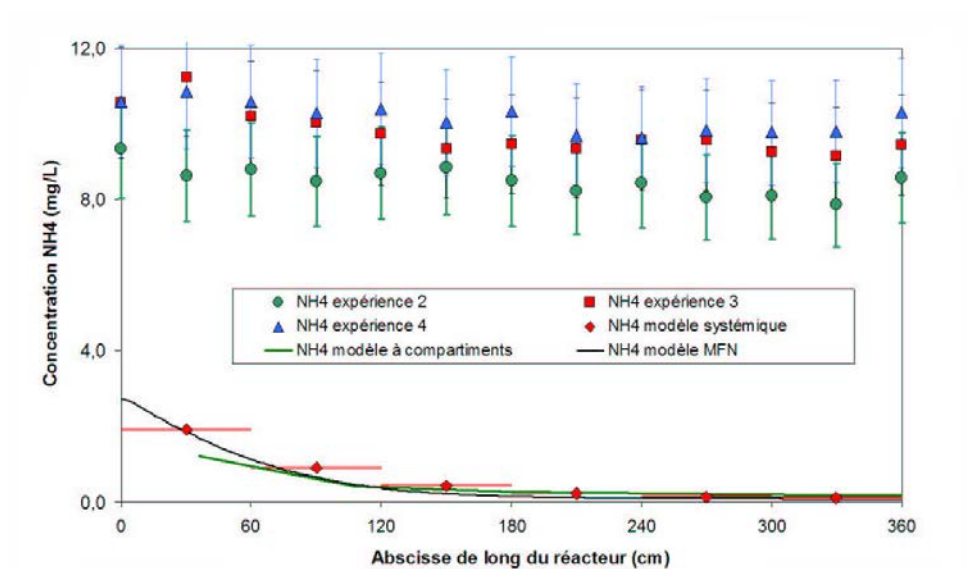
FIG. 5.14 – Comparaison de l'évolution de la concentration en ammonium pour les expériences 2 à 4
