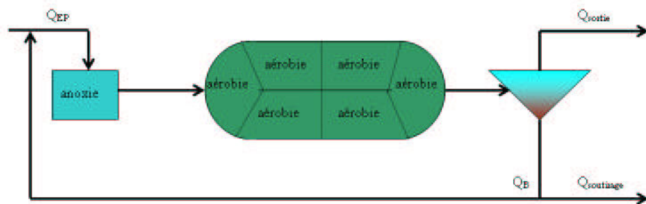
FIG. C.4 – Carrousel avec un bassin d’anoxie en tête
