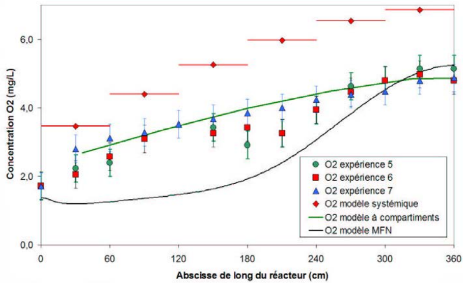
FIG. 5.16 – Comparaison de l'évolution de l'oxygène dissous pour les expériences 5 à 7
