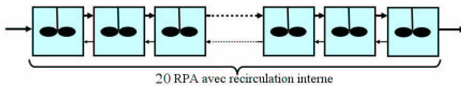
FIG. 4.5 – Schéma détaillant le modèle à compartiments obtenu par l'approche Guha et al. (2006)
