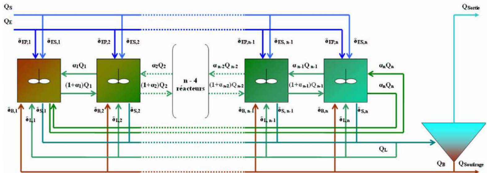
FIG. 3.4 – Structure du modèle systémique complet
