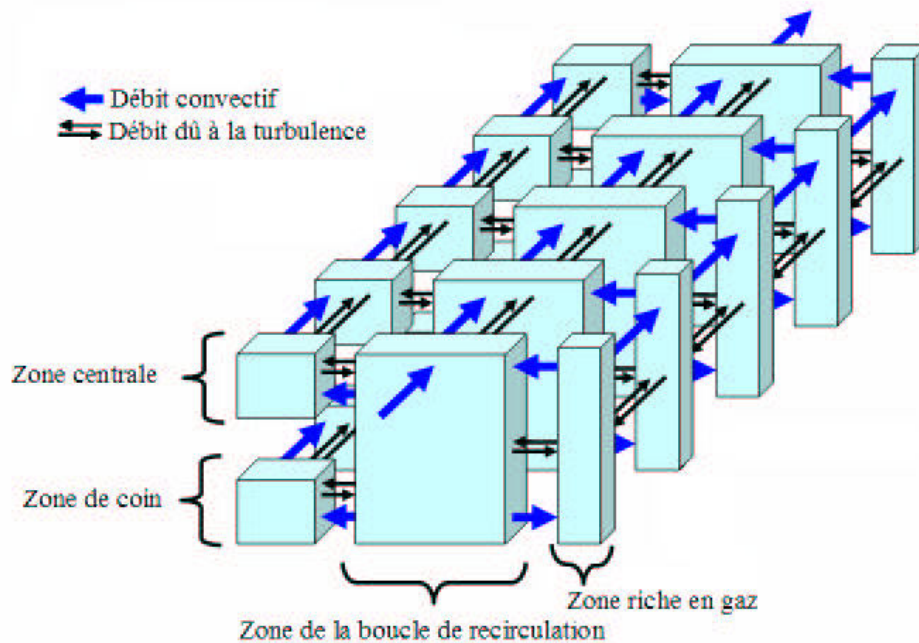
FIG. 4.11 – Schéma détaillant le modèle à compartiment obtenu par la nouvelle approche
