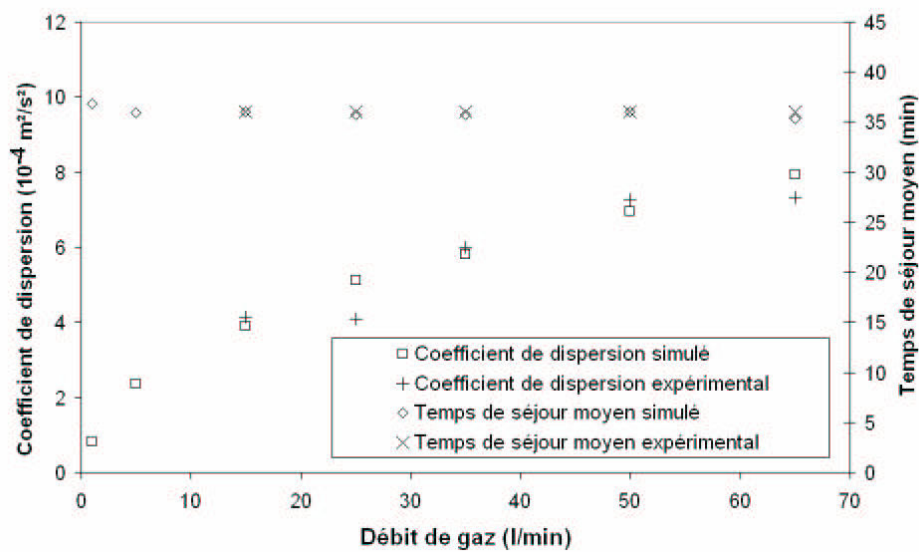
FIG. 1.17 – DTS expérimentales et simulées, avec le modèle RSM, pour différents débit de gaz et un débit liquide égal à 3,5 \text{ L.min}^{-1}
