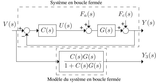
FIG. 2.2 – Générateur de résidus à partir du modèle du système en boucle fermée
