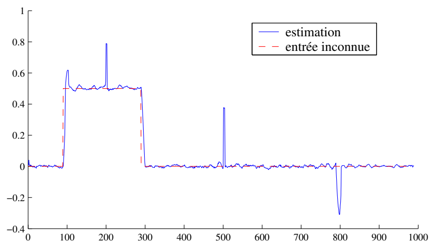
FIG. 4.12 – Estimation de l'entrée inconnue en présence de bruit
