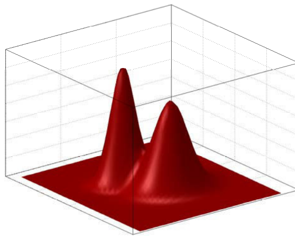
FIG. 3.4 – Densité mélange
