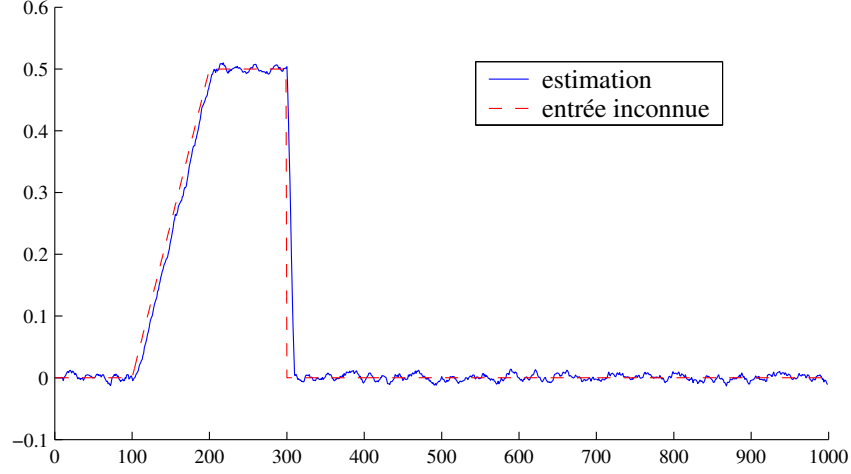
FIG. 4.3 – Entrée inconnue estimée en présence de bruit
