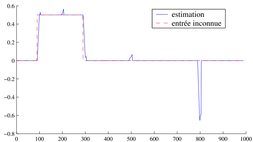
FIG. 4.11 – Estimation de l'entrée inconnue en l'absence de bruit
