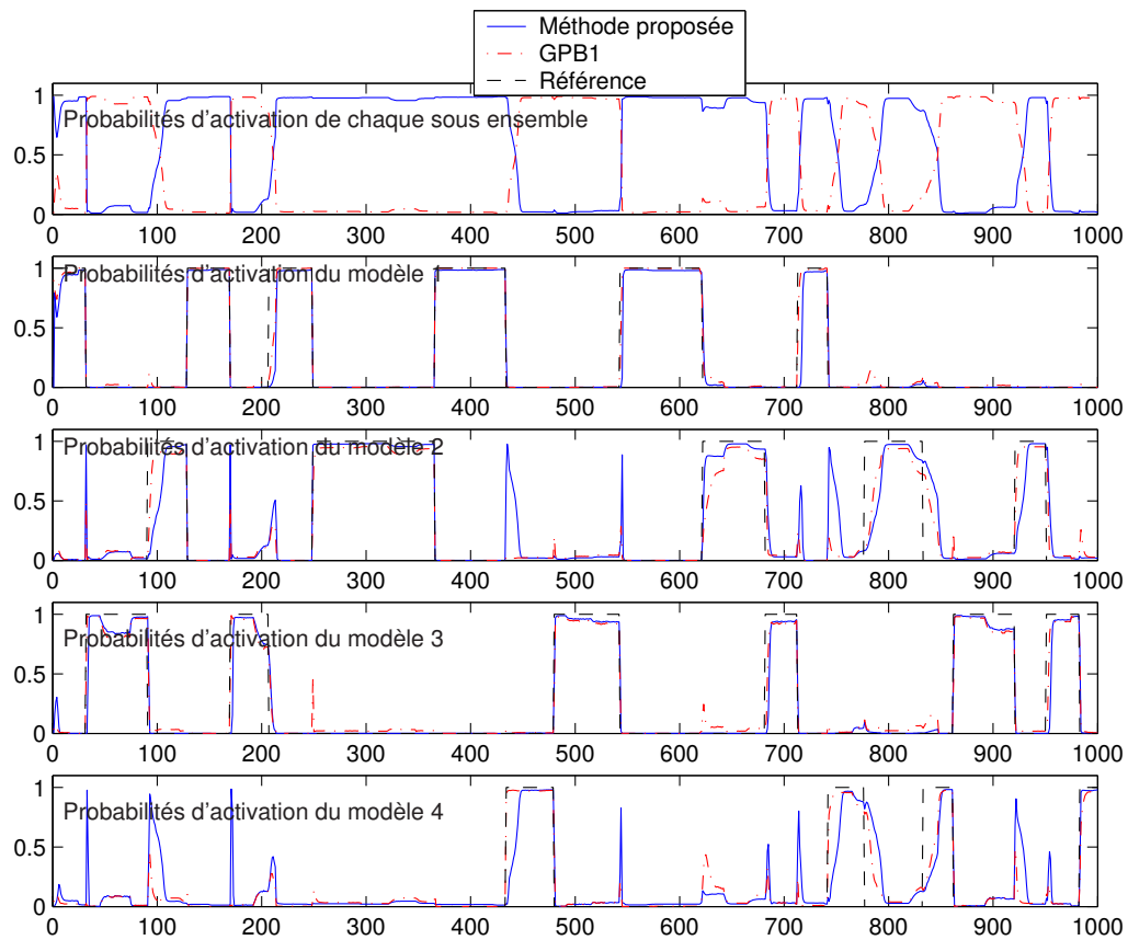
FIG. 6.4 – Probabilités d'activation (méthode directe)
