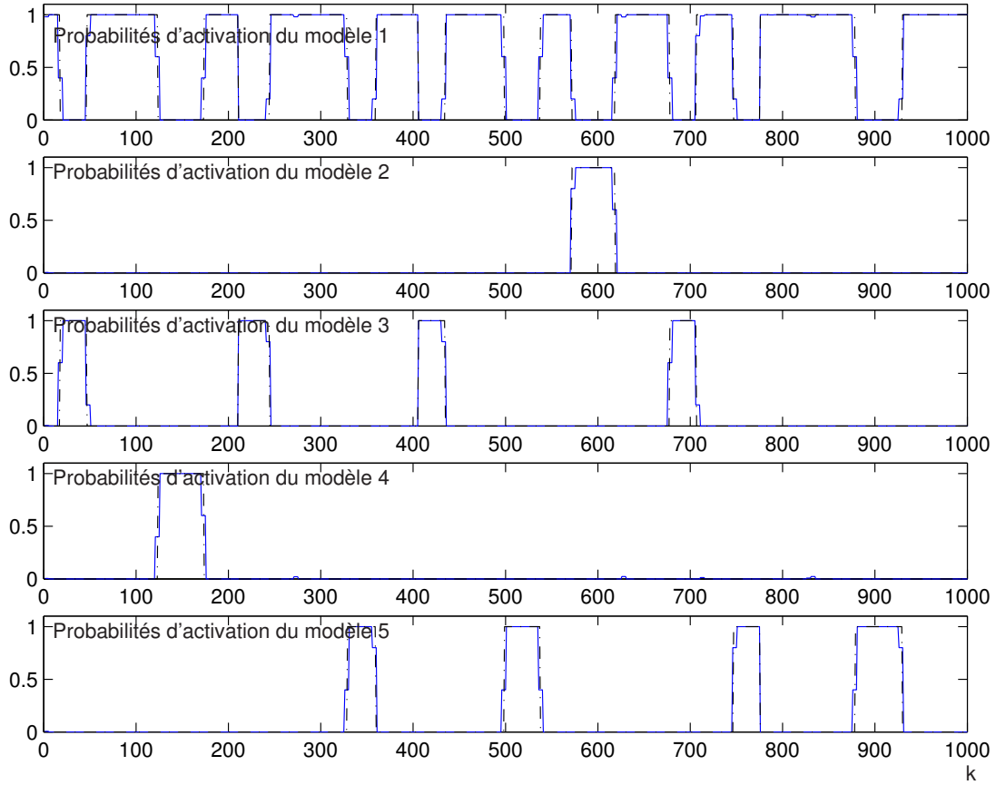
FIG. 2.6 – Probabilités d'activation \mu_i
