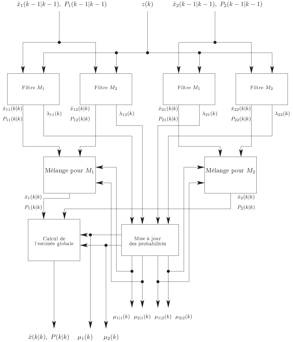
FIG. 1.5 – Estimateur GPB2
