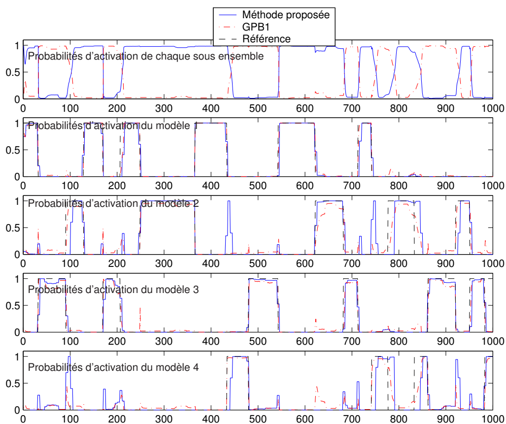
FIG. 6.5 – Probabilités d'activation (méthode hiérarchisée)
