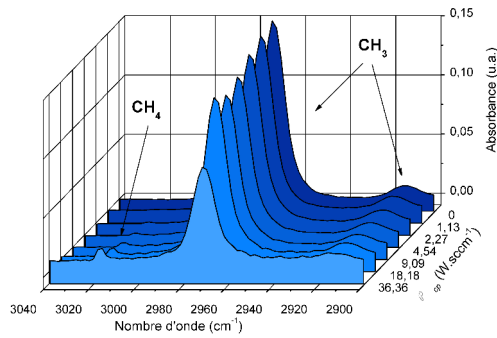
(a) Détail de la bande d'absorption 3040\text{--}2900\text{ cm}^{-1} dans le cas de l'hélium.
