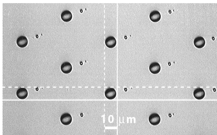
FIGURE 6.3 – Localisation au moyen d'un masque optique : obtention de gouttes de colle Vantico® de 10 μm de diamètre espacées de 40 μm. Crédit photographique : LETI/DOPT.
