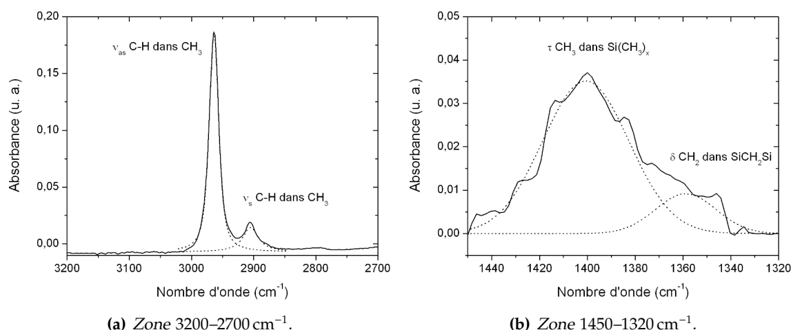
FIGURE 4.22 – Indexation et déconvolution des zones d'absorption infrarouge entre 3200 et 2700 cm -1 et entre 1450 et 1320 cm -1 pour un film mince réalisé à partir d'une décharge de précurseur pur. Conditions de dépôt au tableau 4.8 .
