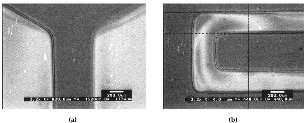
FIGURE 6.4 – Exemples de motifs obtenus par spin-coating de résine positive S1813RS15 grâce au traitement localisé par UVO du polydiméthylsiloxane plasma au travers d'un masque optique. Crédit photographique : LETI/DOPT.
