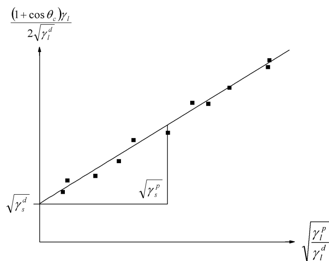
FIGURE 2.11 – Détermination graphique des composantes \gamma_s^d et \gamma_s^p de l'énergie de surface d'un solide à partir du modèle de D. K. Owens et R. C. Wenzel.
