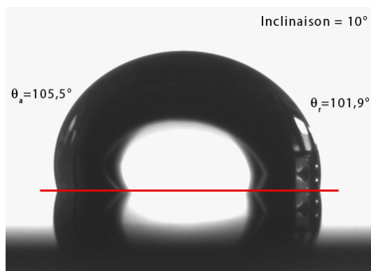
FIGURE 5.6 – Mise en évidence du phénomène d’ancrage de la ligne triple par la photographie d’une goutte d’eau de 10 µL sur une surface de polydiméthylcyclosiloxane plasma inclinée de 10°.
