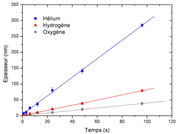
FIGURE 3.9 – Évolution de l'épaisseur du film mince en fonction du temps de traitement. Conditions de dépôt au tableau 3.3 .
