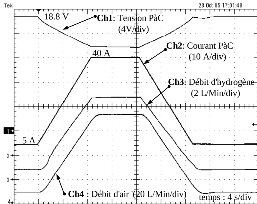
Figure 3.28 : Réponse en tension de la pile à une rampe de courant 5 A / 40 A [Tho05e]. Flux de gaz adaptés au courant débité, pente de courant : 4 \text{ A.s}^{-1} .
