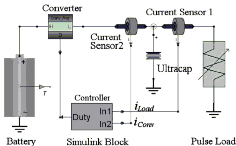
Figure 2.14 : Source hybride batteries-supercondensateurs de L. Gao et al. [Gao05].
