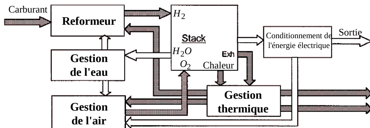
Figure 1.8 : Différents constituants d'un système pile à combustible [Ell01].
