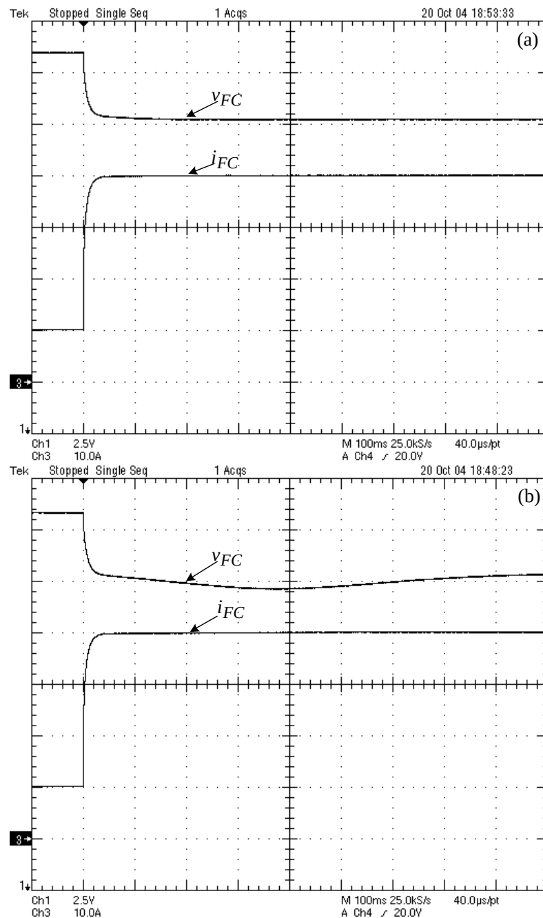
Figure 3.25 : Réponses en tension de la pile à un échelon de courant 10 A / 40 A. (a) : flux de gaz constants (réglés pour 50 A) , (b) : flux de gaz adaptés au courant débité.
