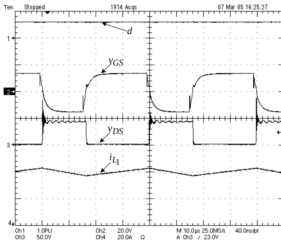
Figure 3.18 : Formes d'ondes associées au convertisseur de pile en régime stationnaire.
