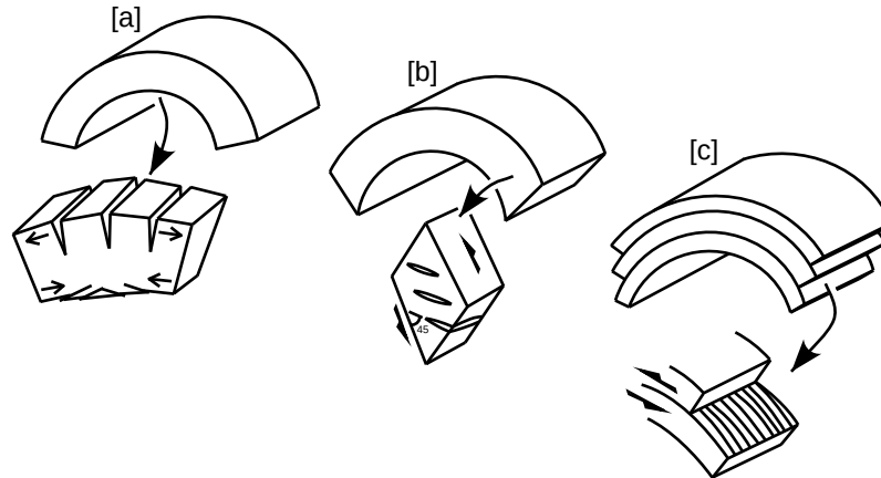
FIG. 1.3 – Les différents modes de déformation par flexion : [a] flexion [b] flexion-écoulement [c] flexion-glissement. Les flèches indiquent le déplacement relatif des particules du domaine (modifié d’après Gidon [1987])
