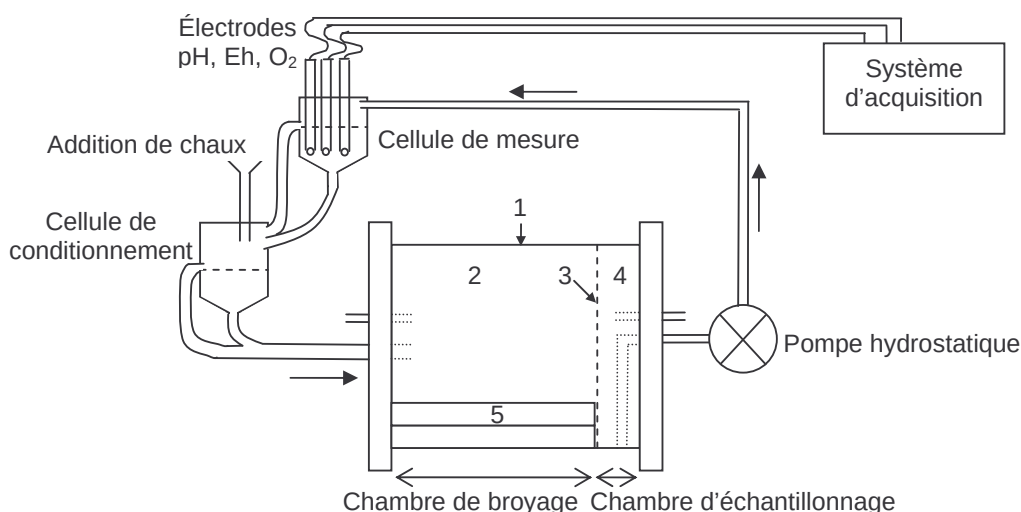
Figure 6.2 : Schéma du broyeur instrumenté de laboratoire utilisé dans la présente étude
