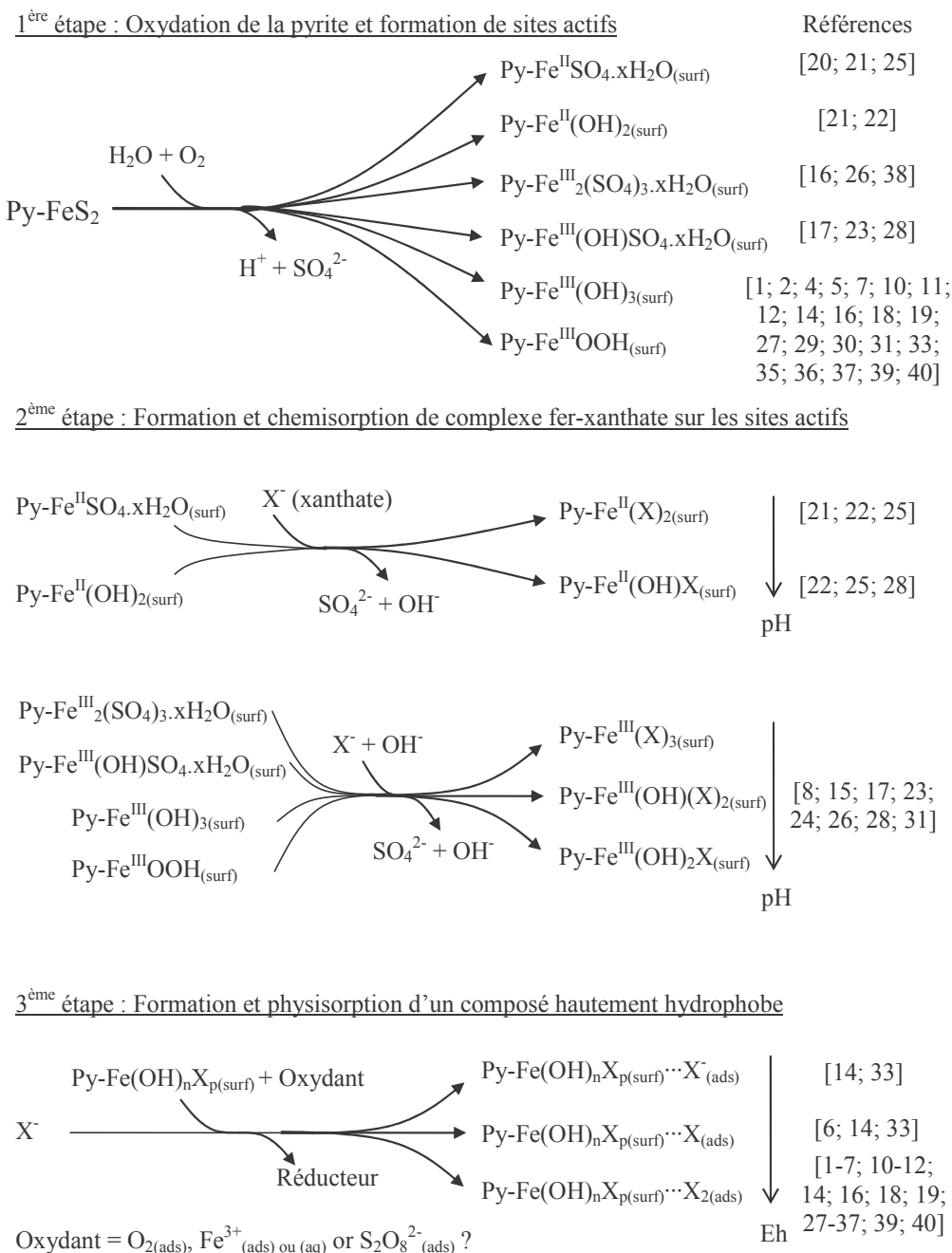
Figure 4.1 : Schéma synthétique des mécanismes d'interaction xanthate-pyrite
