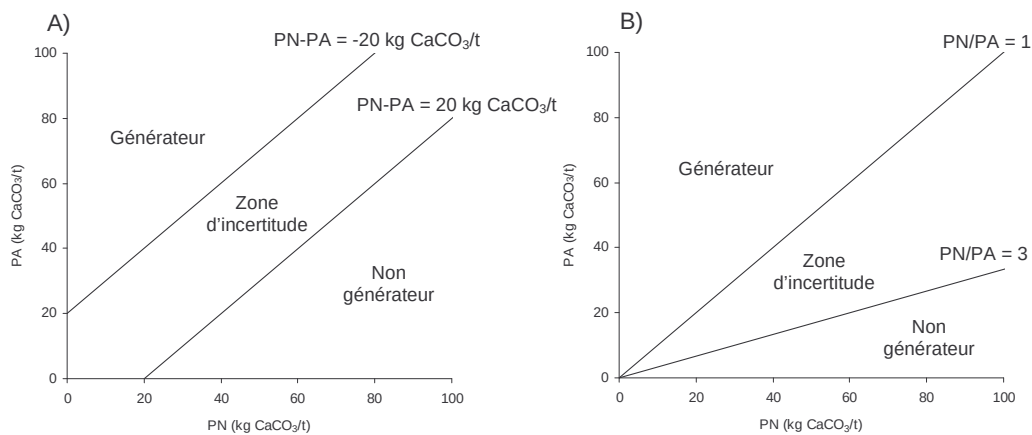
Figure 1.3 : Schémas illustrant les deux critères de classification environnementale de rejets miniers en matière de génération d'acide
