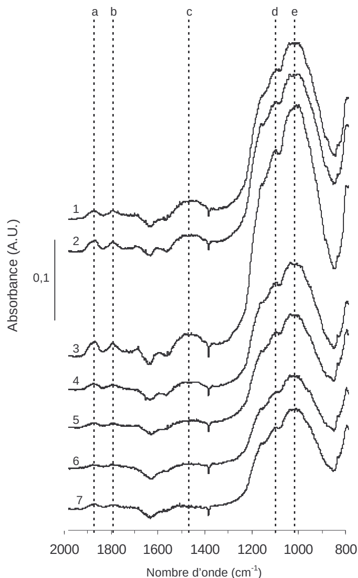
Figure 6.17 : Spectres obtenus par spectroscopie infrarouge en mode réflexion diffuse des concentrés C1 à différents pH de désulfuration, 100g/t de concentration initiale en xanthate
