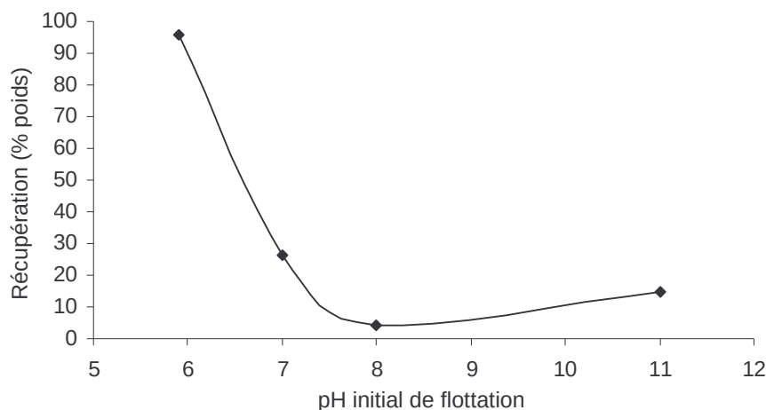
Figure 5.1 : Récupération de pyrite en fonction du pH d'activation à 5 \times 10^{-4} \text{ mol/L} de concentration initiale en xanthate, dépression initiale à pH 11 avec CaO, pH ajusté avec acide sulfurique, sans aération
