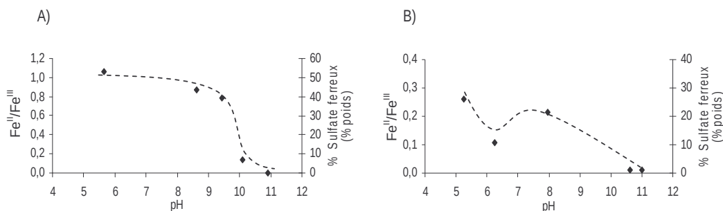
Figure 3.6 : Variation du rapport Fe II /Fe III des sulfates superficiels d'une pyrite conditionnée à différents pH avec du NaOH en solution
