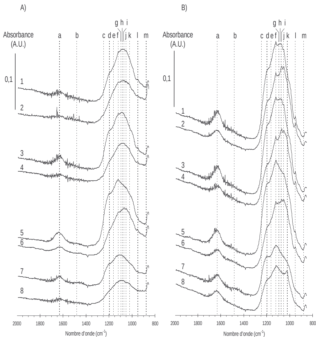
Figure 3.1 : Spectres obtenus par spectroscopie infrarouge en mode réflexion diffuse des deux fractions granulométriques de pyrite
