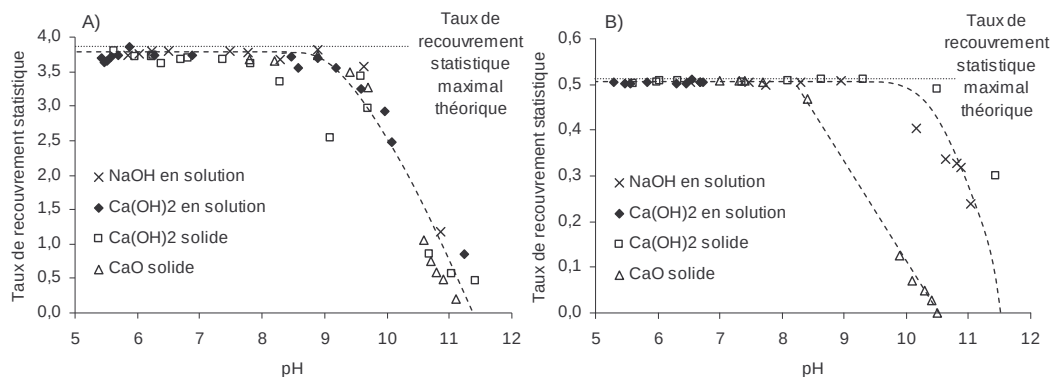
Figure 4.5 : Taux de recouvrement statistique en fonction du pH d'activation pour les deux fractions granulométriques de pyrite (A) 32-63 \mu\text{m} et (B) 0-150 \mu\text{m} , déprimées avec différents types de régulateur de pH, puis activées par ajout d'acide sulfurique pour atteindre un pH cible et finalement conditionnées avec 2 \times 10^{-4} mol/L d'isoamylxanthate de potassium. Les courbes tiretées des graphiques indiquent les tendances issues des données. La droite pointillée indique la valeur du taux de recouvrement statistique maximal théorique selon la concentration en xanthate utilisée
