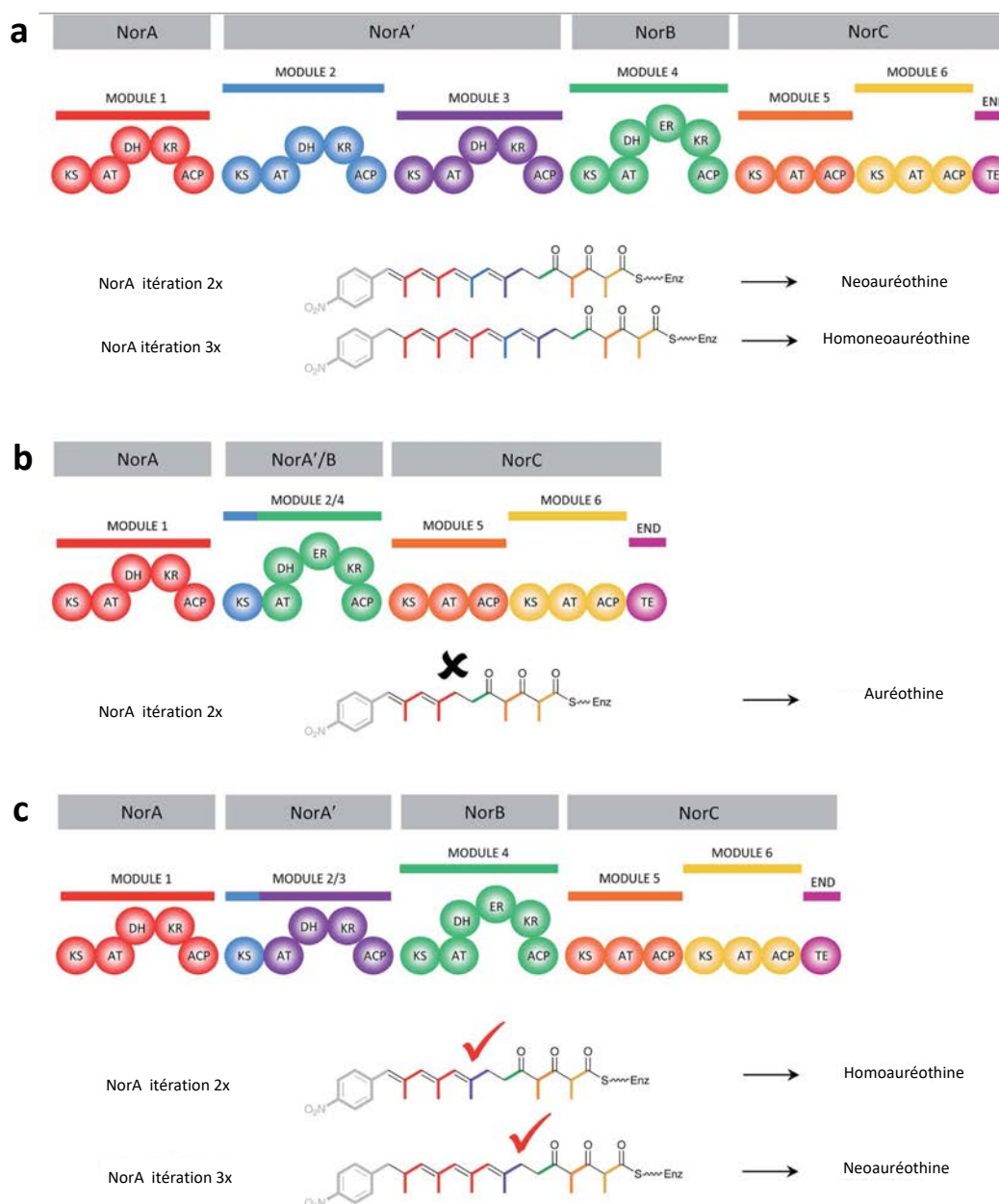
Figure 23 : Suppression de modules au sein de la neoaureothine synthase (adaptée de Weissman, 2016). a : La PKS native synthétise la neoaureothine grâce à deux itérations du premier module NorA. Si trois itérations ont lieu, alors l'homoneoaureothine est synthétisée. b : Les modules 2 et 3 de NorA' sont supprimés, et seule la KS 2 est conservée afin de maintenir l'interface naturelle avec l'ACP 1 . Pourtant, cette suppression donne naissance à une PKS non fonctionnelle. c : L'interface naturelle ACP 1 -KS 2 est maintenue, et seuls les autres domaines du module 2 sont supprimés. Cette construction a permis la synthèse des deux produits attendus, plus courts de trois carbones par rapport au polycétide naturel.
