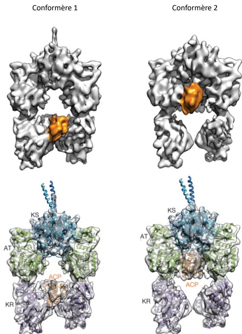
Figure 29 : Structures cryo-EM de PikAIII sous forme holo (tirée de Dutta et al., 2014). Représentation de la structure cryo-EM de PikAIII en solide ou en transparent avec les structures à haute résolution positionnées au sein de la carte EM. L'ensemble s'agence en une forme d'arche, le domaine KS homodimérique formant le dôme et les domaines AT et KR se positionnant consécutivement en dessous. L'ACP (en orange) se trouve en contact soit avec le domaine KR (en violet) (conformère 1) ou avec le domaine AT (en vert) (conformère 2).
