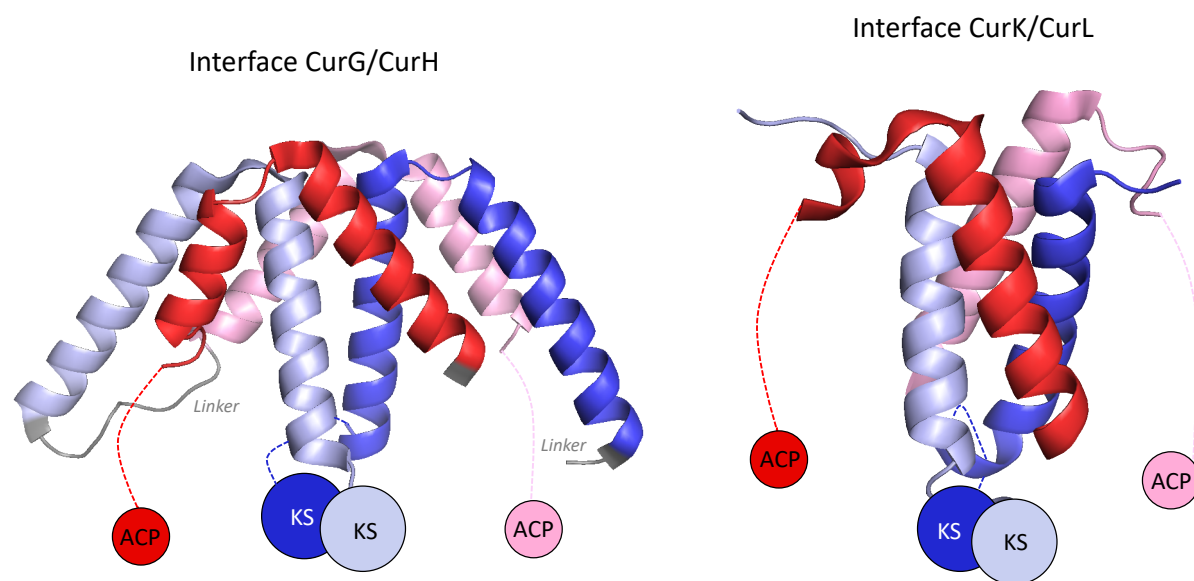
Figure 36 : Structures cristallographiques de deux interfaces de docking trouvées chez la curacine A synthase (PDB : 4MYY, 4MYZ).
