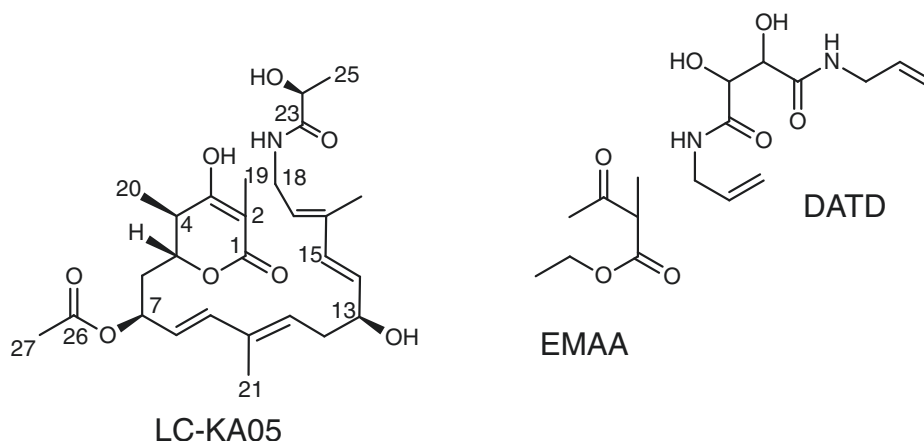
Figure 51 : Structures du substrat naturel de LkcE, LC-KA05, et des deux analogues : l'éthyl 2-méthylacétoacétate (EMAA) et le N,N'-diallyl-L-tartardiamide (DATD), utilisés pour mimer une partie de ce substrat naturel.
