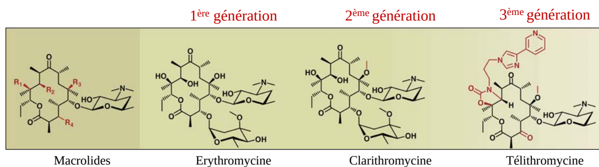
Figure 4 : Générations successives des macrolides obtenus par héli-synthèse (adaptée de Fischbach et Walsh, 2009).
