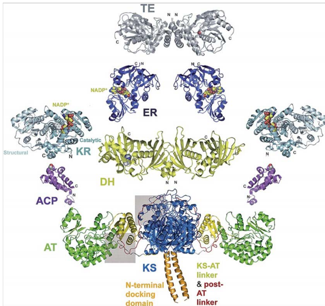
Figure 27 : Structures haute résolution de domaines individuels et de didomaines de PKS modulaires (tirée de Weissman, 2017).
