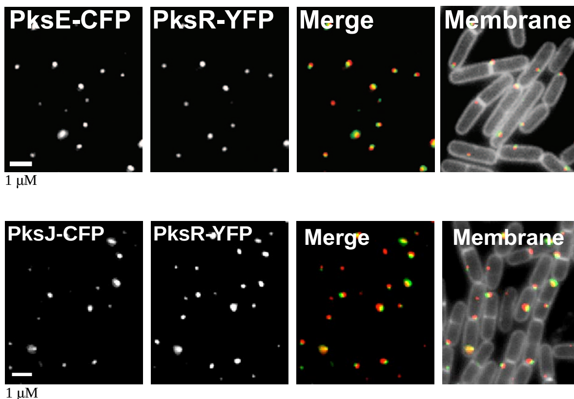
Figure 40 : Co-localisation au sein des cellules de différentes protéines impliquées dans la synthèse du bacillaène (adaptée de Straight et al., 2007).
